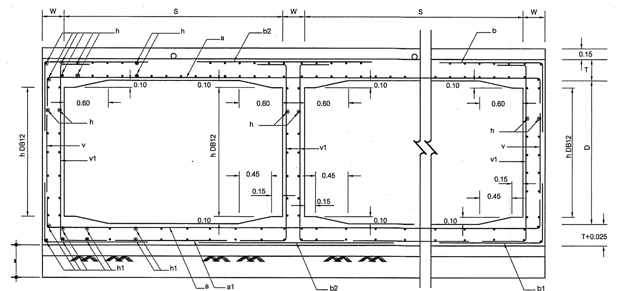
รูปตัด ๓-๓ NOT TO SCALE
