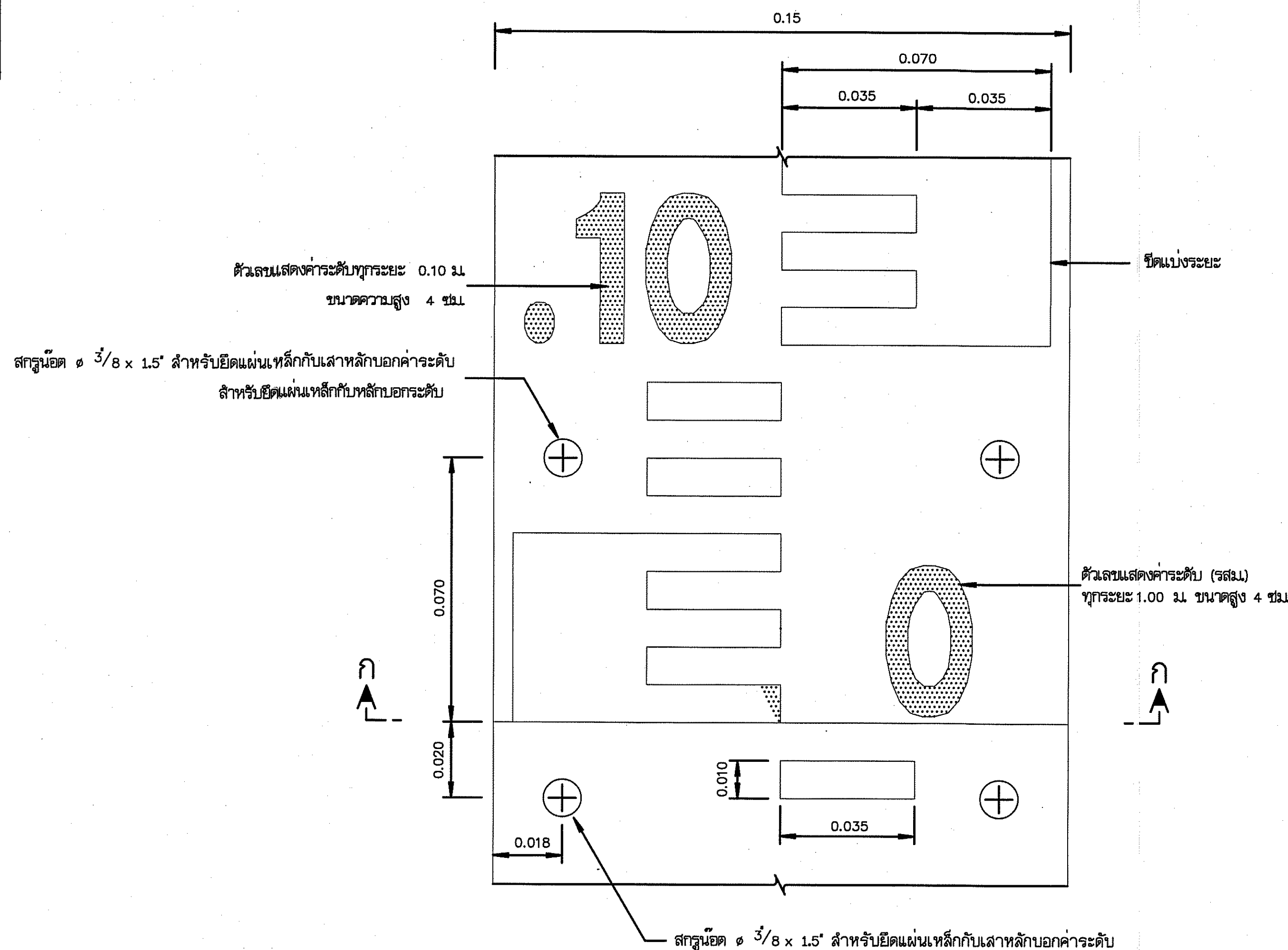
ขยายแผ่นเหล็กบอกค่าระดับ
