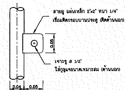
แบบขยายสายขุม ไม่แสดงภาคควาส่วน
