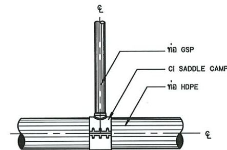
การบรรจุท่อสามทาง HDPE กับท่อ GSP แบบ CI SADDLE CLAMP (สำหรับอาคารจุดปล่อยน้ำ อาคารประจําขยะ อาคารท่อระบายอากาศ กรณีท่อส่งน้ำขนาดเส้นผ่าศูนย์กลางน้อยกว่าหรือเท่ากับ 315 มม.)
