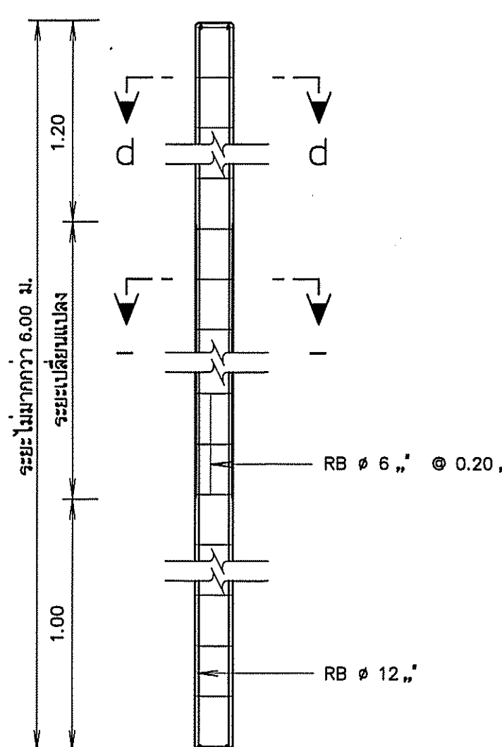
รายละเอียดเสาป้าย ศสล. มาตราส่วน 1:20
