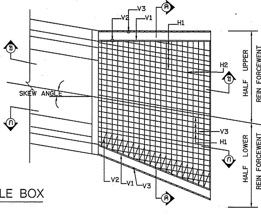
รูปตัด ๘ NOT TO SCALE
