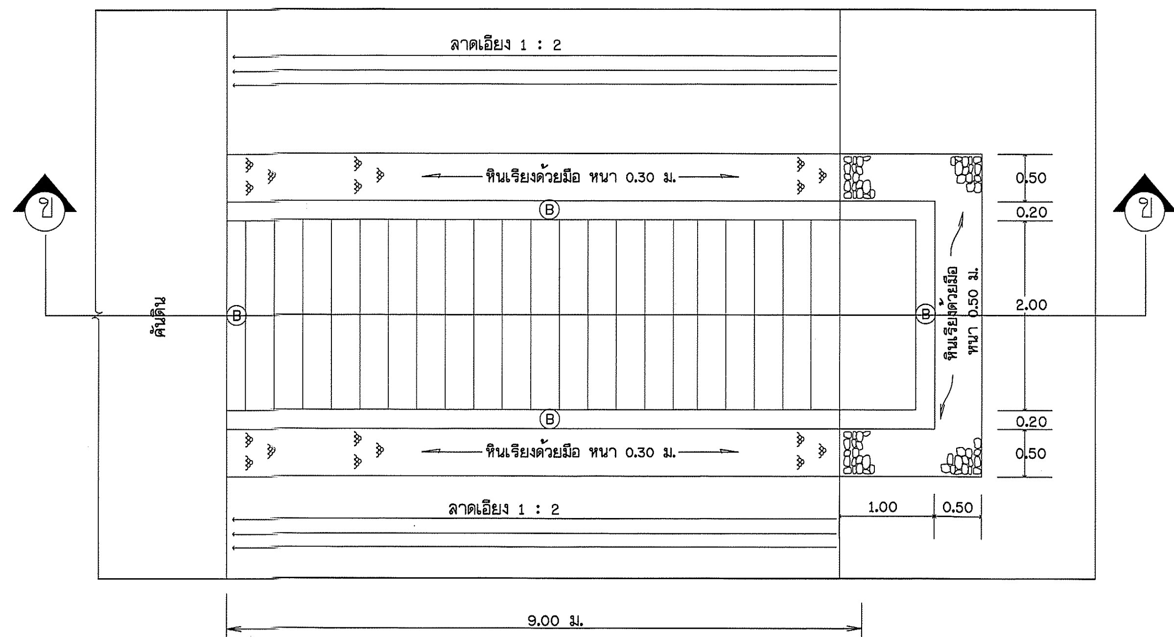
แปลนบันได คสล. แบบไม่มีชันพัก ไม่แสดงมาตราส่วน
