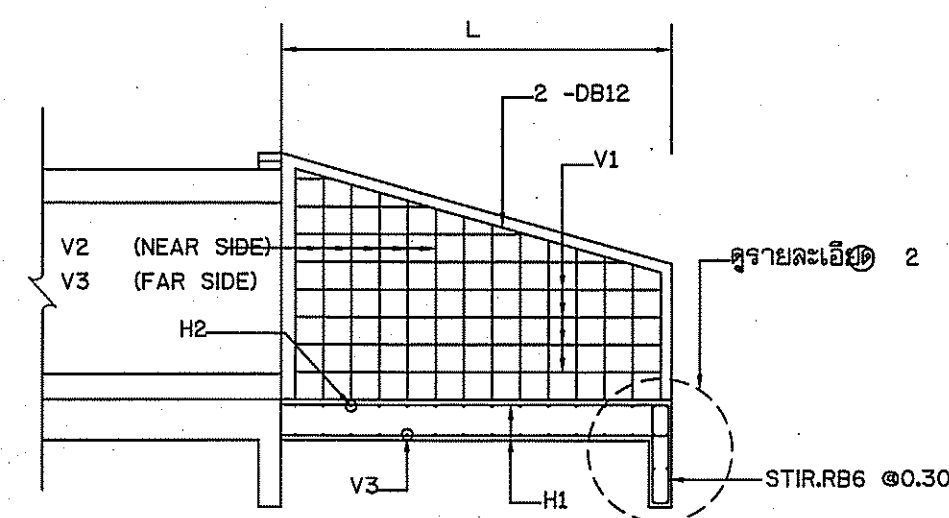
รูปตัด ๒ NOT TO SCALE
