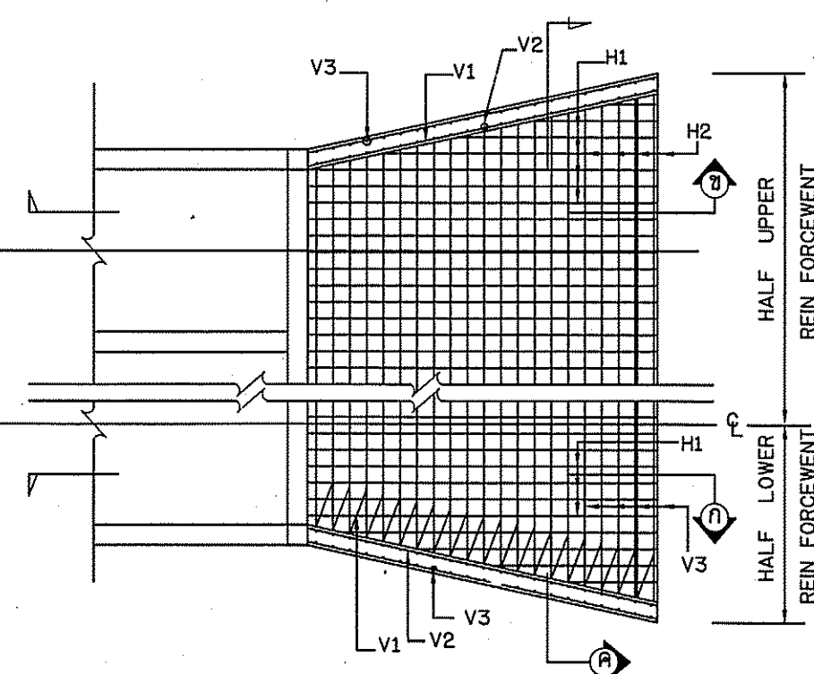
รูปตัด ๖ NOT TO SCALE
