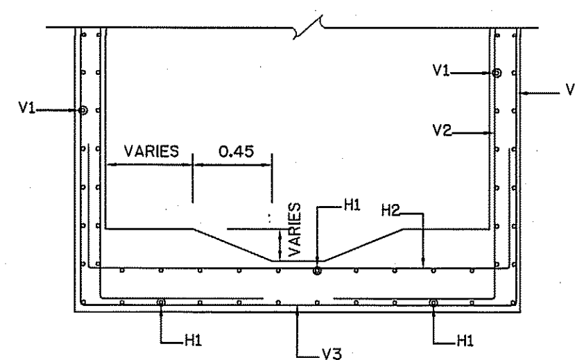
รูปตัด ๑๕ NOT TO SCALE
