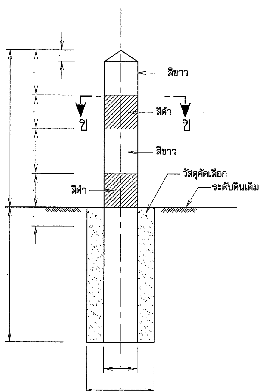
หลักริมคันดิน
