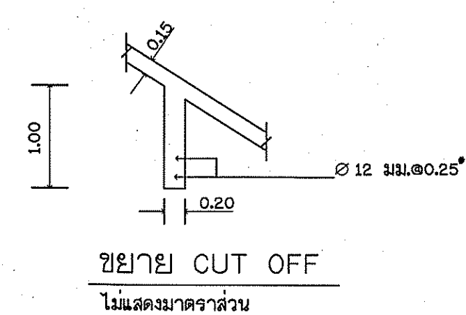
รูปตัด (ก) - (ก) (ความหนาพื้น 0.15 ม.) ไม่แสดงมาตราส่วน
