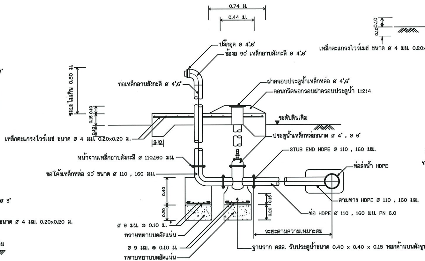
รูปตัด ข - ข แสดงการติดตั้งประตูระบายตะกอน
