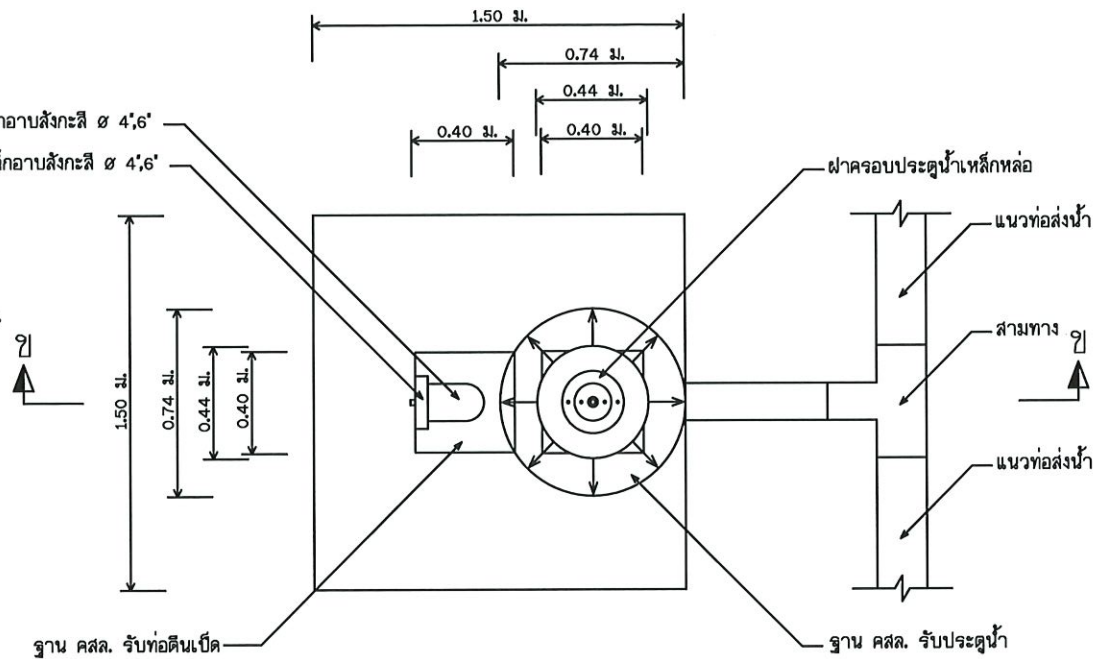
แปลนประตูระบายตะกอน
