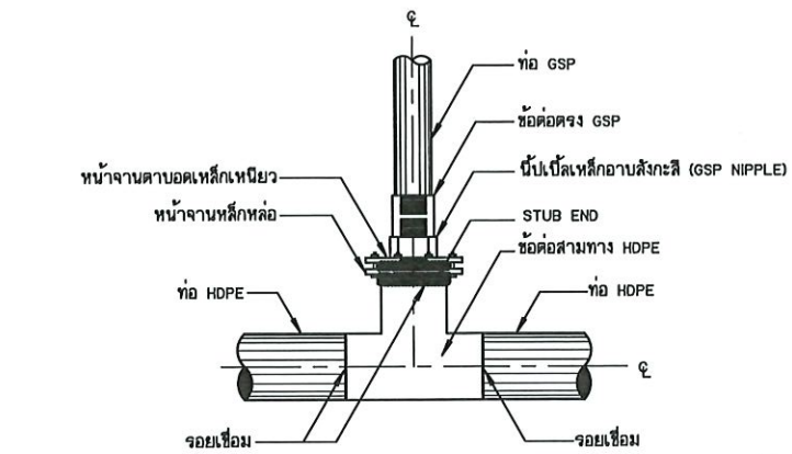
การบรรจุท่อสามทาง HDPE กับท่อ GSP แบบข้อต่อ (สำหรับอาคารจุดปล่อยน้ำ อาคารประจําขยะ อาคารท่อระบายอากาศ กรณีท่อส่งน้ำขนาดเส้นผ่าศูนย์กลางมากกว่า 315 มม.)
