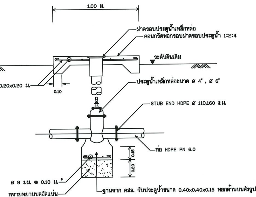
รูปตัด ค - ค แสดงการติดตั้งประตูปะยายตะกอน มาตราส่วน No Scale
