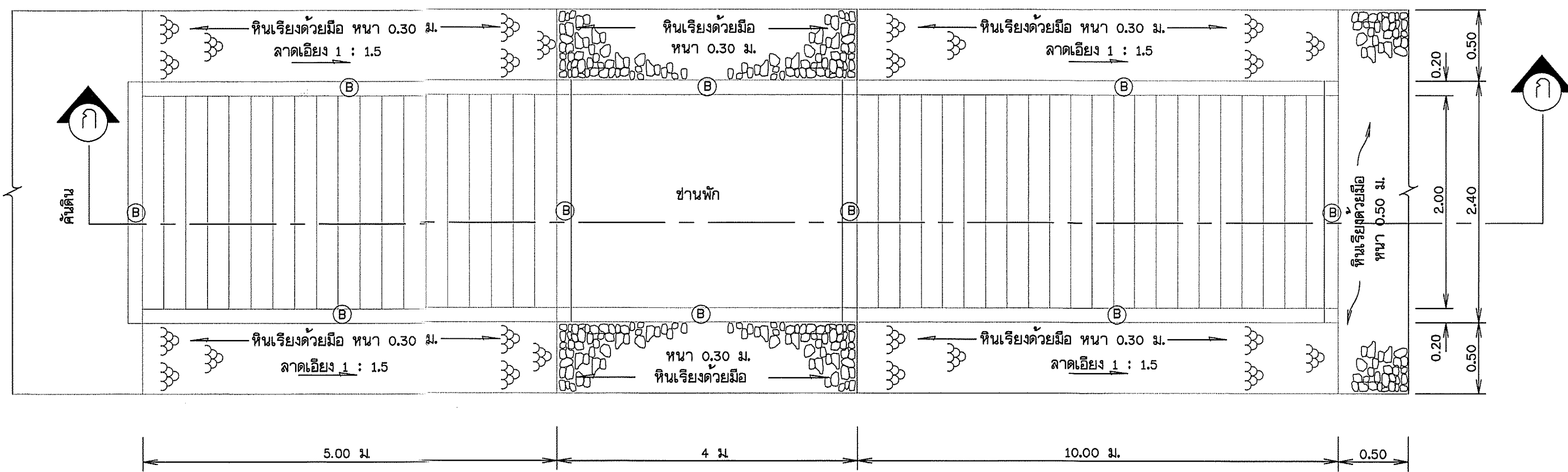
แปลนบ้านโต คสล. แบบมีชานพัก ไม่แสดงมาตราส่วน
