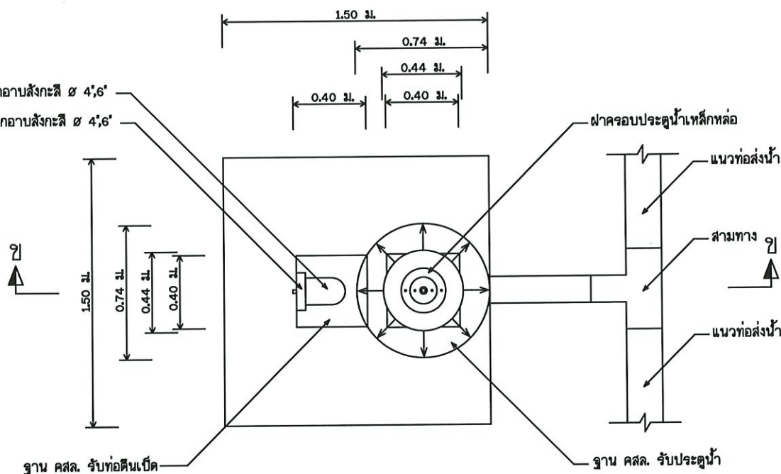
แปลนประตูปะยายตะกอน มาตราส่วน No Scale
