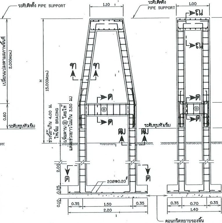
คอม่อรับท่อแบบที่ 2
