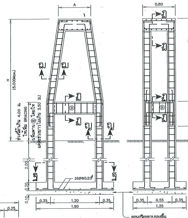
คอม่อรับท่อแบบที่ 1
