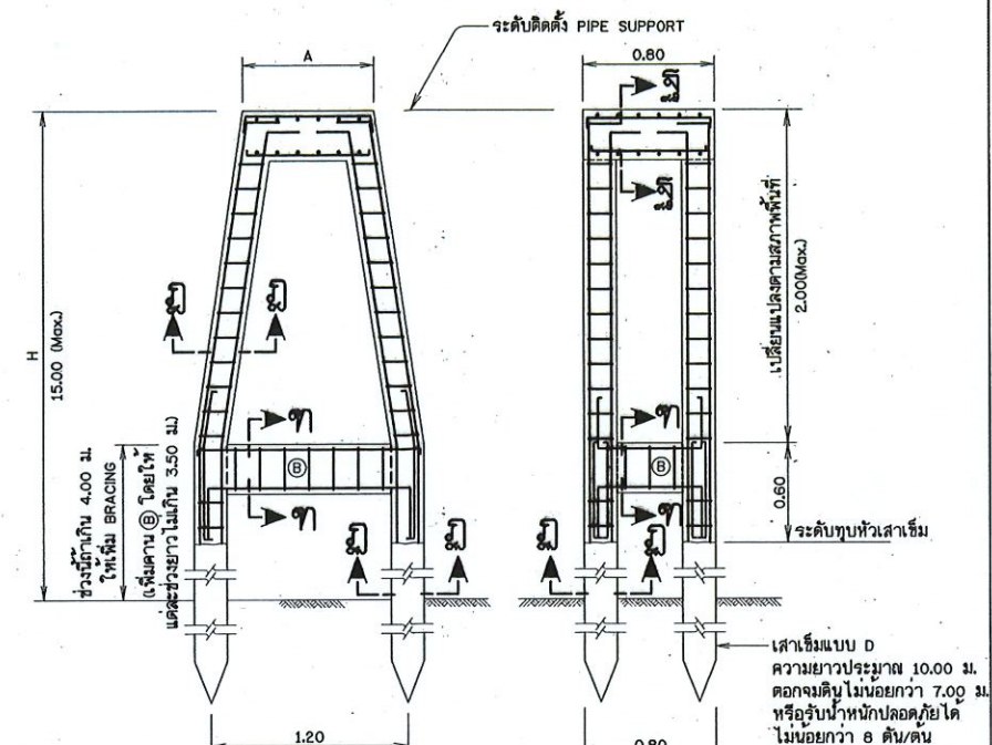
รูปตัดตามขวาง
