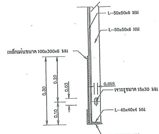
รูปด้านตั้ง (ไม่แสดงเหล็กฉาก)
