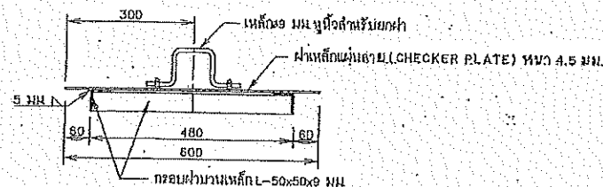
รูปตัด ข-ข
