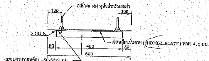
รูปตัด จ-จ
