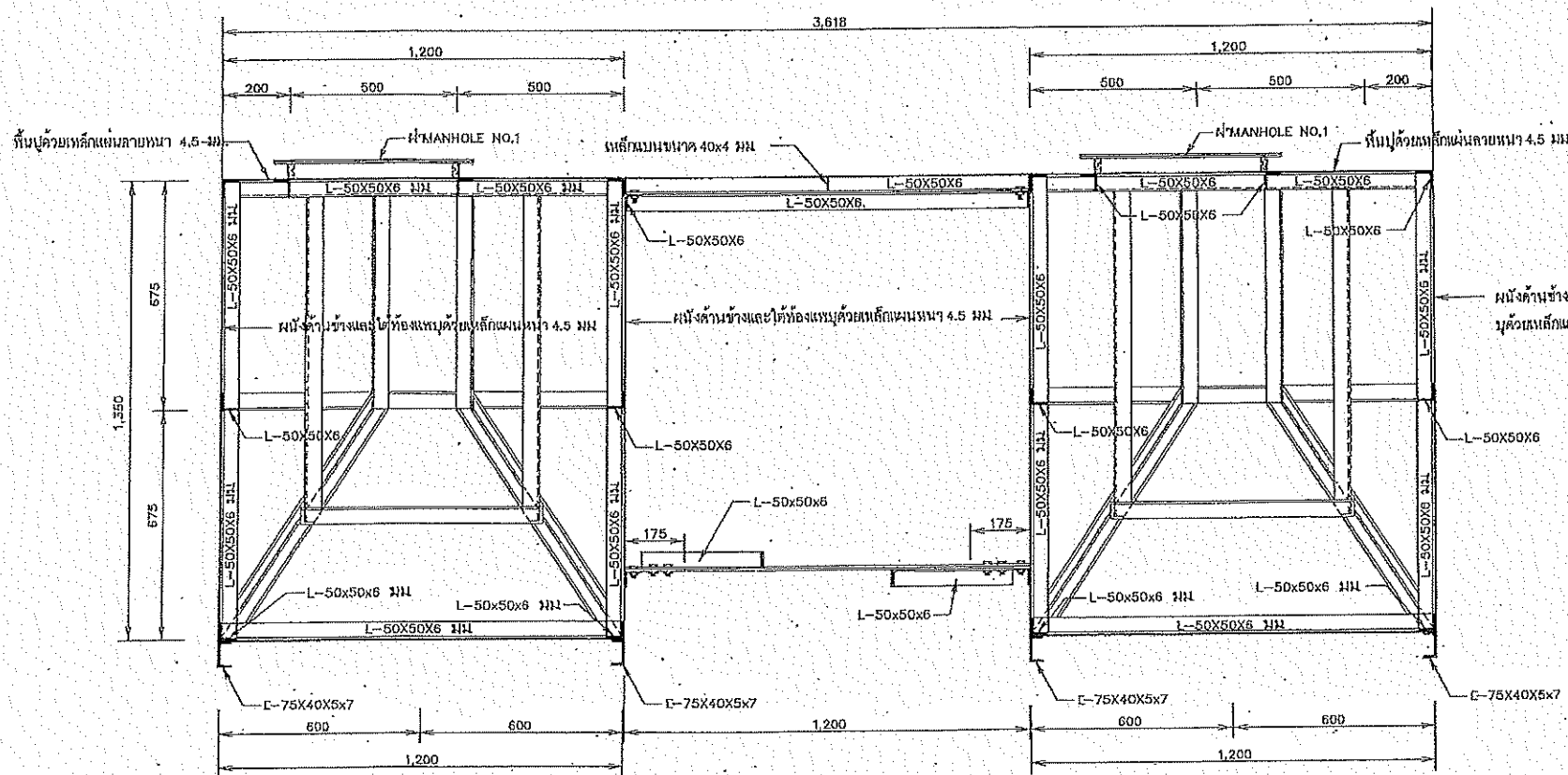
รูปตัด ง - ง
