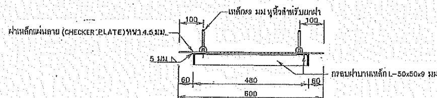
รูปตัด ด-ด
