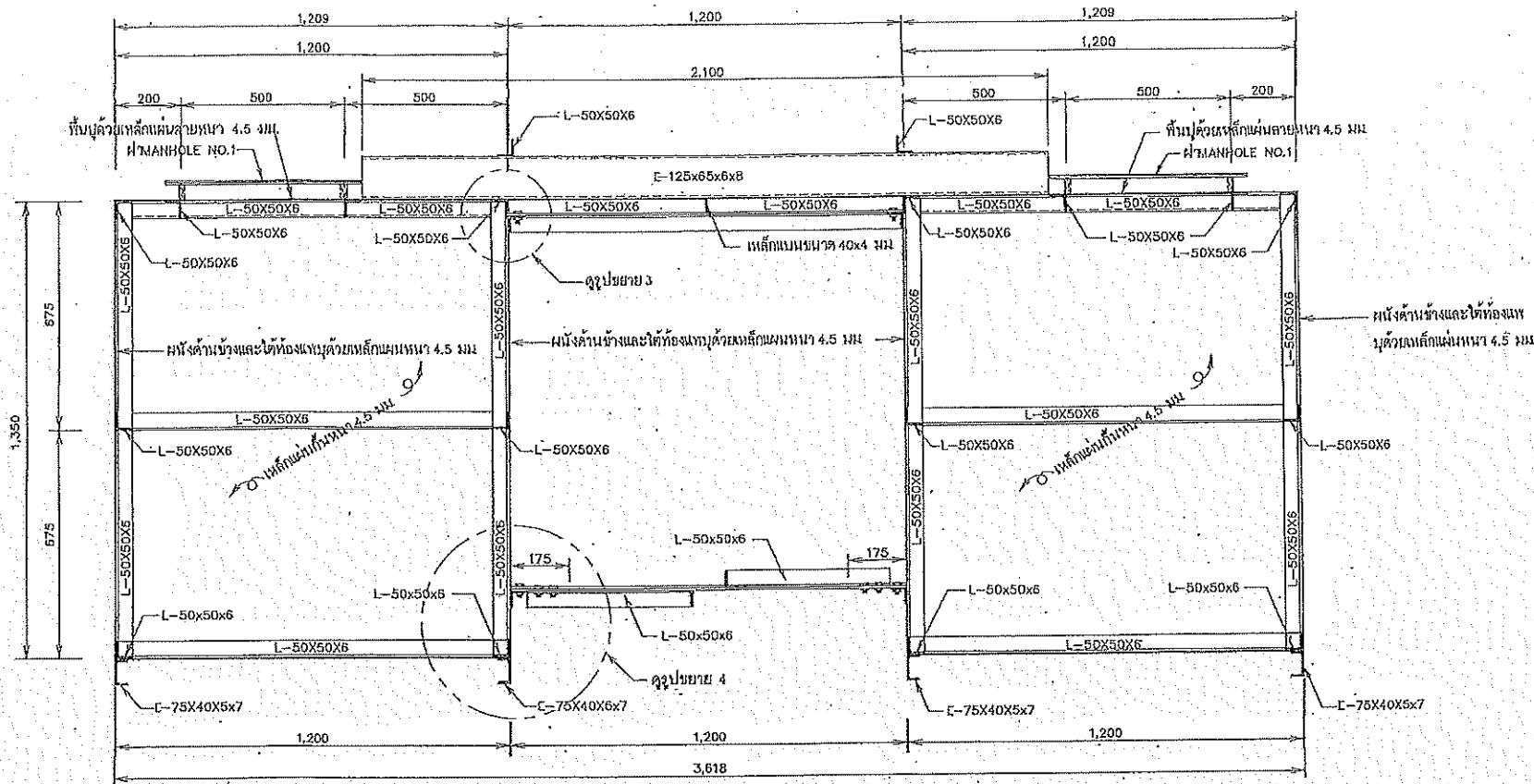
รูปตัด ค - ค
