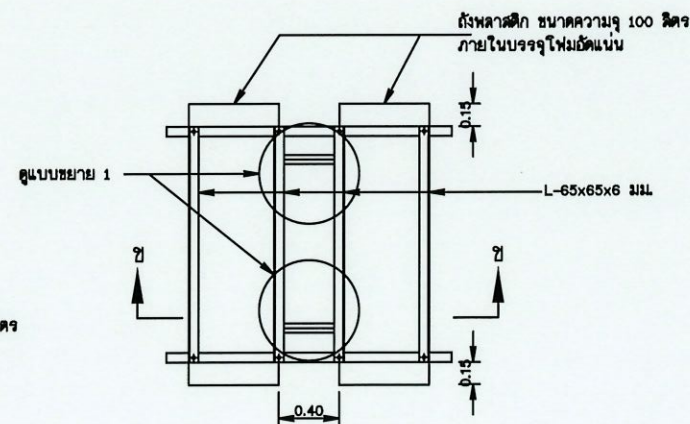
ทุ่นรับท่อวางตัวนอน
