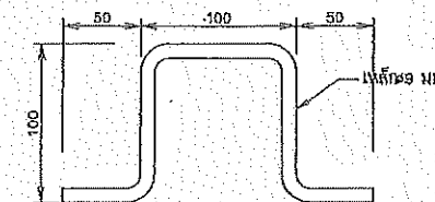
รูปขยายเหล็กหัวหัว MANHOLE
