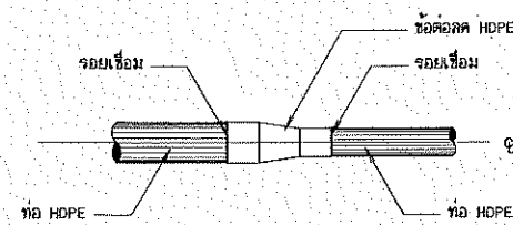
การบรรจุท่อ HDPE กับข้อต่อคดท่อ HDPE
