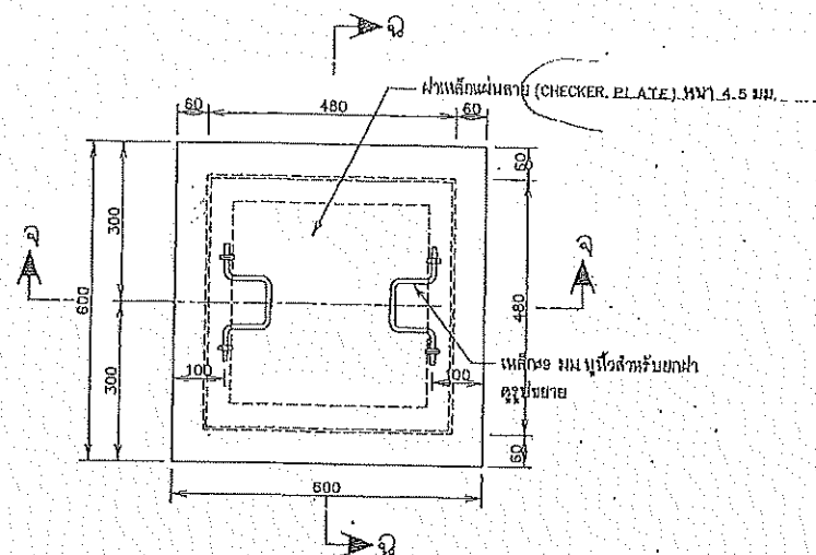
แปลน MANHOLE NO.1
