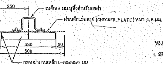
รูปตัด ฟ-ฟ
