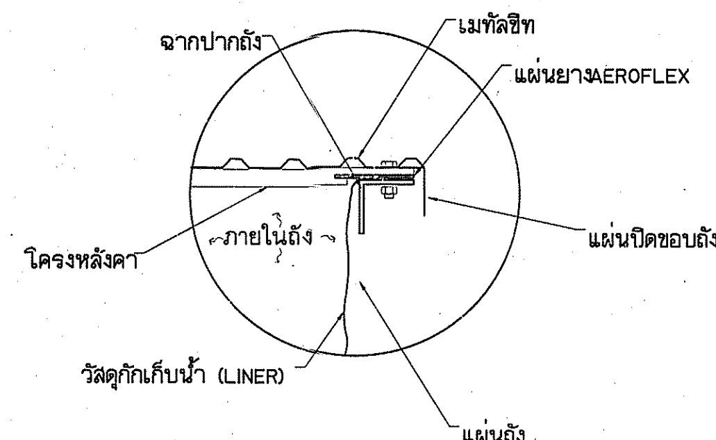
แบบขยาย 3- จุดยึดหลังคาถึงแผ่นถึง Scale NTC.
