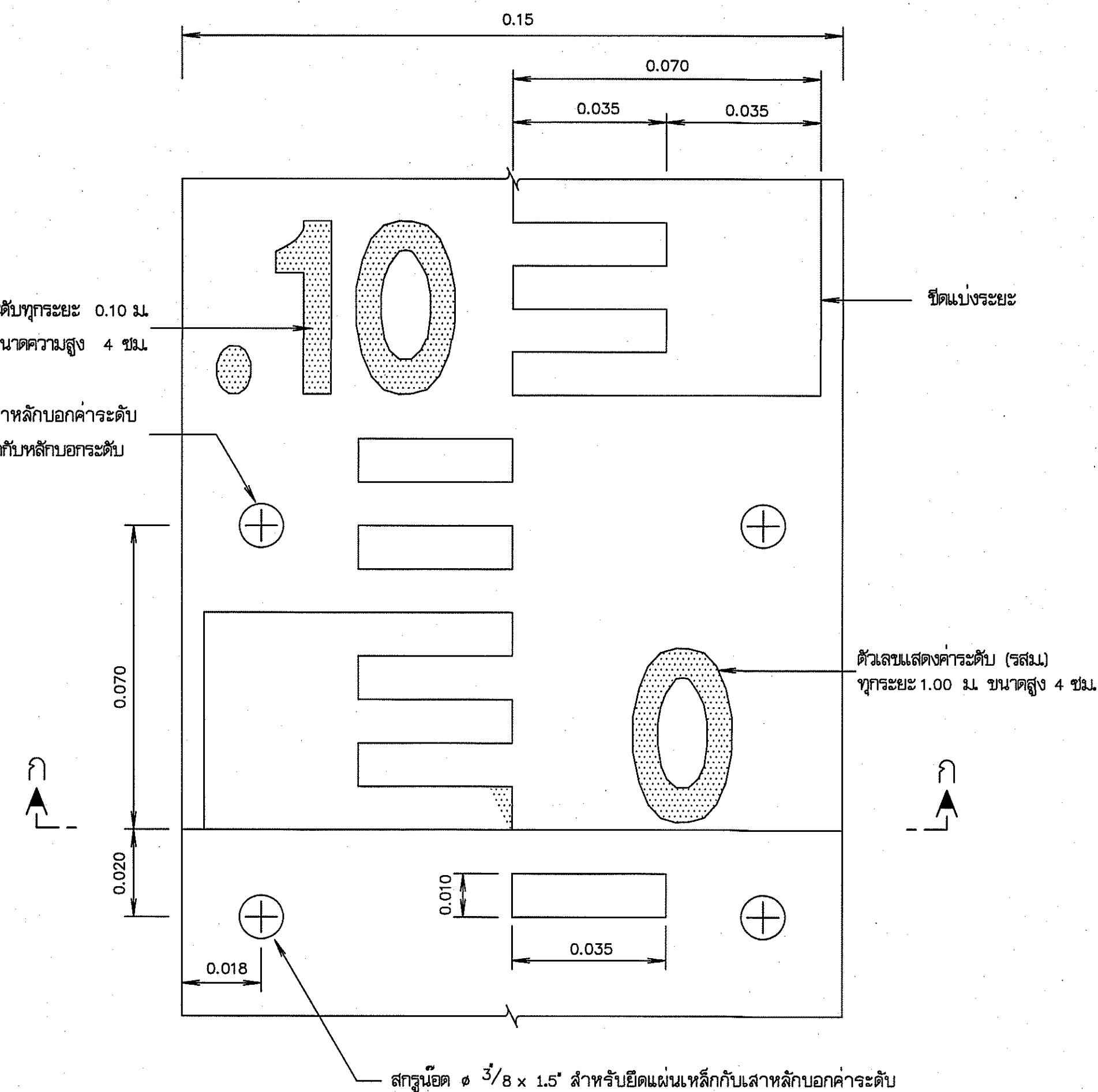
ขยายแผ่นหลักบอกระดับ
