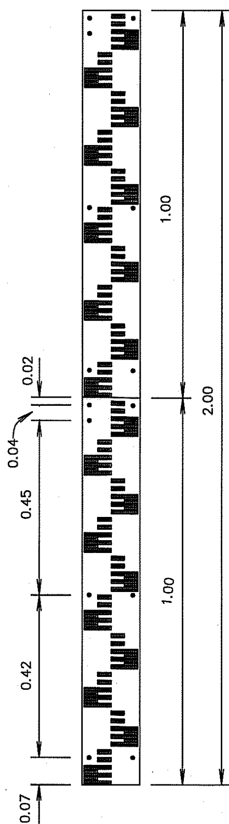
แผ่นหลักบอกระดับ
