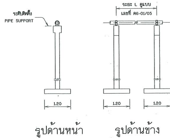
คอมม่อรับท่อแบบที่ 1
