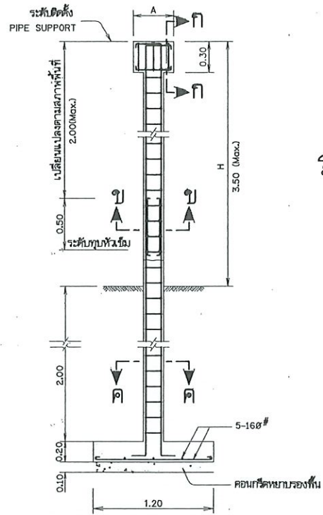
การเสริมเหล็ก คอมม่อแบบที่ 1
