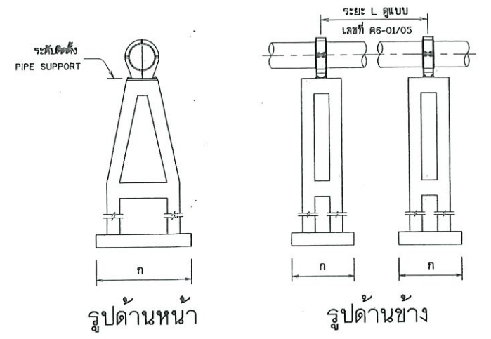
คอมม่อรับท่อแบบที่ 3,4
