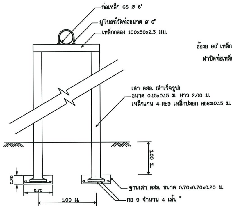
ขยายเสาร์ป๋อส่งน้ำ
