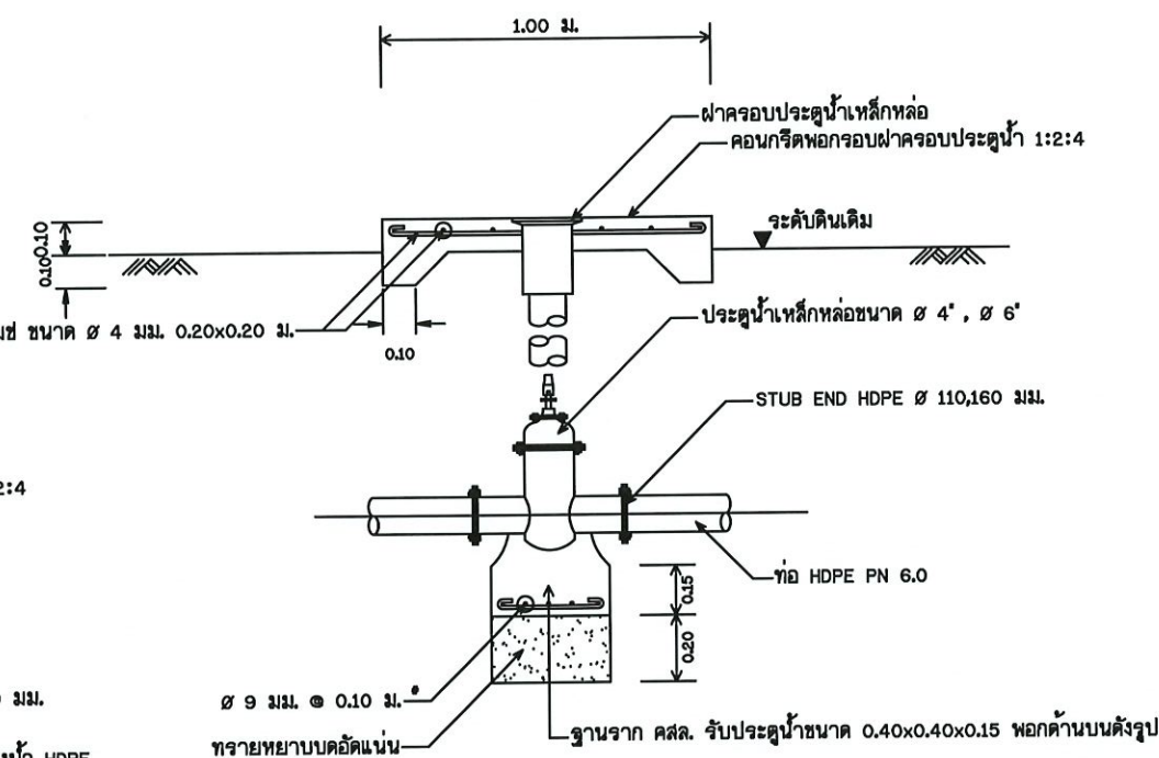
รูปตัด ค - ค แสดงการติดตั้งประตุน้ำใต้ดิน
