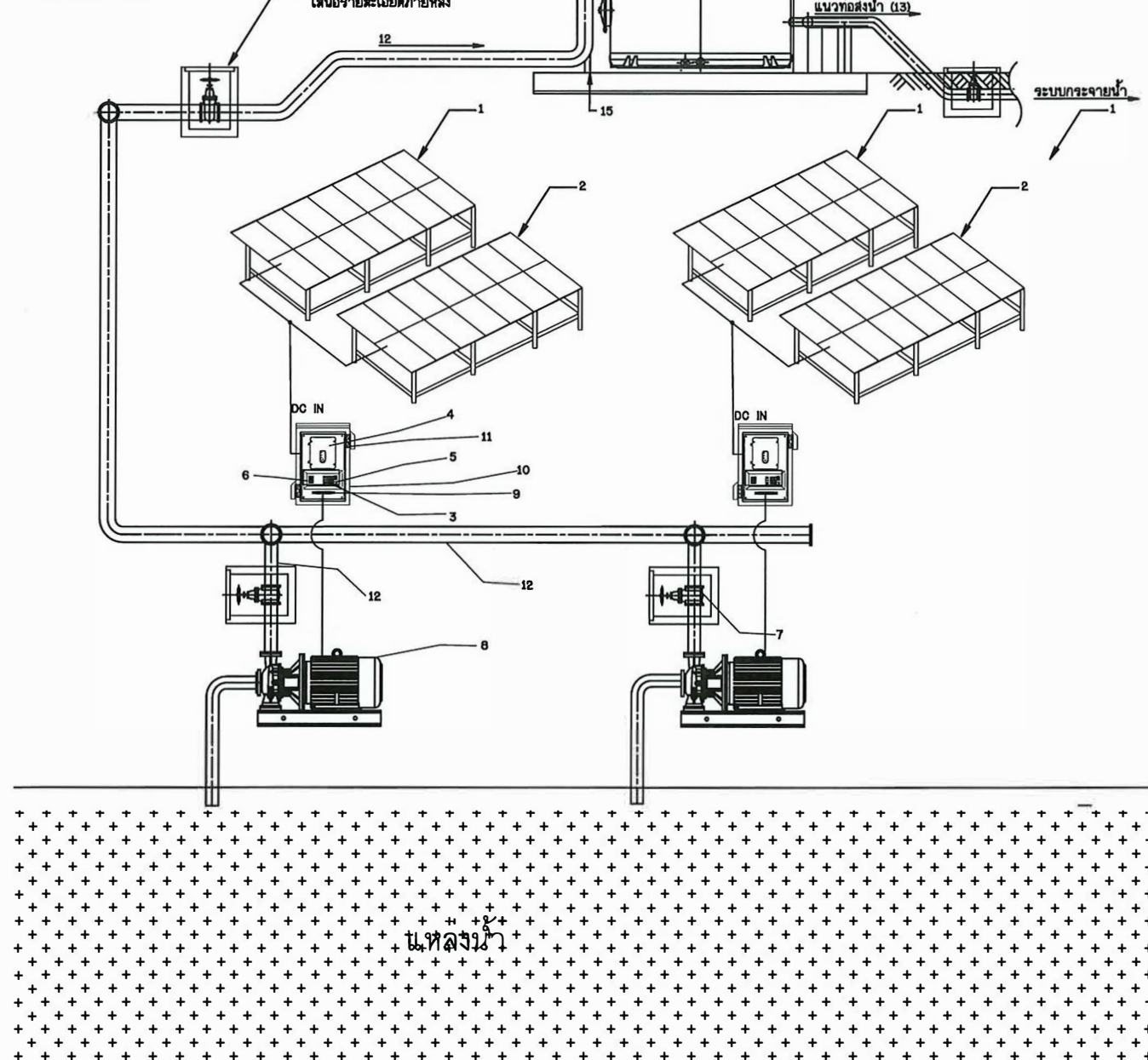
แบบระบบกระจายน้ำด้วยพลังงานแสงอาทิตย์ มาตรฐาน โมเดลมาตรฐาน
