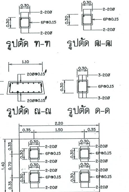
รูปตัด ด-ด
