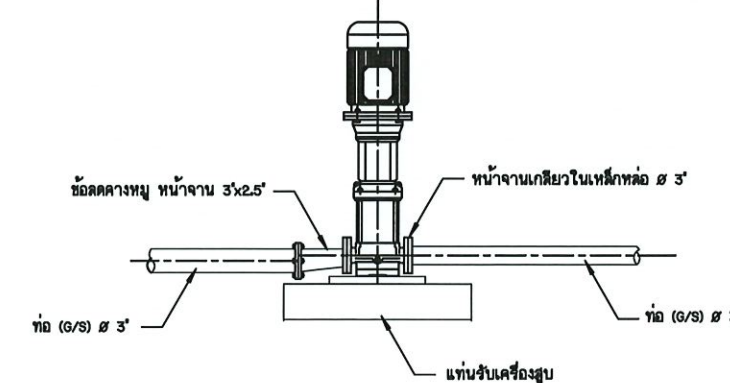
การต่อท่อเครื่องสูบน้ำ ไม่แสดงมาตราส่วน
