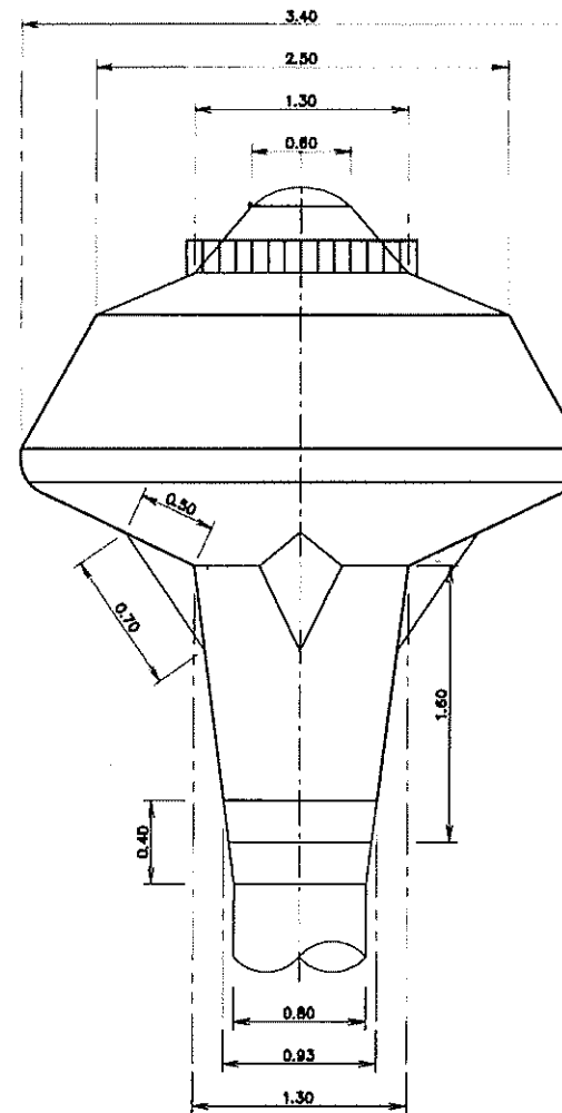
แบบขยายแมนโฮลบนของถังสูง ไม่แสดงมาตราส่วน
