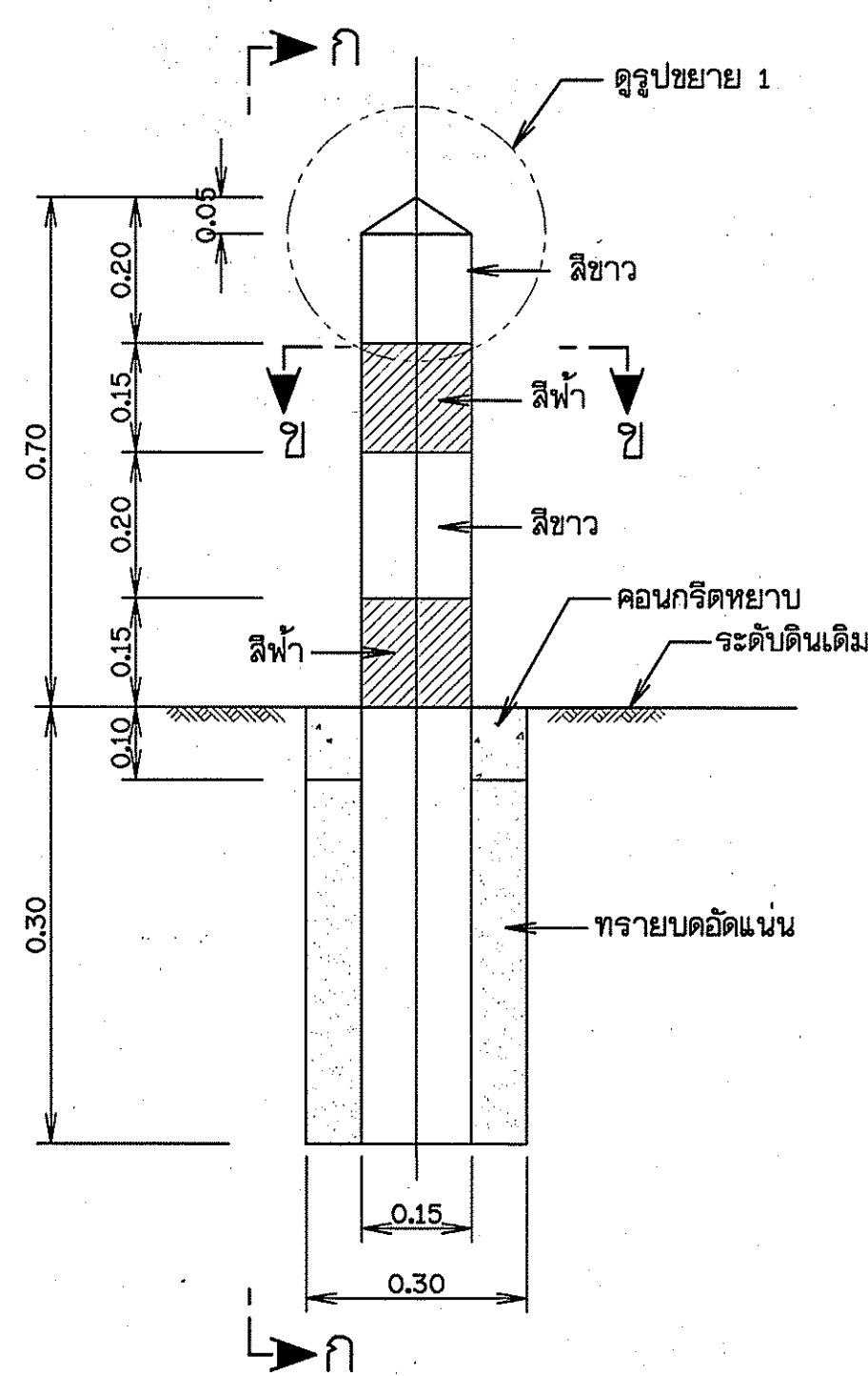
เสาส.ค.ส. แสดงแนวท่อส่งน้ำ
