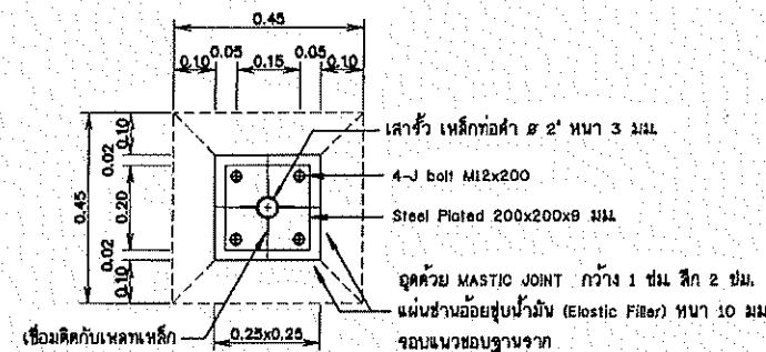
รูปตัด ข-ข ไม่แสดงขนาดจริง
