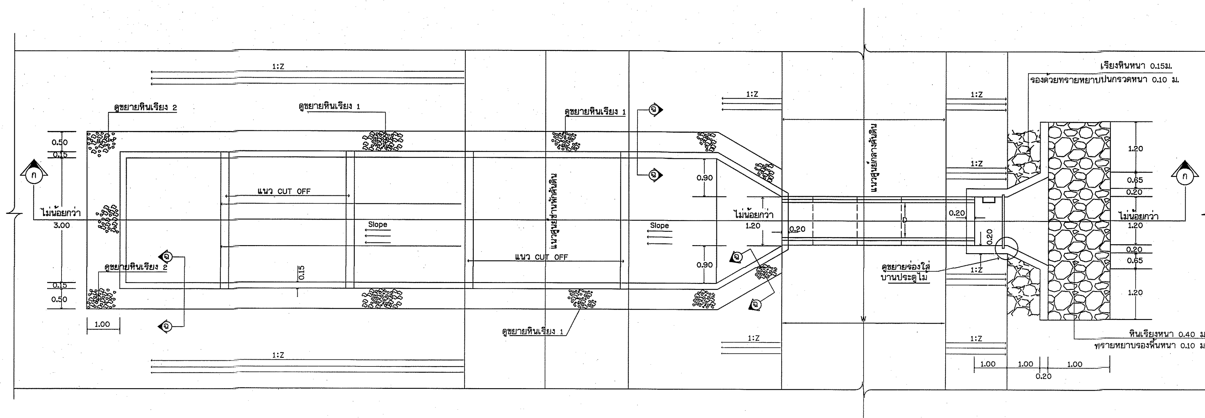
แปลนอาคารทางน้ำออก ไม่แสดงมาตราส่วน
