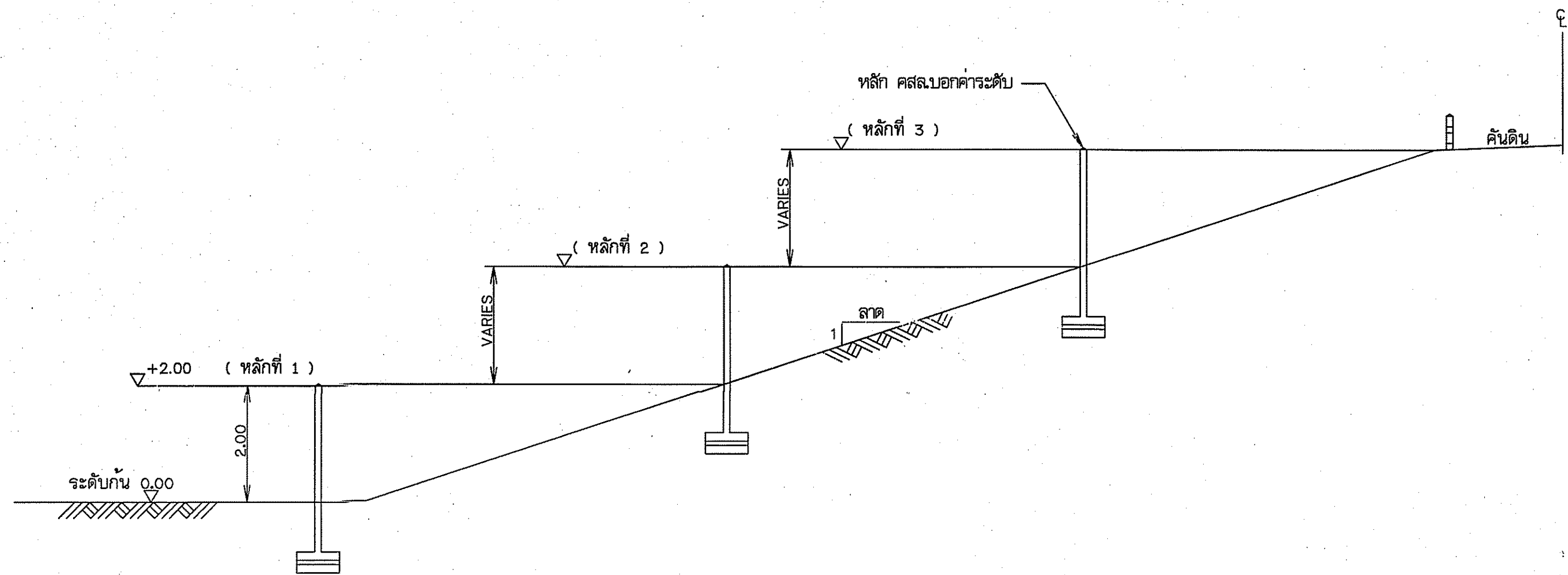
รูปตัดทั่วไปแสดงตำแหน่งหลักบอการค้าระดับน้ำ ไม่แสดงขนาดราส่วน
