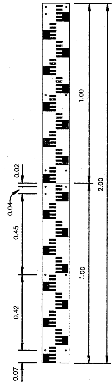
แผ่นหลักบอกระดับ มาตราส่วน 1:10
