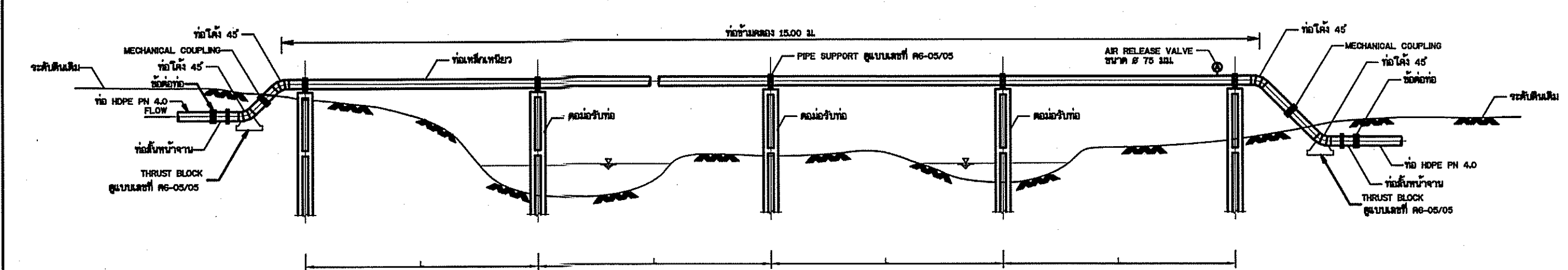
แบบขยายการวางท่อข้ามห้วย มาตราส่วน No Scale
