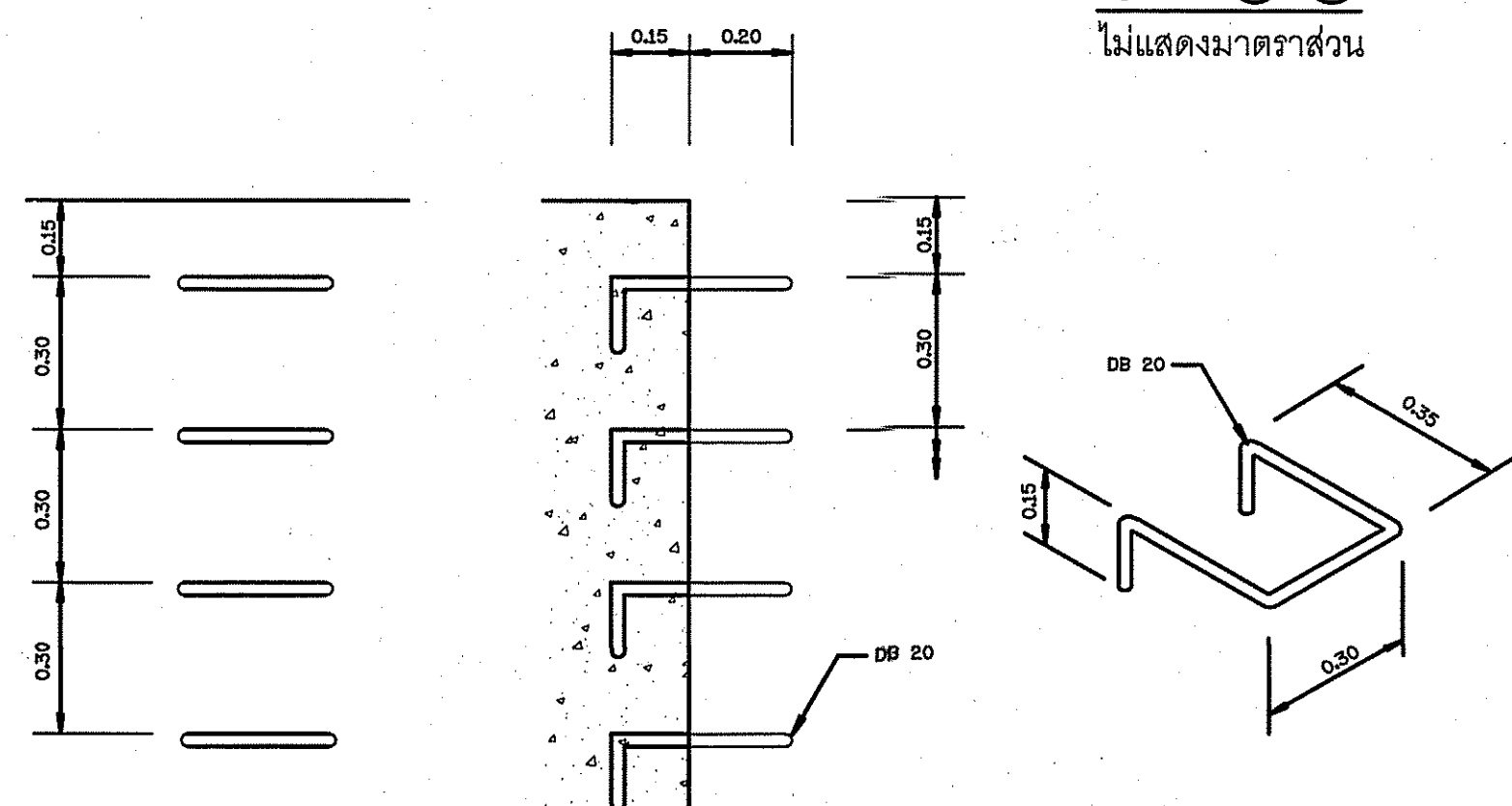
รูปขยายบันไดลิง ไม่แสดงมาตราส่วน
