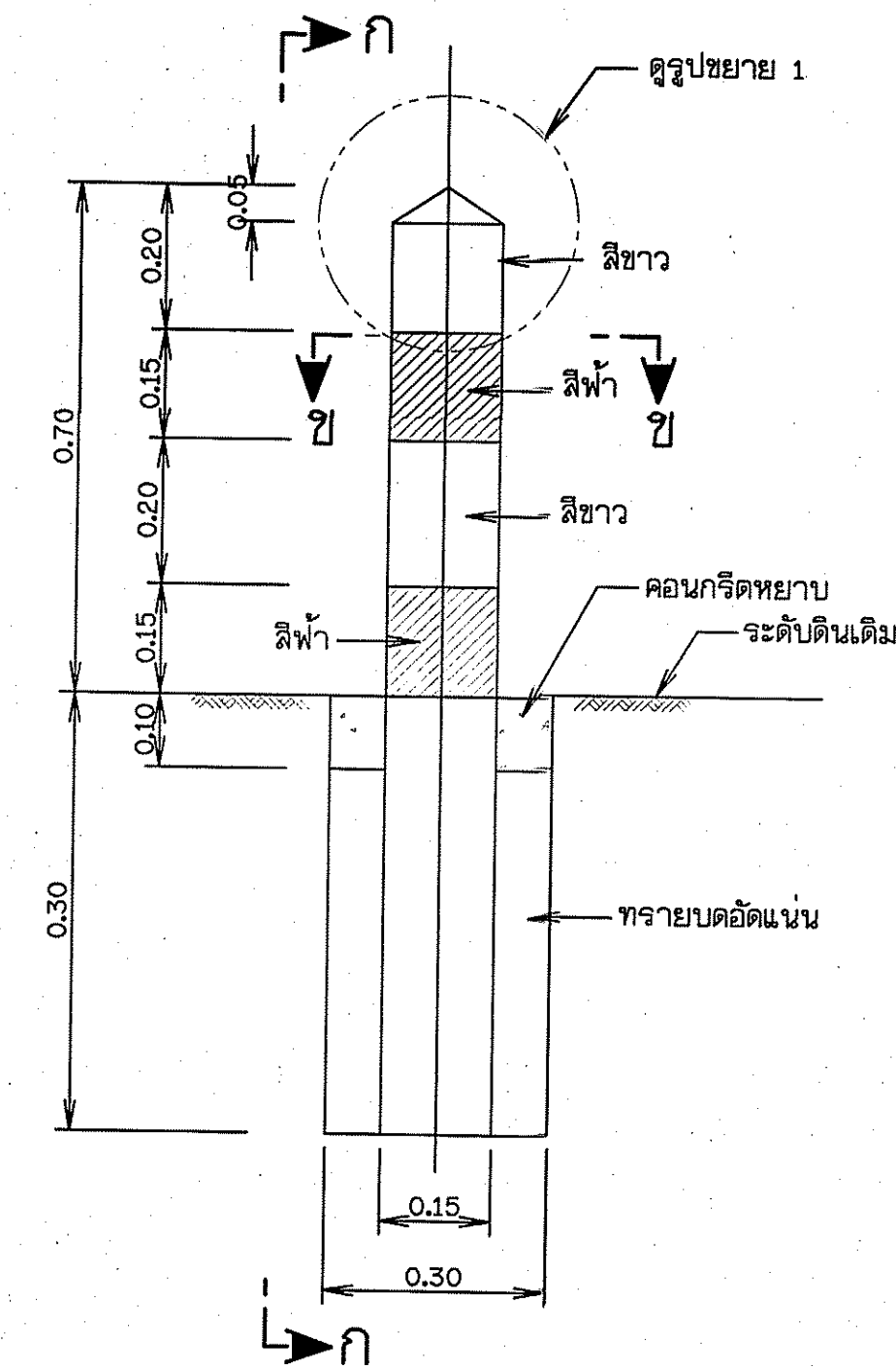
เสา ค.ส.ล. แสดงแนวท่อส่งน้ำ
