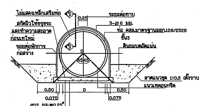
รูปตัดการวางท่อ คล.ล. ไม่แสดงมาตราส่วน
