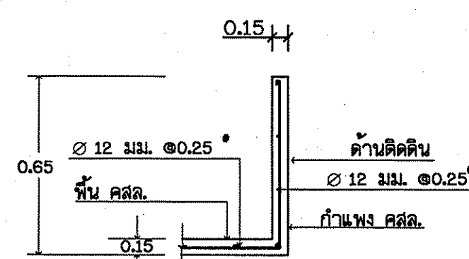
รูปตัด ก-ก (ความหนาพื้น 0.15 ม.) ไม่แสดงมาตราส่วน
