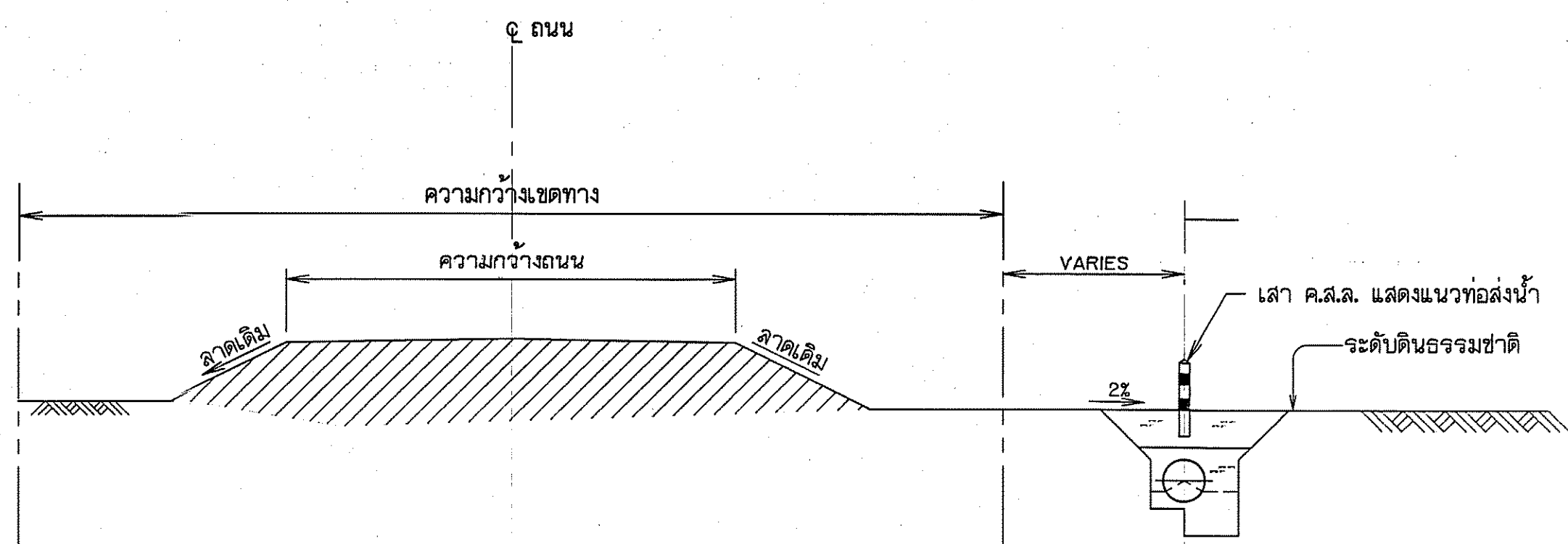
รูปตัดแสดงการวางท่อส่งน้ำ ไม่แสดงมาตราส่วน
