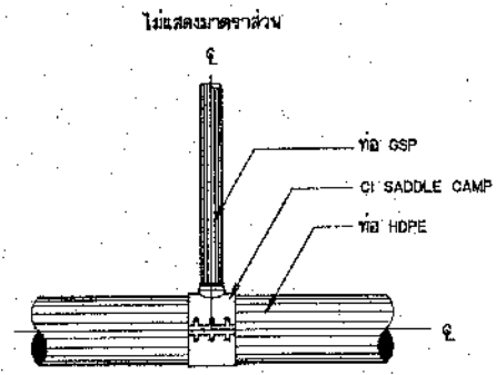
การบรรจุท่อสามทาง HDPE กับท่อ GSP แบบ CI SADDLE CLAMP (สำหรับอาคารชุดปล่อยน้ำ อาคารประจวบประจวบตอน อาคารท่อระบายอากาศ กรณีท่อส่งน้ำขนาดเส้นผ่าศูนย์กลางน้อยกว่าหรือเท่ากับ 315 มม.)
