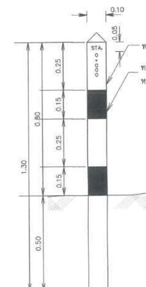
แสดงสัดส่วนหลักบอกแนวท่อ
