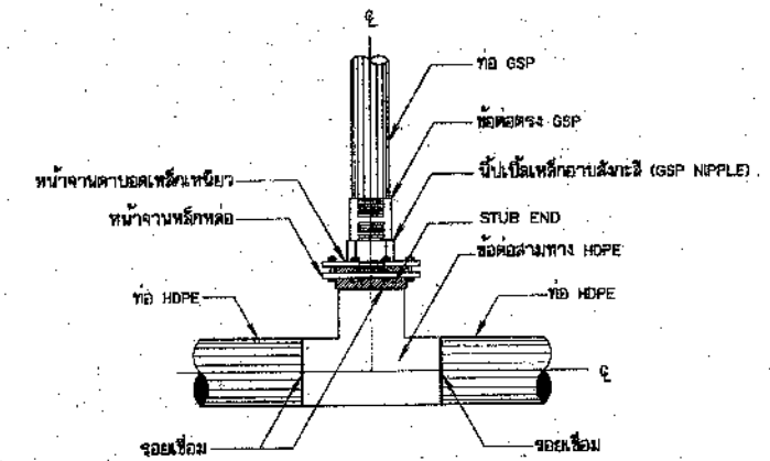
การบรรจุท่อสามทาง HDPE กับท่อ GSP แบบข้อต่อ (สำหรับอาคารชุดปล่อยน้ำ อาคารประจวบประจวบตอน อาคารท่อระบายอากาศ กรณีท่อส่งน้ำขนาดเส้นผ่าศูนย์กลางน้อยกว่า 315 มม.)
