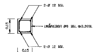
รูปตัด ก - ก
