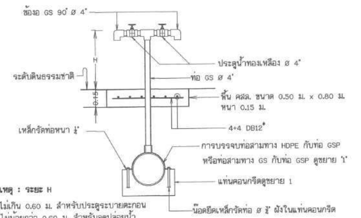
รูปตัดอาคารจุดปล่อยน้ำ 2 ด้าน
