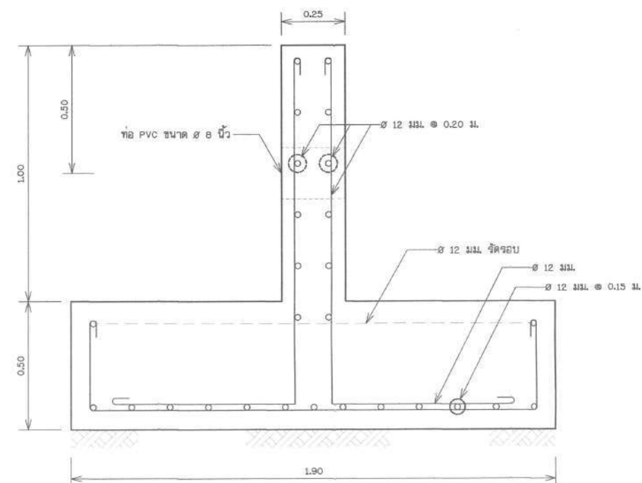
แสดงการเสริมเหล็ก
