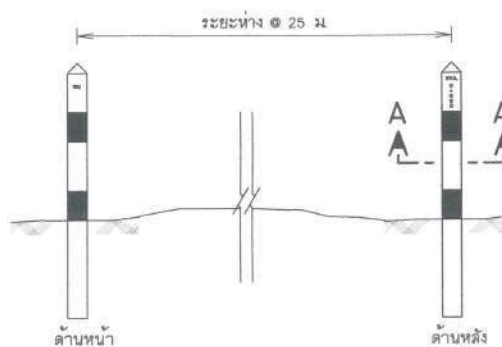
แสดงการวางหลักบอกแนวท่อ
