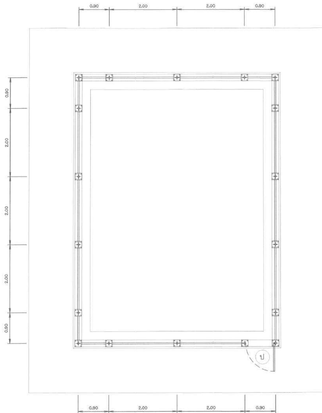
แบบแปลนรั้วลวดตาข่าย (ถึงเก็บน้ำ-ถึงพิกน้ำขนาดความจุไม่น้อยกว่า 100 ลบ.ม.)
