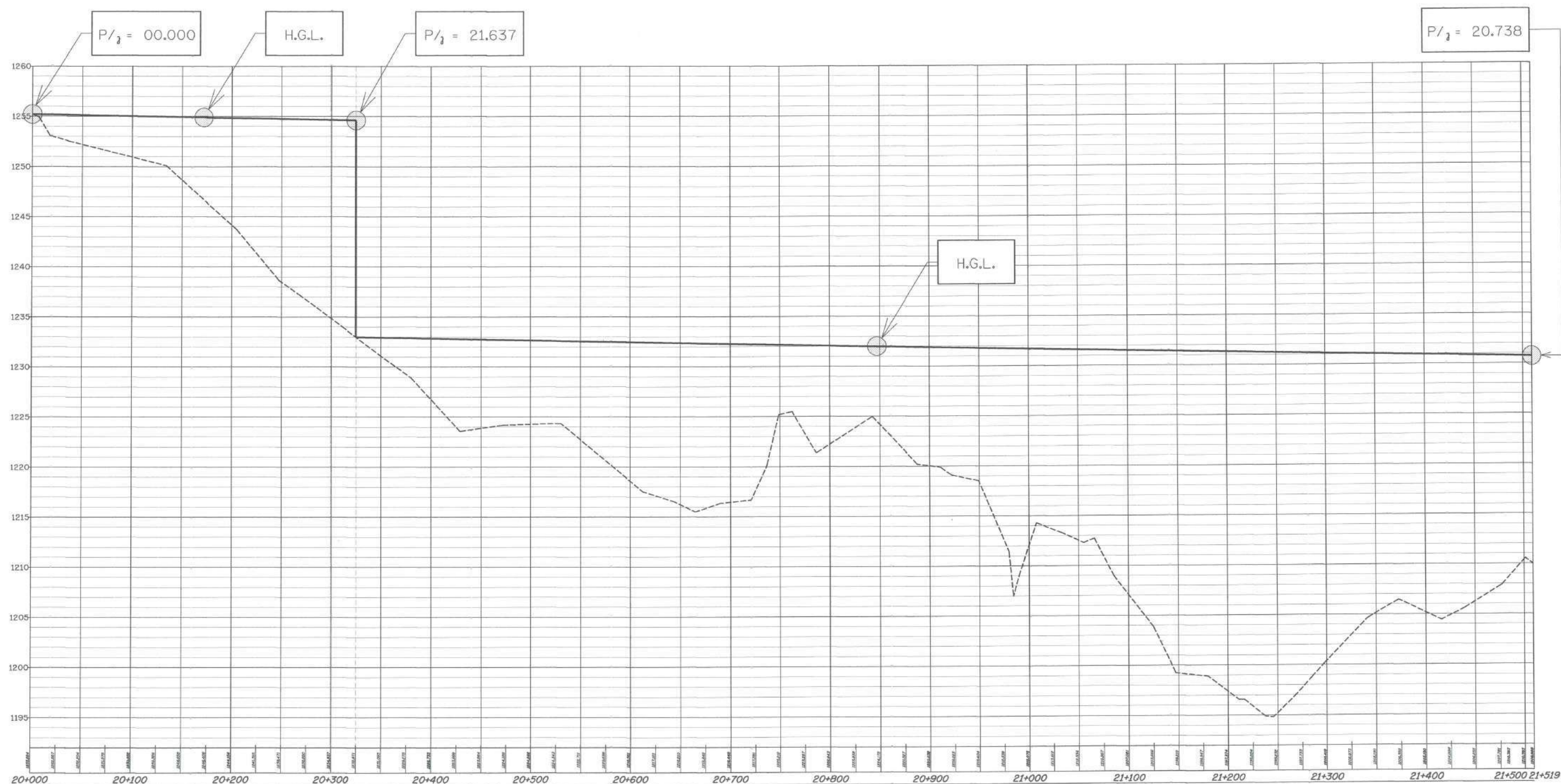
รูปตัดตามแนวยาวแสดง H.G.L. สาย RMP STA. 20+000 - 21+519
