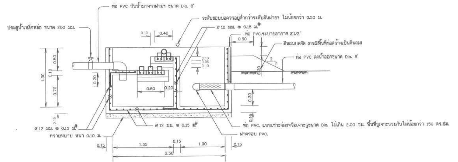
รูปตัด ฅ - ฅ
