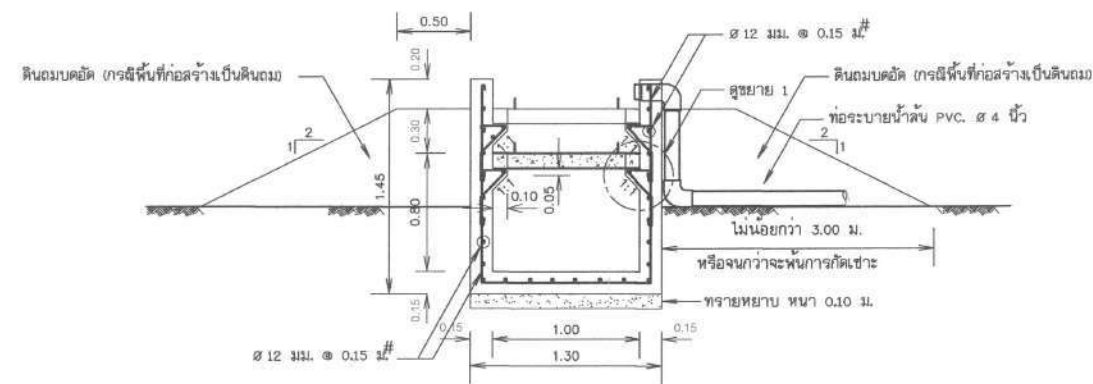
รูปตัด ฅ - ฅ
