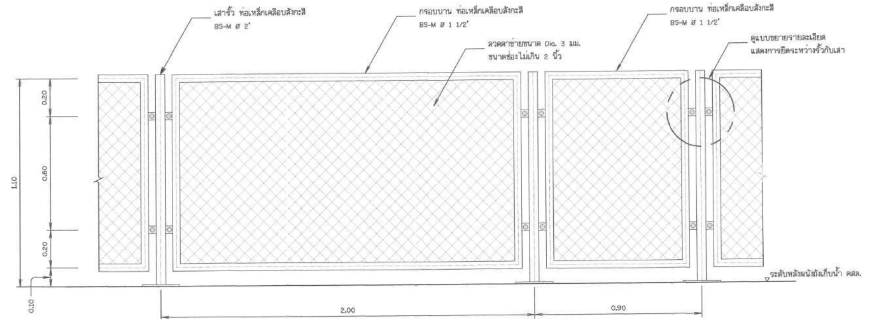
แบบขยายราวกันตก
