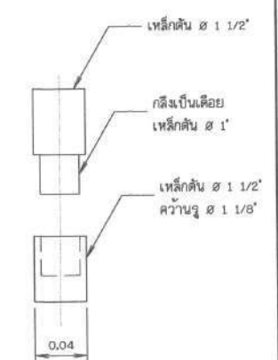
แบบขยายบานพับประตูเหล็ก
