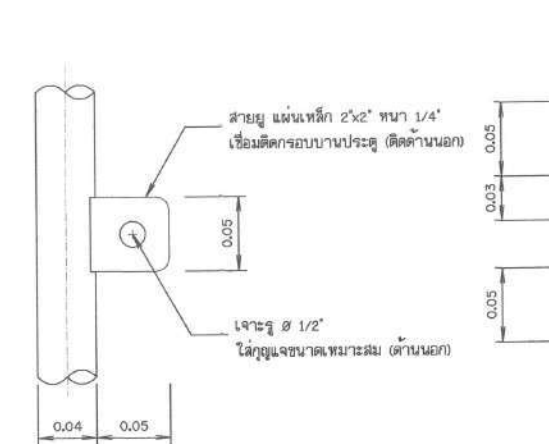
แบบขยายสายยู
