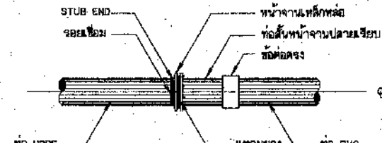
การบรรจุท่อ HDPE กับท่อ PVC. ไม่แสดงมาตราส่วน
