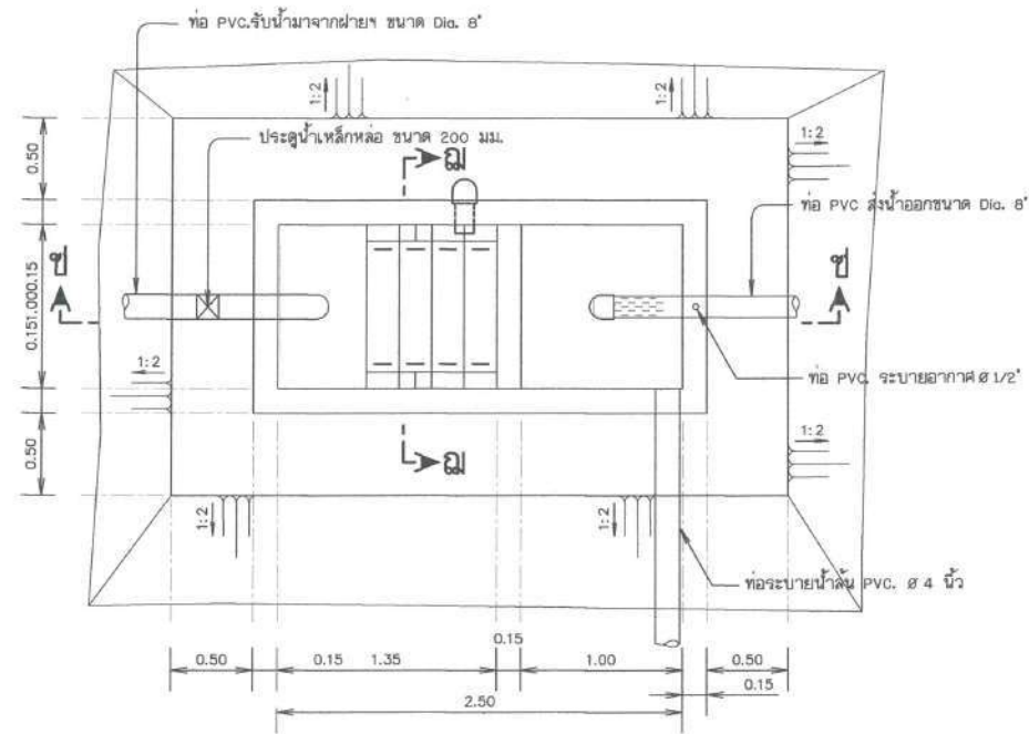
แปลนบ่อตกตะกอน
