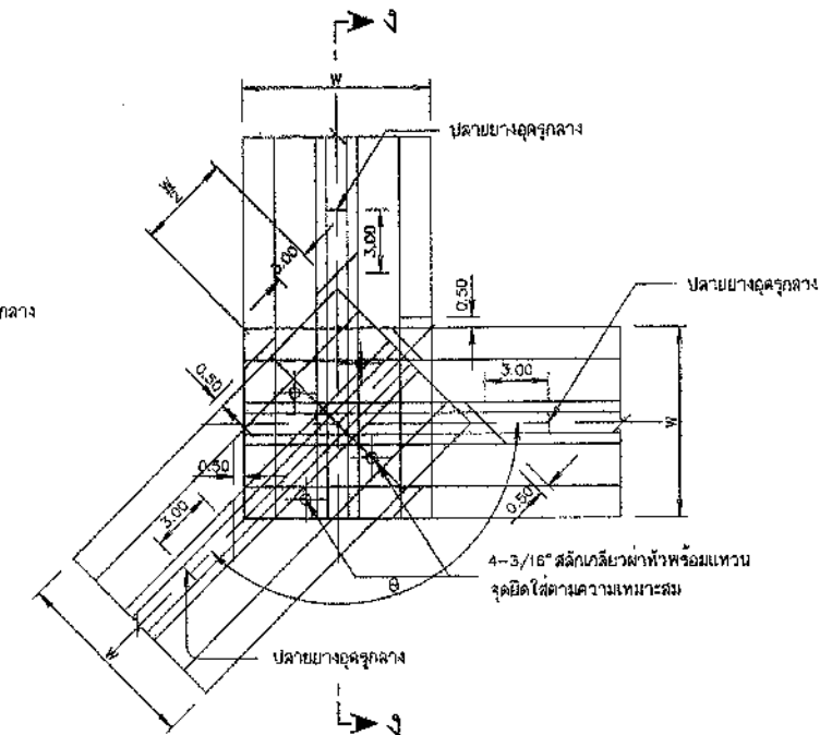
การต่อมุมกันทั้ง 3 ด้าน ไม่แสดงมาตราส่วน
