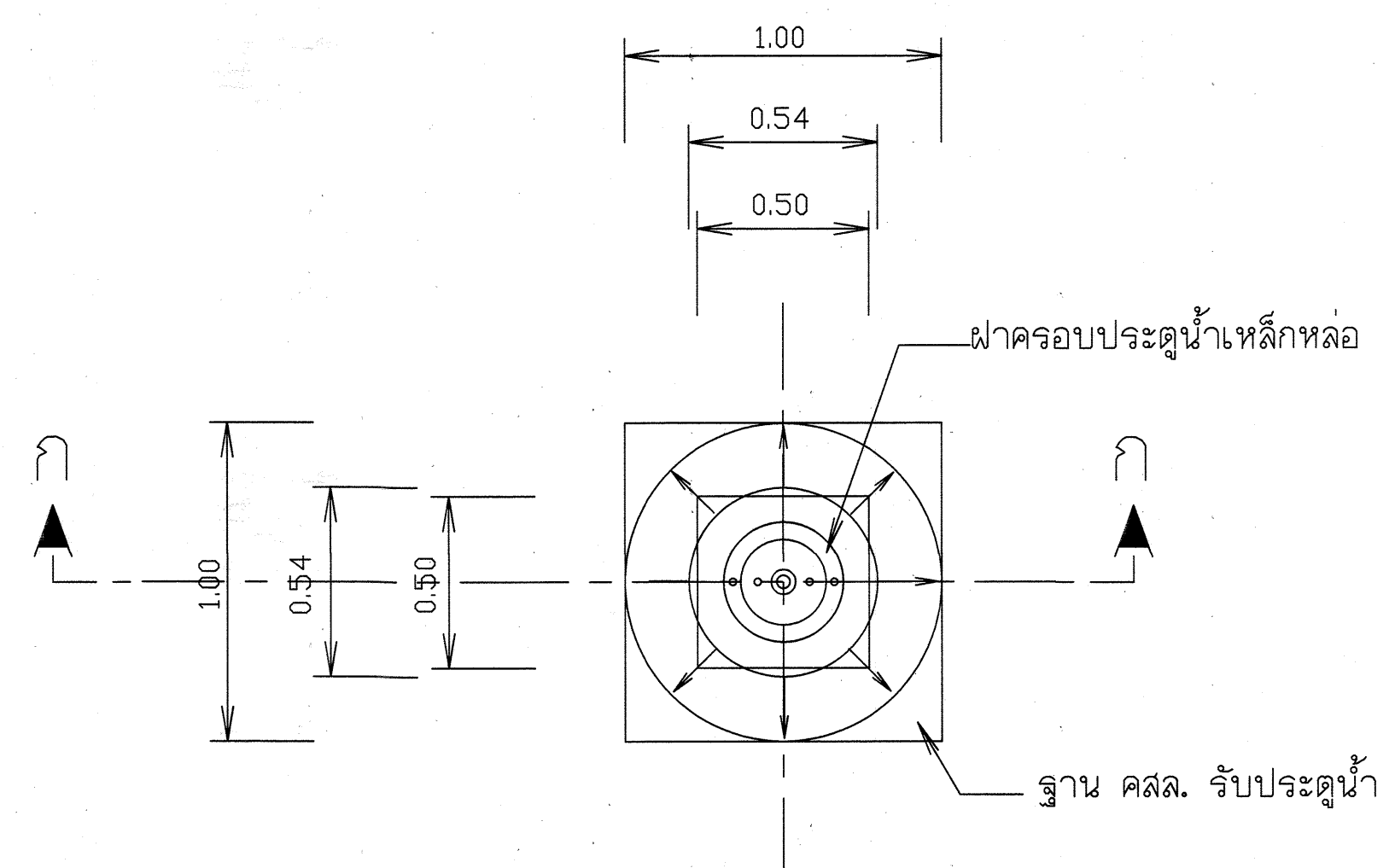
แปลนแสดงจุดติดตั้งประตูกวควบคุมท่อย้ายน้ำ ขนาด 400 มม. มาตรฐาน 1:75
