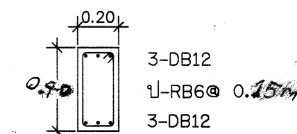
แบบขยายโครงสร้างคานรับ (BE) SCALE 1:100
