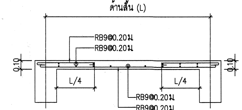
แบบขยายพื้น (SA) SCALE 1:100
