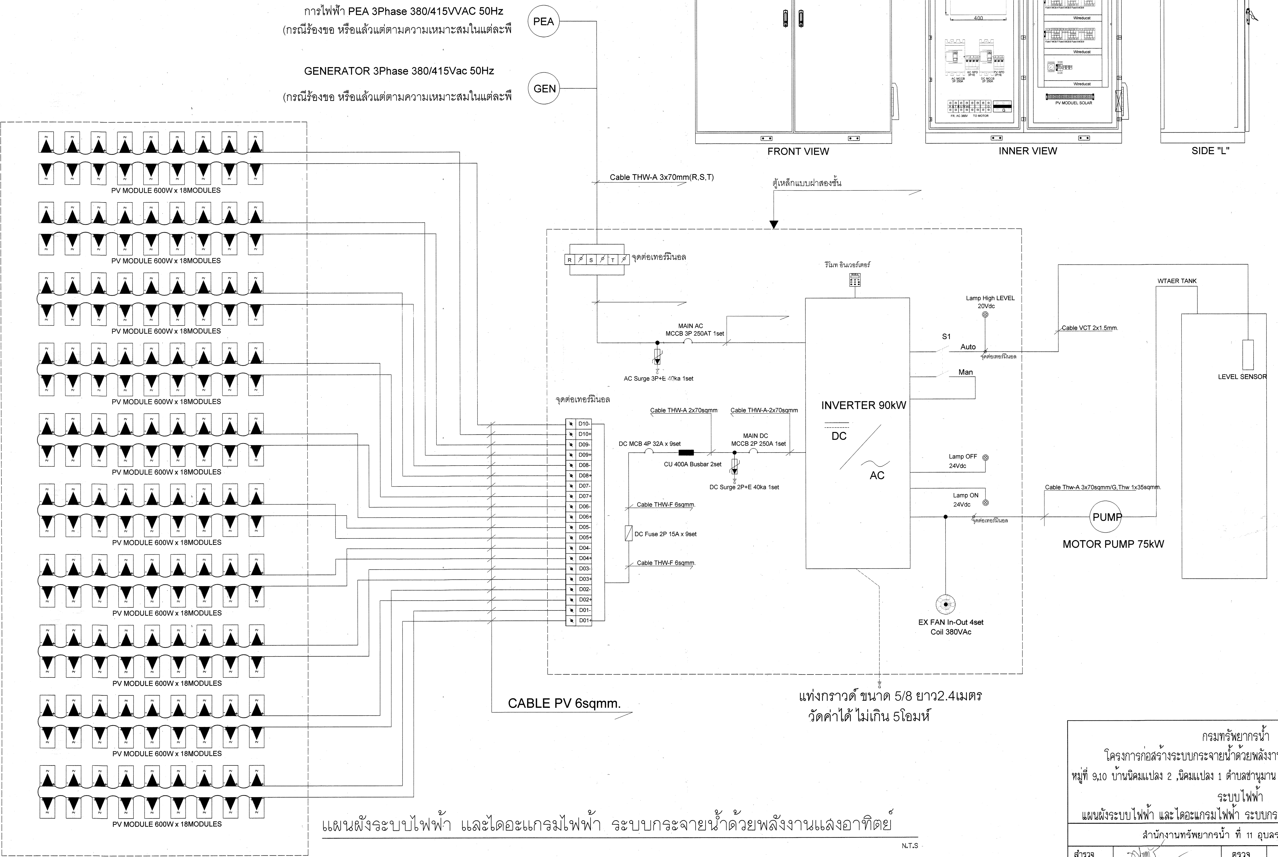
PV MODULE 600Wx18MODULES x9STRINGS
