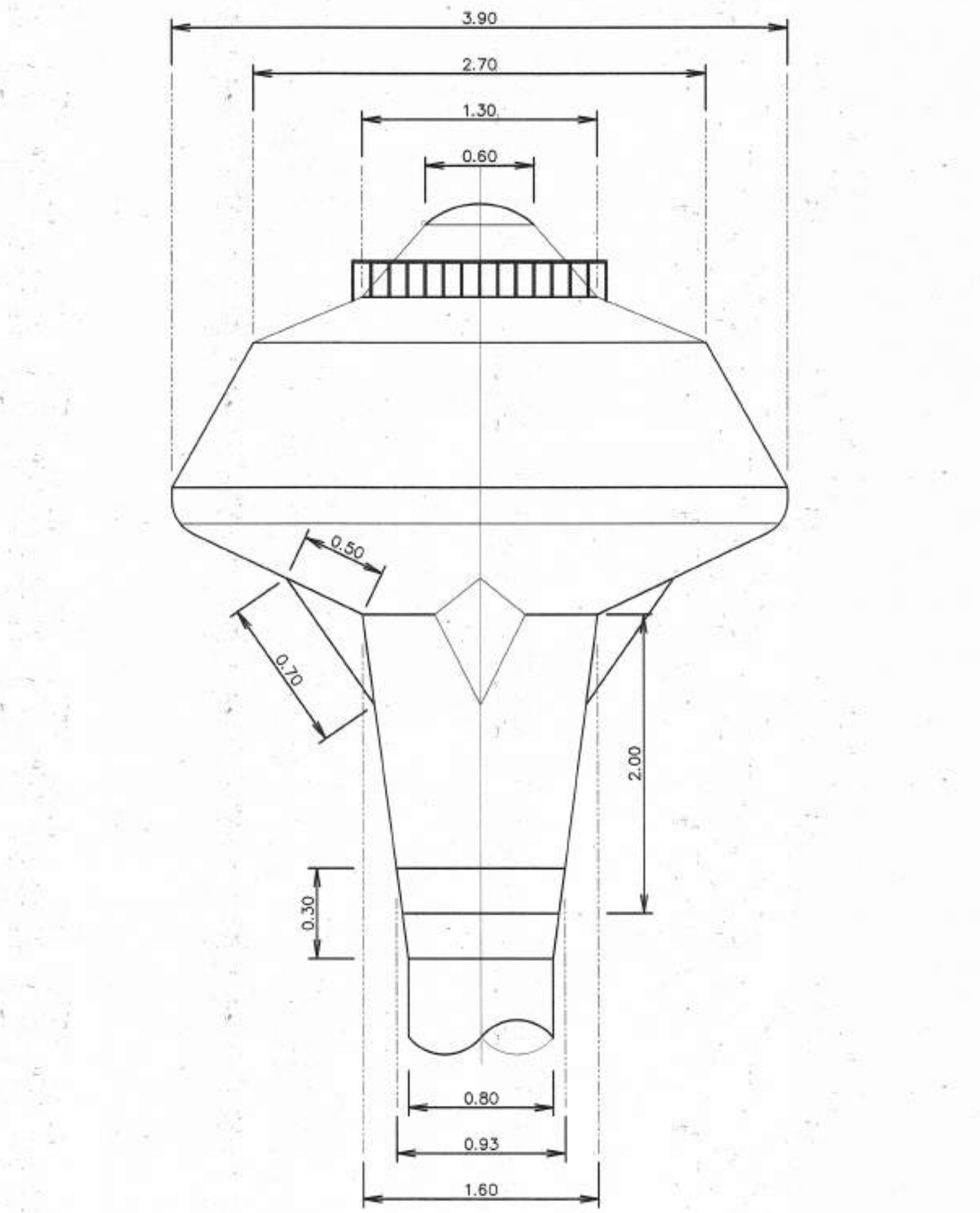
แบบขยายแมนโฮลบนหอดึงสูง
