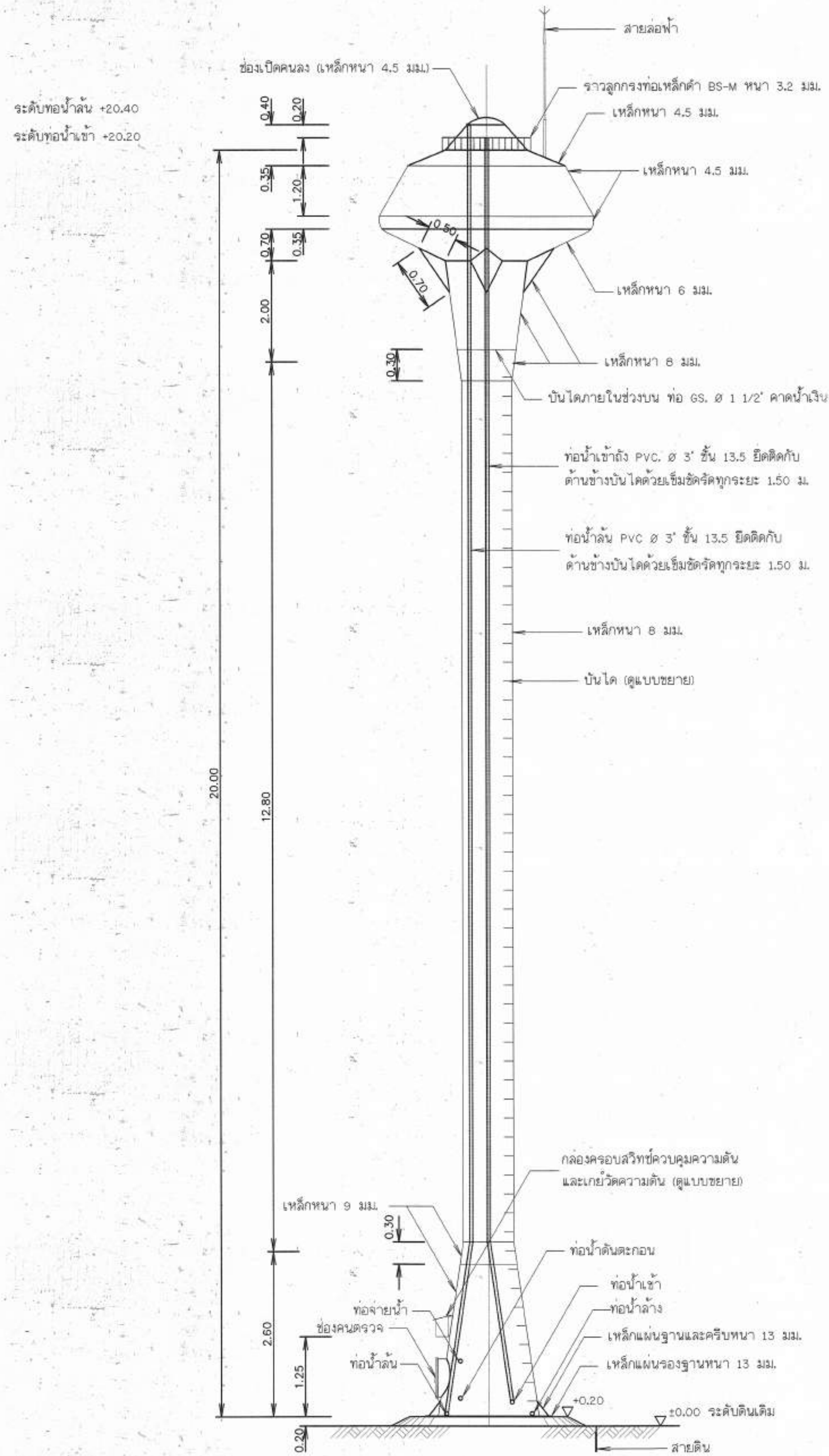
รูปด้านข้างหอดึงสูง แบบถังเหล็กรูปทรงแชมเปญ
