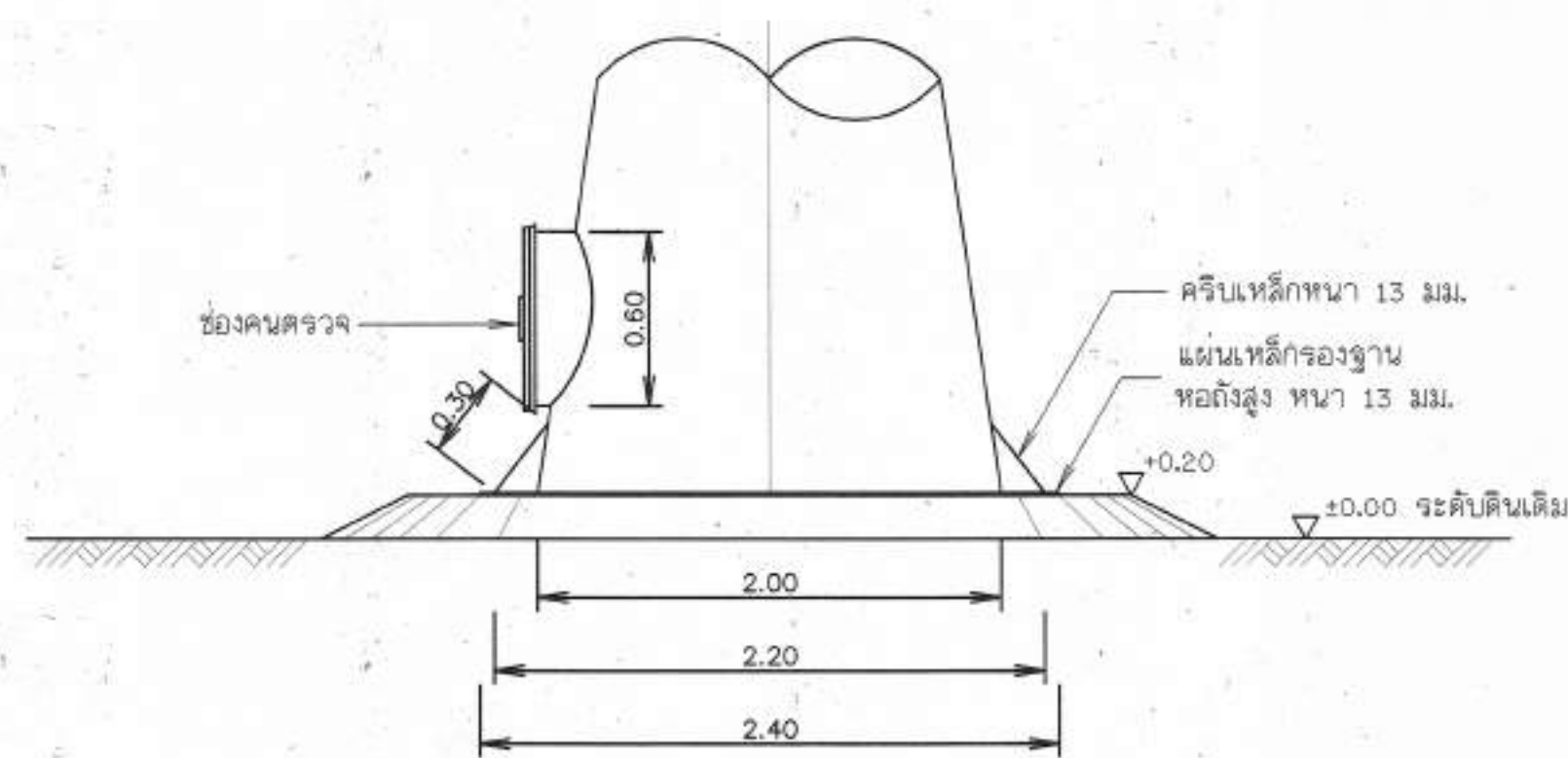
แบบขยายแมนโฮลล่างหอดึงสูง
