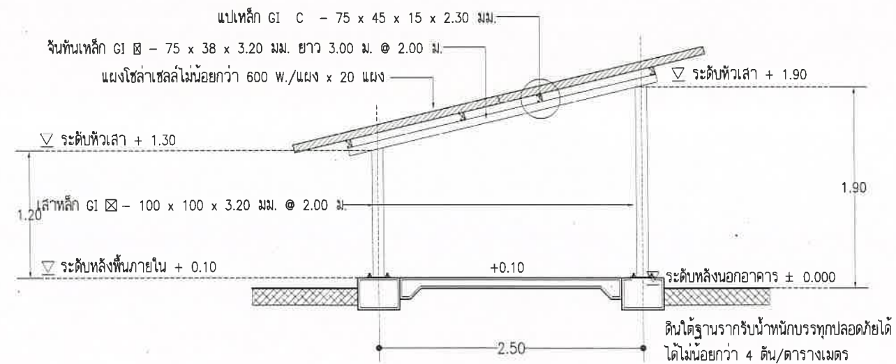
รูปตัดตามขวาง
