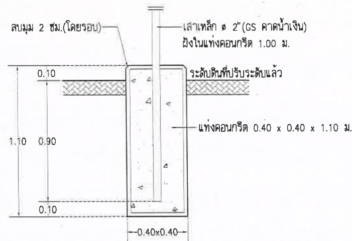
ขยาย F1 SCALE 1:25
