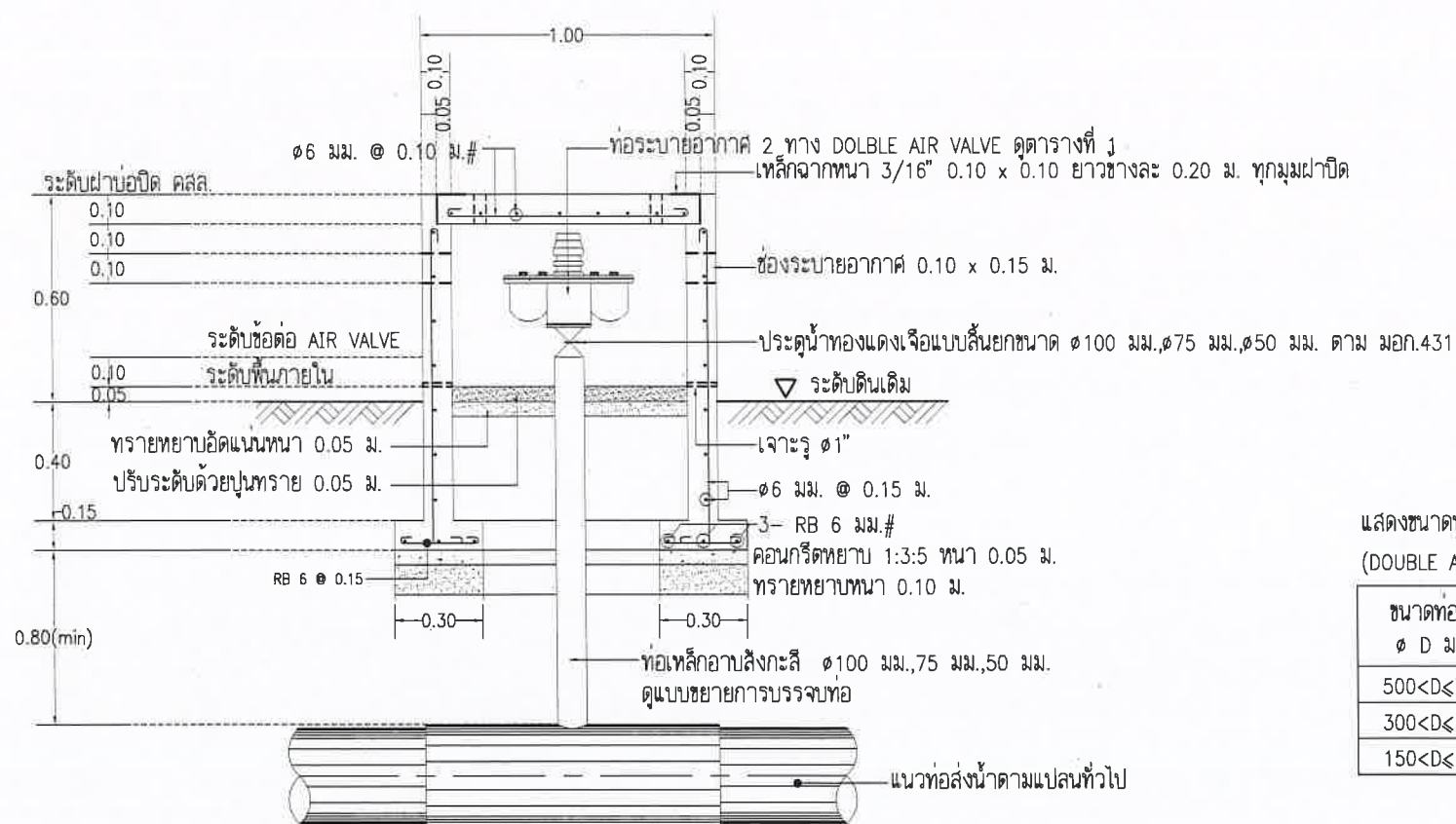
รูปตัดอาคารท่อระบายอากาศ 1:25
