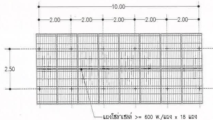
แปลนแสดงอาคารแผงโซล่าเซลล์
