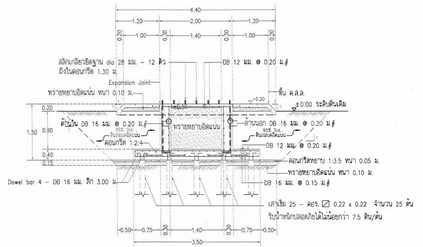
รูปตัดฐานรากหอถังสูง (แบบเสาเข็ม)
