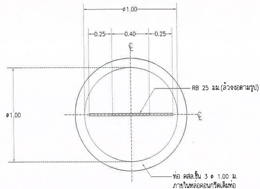
แปลนท่อสมอยึดอาคารโรงสูบน้ำ
