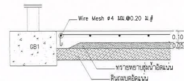
ขยายพื้น GS
