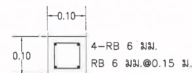
แบบขยายเหล็กเสริมหลักบ่อแก้ว มาตราส่วน 1:15
