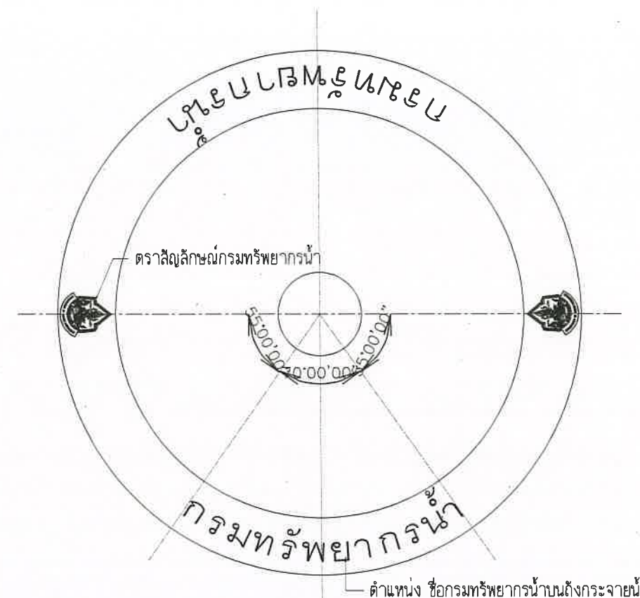
รูปขยายแสดงขนาดตราและชื่อกรมทรัพยากรน้ำจนถึงกระจายน้ำ ไม่แสดงมาตราส่วน
