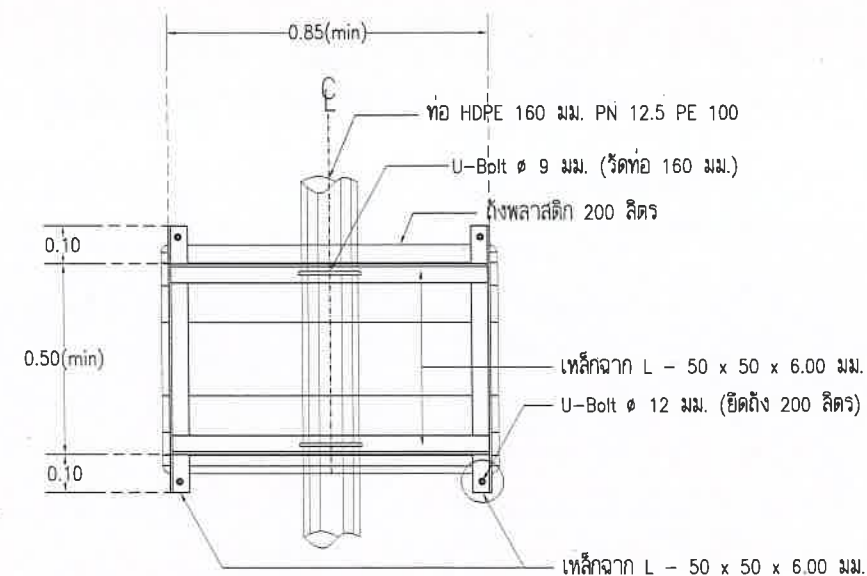
แปลนท่อนลอย
