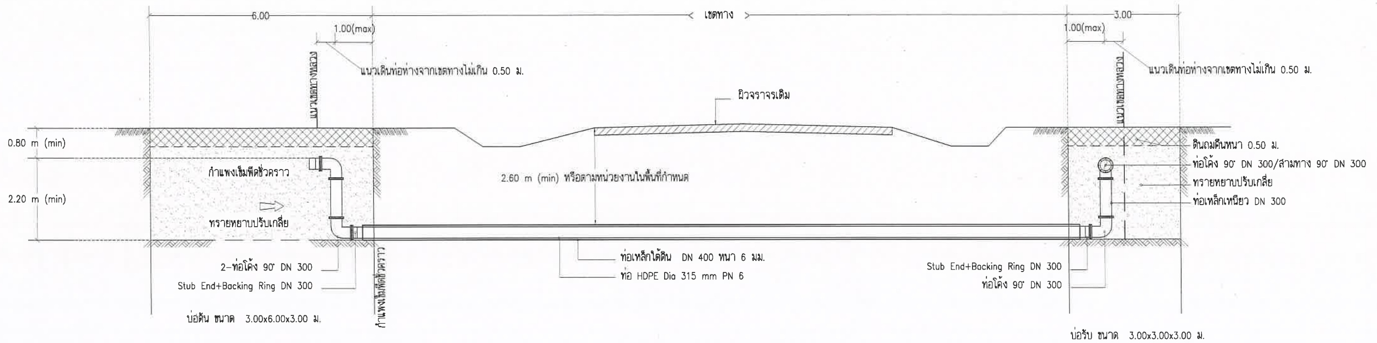
งานติดตั้งท่อปลอกลอดถนน (pipe jacking) SCALE 1:100
