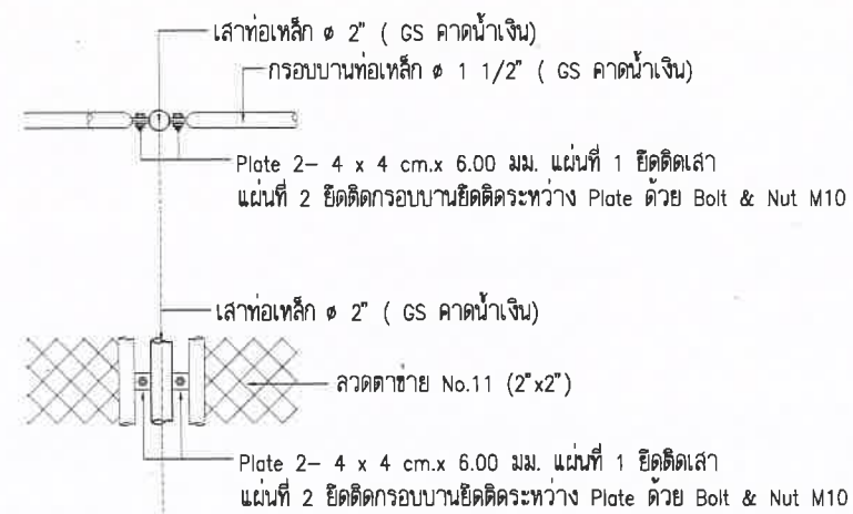
แบบขยาย 1 SCALE 1:20
