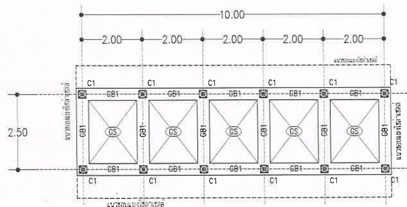
แปลนคานคอดิน เสา พื้น รับแผงโซล่าเซลล์
