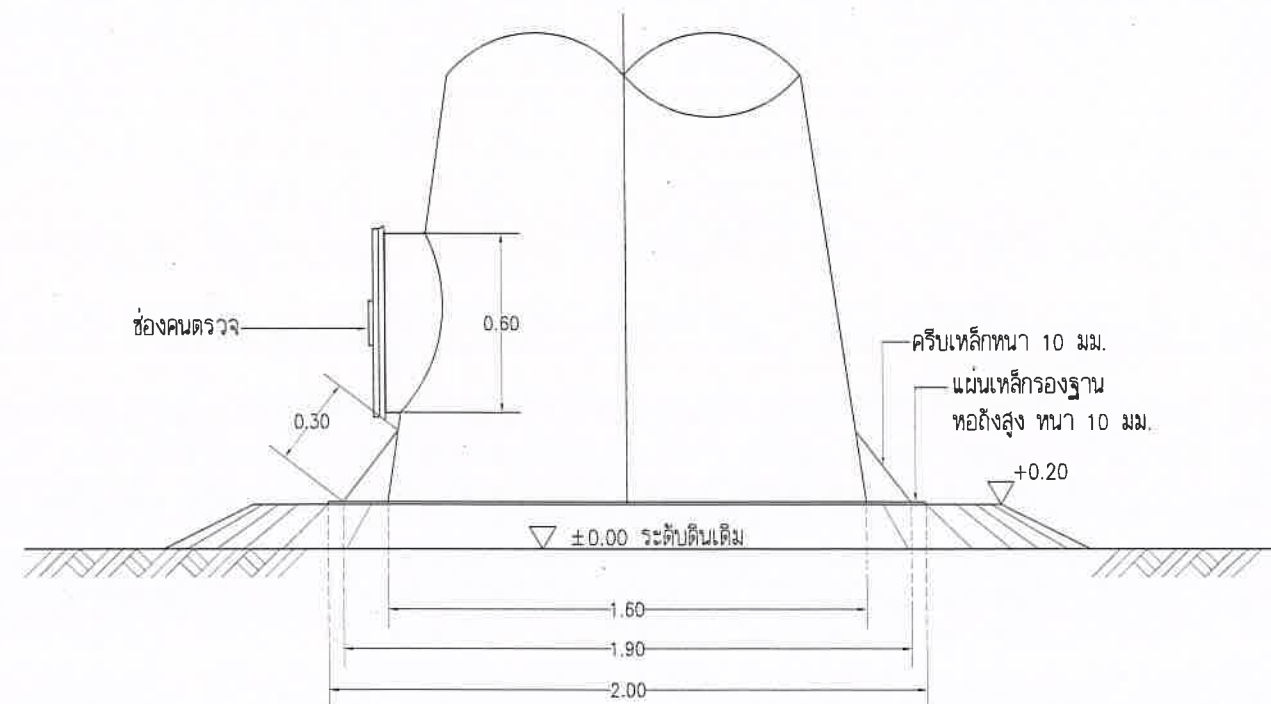
แบบขยายแมนโฮลล่างท่อถึงสูง ไม่แสดงมาตราส่วน
