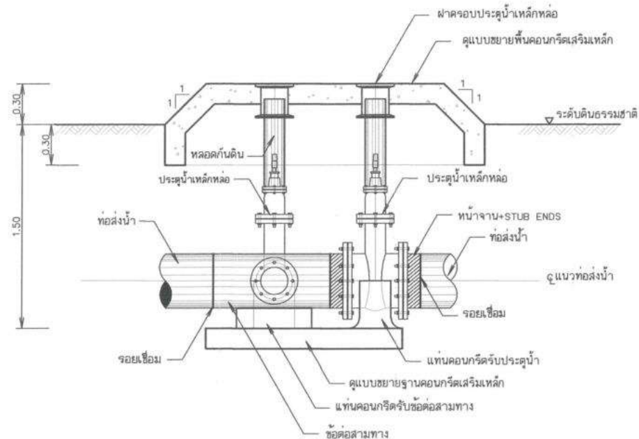
รูปตัดอาคารจตุรภาค
