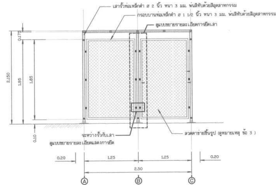
แบบขยายรั้ว 2 มาตราส่วน 1:50
