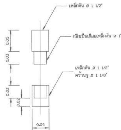
แบบขยายบานพับหัวเหล็ก มาตราส่วน 1:5
