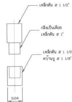
แบบขยายบานพับที่เหล็ก
