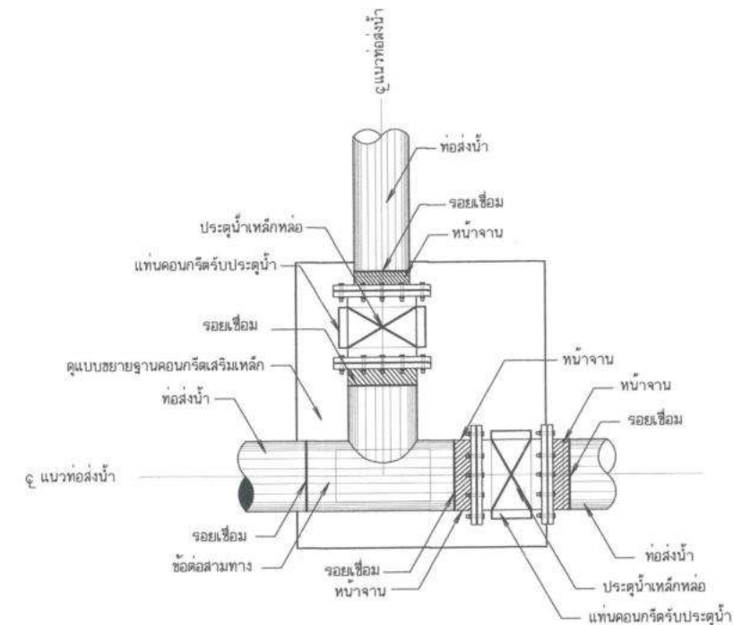
รูปขยายการติดตั้งอาคารจตุรภาค
