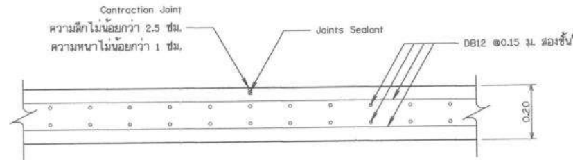
แบบขยายรอยต่อพื้น
