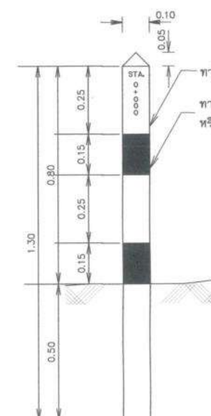
แสดงสัดส่วนหลักบอกแนวท่อ
