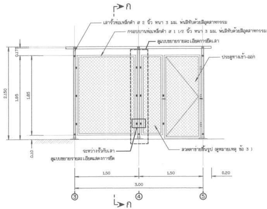
แบบขยายรั้ว 1 มาตราส่วน 1:50
