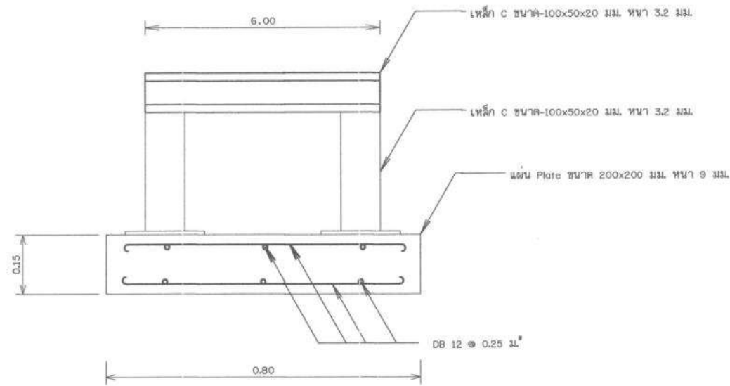
รูปด้าน โครงสร้างรับท่อ
