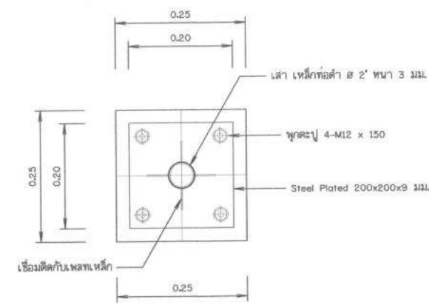
ฐานรากโครงสร้างอาคารคลุม มาตราส่วน 1:10
