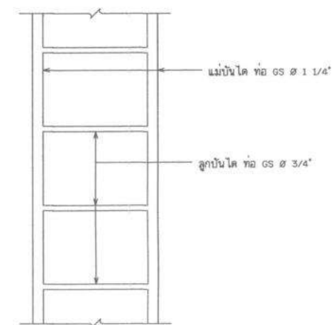
ขยายบันไดเหล็ก ไม่แสดงมาตราส่วน
