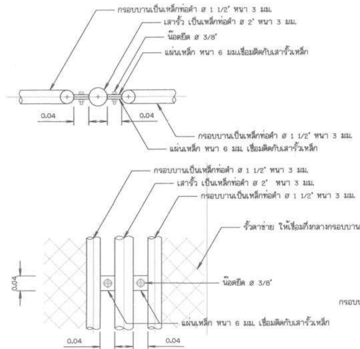
แบบขยายรายละเอียดแสดงการยึดระหว่างรั้วกับเสา มาตราส่วน 1:10
