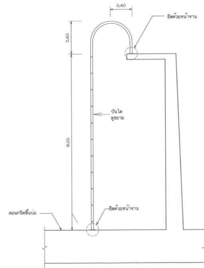
บันไดเหล็ก ไม่แสดงมาตราส่วน
