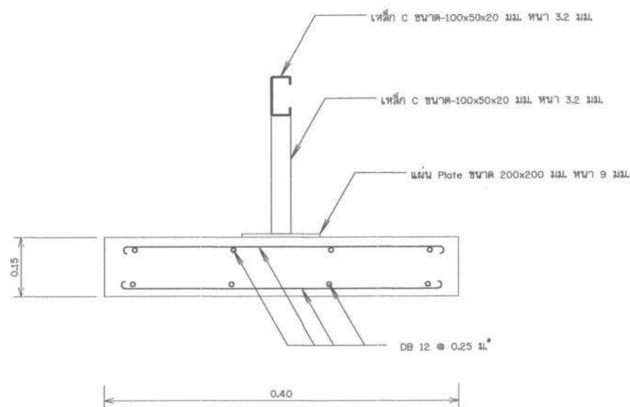
รูปตัด โครงสร้างรับท่อ
