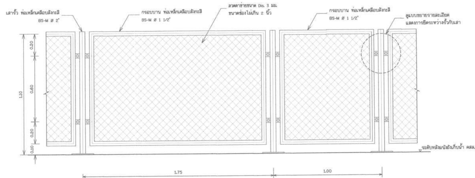
แบบขยายราวกันตก
