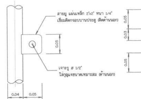
แบบขยายสายยู่
