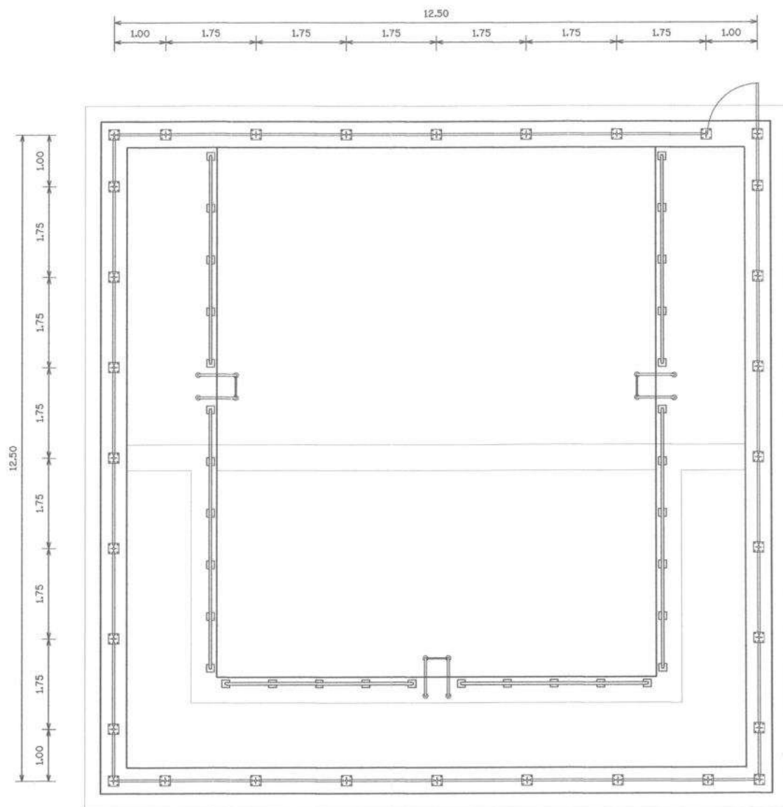
แบบแปลนรั้วลวดตาข่าย (บ่อสูบน้ำ คลส.)
