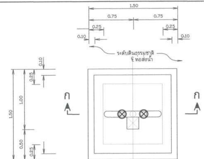
แปลนอาคารจุดปล่อยน้ำ 2 ด้าน
