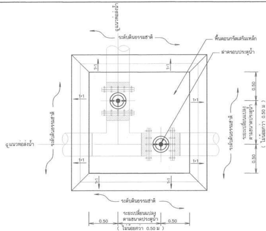
แปลนอาคารจตุรภาค
