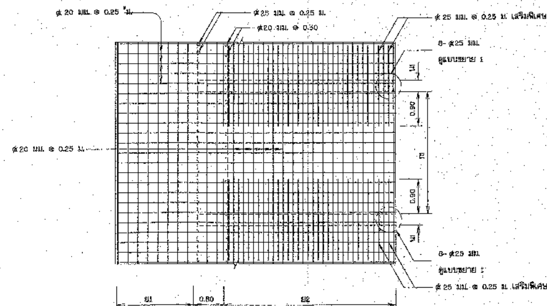
รูปตัด 4-ก (พื้นด้านบน)
