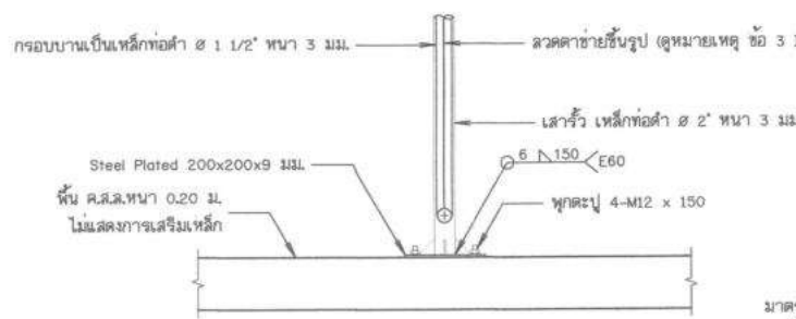
แบบขยายรายละเอียดแสดงการยึด ไม่แสดงมาตราส่วน
