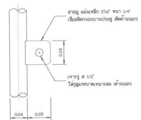
แบบขยายสายยู มาตราส่วน 1:5
