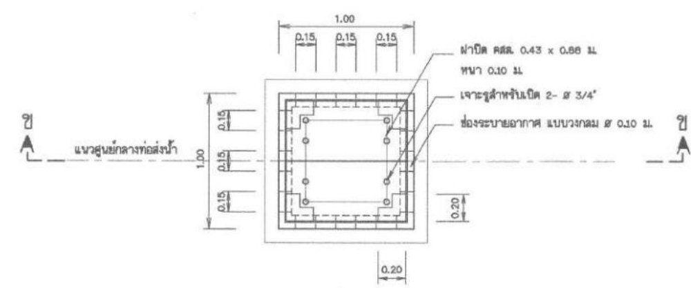
แปลนอาคารท่อระบายอากาศ มาตราส่วน 1:20
