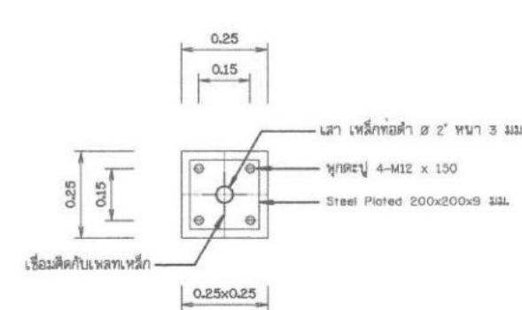
ฐานรากโครงสร้างอาคารคลุม ไม่แสดงมาตราส่วน
