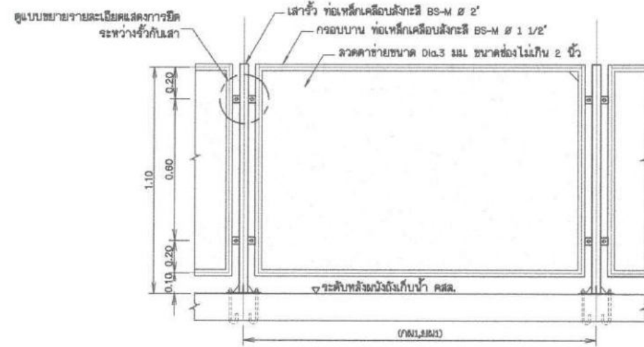
แบบขยายราวกันตก (สำหรับกับน้ำ คสล. แบบไม่มีฝ้า)
