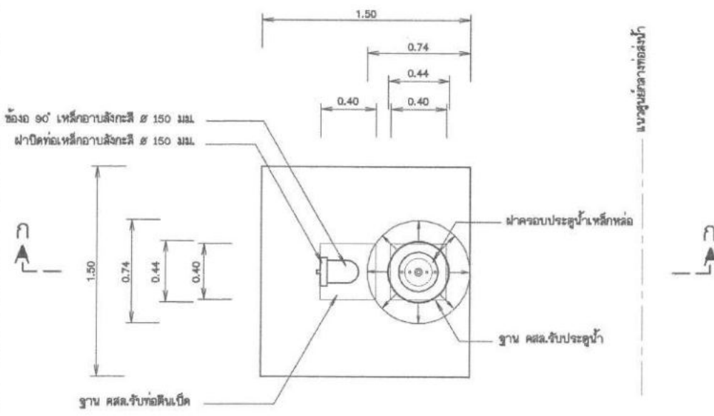
แปลนอาคารประตูลอยน้ำตะกอน มาตราส่วน 1:20
