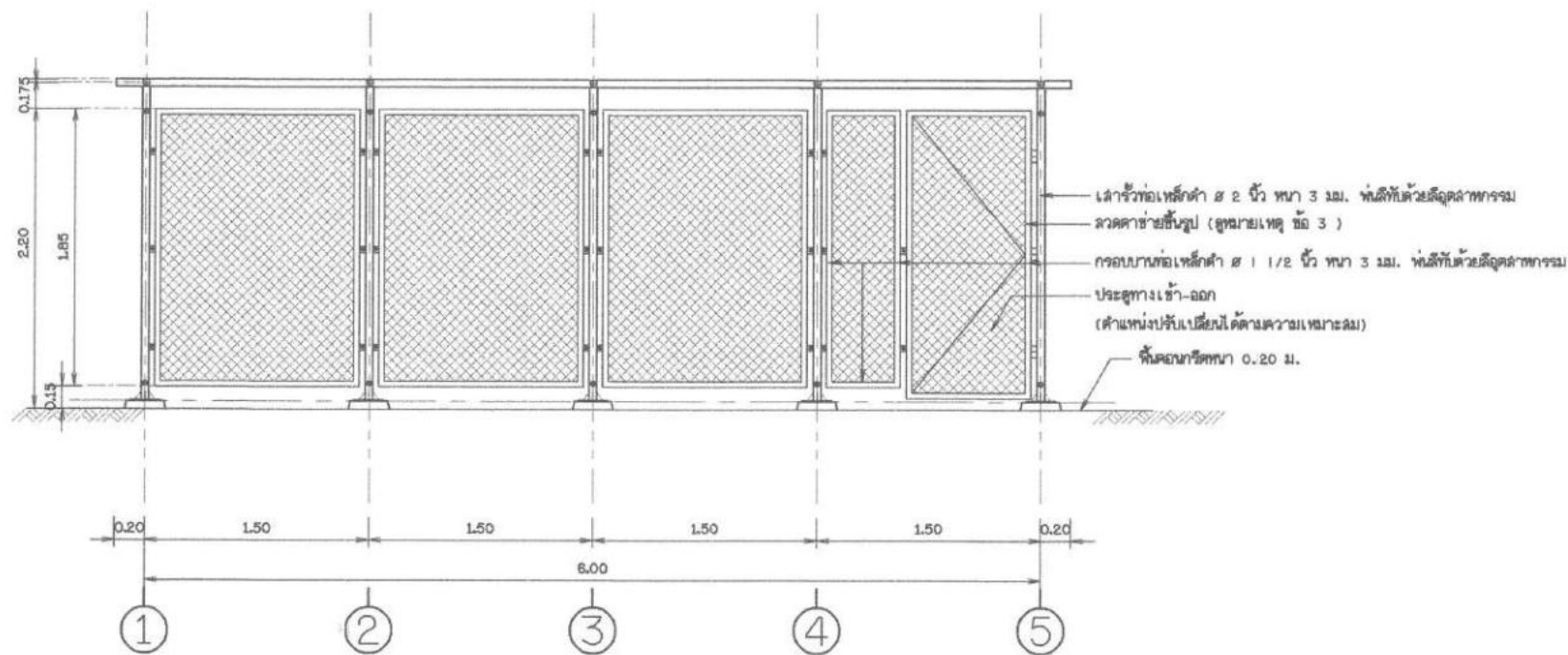
แบบขยายรั้ว 1 ไม่แสดงมาตราส่วน
