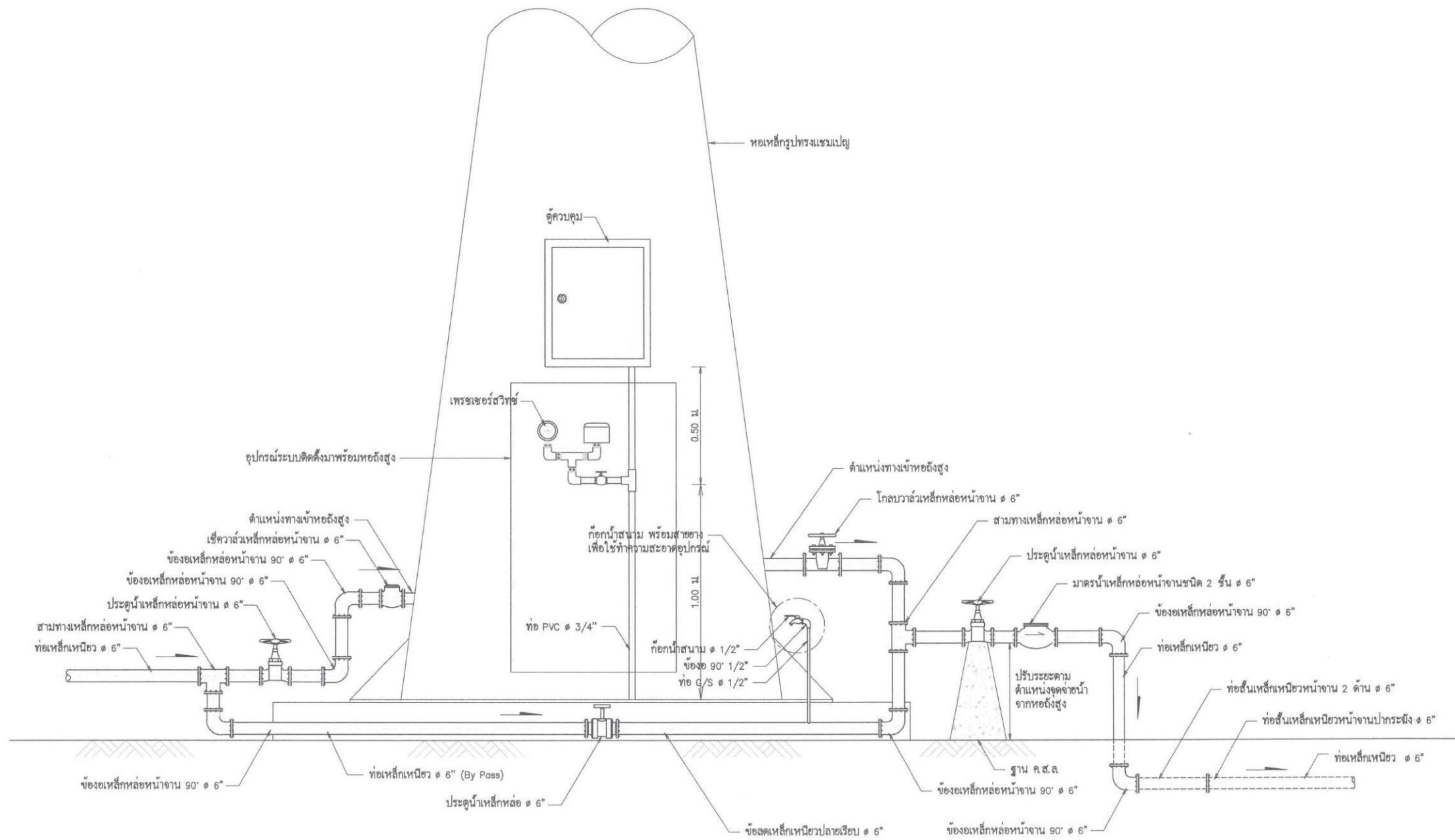
รูปแสดงรายละเอียดการต่อท่อและอุปกรณ์ออกจากถังเหล็กรูปทรงแฉมแปญ ไม่แสดงมาตราส่วน
