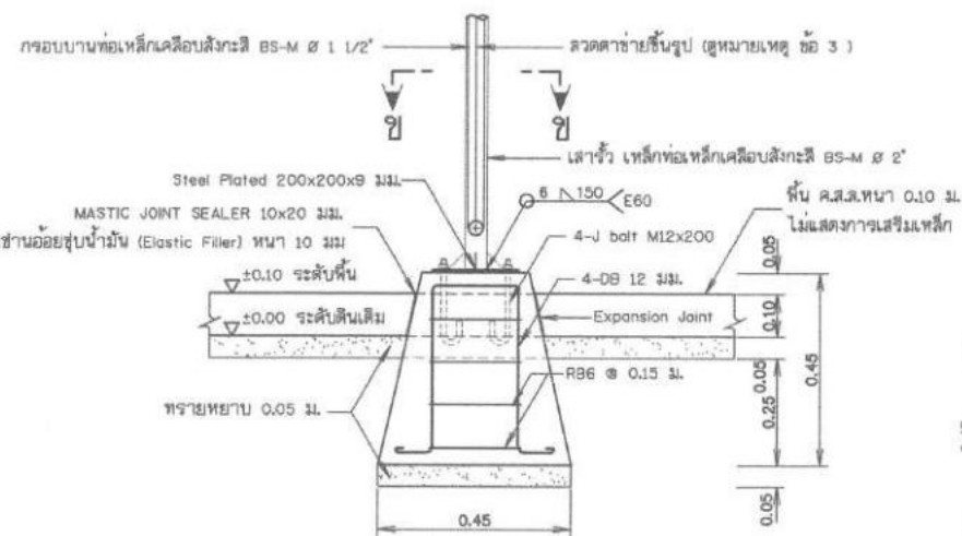
รูปขยายฐานรากโครงสร้างรับแผง F1 (คอนกรีตเสริมเหล็ก หรือเสาเข็มรูปทรงสี่เหลี่ยม) ไม่แสดงมาตราส่วน
