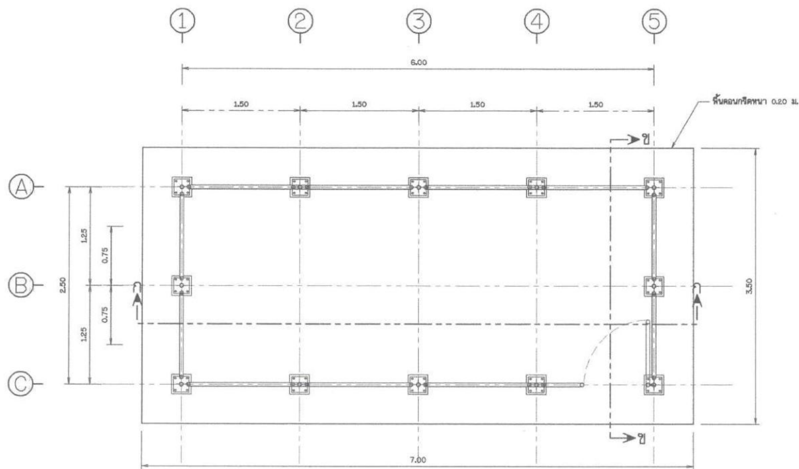
แปลนเสาและรื้อ โมเดลขนาดจริง
