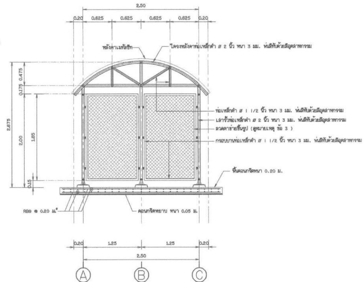
รูปตัด ข - ข โมเมนต์ขนาดจั่วหัว
