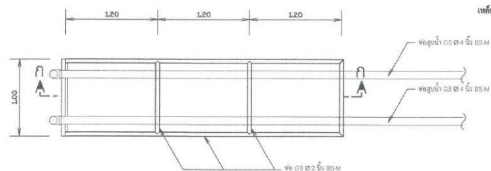
แปลนโครงสร้างรับท่อสูบน้ำ
