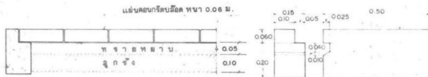
ขยายคันคอนกรีต I-10
