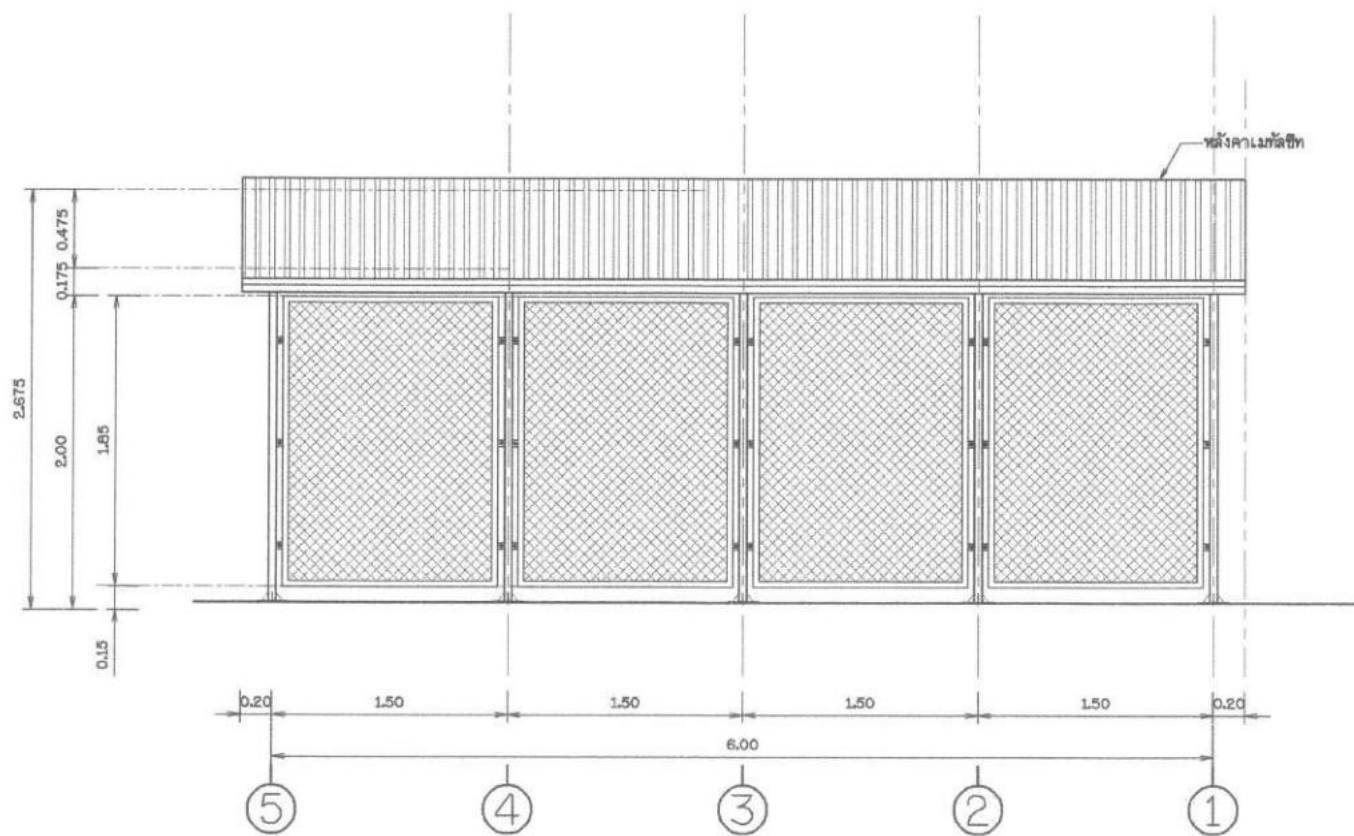
รูปด้าน 1 ไม่แสดงขนาดตัว
