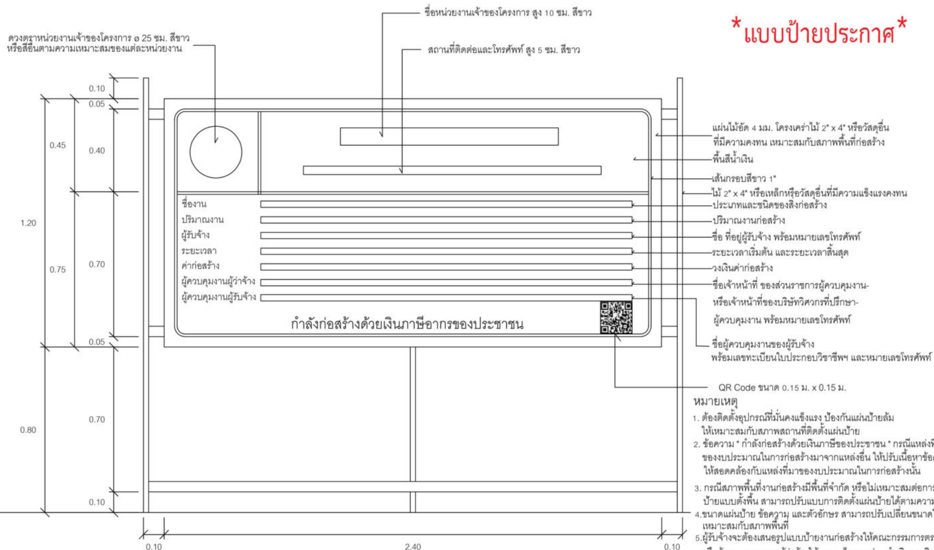
รูปด้านหน้า 1 : 50
