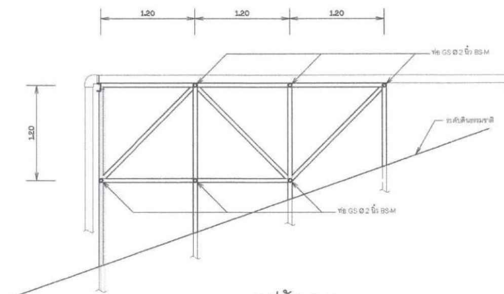
รูปตัด A-A
