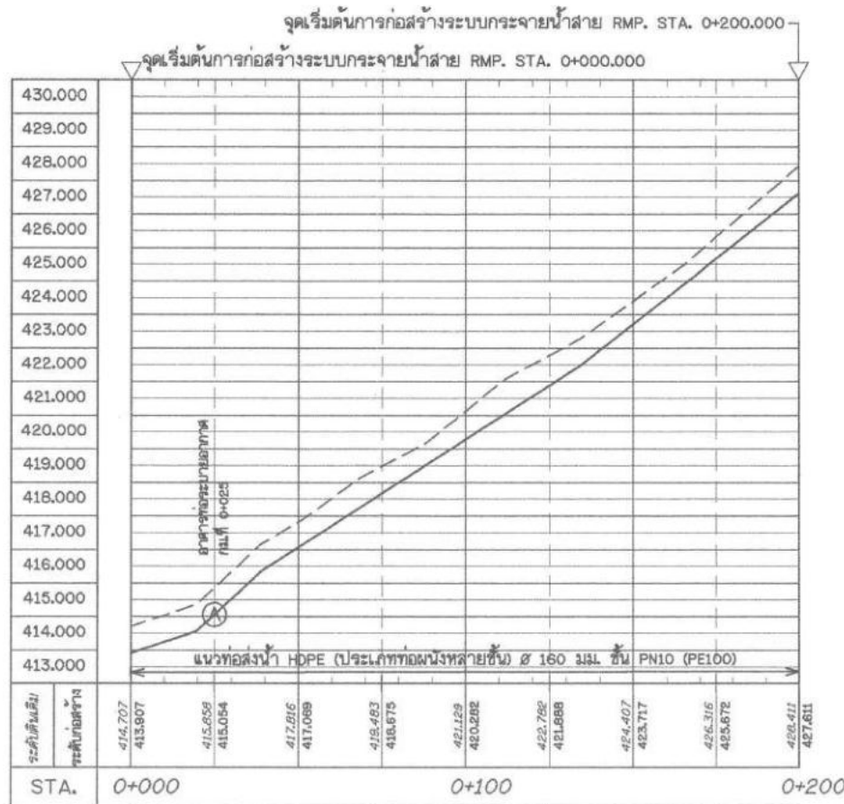
แปลนระบบส่งน้ำ สาย RMP. STA. 0+000 - 0+200 มาตราส่วน 1:1,000
