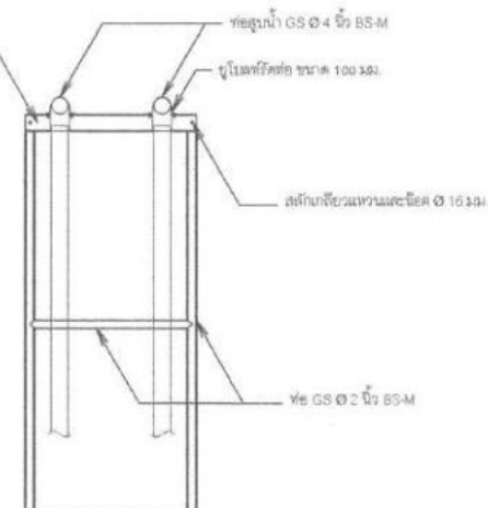
รูปด้านหน้า
