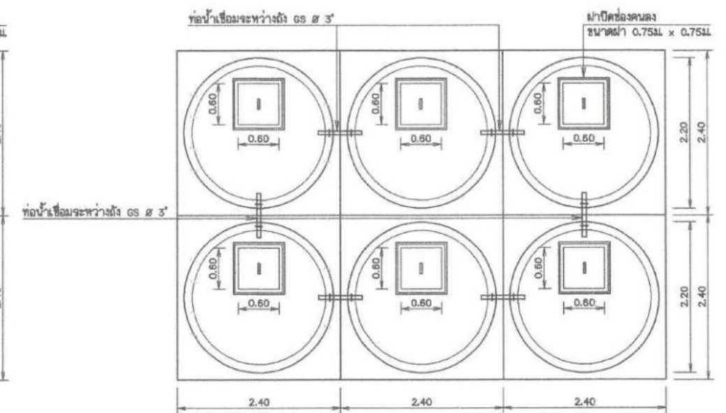
แบบ 6 ถึง มาตราส่วน 1:40
