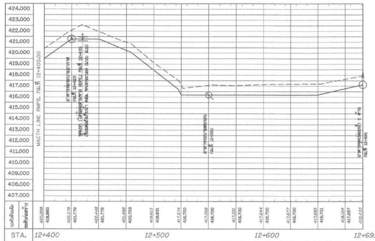
รูปตัดตามแนวยาว มาตรฐาน 1:500 แนวราบ 1:1,000
