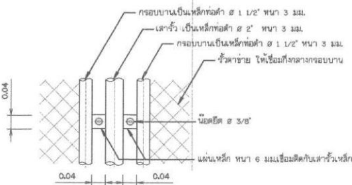
แบบขยายรายละเอียดแสดงการยึดระหว่างรั้วกับเสา ไม่แสดงมาตราส่วน
