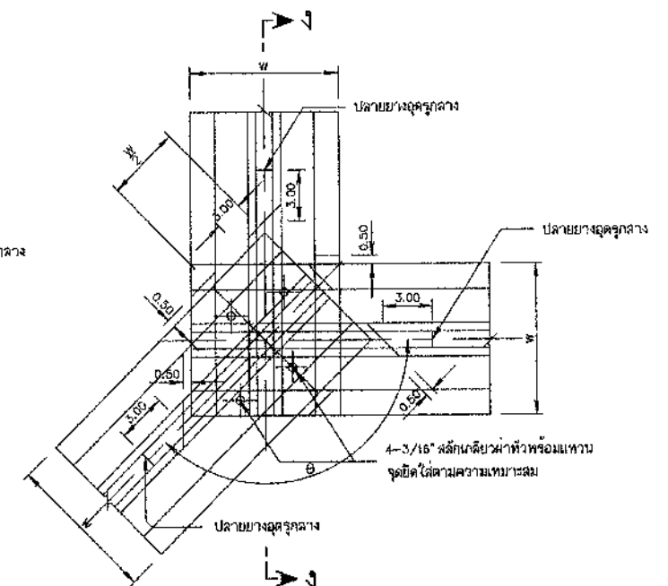
การต่อมุมกันทั้ง 3 ด้าน ไม่แสดงมาตราส่วน
