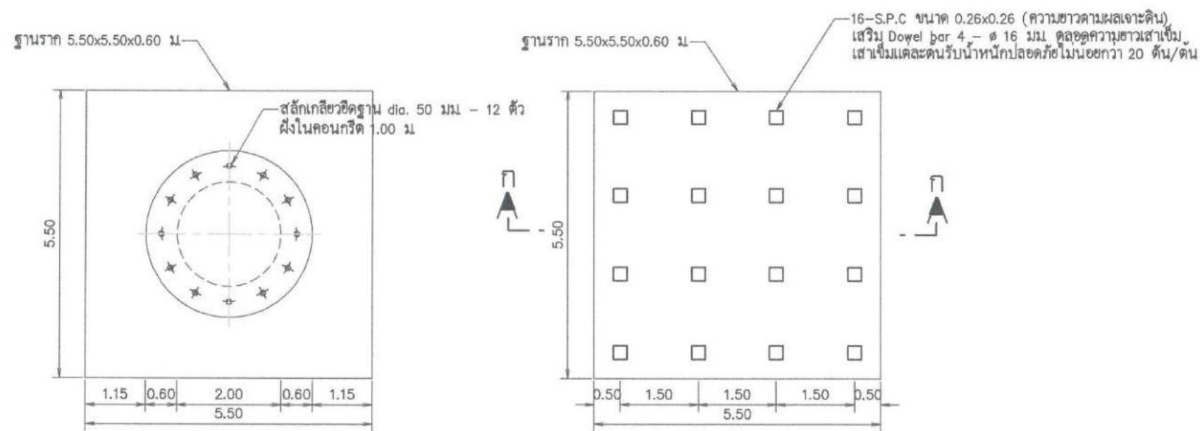
แปลนฐานรากหอถังสูง (แบบเสาเข็ม) ไม่แสดงมาตราส่วน
