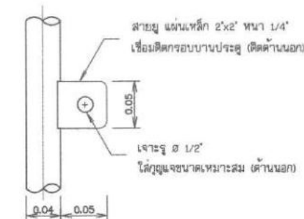
แบบขยายสายลึง ไม่แสดงมาตราส่วน
