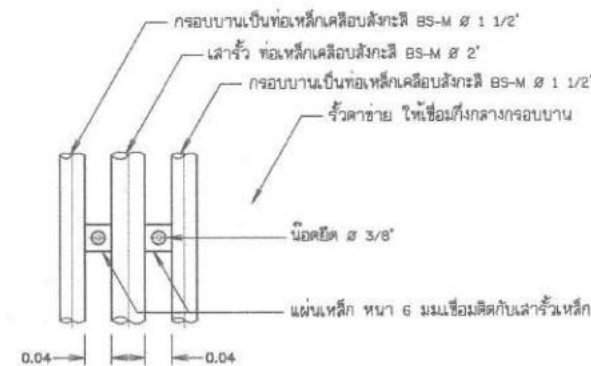
แบบขยายรายละเอียดแสดงการยึดระหว่างหัวกับเสา ไม่แสดงมาตราส่วน
