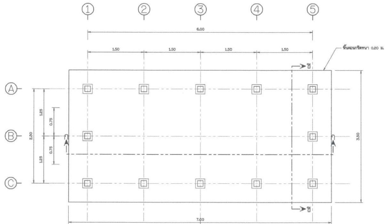
แบบแปลน โมเดลขนาดจริง
