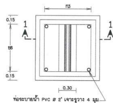
แปลนบ่อประตูปังคังน้ำ มาตราส่วน 1:20
