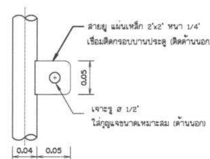
แบบขยายสายเย็บ ไม่แสดงขนาดราวล้วน
