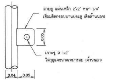
แบบขยายสายยู ไม่แสดงขนาดบางส่วน
