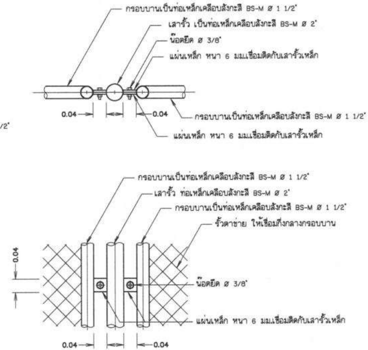
แบบขยายรายละเอียดแสดงการยึดระหว่างร้วกับเสา ไม่แสดงขนาดบางส่วน
