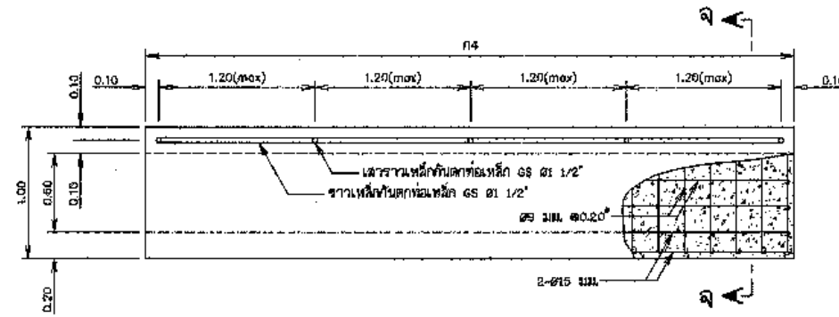
รูปขยาย 2 พื้นสะพานสำเร็จรูป
