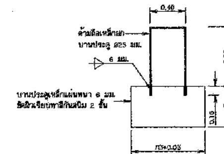
บานประตูเหล็ก
