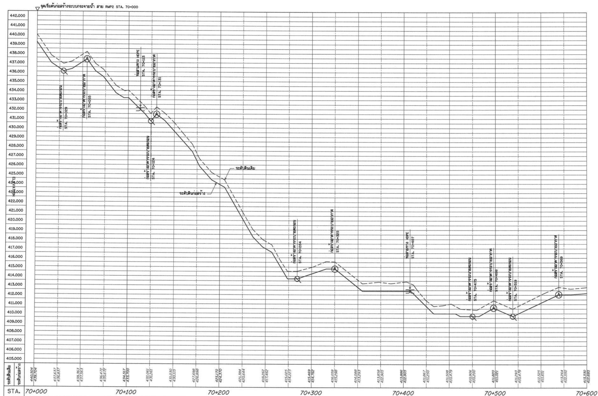
รูปตัดตามแนวยาวระบบกระจายน้ำ สาย RMP STA. 70+000 - 70+600 มาตรฐาน มาตรฐาน 1:1,000 แนวตั้ง 1:100
