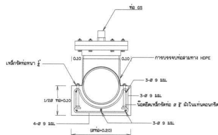
รูปตัดขยาย "1" มาตราส่วน 1:10
