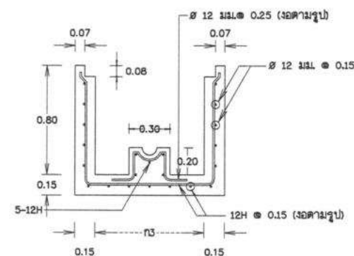
เหล็กเสริมบ่อประตูปังคังน้ำ มาตราส่วน 1:20
