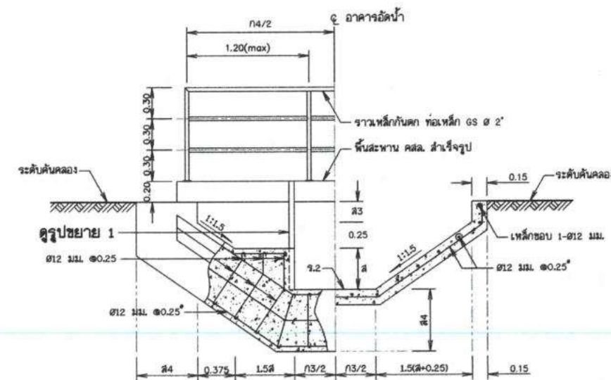
รูปตัด ข-ข
