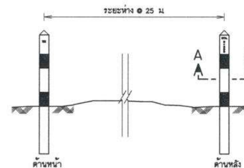
แสดงการวางหลักบ่อแนวทอ มาตราส่วน 1:20
