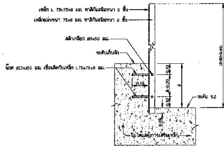
รูปตัด ง-ง
