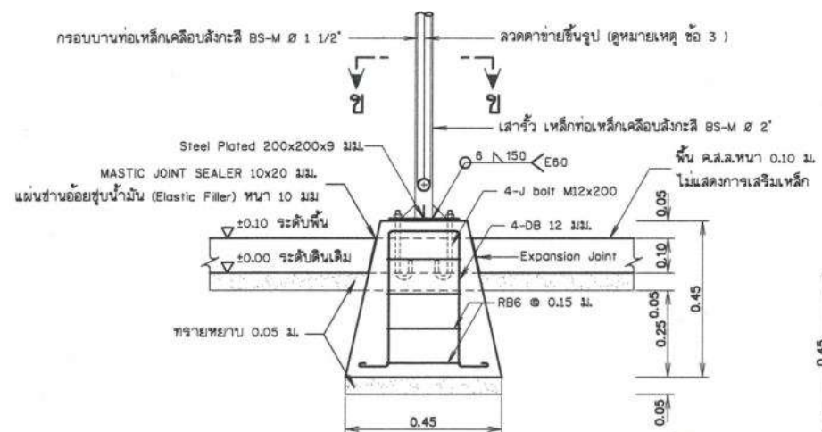
รูปขยายฐานจากโครงสร้างรับแผง F1 (คอม่อ คสล. หล่อสำเร็จรูปพร้อมติดตั้ง) ไม่แสดงขนาดบางส่วน
