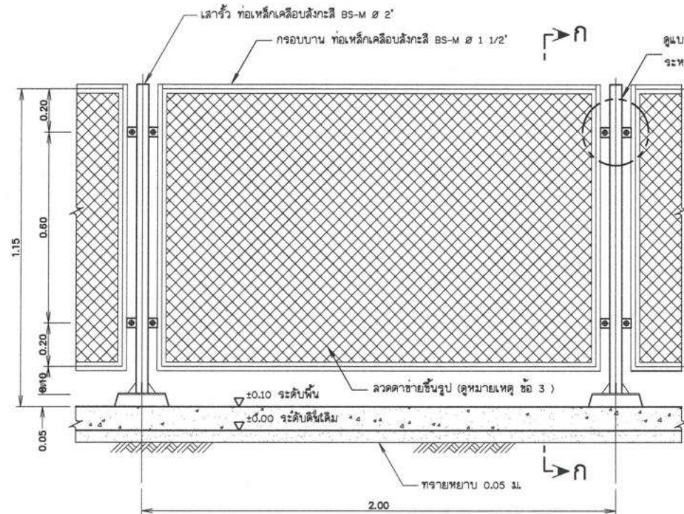
แบบขยายร้วลดต่ำ ไม่แสดงขนาดบางส่วน
