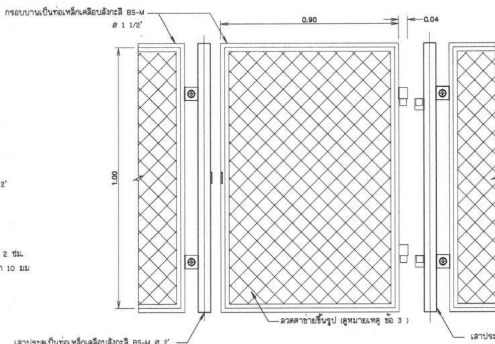
แบบขยายรายละเอียดประตู ไม่แสดงขนาดบางส่วน
