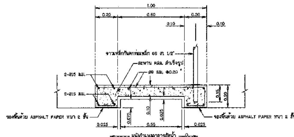
รูปตัด จ-จ
