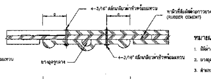
รูปตัด จ-จ ไม่แสดงขนาดส่วน
