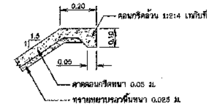
รูปขยาย 3
