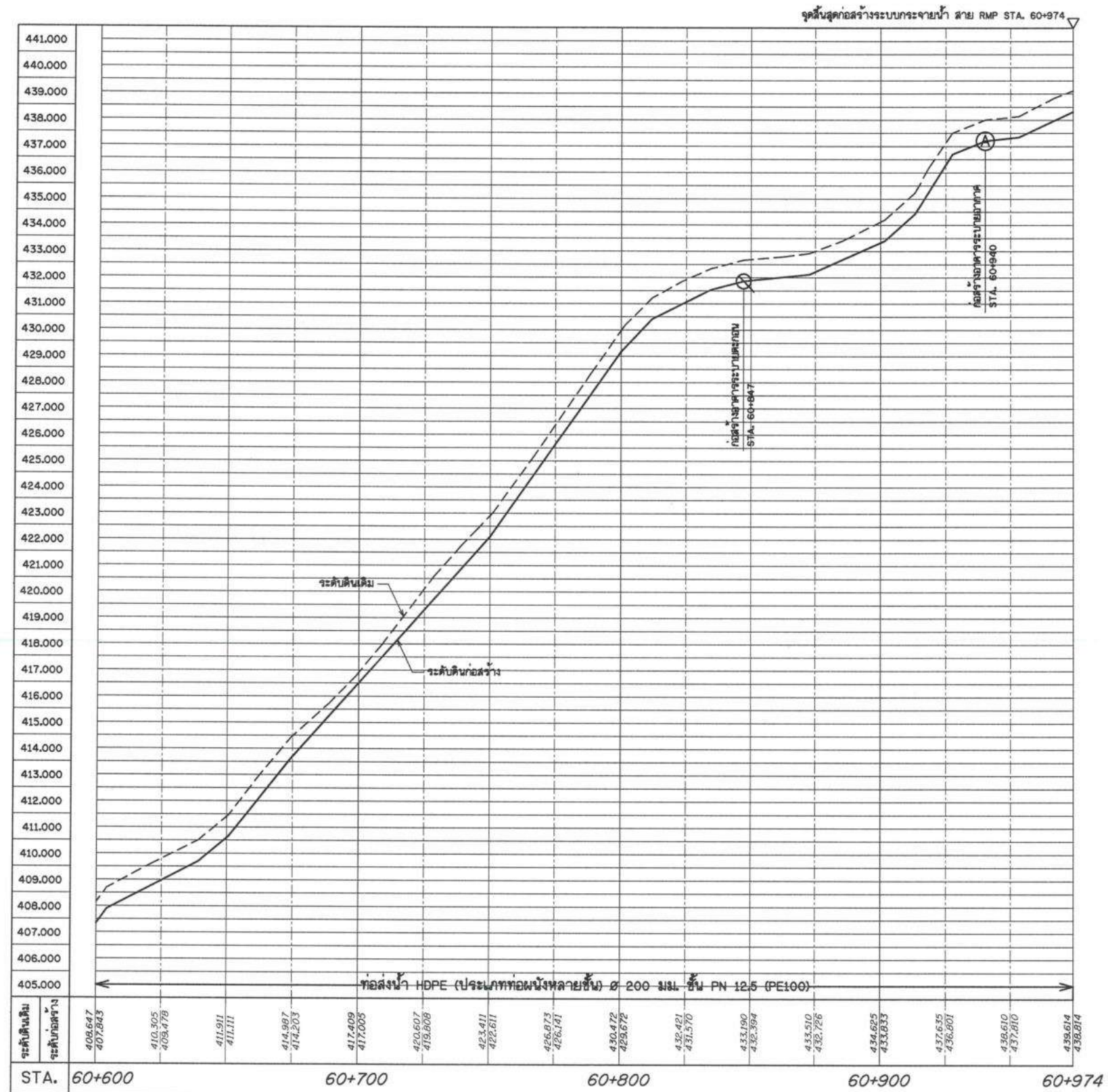
รูปตัดตามแนวยาวระบบกระจายน้ำ สาย RMP STA. 60+600 - 60+974 มาตรฐาน มาตรฐาน 1:1,000 แนวตั้ง 1:100
