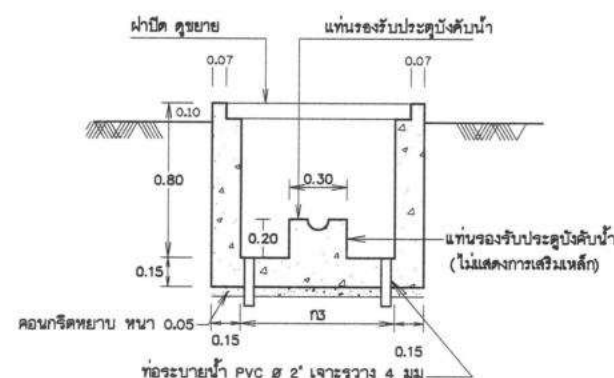
รูปตัด 1 - 1 มาตราส่วน 1:20
