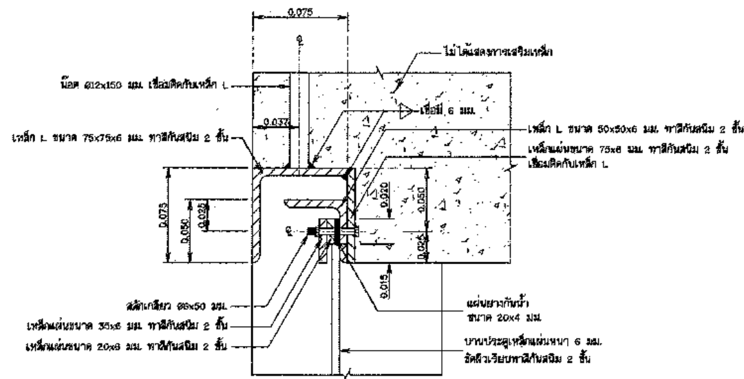
รูปขยาย 4 แสดงการติดตั้งบานประตู
