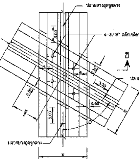
การต่อพาดทับกันไม่ทำมุมฉาก ไม่แสดงขนาดส่วน
