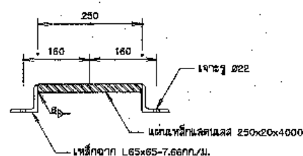
รูปขยายเหล็กเสริม
