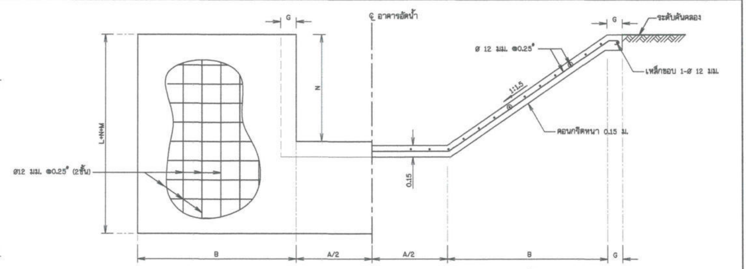
รูปตัด ข-ข ไม่แสดงขนาดบางส่วน
