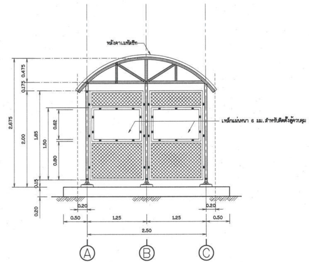
รูปด้าน 2 ไม่แสดงขนาดราวกว้าง
