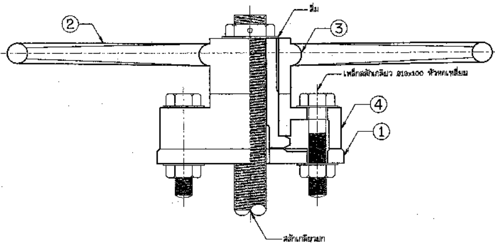
แสดงการติดตั้ง มาตราส่วน 1:2
