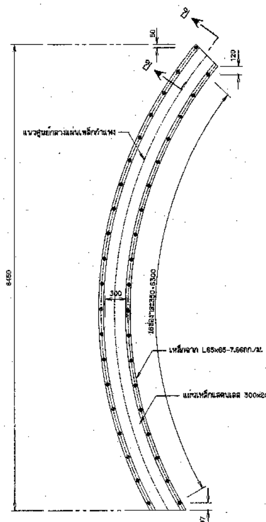
การติดตั้งเหล็กกำแพง
