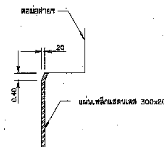
รูปตัด ข-ข
