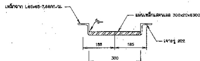
รูปขยายเหล็กกำแพง
