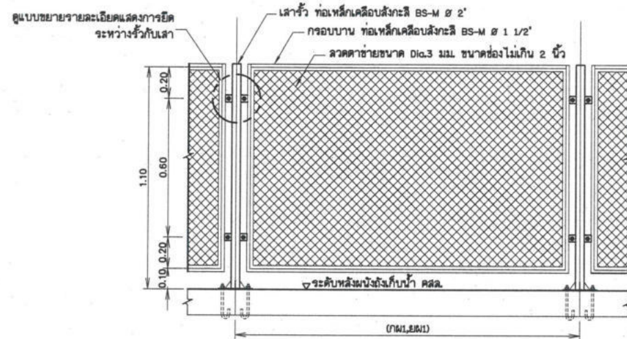
แบบขยายราวกันตก (สำหรับถังเก็บน้ำ คสล. แบบไม่มีฝาท็อป)
