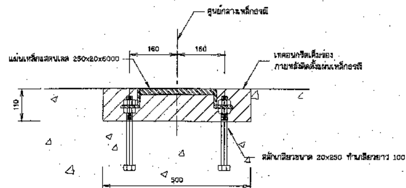
การติดตั้งเหล็กเสริม
