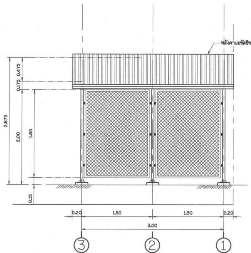
รูปด้าน 1 โมเดลขนาดจริง
