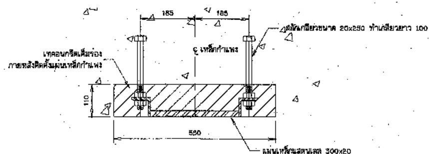
การติดตั้งเหล็กกำแพง
