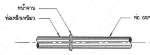
การบรรจบท่อเหล็กเหนียวกับท่อ GSP.
