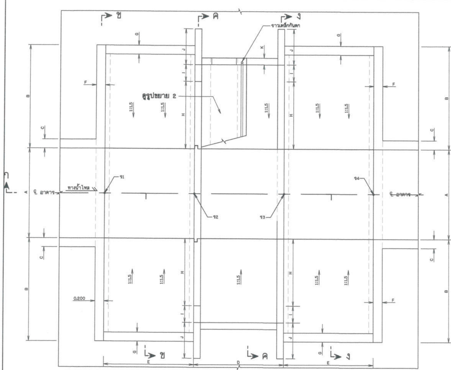
แปลนอาคารอัดน้ำ ไม่แสดงขนาดบางส่วน
