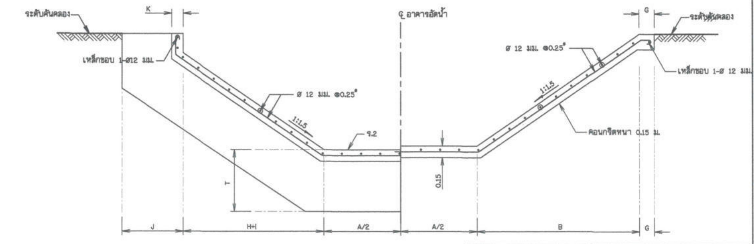
รูปตัด ง-ง ไม่แสดงขนาดบางส่วน
