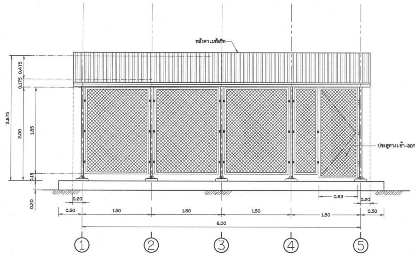
รูปด้าน 1 ไม่แสดงขนาดราวกว้าง
