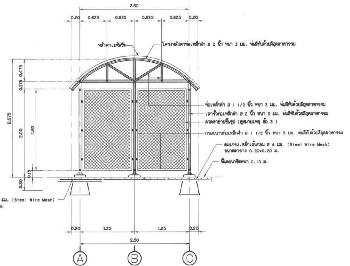
รูปตัด ข - ข โมเมนต์ขนาดจั่ว
