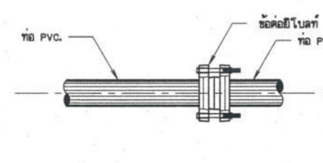
การบรรจบท่อ PVC. กับท่อ PVC.
