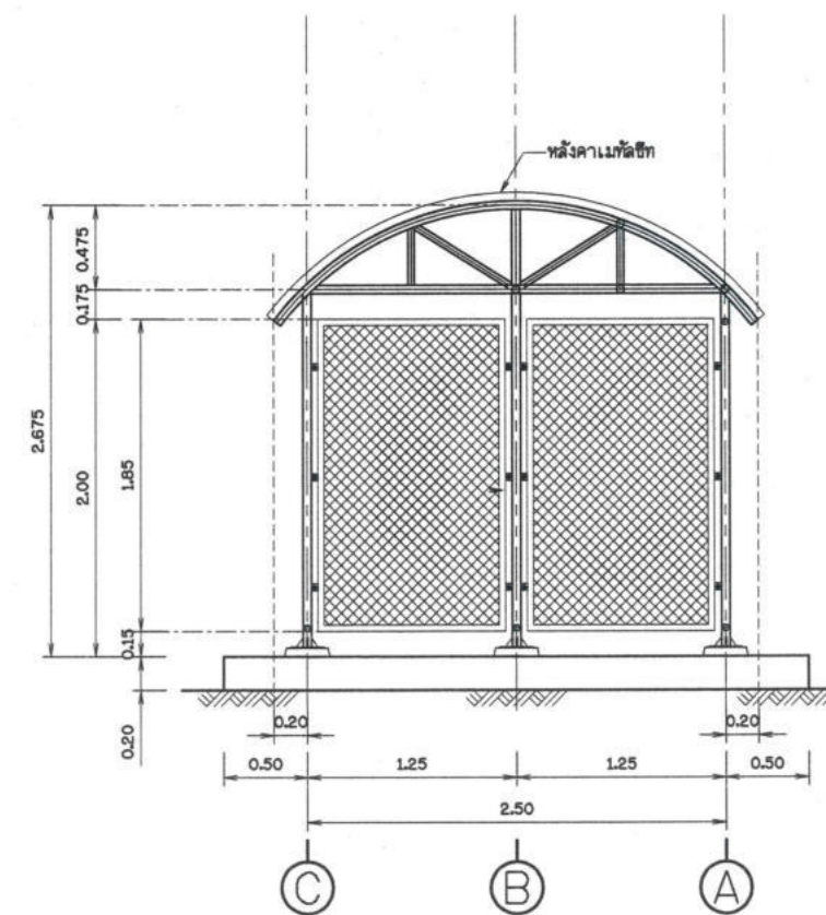
รูปด้าน 4 ไม่แสดงขนาดราวกว้าง
