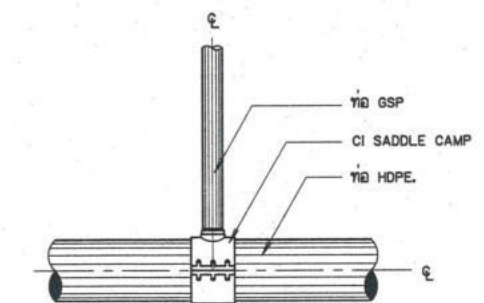
การบรรจบท่อสามทาง HDPE. กับท่อ GSP
