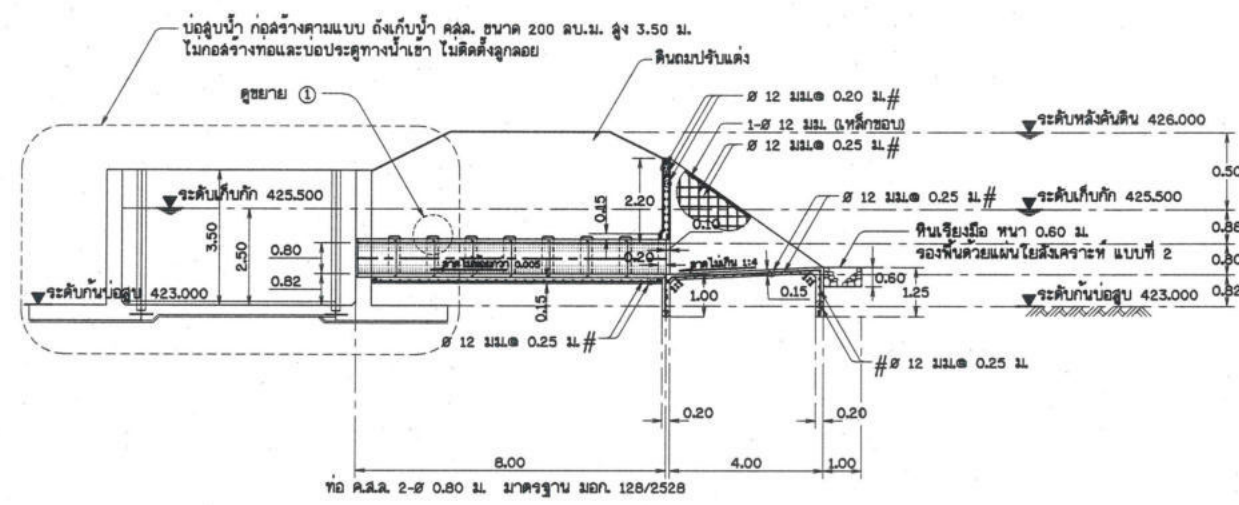
รูปตัดแนว ก - ก มาตราส่วน 1:50
