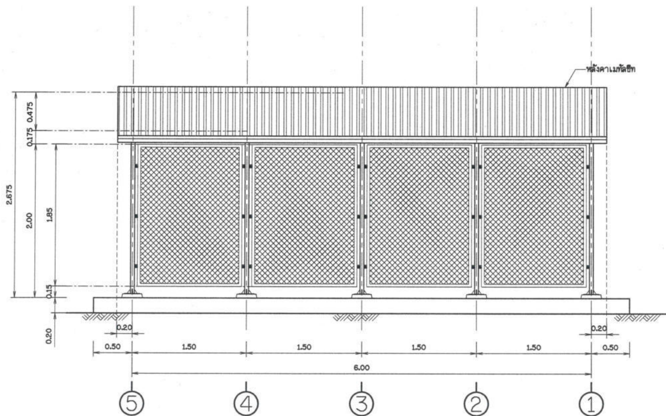
รูปด้าน 3 ไม่แสดงขนาดราวกว้าง
