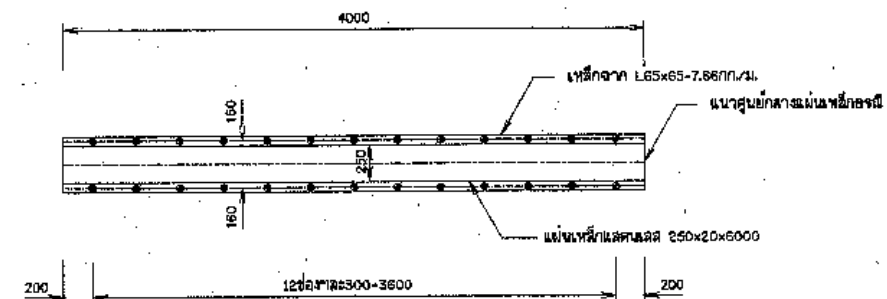
การติดตั้งเหล็กเสริม
