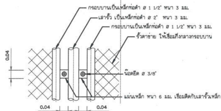
แบบขยายรายละเอียดแสดงการยืระหว่างรื้อกับเสา
