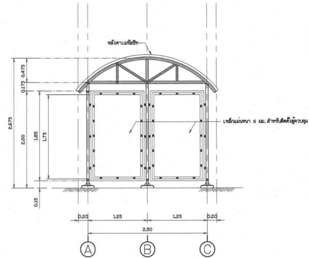
รูปด้าน 2 โมเดลขนาดจริง
