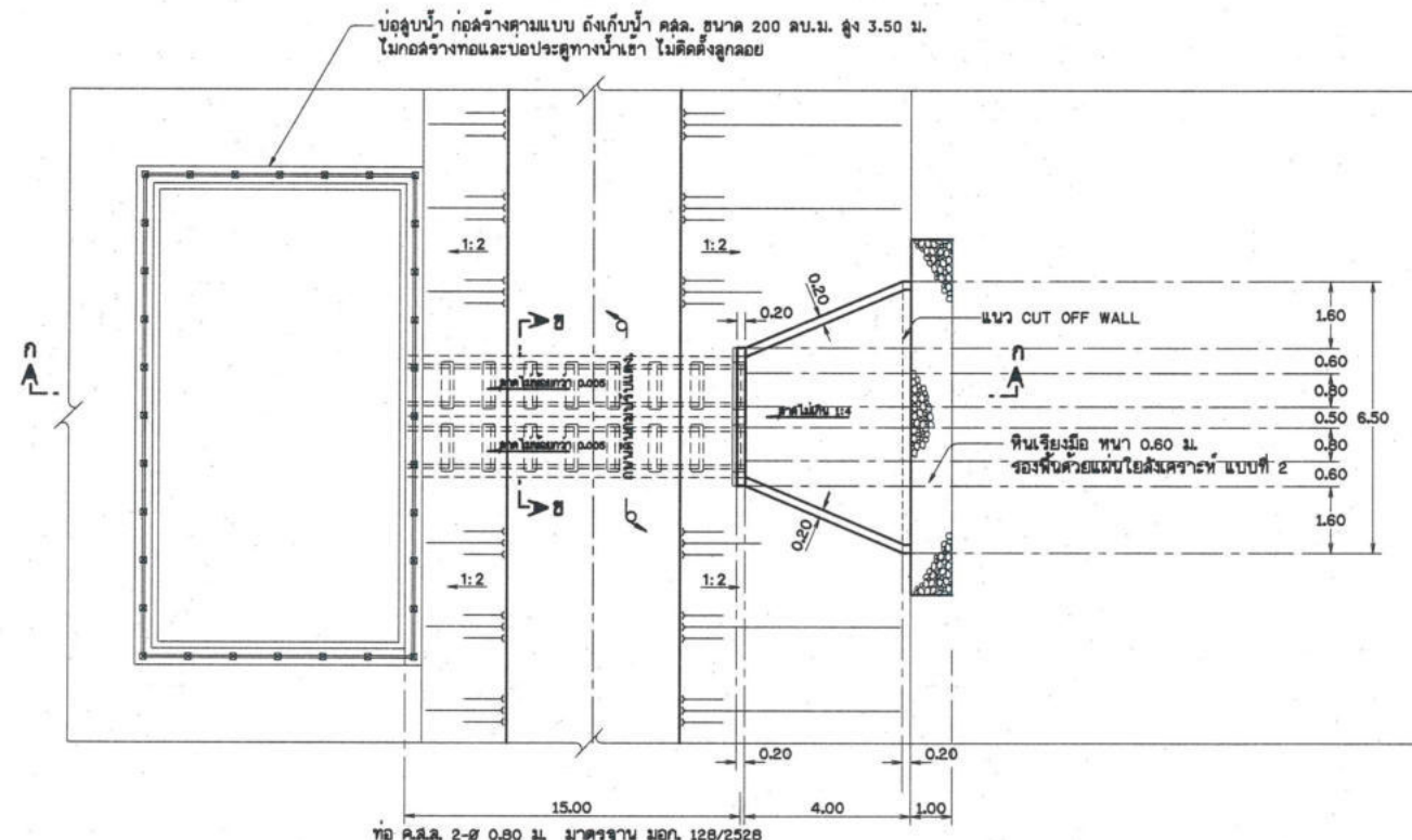
แปลนอาคารท่อทางน้ำเข้าบ่อสูบน้ำ มาตราส่วน 1:50
