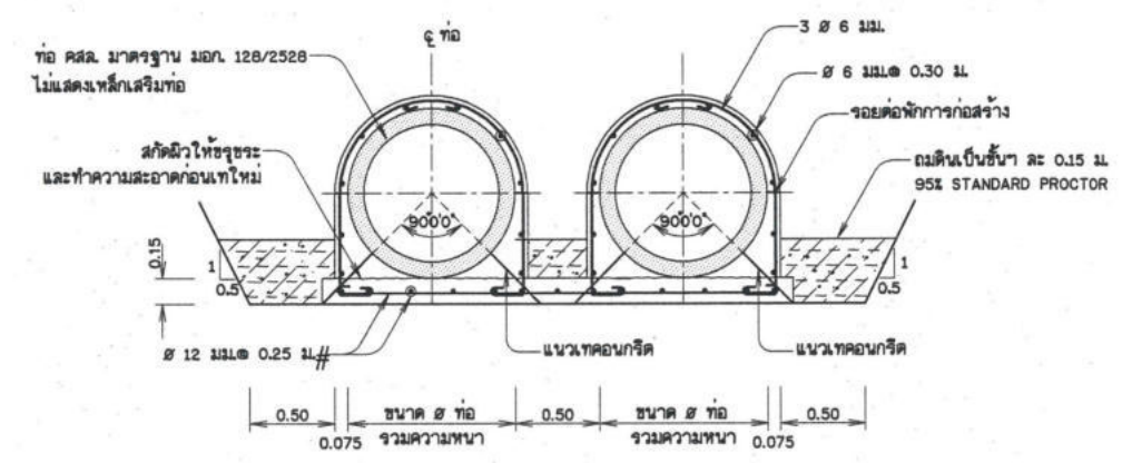
รูปตัดแนวนอน ข - ข มาตราส่วน 1:25
