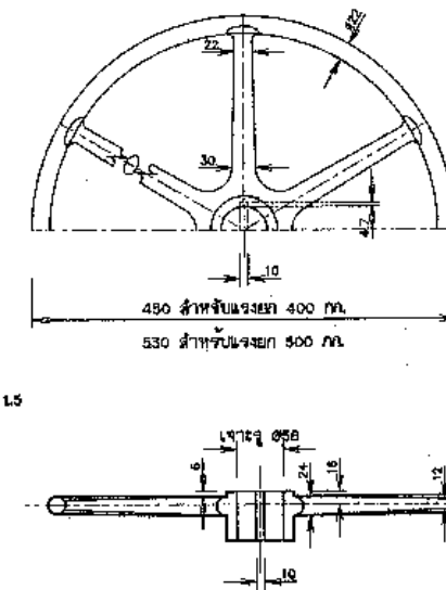
② ล้อมือหมุน มาตราส่วน 1:5 เหล็กหล่อ
