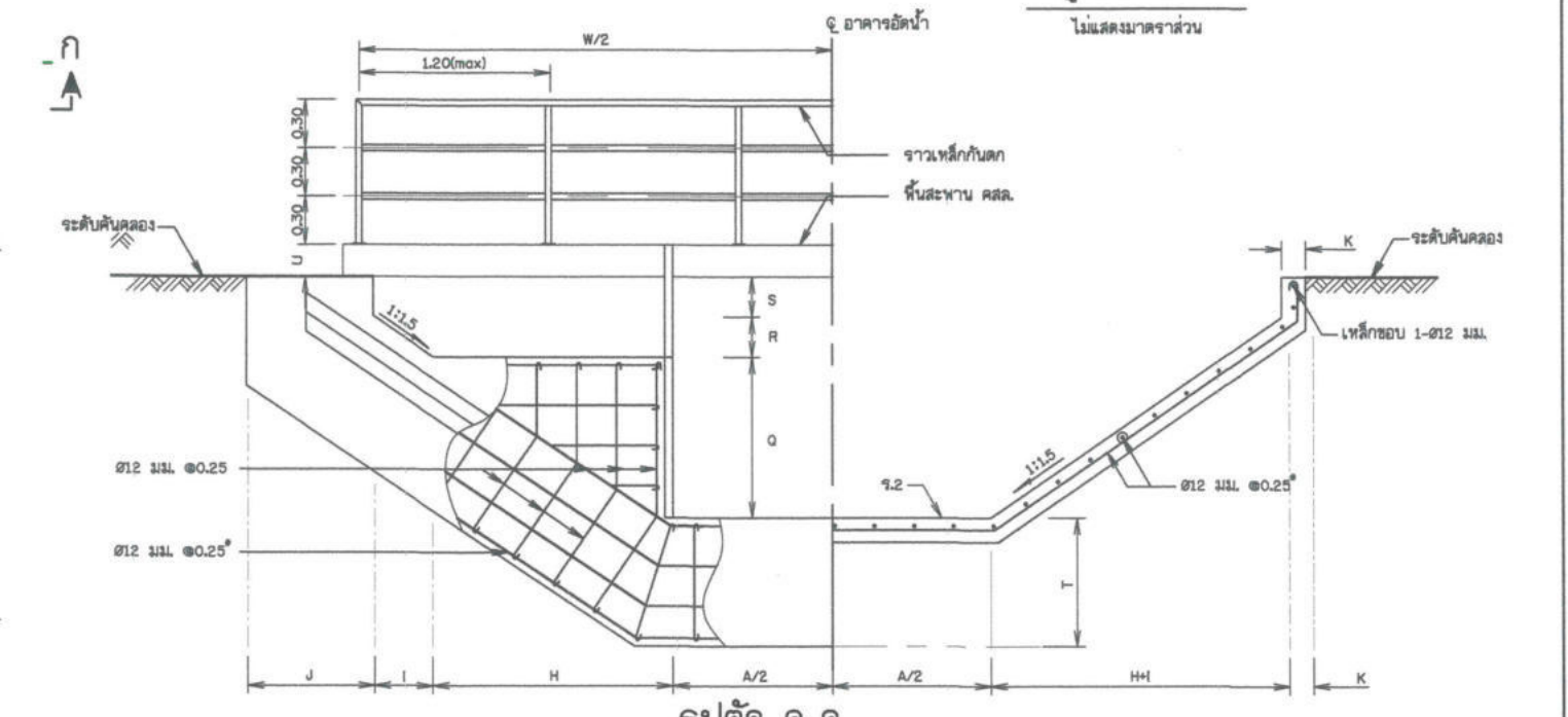
รูปตัด ค-ค ไม่แสดงขนาดบางส่วน
