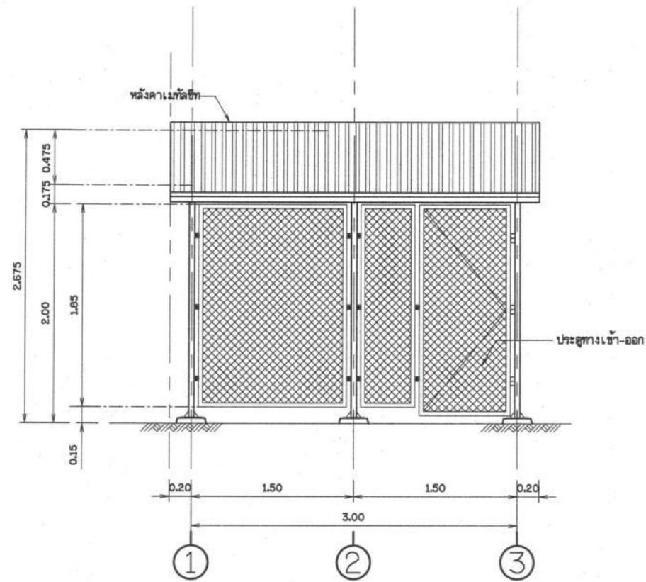
รูปด้าน 1 โมเดลขนาดจริง
