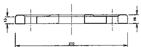
① ฐาน มาตราส่วน 1:2 เหล็กหล่อ
