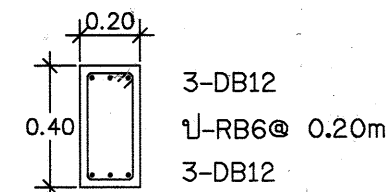
แบบขยายโครงสร้างคาน BA SCALE 1:100
