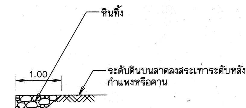
ขยายขึ้น ๑ ถึง ๒
