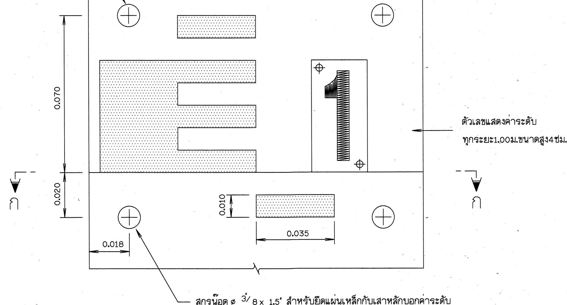
ขยายแผ่นหลักบอกระดับน้ำ
