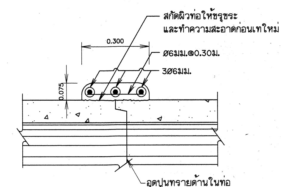
รูปตัด ข - ข
