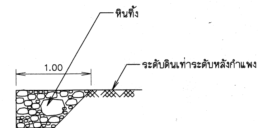
ขยายขึ้น ๑ ถึง ๒
