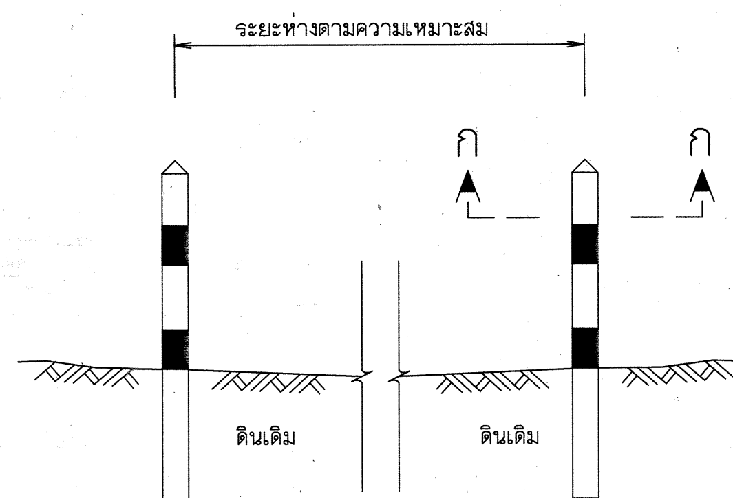
รูปขยายหลักแนวท่อ ค.ส.ล. มาตราส่วน 1:20
