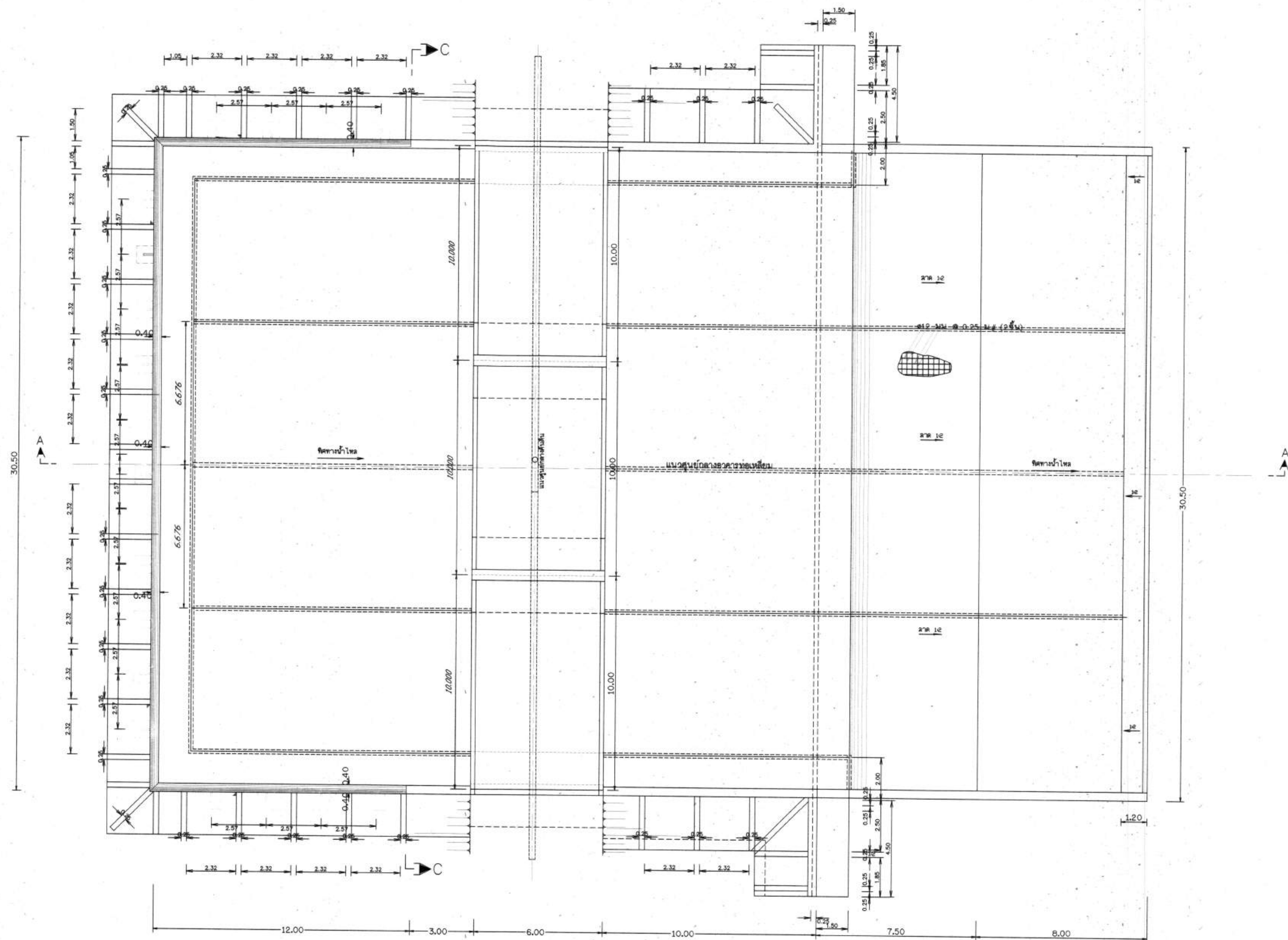
แปลนอาคารระบายนํ้า มาตราส่วน 1:100
