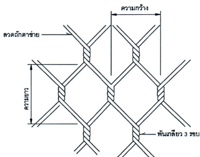
รูปที่ ๒ ลักษณะเกลียวกล่องลวดตาข่ายเหล็กเคลือบสังกะสีผสมอลูมิเนียม GABIONS
