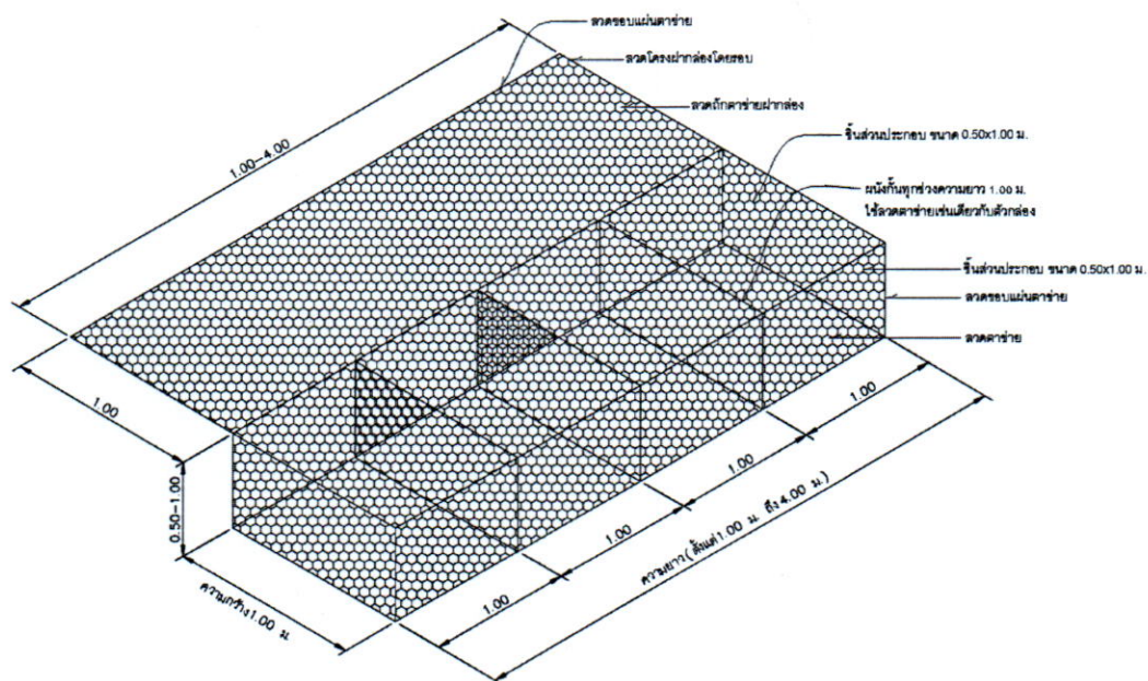
รูปที่ ๑ ขนาดกล่องลวดตาข่ายเหล็กเคลือบสังกะสีผสมอลูมิเนียม GABIONS
