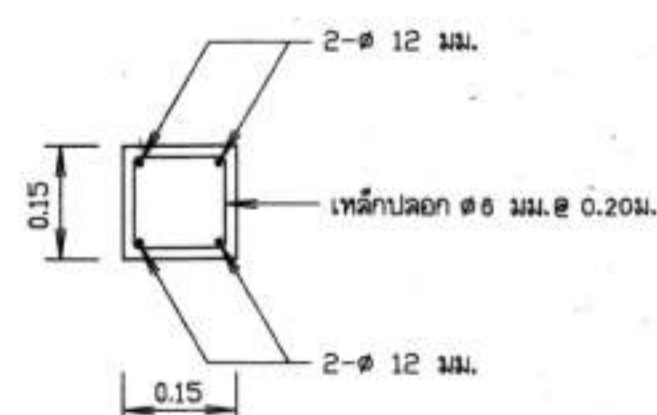
รูปตัด 1 - 1 มาตราส่วน 1:40
