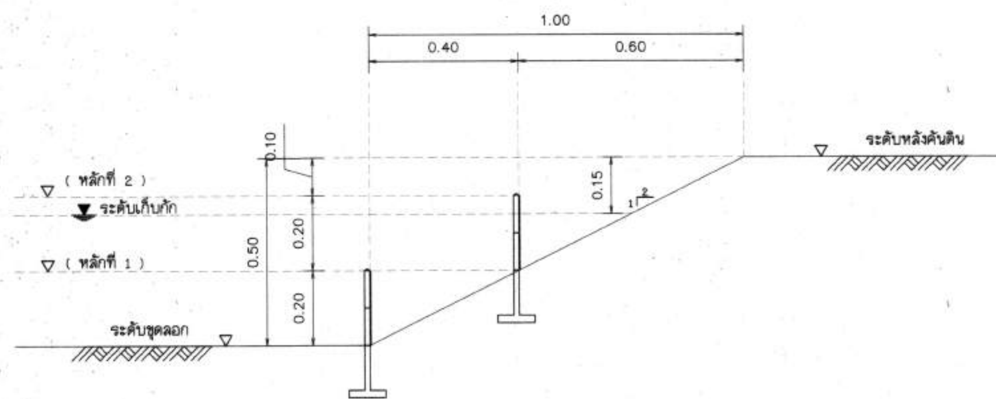
รูปตัดทั่วไปแสดงตำแหน่งหลักบอกค่าระดับน้ำ
