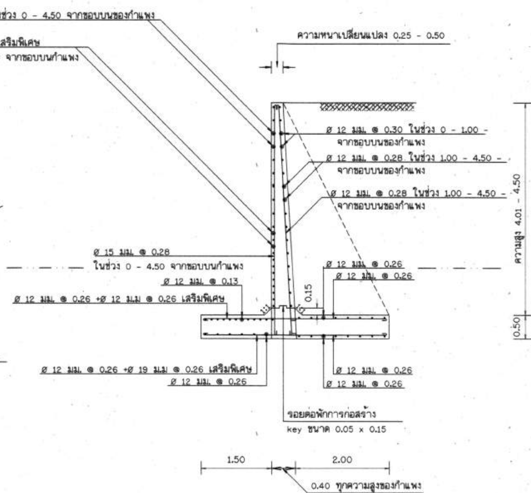
รูปตัดตามขวางของกำแพงบึ่งกลางช่วง มาตราส่วน 1 : 50
