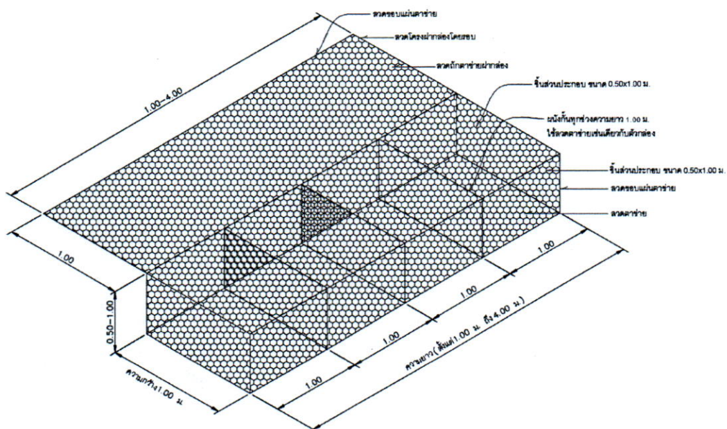
รูปที่ ๑ ขนาดกล่องลวดตาข่ายเหล็กเคลือบสังกะสีผสมอลูมิเนียม GABIONS
