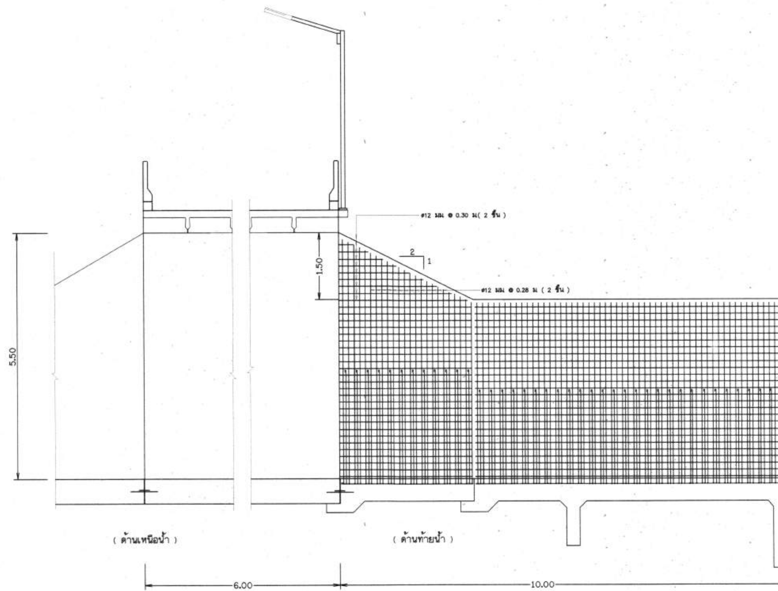
รูปตัดขยายการเสริมเหล็กจากบนลงล่าง 1.50 ม. มาตราส่วน 1:50
