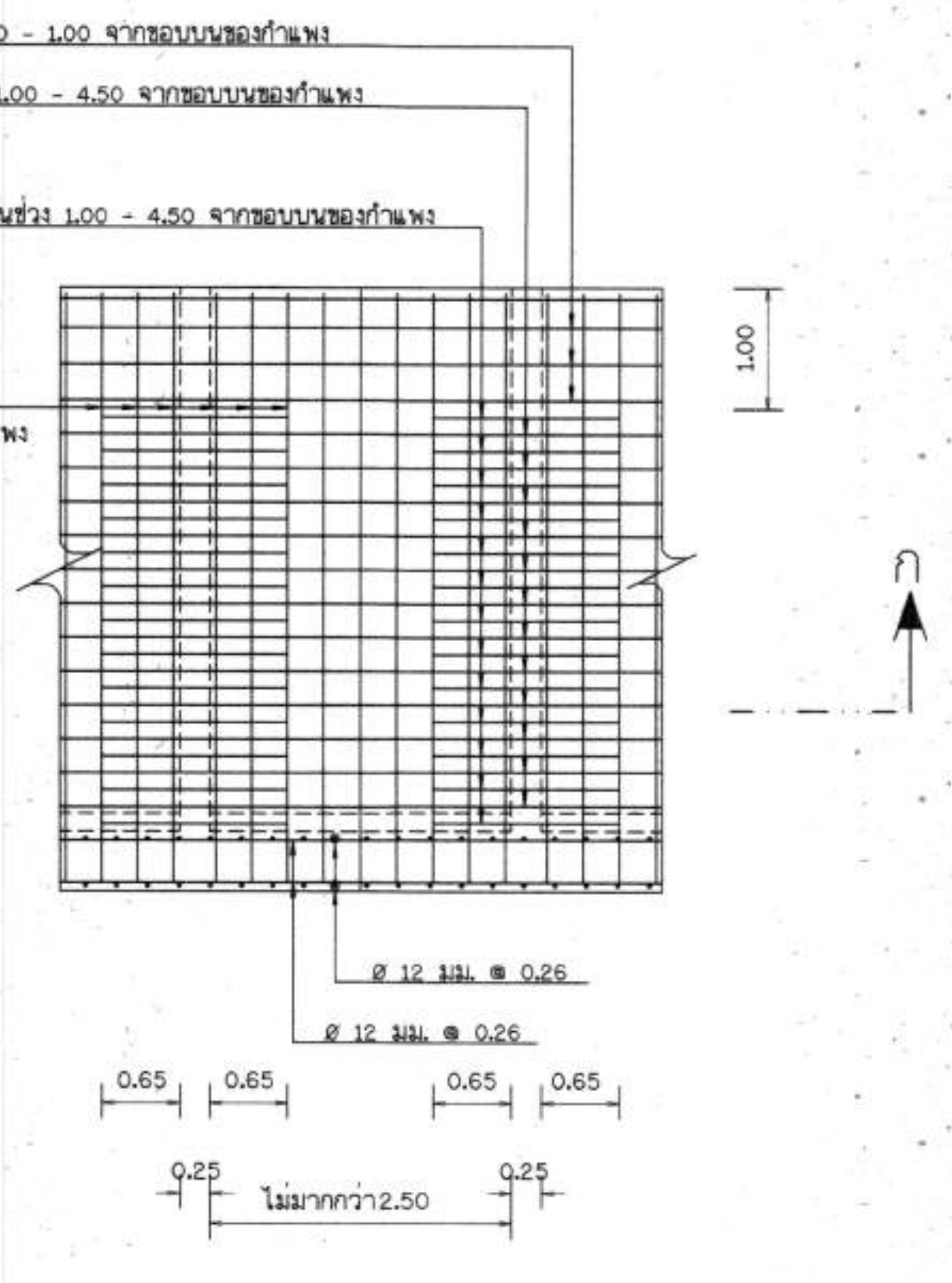
รูปตัดตามยาวของกำแพงบ้านติดดิน มาตราส่วน 1 : 50
