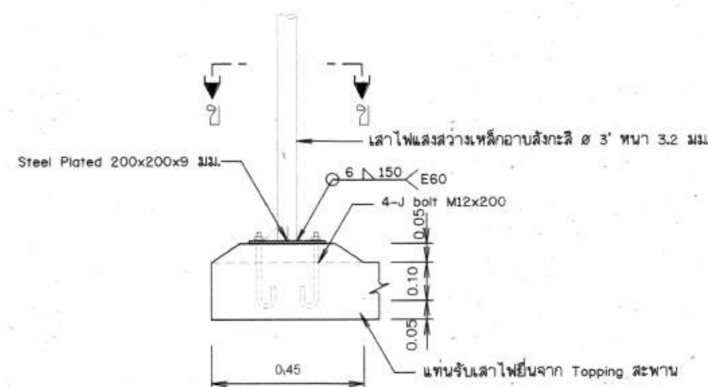
รูปขยายฐานรับเสาไฟฟ้าพลังแสงอาทิตย์ ไม่แสดงมาตราส่วน
