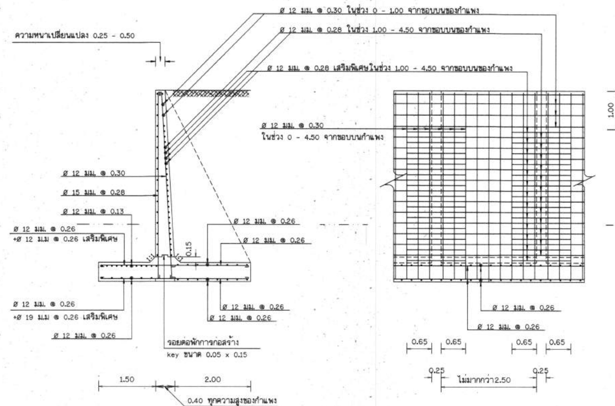
รูปตัดตามขวางของกำแพงบึ่งค้ำยัน มาตราส่วน 1 : 50
