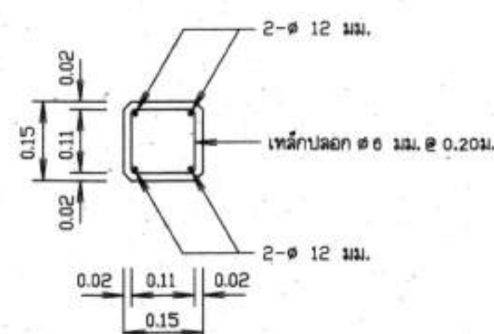
รูปตัด 2 - 2 มาตราส่วน 1:40
