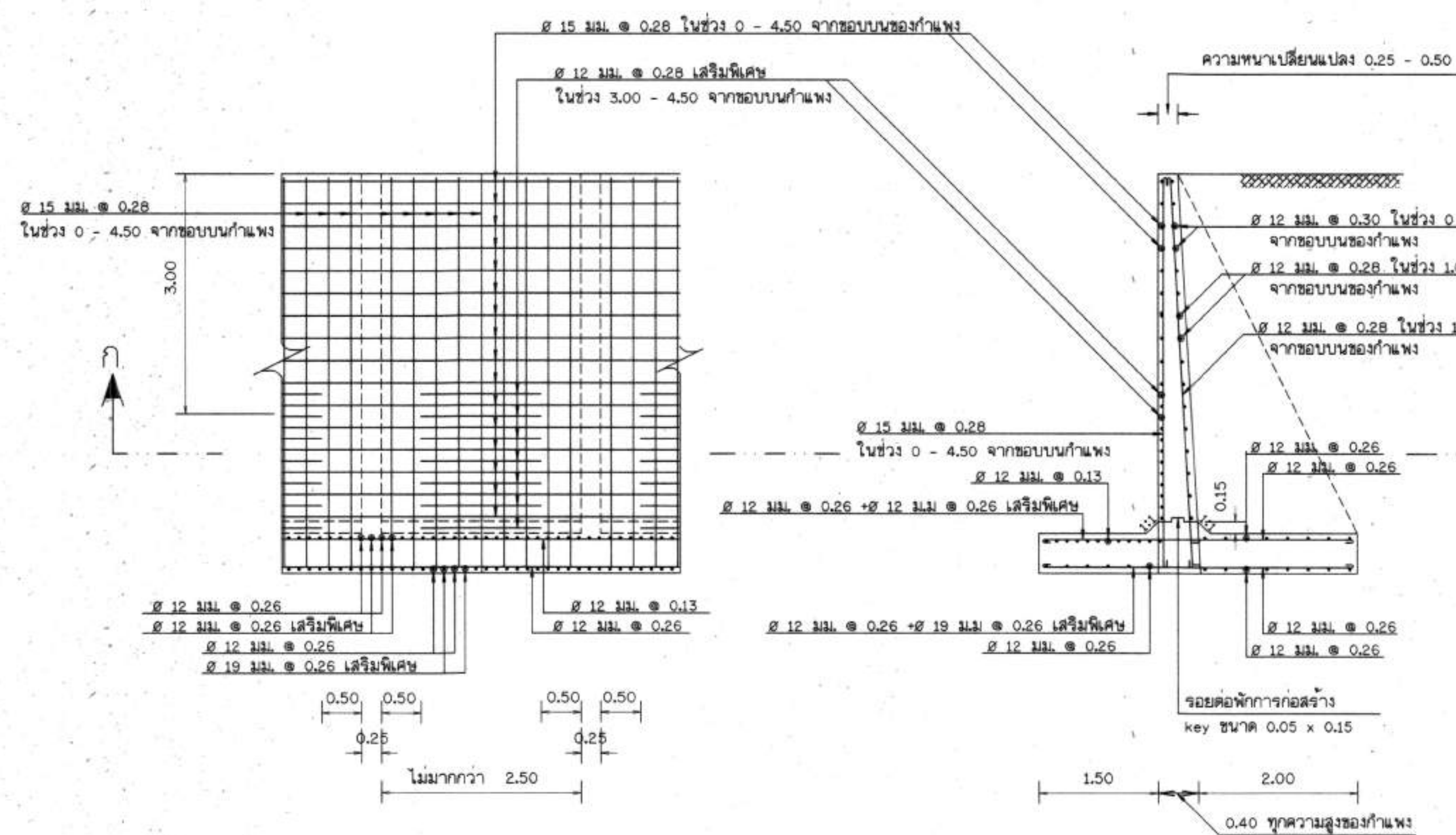
รูปตัดตามยาวของกำแพงบ้านไม้ติดดิน มาตราส่วน 1 : 50
