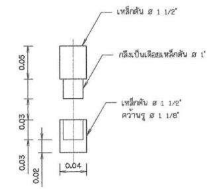
แบบขยายบานพับประตูเหล็ก ไม่แสดงขนาดราส่วน
