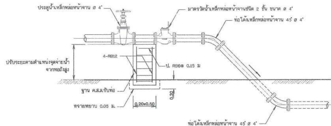
13. การติดตั้งมาตรวัดน้ำบนพื้นดิน 4" ไม่แสดงขนาดจาล้วน
