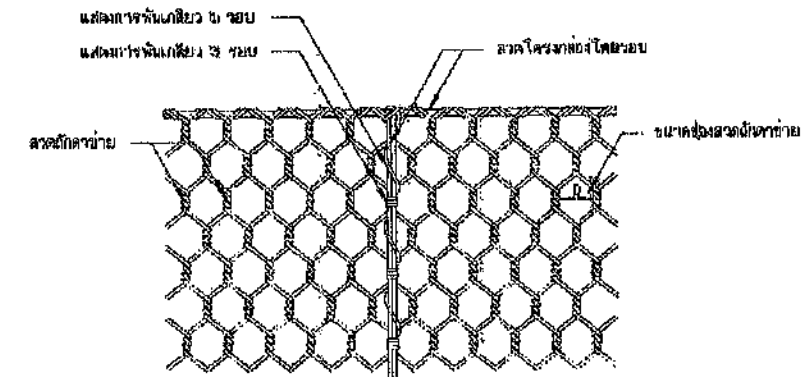
รูปแสดงการผันลวดระหว่างกล่องลวดตาข่ายและฟาบิด
