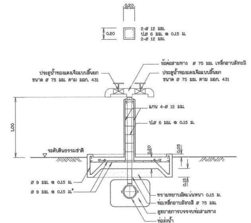
รูปตัด ก - ก
