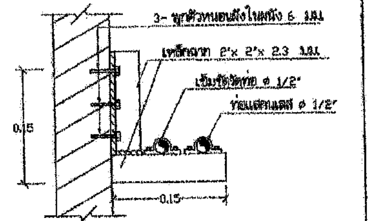
ขยายเหล็กรับท่อสารส้มของไฮดรอลิค 1:5
