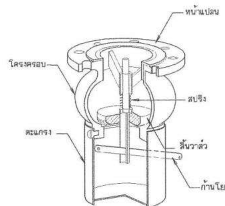
ฟุตวาล์ว แบบกันโยก ไม่แสดงขนาดจาล้วน
