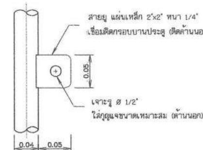
แบบขยายสายยู
