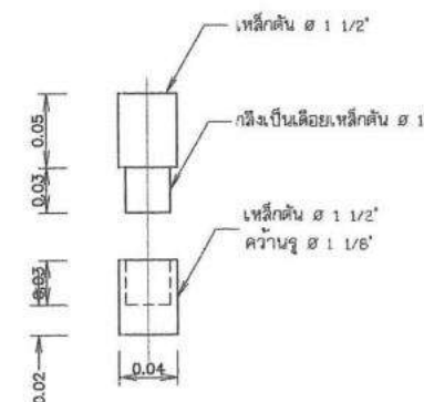
แบบขยายบานพับหัวเหล็ก
