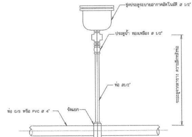
12. การติดตั้งประตูปรับอากาศอัตโนมัติ ไม่แสดงขนาดจาล้วน
