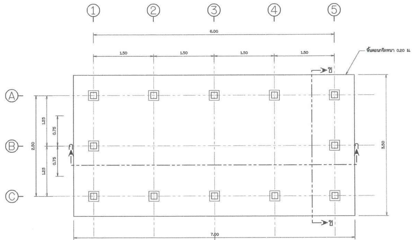
แบบแปลน ไม้แฉดขนาดจาล้วน
