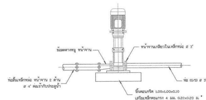
14. การต่อท่อเครื่องสูบน้ำ ไม่แสดงขนาดจาล้วน
