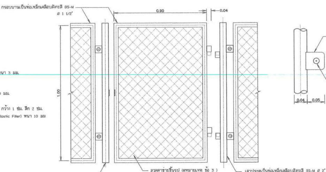
แบบขยายรายละเอียดประตู
