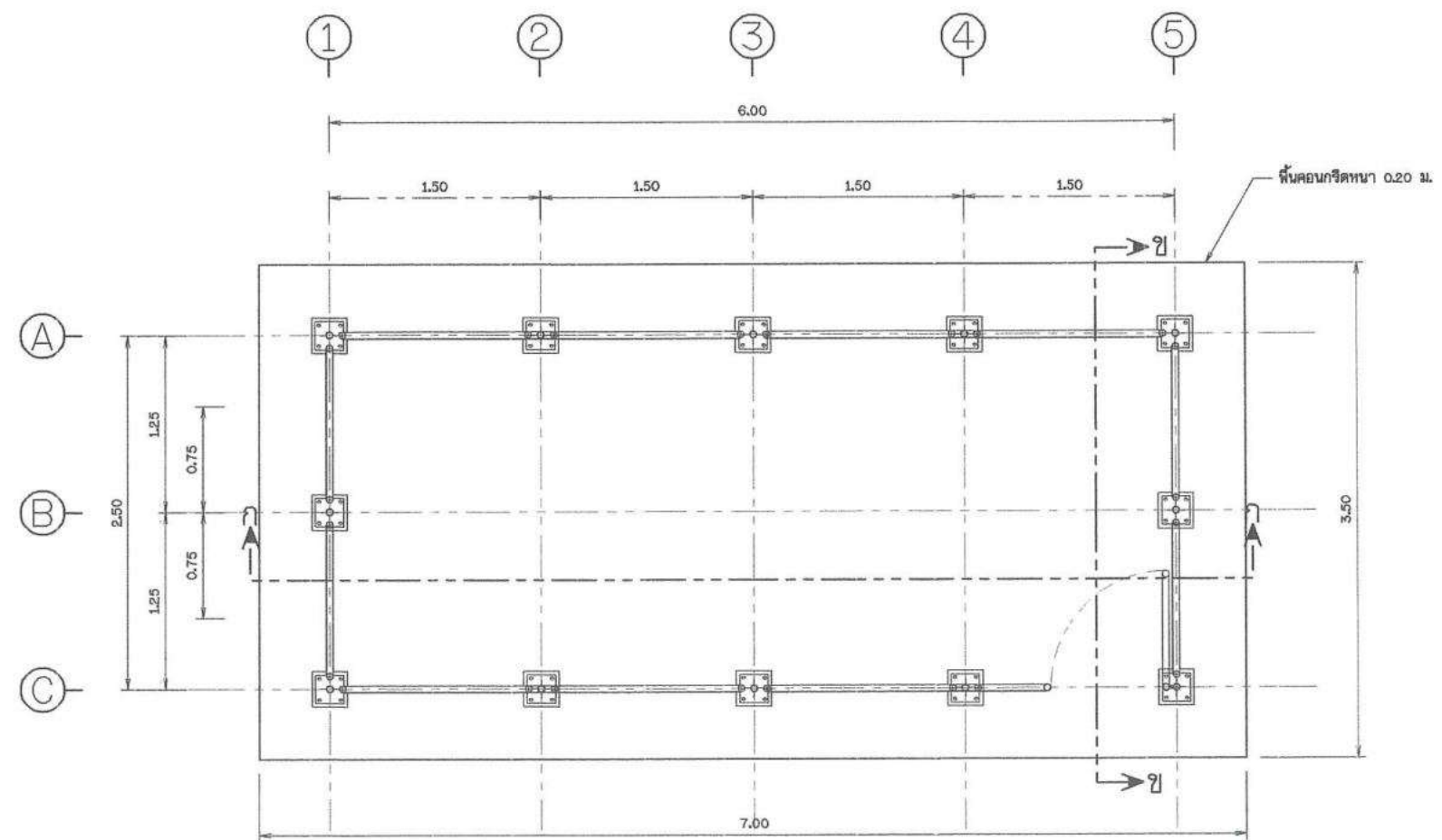
แปลนเสาและรื้อ ไม้แฉดขนาดจาล้วน
