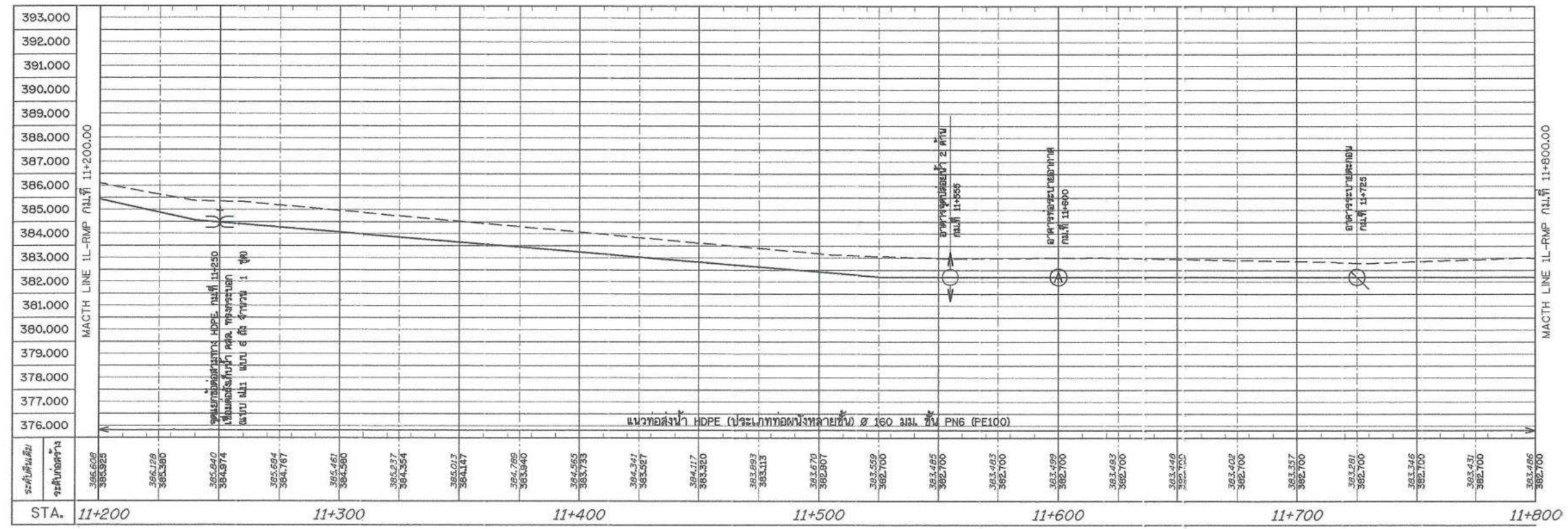
แปลนระบบส่งน้ำ สาย 1L-RMP. STA. 11+200 - 11+800 มาตรฐาน 1:1,000
