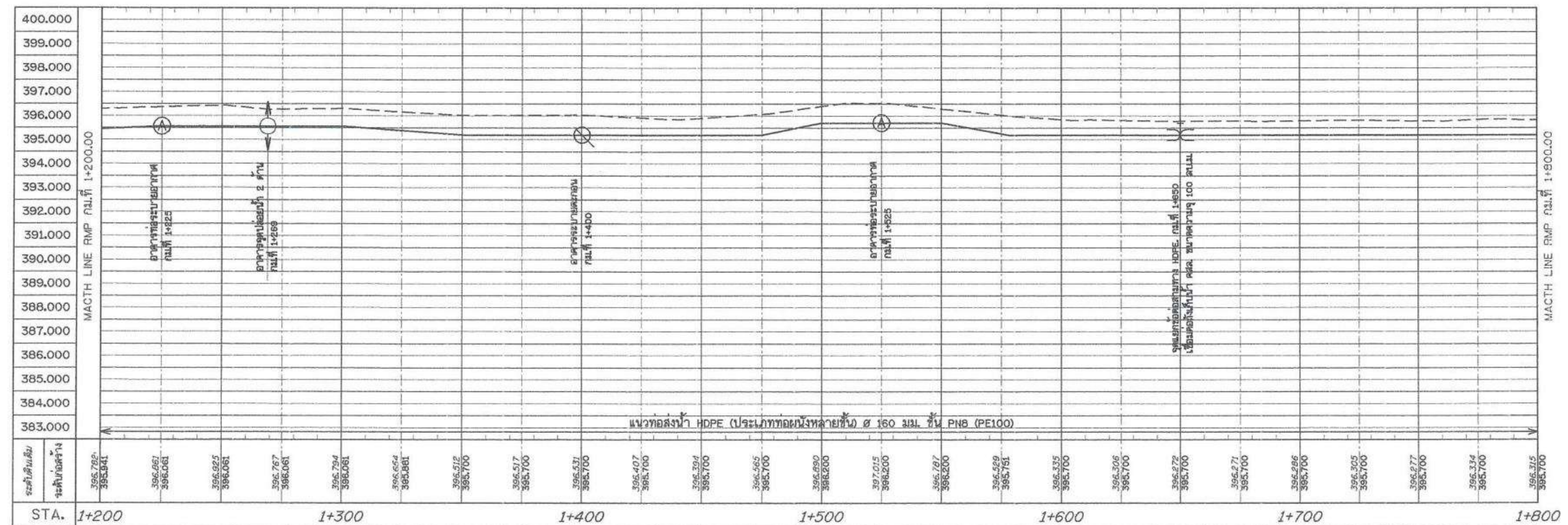
แปลนระบบส่งน้ำ สาย RMP. STA. 1+200 - 1+800 มาตรฐาน 1:1,000
