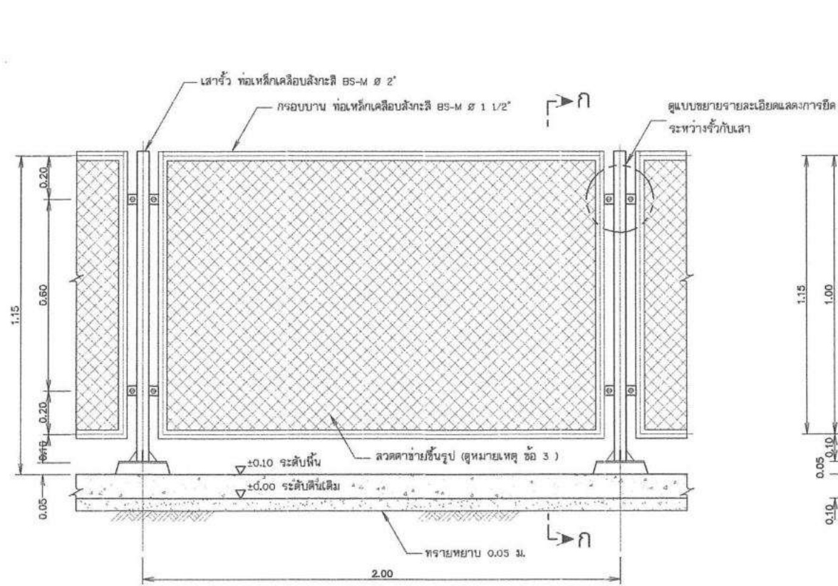
แบบขยายหัวลวดตาข่าย
