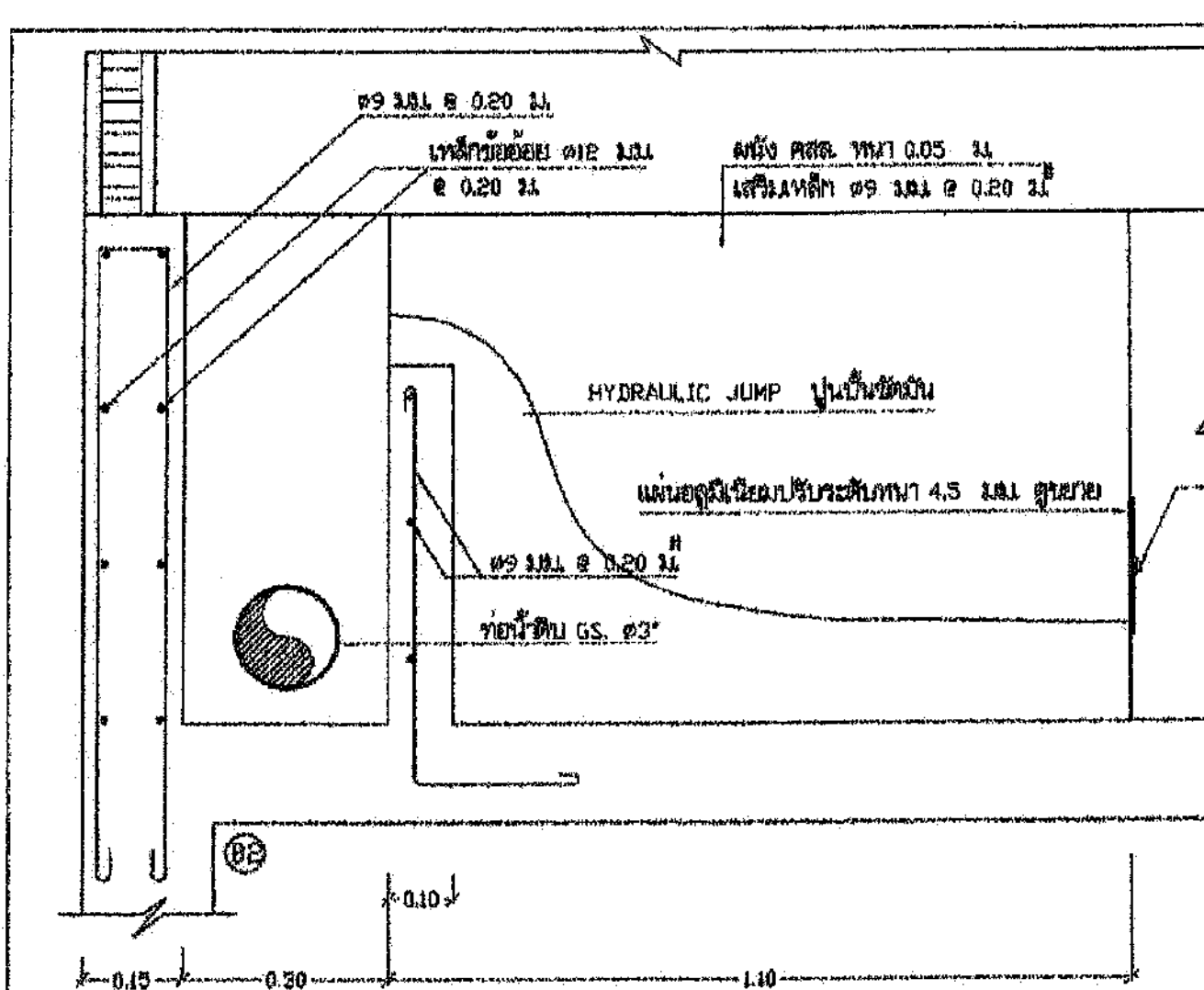
รูปตัด (A) - (B) 1 : 10
