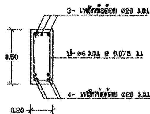
รูปตัด (B) - (B) 1:20
