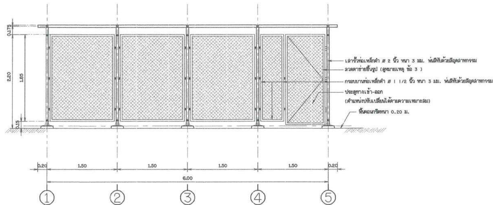
แบบขยายรั้ว 1 ไม่แสดงขนาดราส่วน
