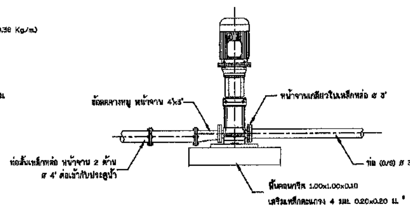
18. การต่อท่อเครื่องสูบน้ำ ไม่แสดงขนาดส่วน
