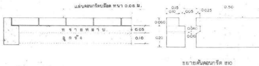
รูป ขยาย คอก ม่อ 1:5
