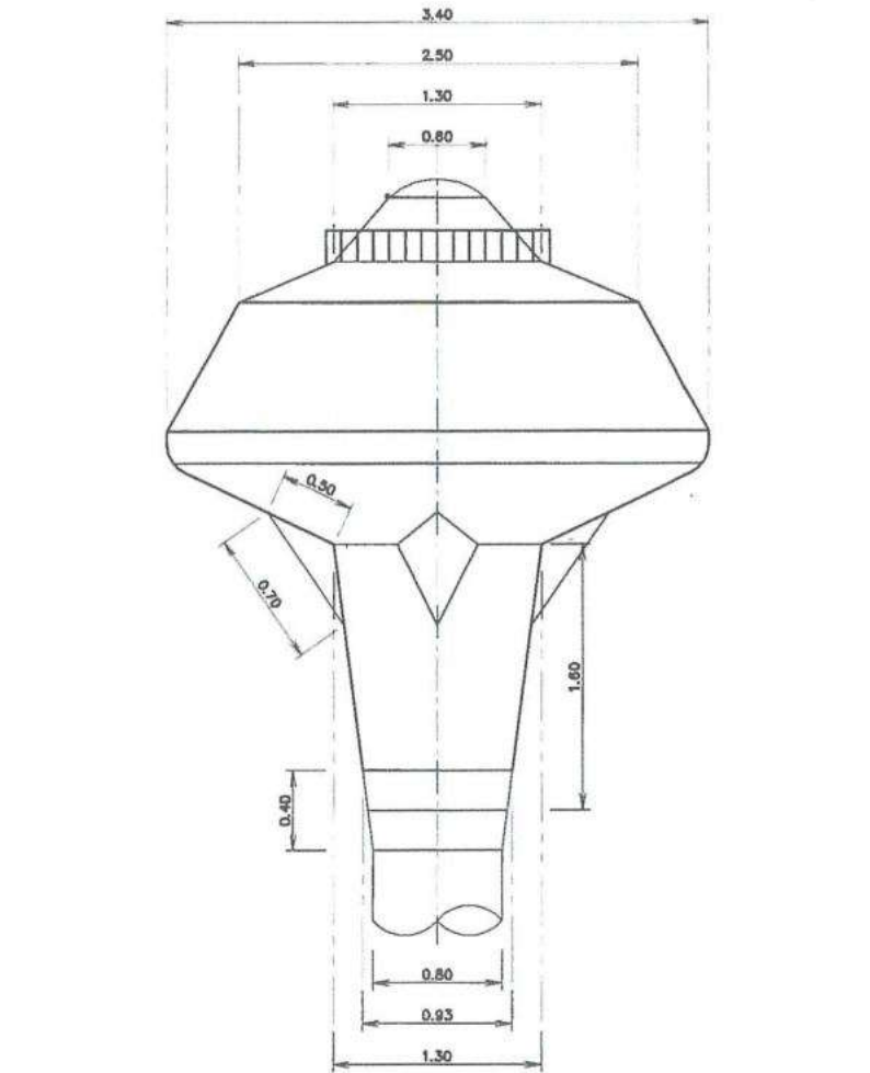
แบบขยายแมนโซลบนของถังสูง ไม่แสดงมาตราส่วน
