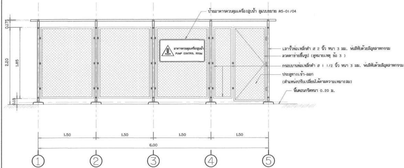
แบบขยายรั้ว 1 ไม่แสดงขนาดราวล้วน
