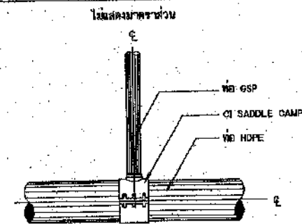
การบรรจุบ่อสามทาง HDPE กับท่อ GSP
