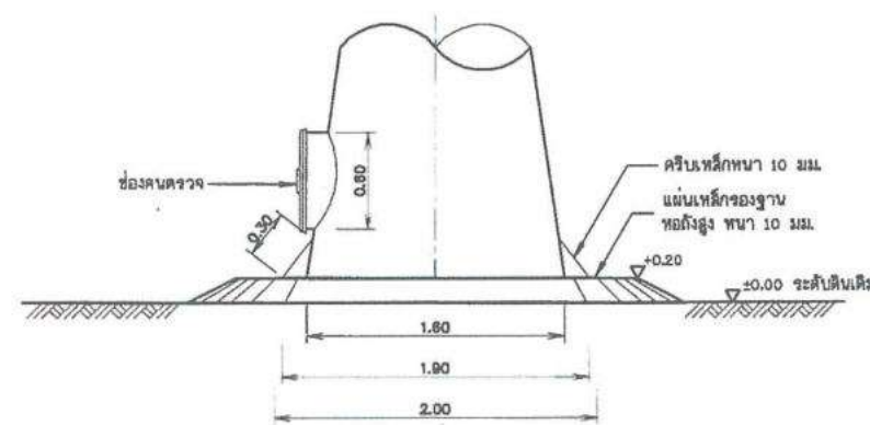
แบบขยายแมนโซลล่างของถังสูง ไม่แสดงมาตราส่วน
