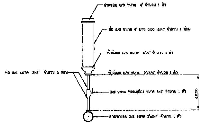
11. ช้องเดิมน้ำ ไม่แสดงขนาดส่วน
