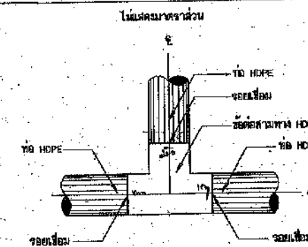
การบรรจุบ่อสามทาง HDPE กับท่อ HDPE
