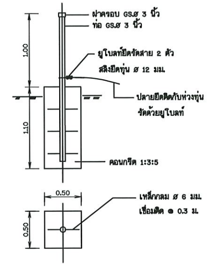
รูปขยายเสายึดแฉ มาตราส่วน 1:50
