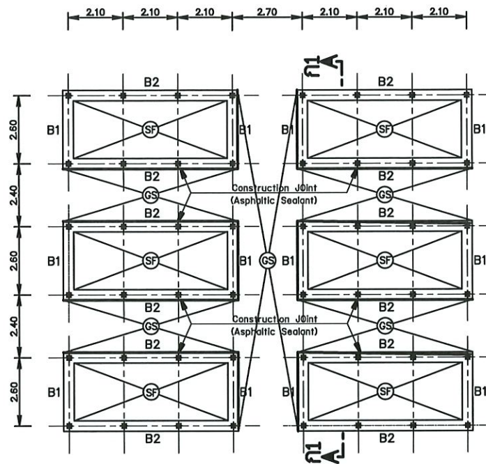
แปลนคานคอดินแผงเซลล์พลังงานแสงอาทิตย์
