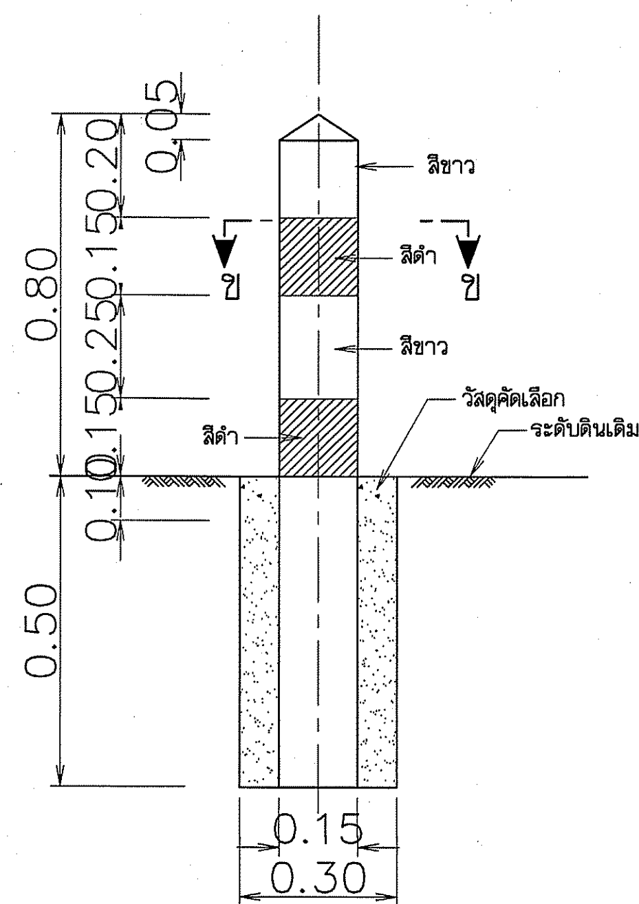
หลักริมคันดิน
