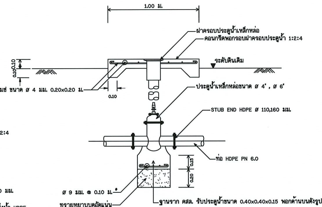
รูปตัด ค - ค แสดงการติดตั้งประตูป้ายใต้ดิน มาตราส่วน No Scale
