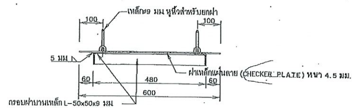
รูปตัด จ-จ
