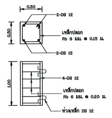
รูปขยายฐาน คสล. ยึดแฉ มาตราส่วน 1:50
