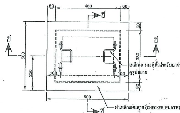
แปลน MANHOLE NO.2
