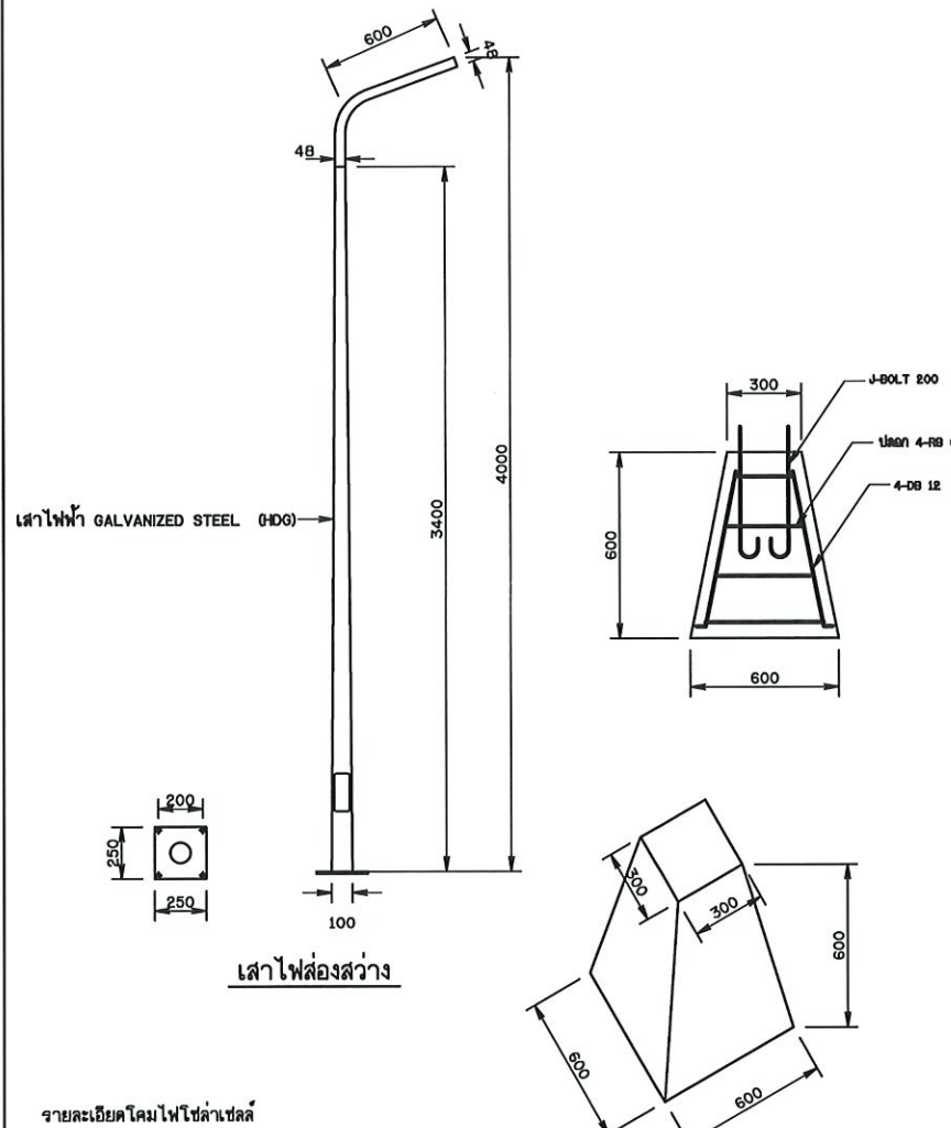
ต่อม่อเสาไฟ
