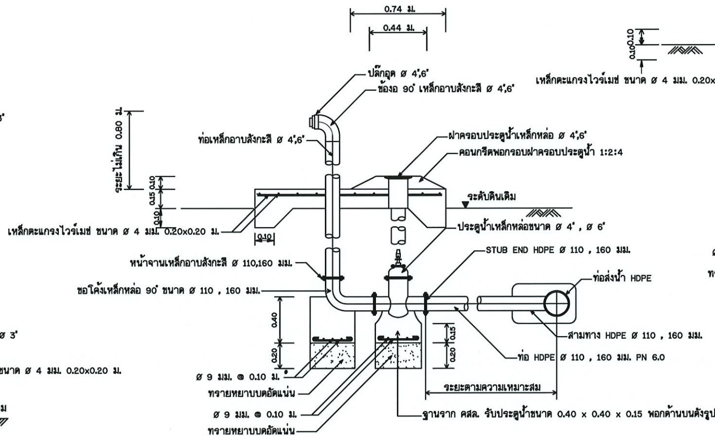
รูปตัด ข - ข แสดงการติดตั้งประตูป้ายตะกอน มาตราส่วน No Scale
