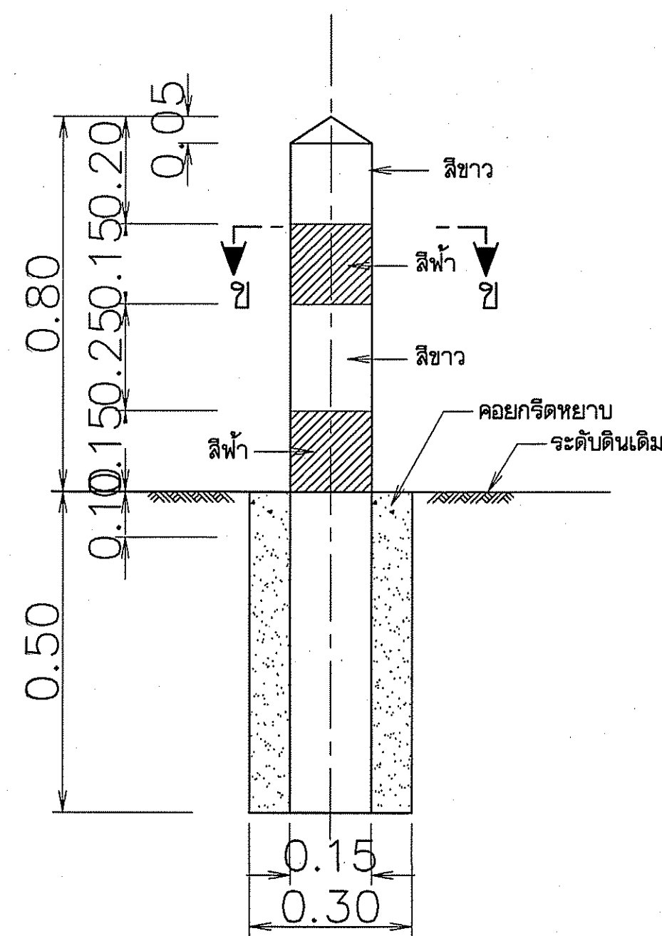
หลักบอกแนวท่อ
