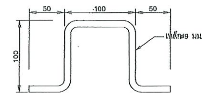
รูปขยายเหล็กหัว MANHOLE
