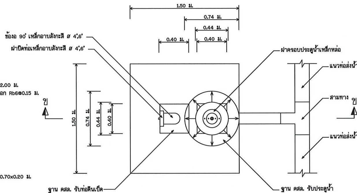
แปลนประตูป้ายตะกอน มาตราส่วน No Scale
