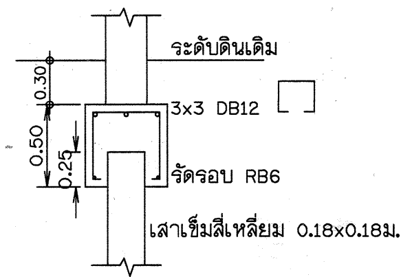
แบบขยายฐานรากอาคารควบคุม SCALE 1:100
