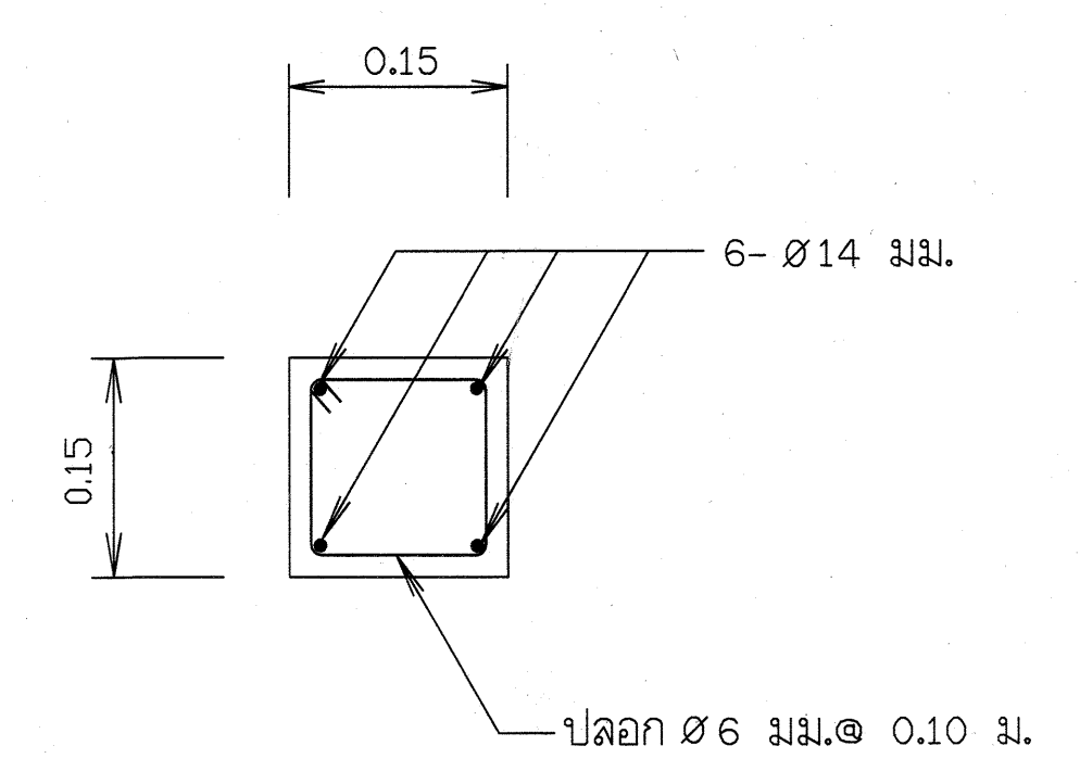
รูปตัด ก - ก มาตรฐาน 1:5
