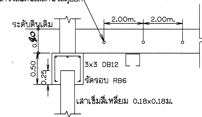
แบบขยายฐานรากรับคานหัว (FE) มาตราส่วน 1:100
