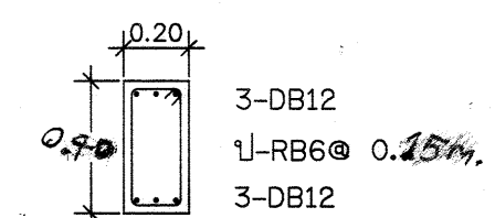
แบบขยายโครงสร้างคานหัว (BE) SCALE 1:100
