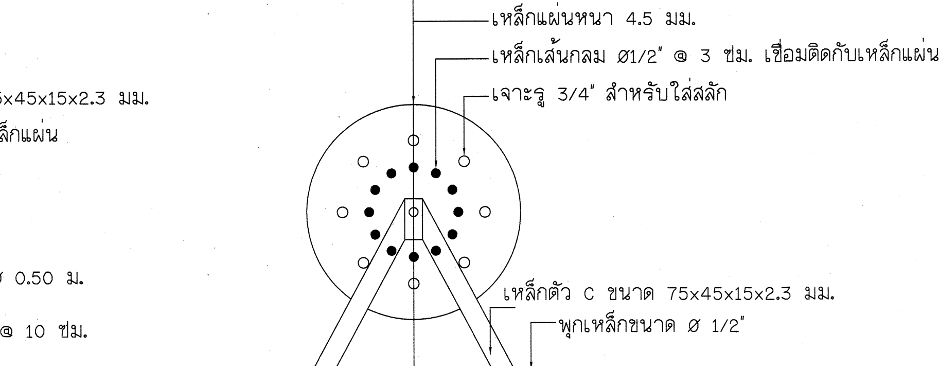
รูปขยายบันได
