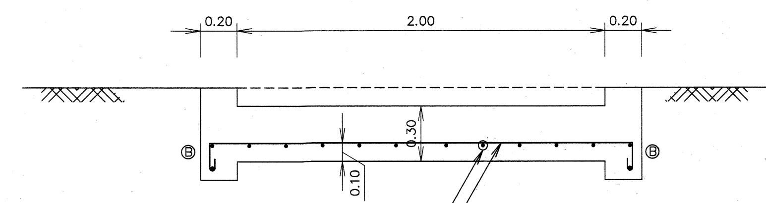
รูปตัด ข - ข มาตราส่วน 1:20
