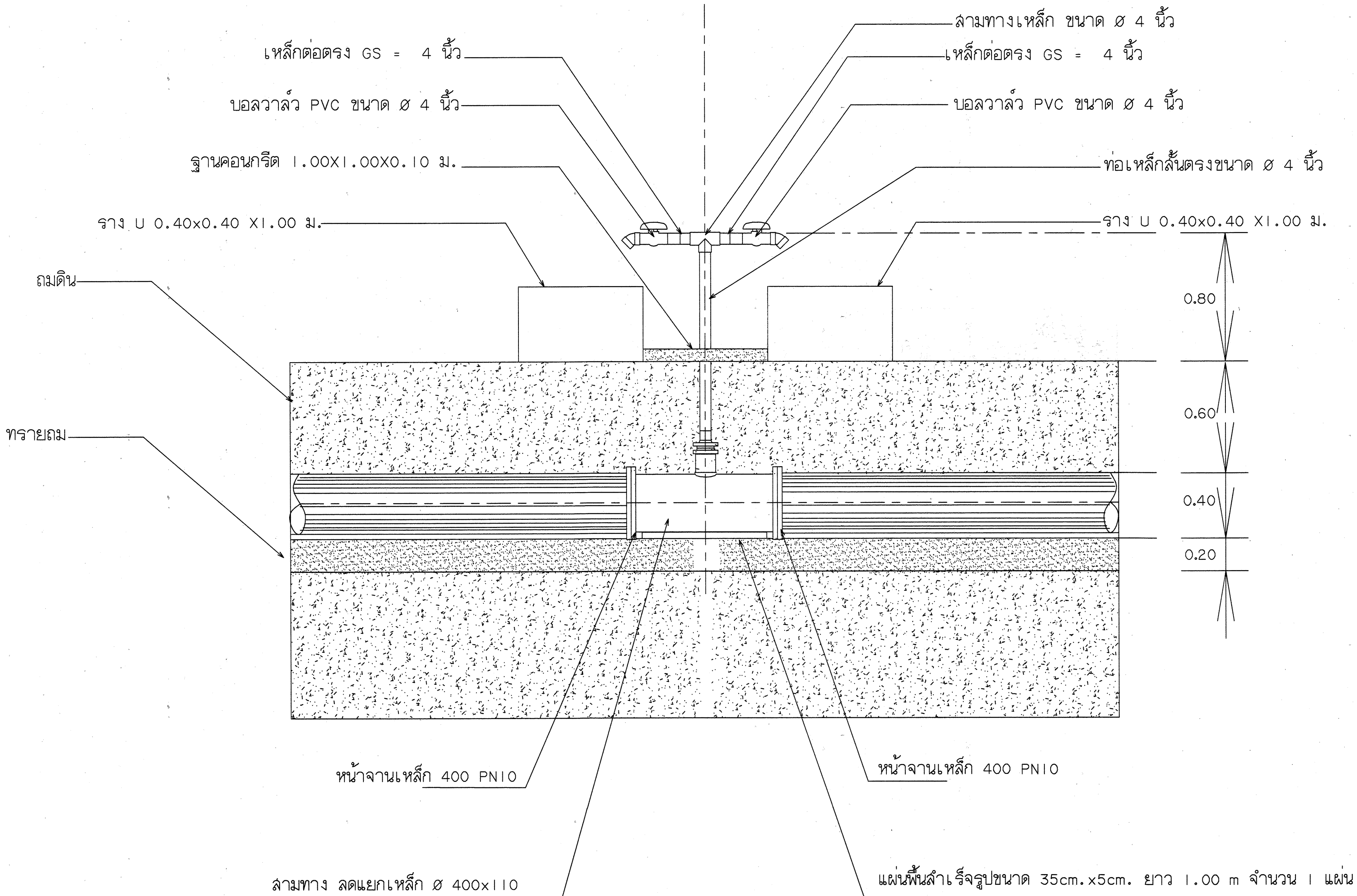
รูปตัด ราง U
