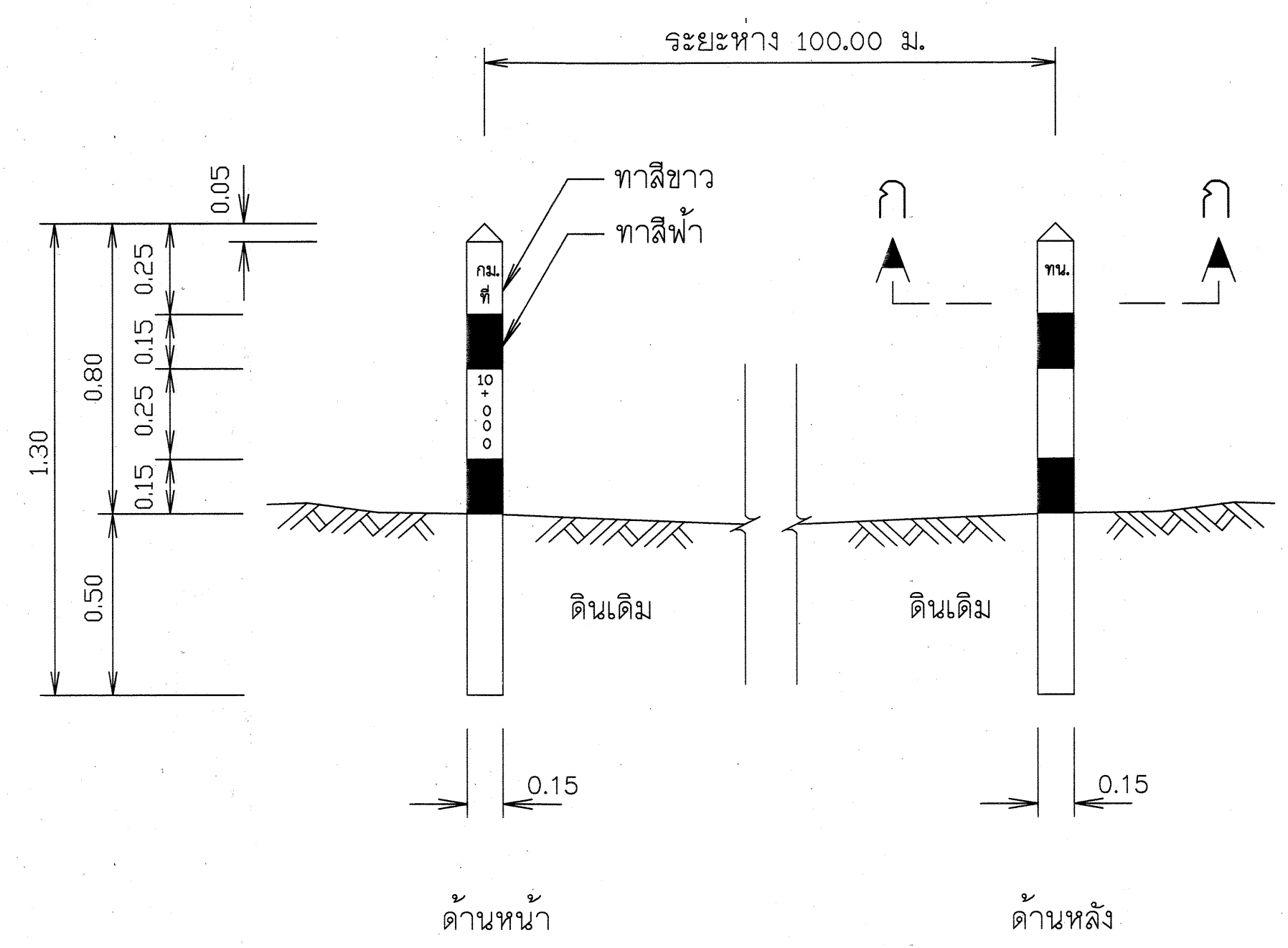
รูปขยายหลักแนวทอ คสล. มาตรฐาน 1:20
