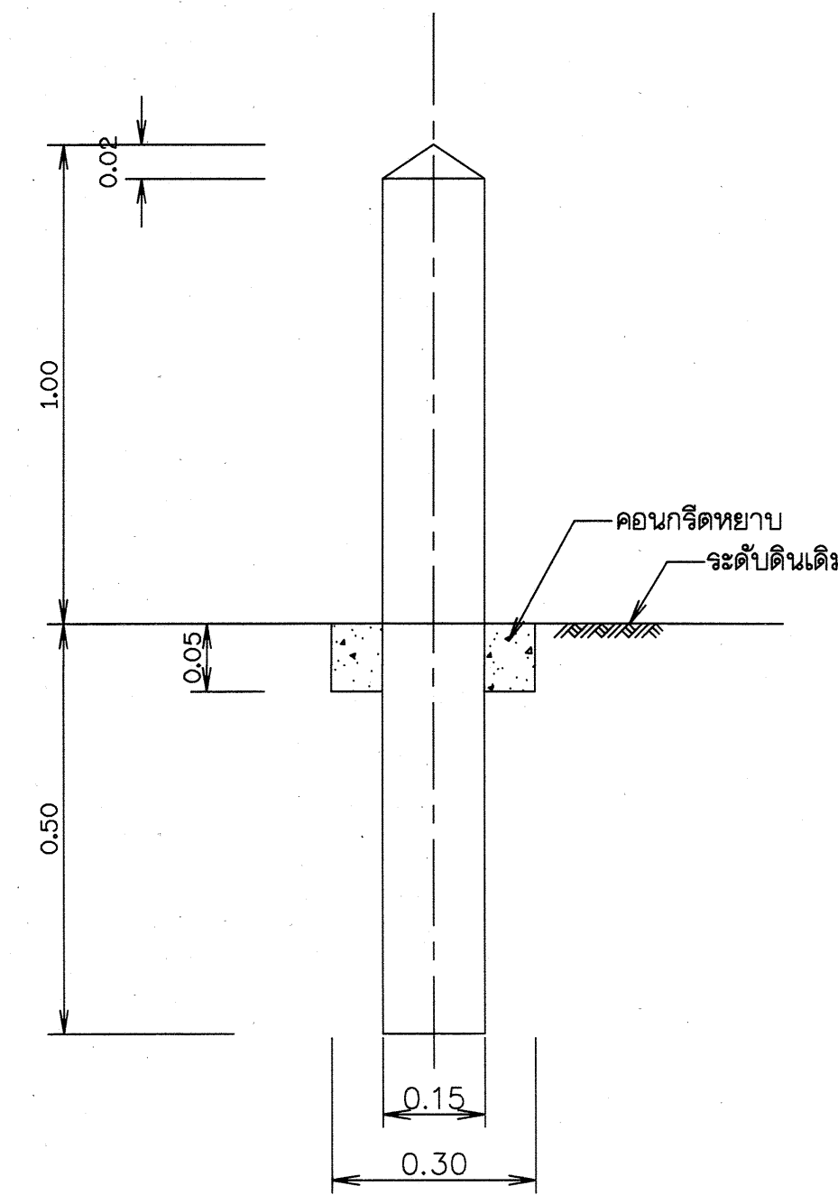
รูปตัด ก-ก แบบที่ 2 แล่ดงจุดหักเลี้ยว ไม่แล่ดงมาดราล่วน
