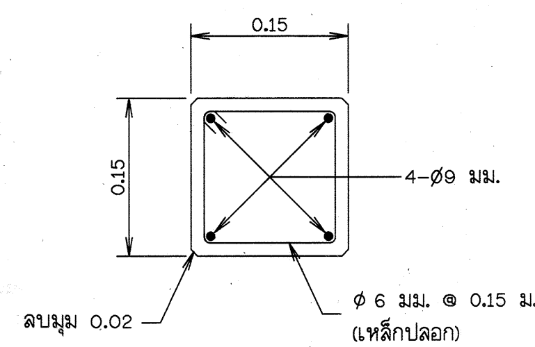
รูปตัด ข-ข ไม่แล่ดงมาดราล่วน
