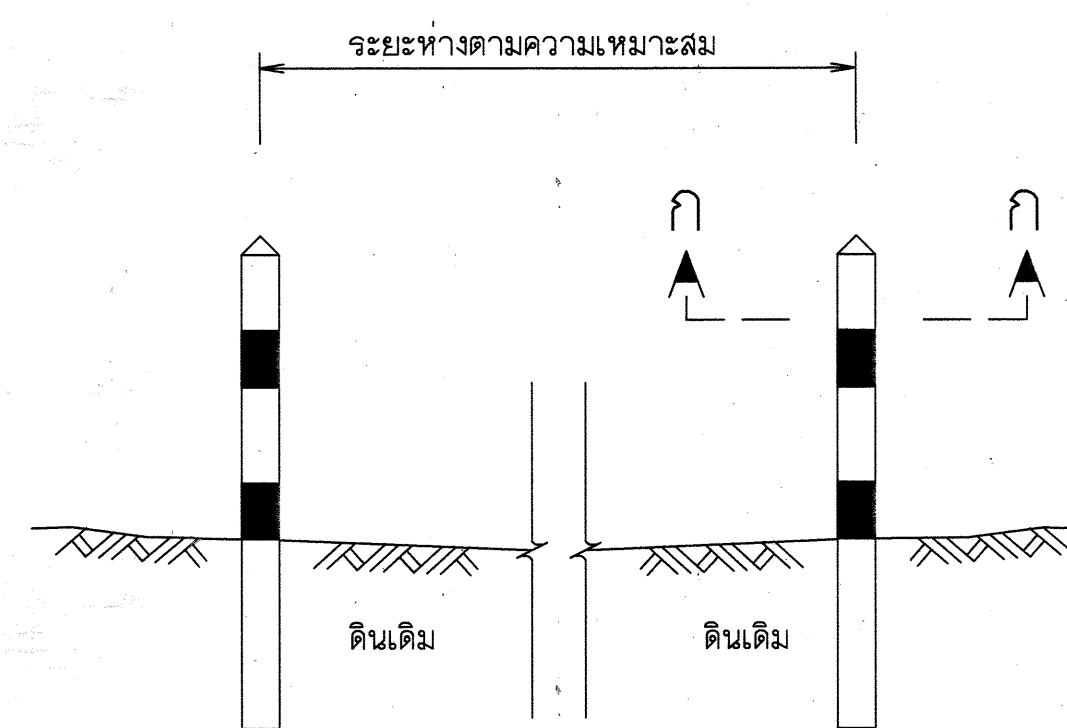
รูปขยายหลักแนวท่อ ค.ล.ล. มาดราล่วน 1:20
