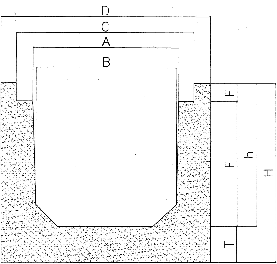
รูปตัด ราง U
