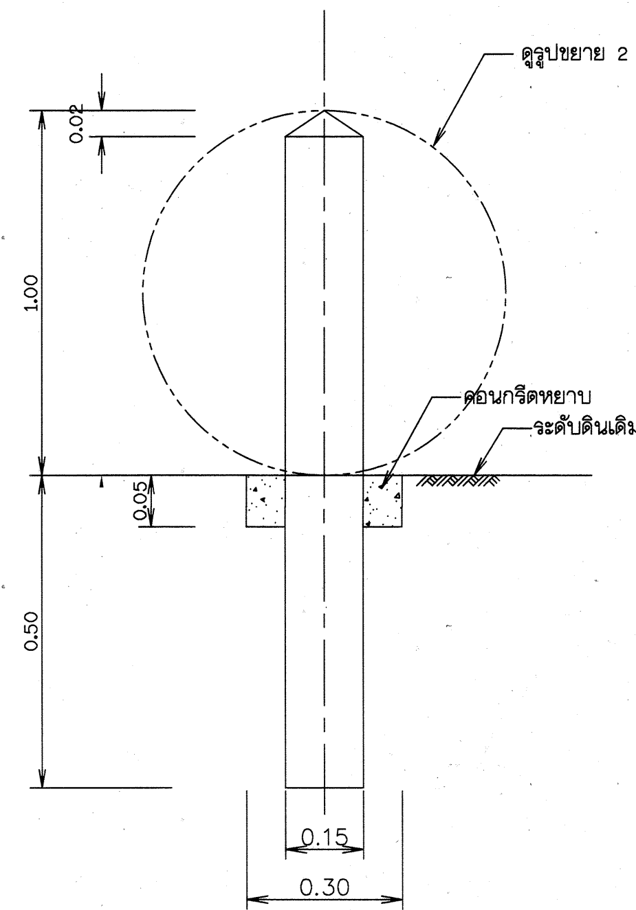
รูปตัด ก-ก แบบที่ 1 แล่ดง กม.ท่อน้ำ ไม่แล่ดงมาดราล่วน
