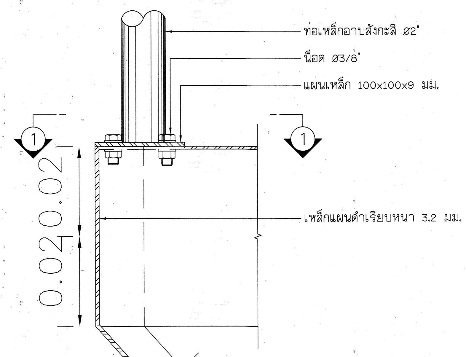
แบบขยาย "ข"
