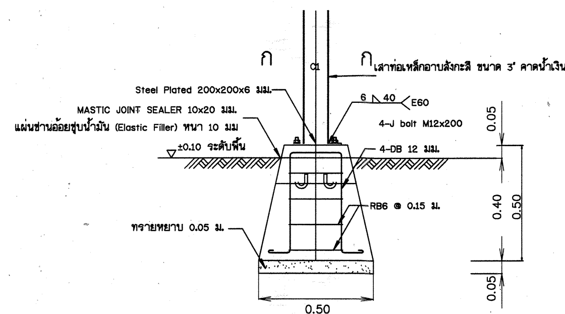
รูปขยายต่อม่อชุดกล้องวงจรปิด (ต่อม่อ คสล. หรือตัวจับรูปทรงเดิมเดิม) ไม่แสดงขนาดฐาน
