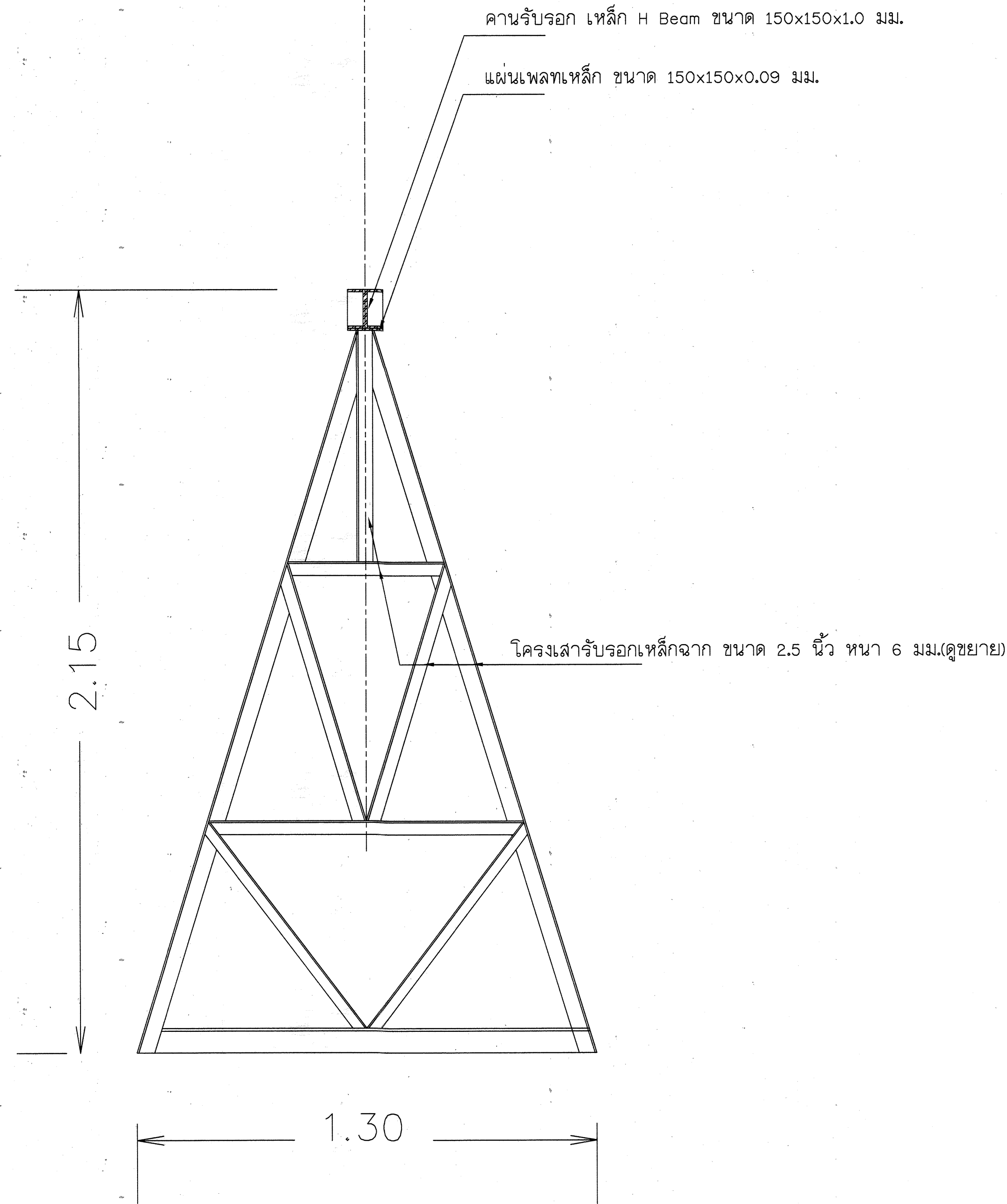
รูปตัดขยายชุดคานารอก มาตราส่วน 1 : 100
