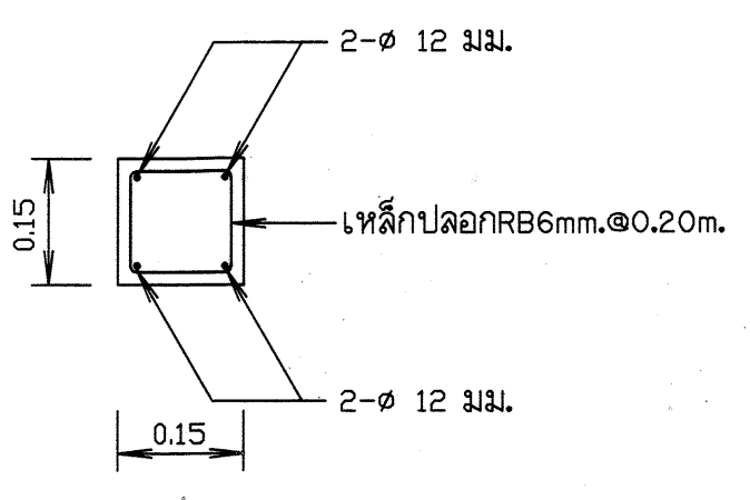
รูปตัด ก - ก มาตรฐาน 1:10
