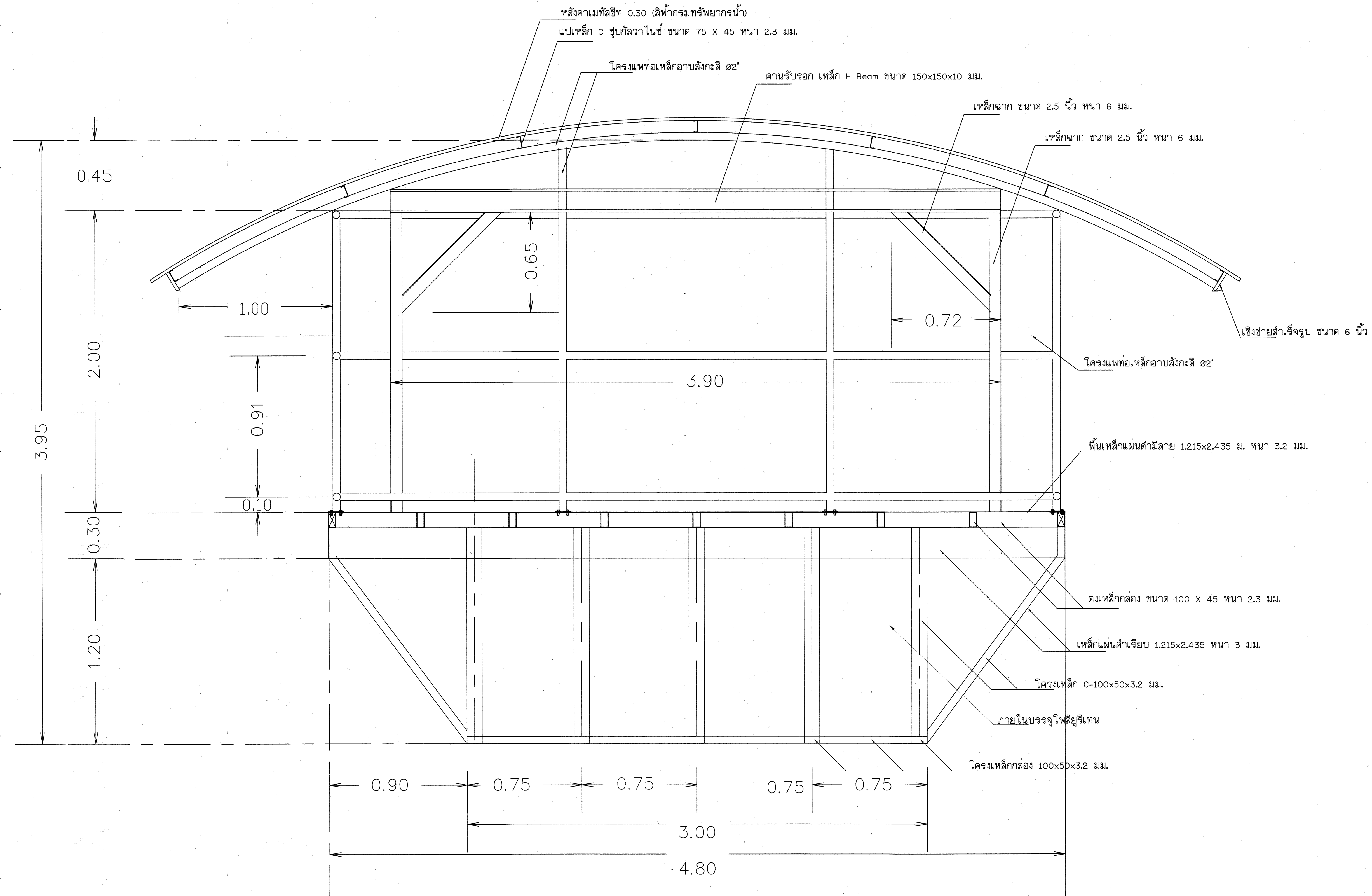
รูปตัดขยาย A - A มาตรฐาน 1:100
