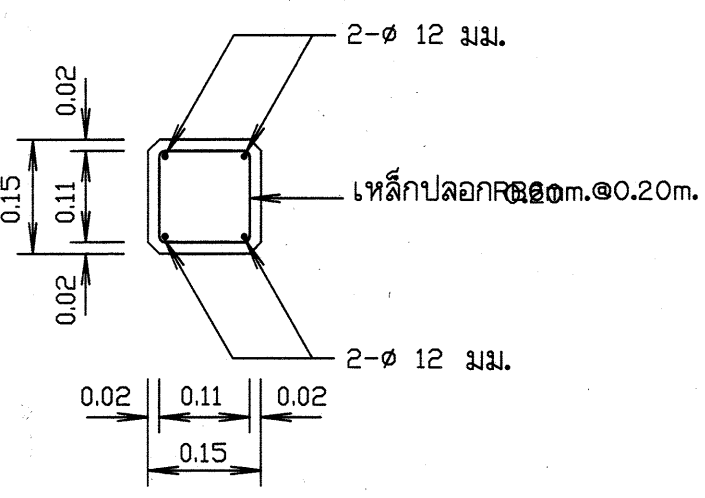
รูปตัด ข - ข มาตรฐาน 1:10
