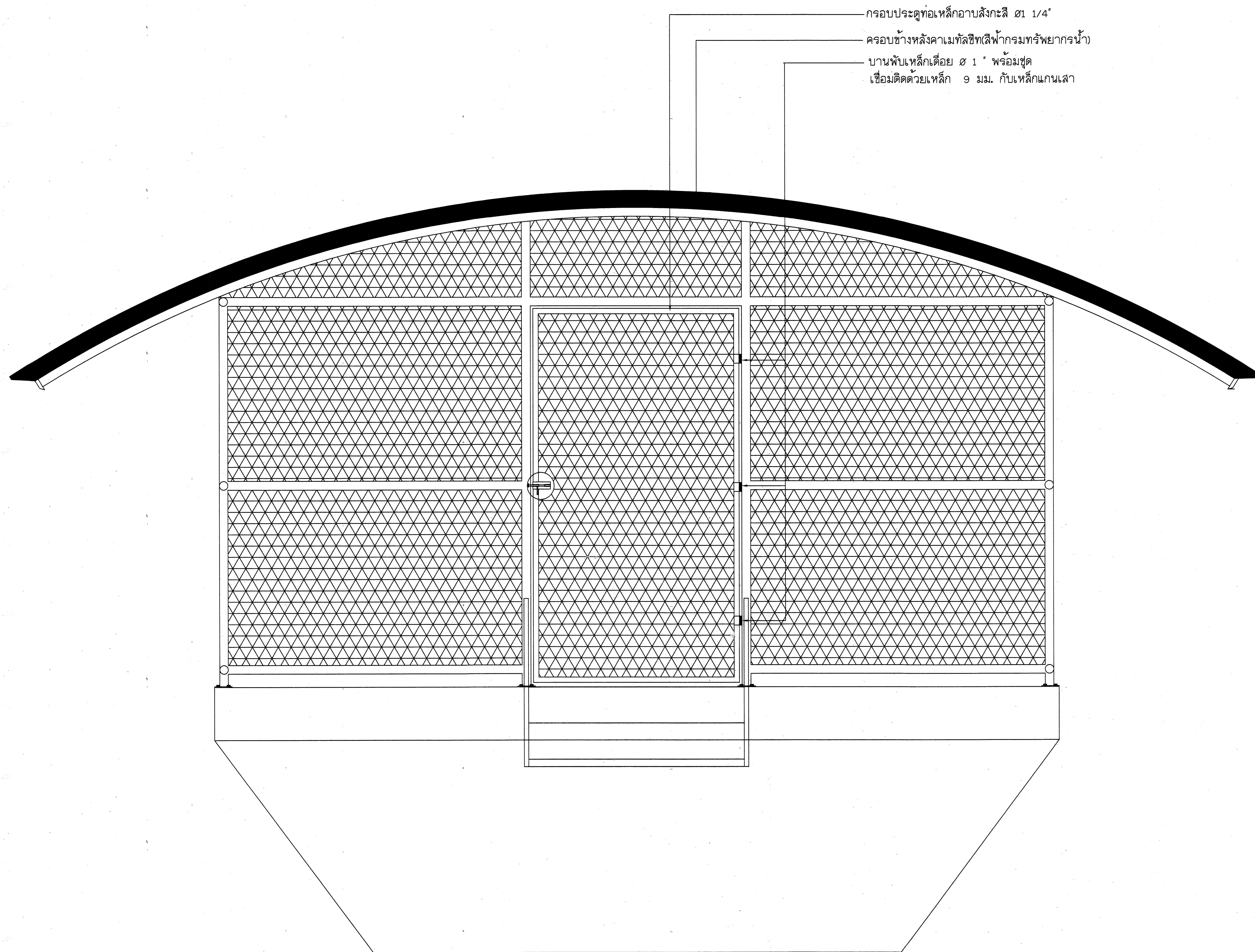
อุปกรณ์หน้า มาตราส่วน 1:100
