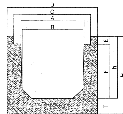
รูปตัด ราง U
