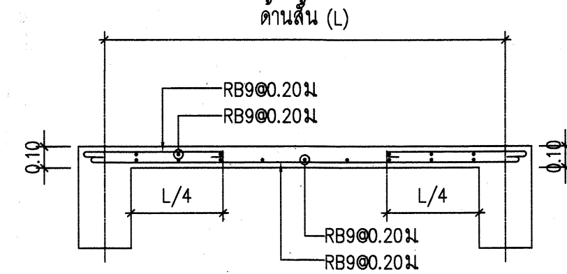
แบบขยายพื้น (SA) มาตราส่วน 1:100
