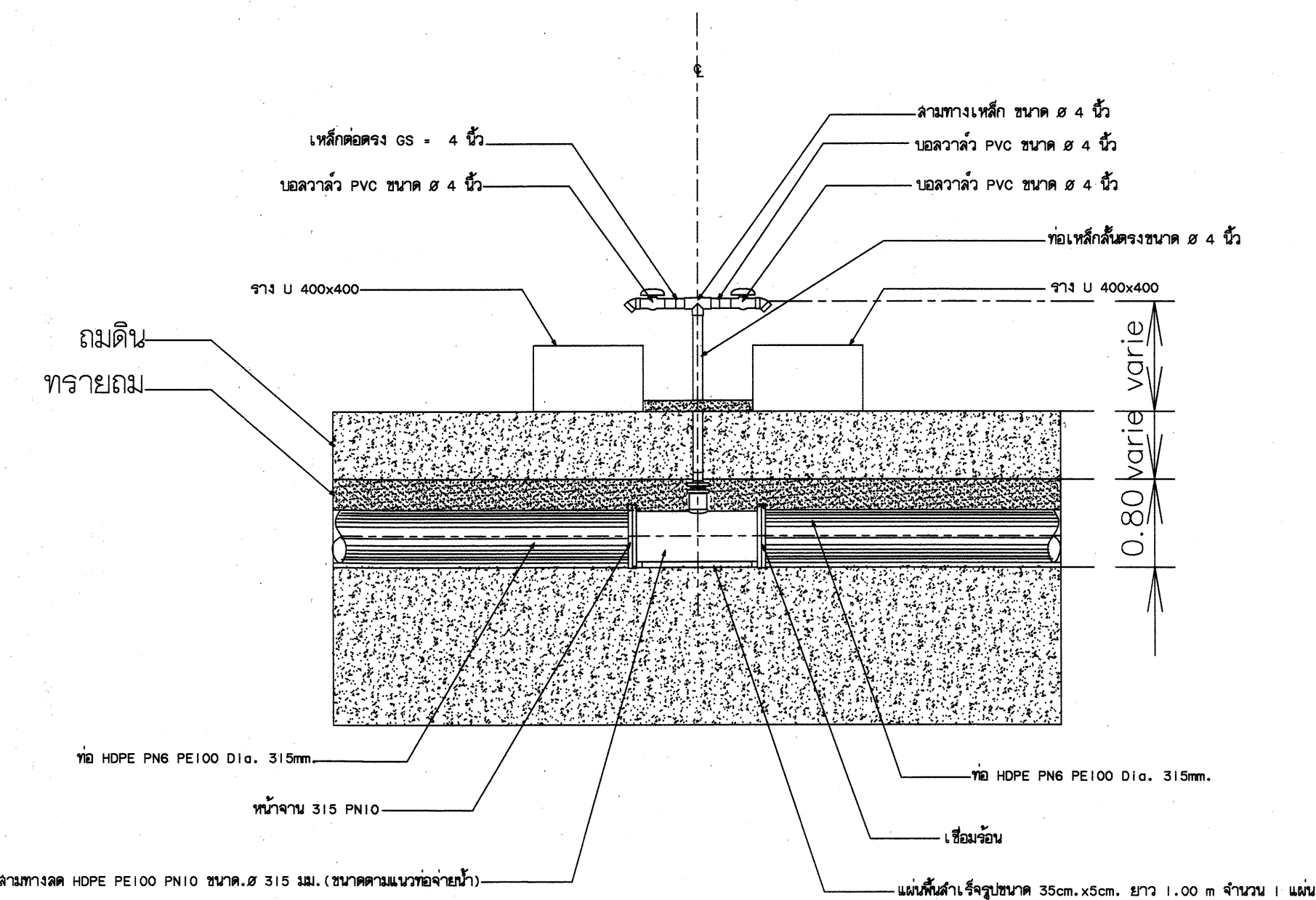
รูปตัด แสดงการติดตั้งจุดกระจายน้ำสำหรับท่อHDPE Dia.315mm. มาตราส่วน 1:100
