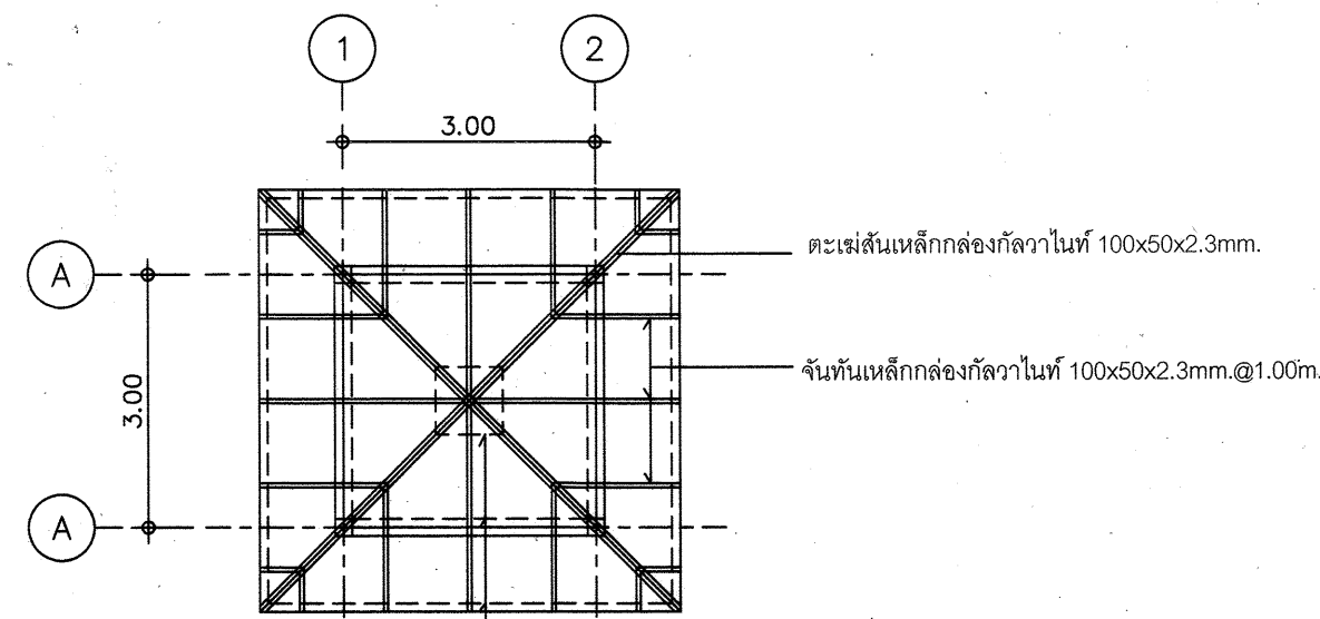
แปลนโครงสร้างชั้นหลังคา-2 มาตราส่วน 1:100
