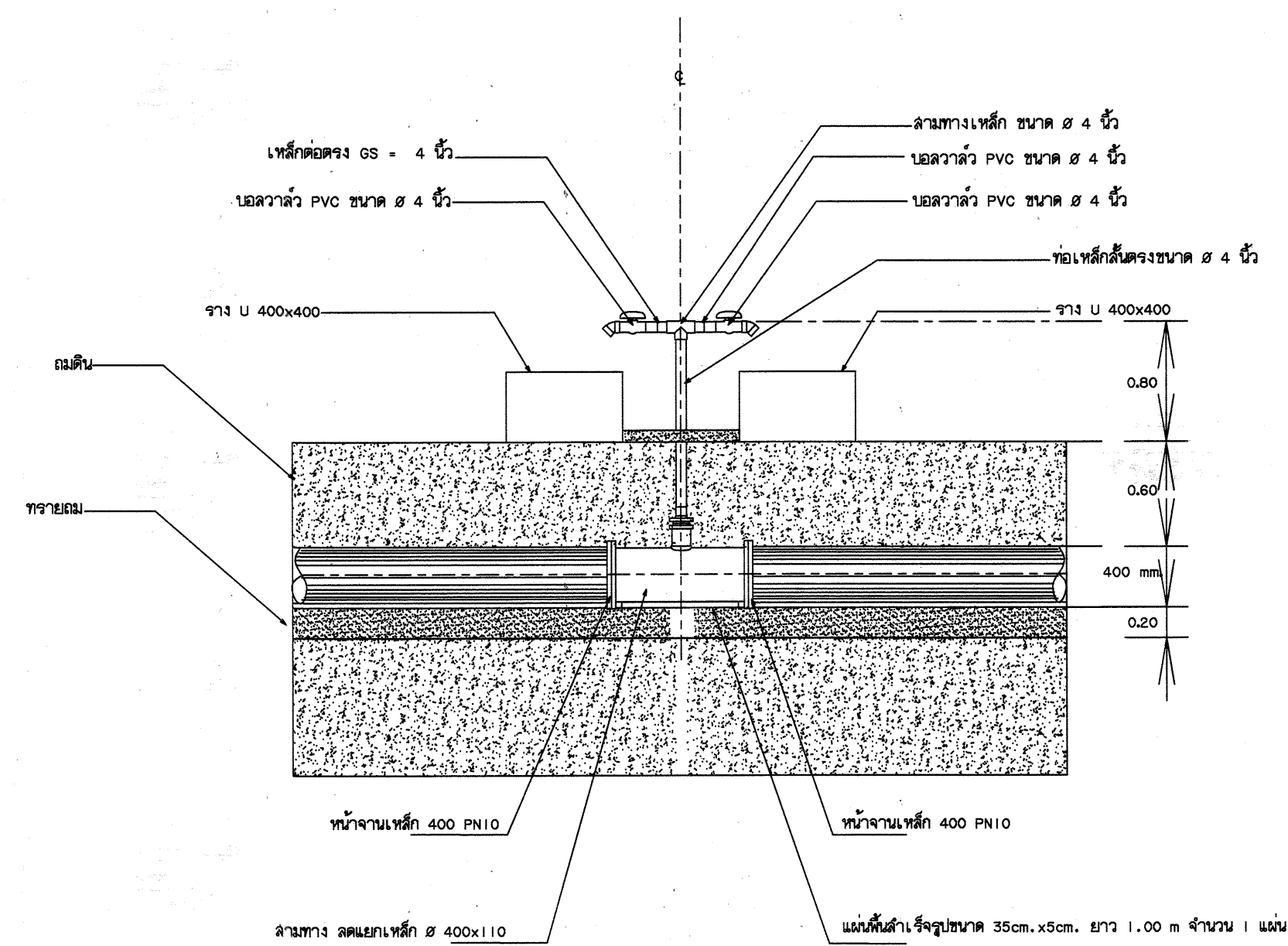
รูปตัด แสดงการติดตั้งจุดกระจายน้ำสำหรับท่อเหล็กขนาด Dia.400mm. มาตราส่วน 1:50
