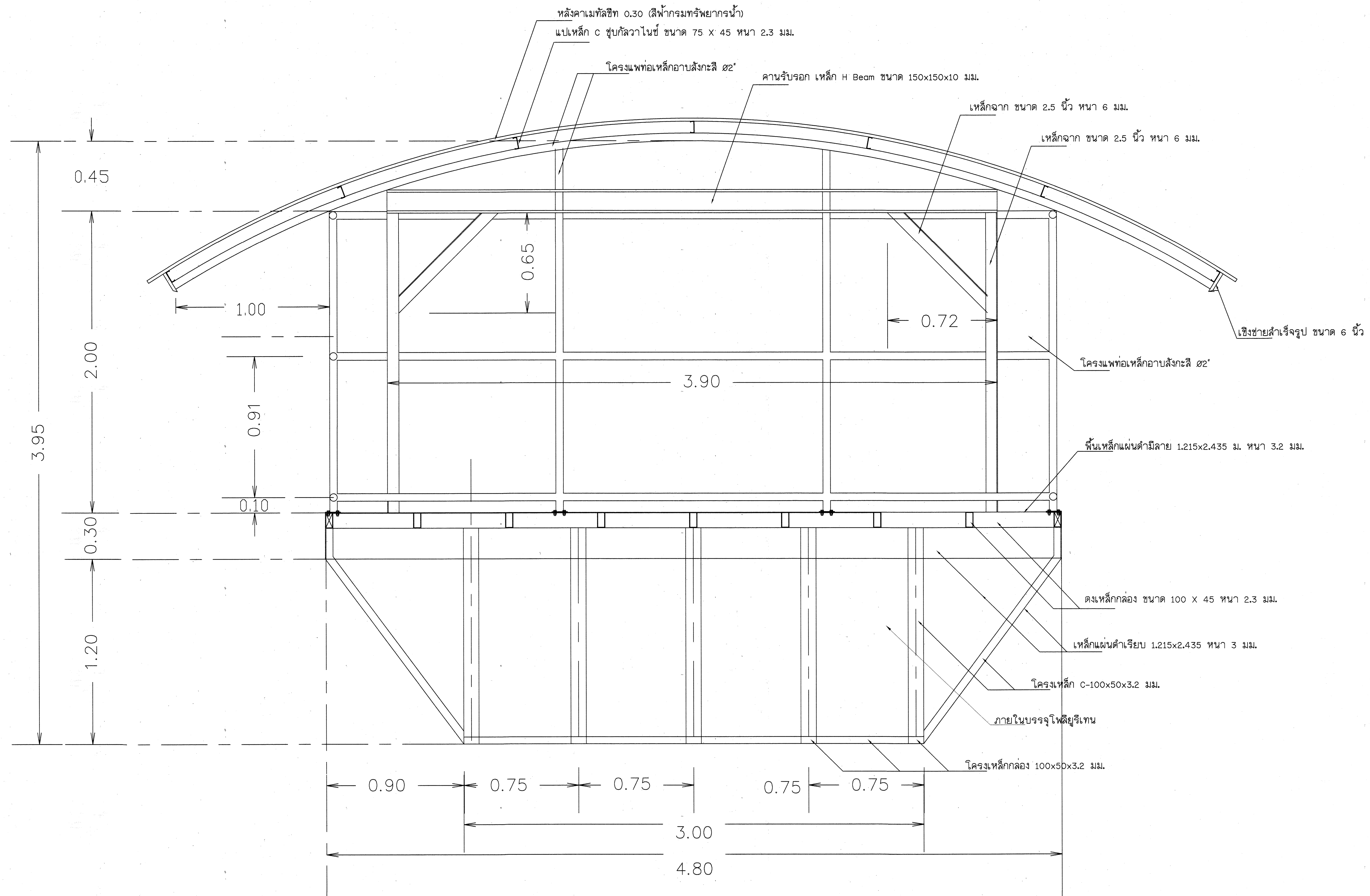
รูปตัดขยาย A - A มาตรฐาน 1:100
