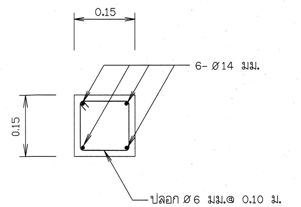
รูปตัด ก - ก
