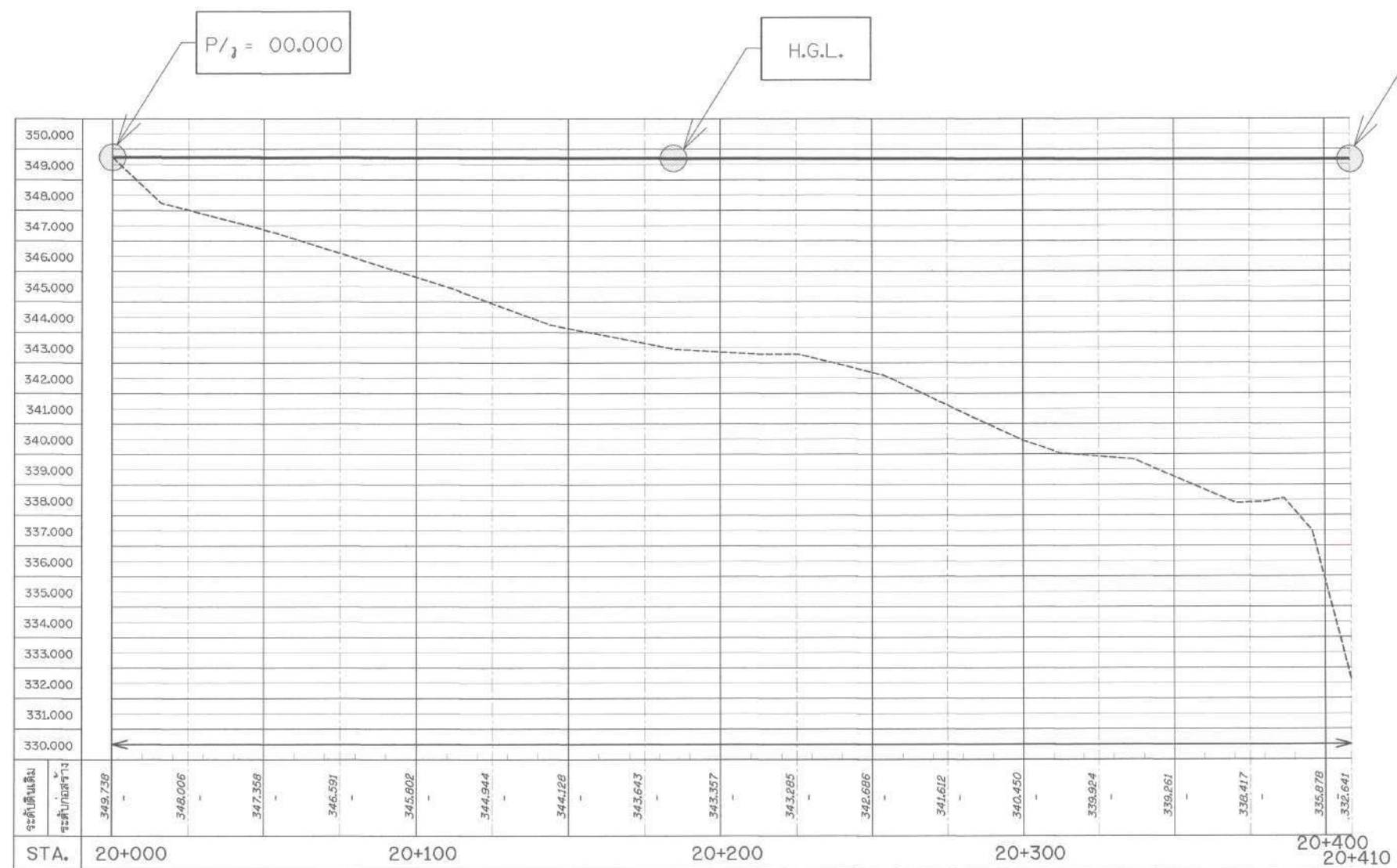
รูปตัดตามแนวยาวแสดง H.G.L. สาย RMP STA. 20+000 - 20+410
