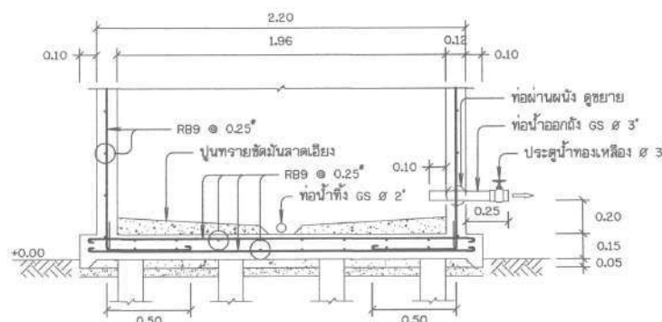
แสดงการเสริมเหล็กพื้นถัง
