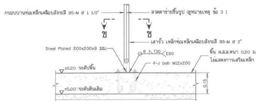
รูปขยายฐานรากโครงสร้างรับแผง F1
