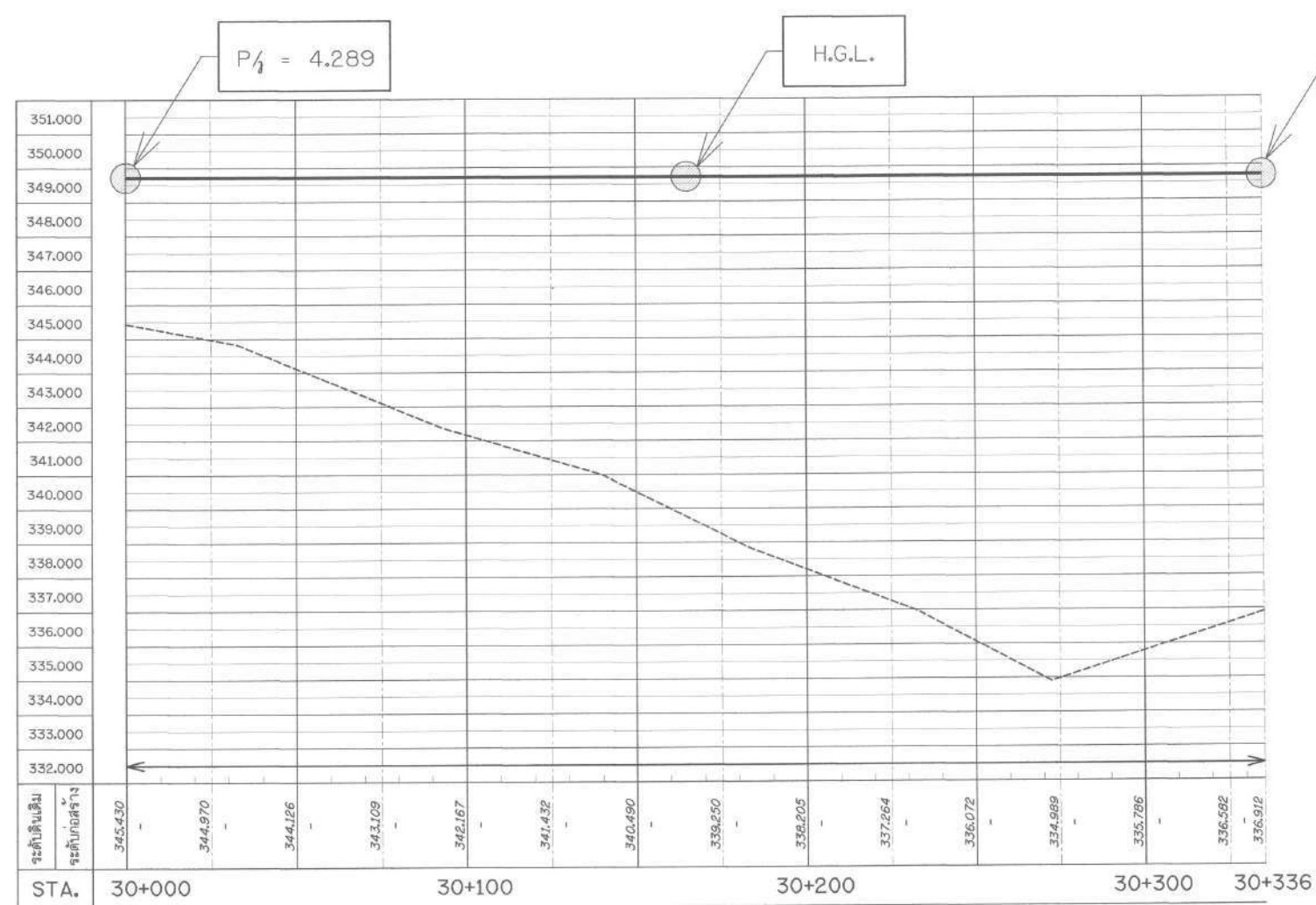
รูปตัดตามแนวยาวแสดง H.G.L. สาย 1L-RMP STA. 30+000 - 30+336
