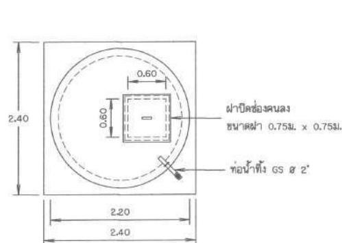
แปลน
