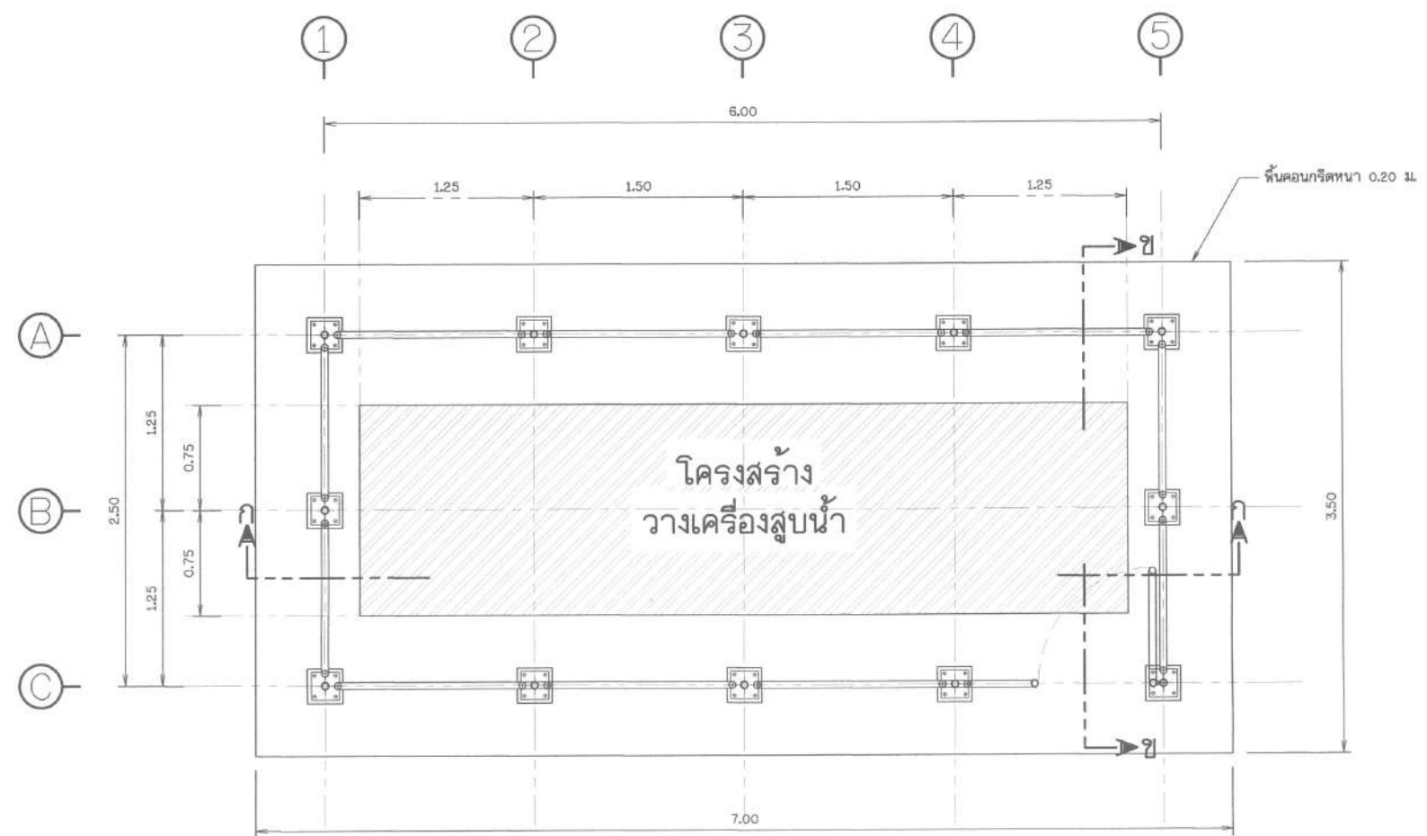
แปลนเสาและรื้อ ไม่แสดงมาตราส่วน
