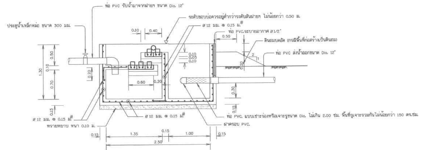
รูปตัด ช - ช
