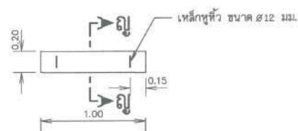
แปลนฝาบ่อดักตะกอน
