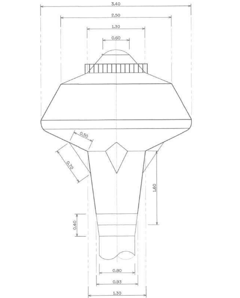
แบบขยายแมนโฮลบนของถังสูง ไม่แสดงมาตราส่วน
