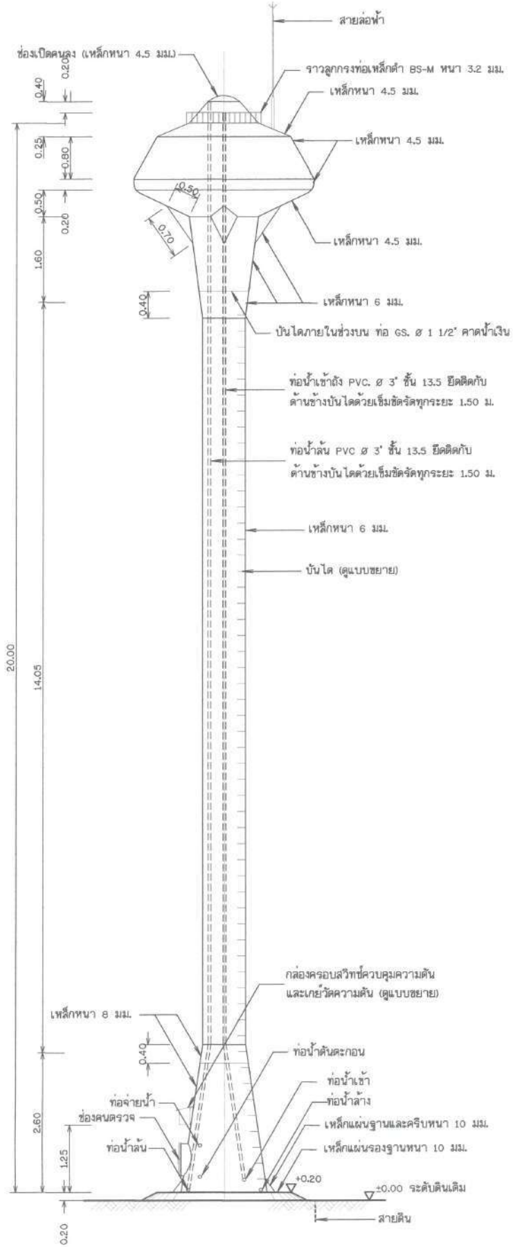
รูปด้านข้างของถังสูง แบบถังเหล็กทรงกลมแป้น ไม่แสดงมาตราส่วน
