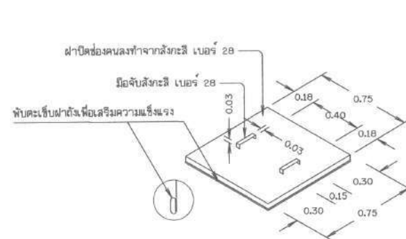
ขยายฝาปิดช่องคนลง
