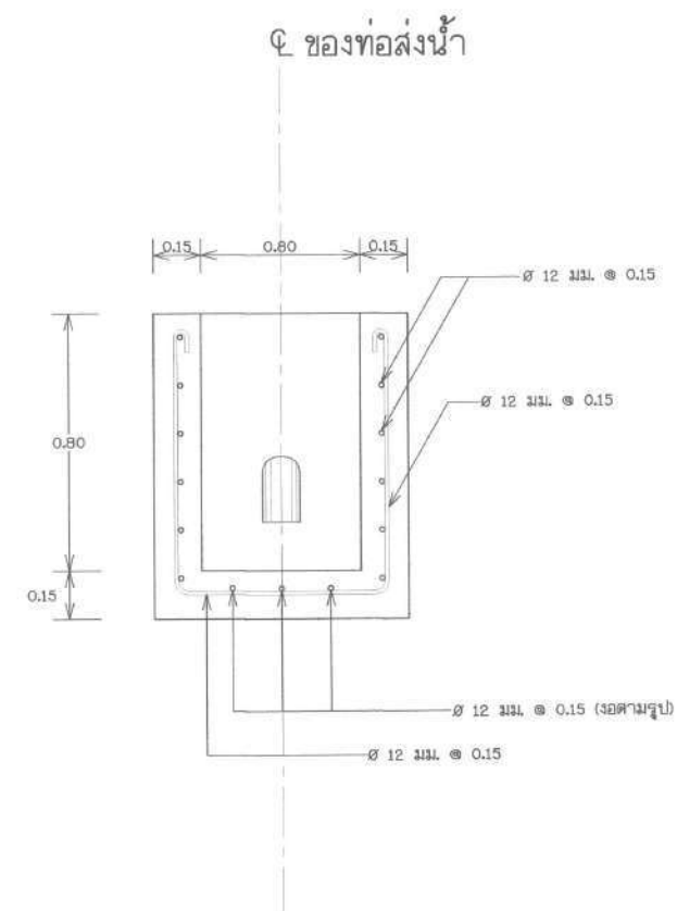
รูปตัดแนว ข - ข
