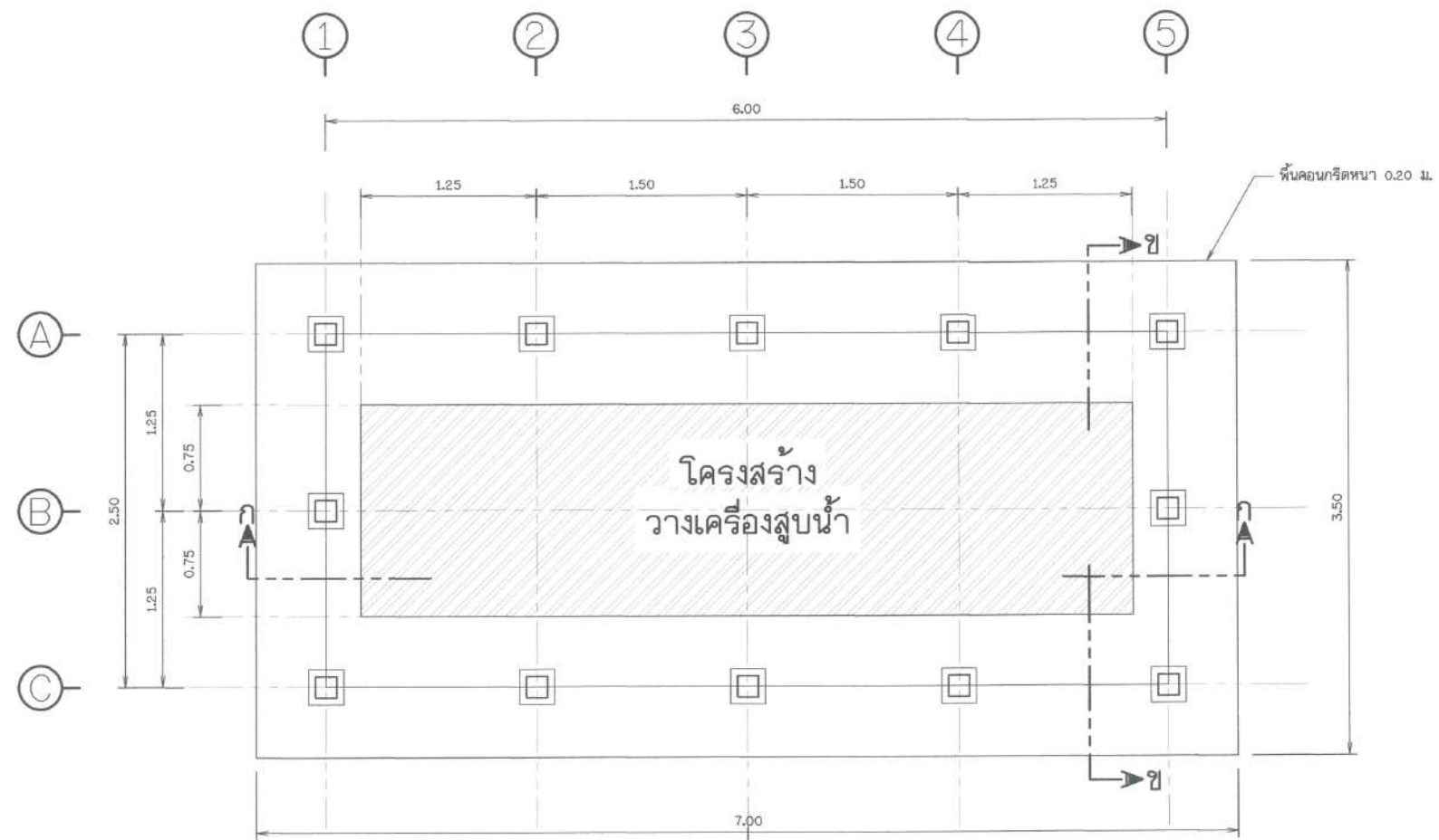
แบบแปลน ไม่แสดงมาตราส่วน
