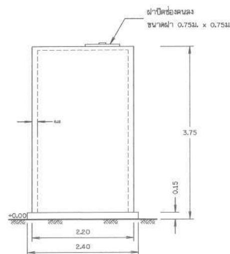
ด้านข้าง
