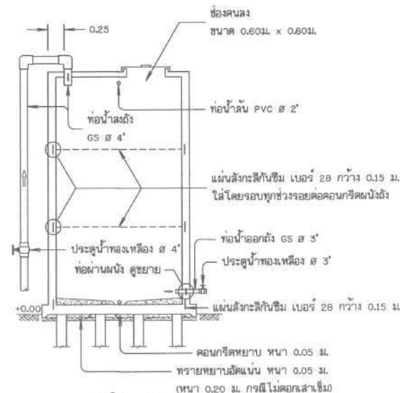
รูปตัด (1)
