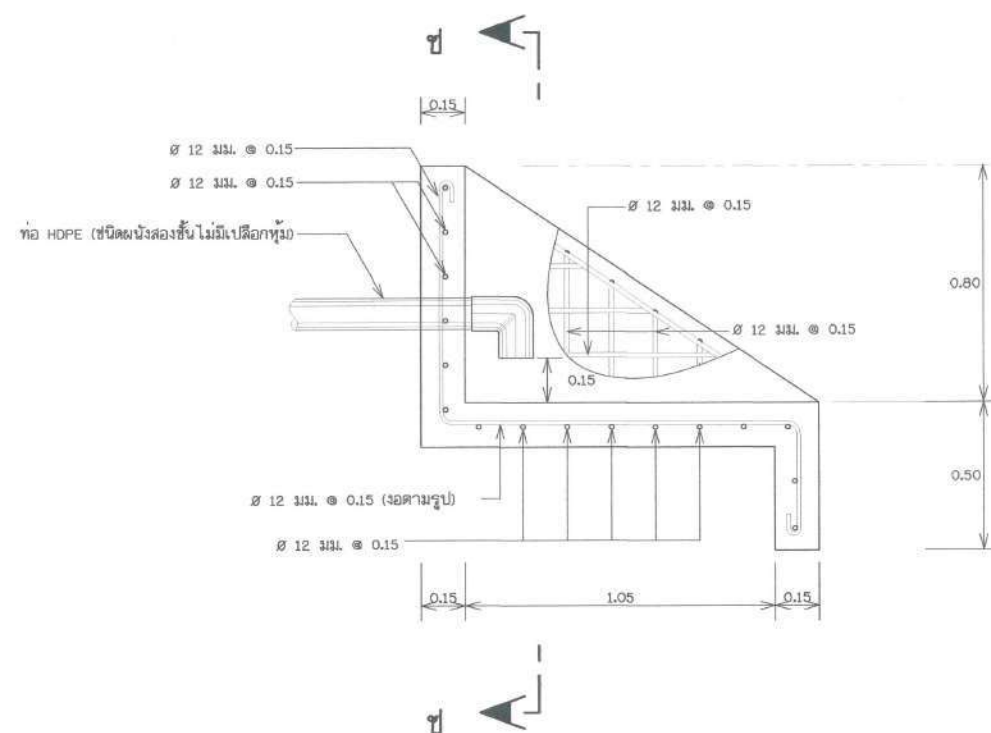
ขยายอาคารสลายพลังงาน
