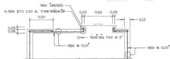
แสดงการเสริมเหล็กฝาลัง
