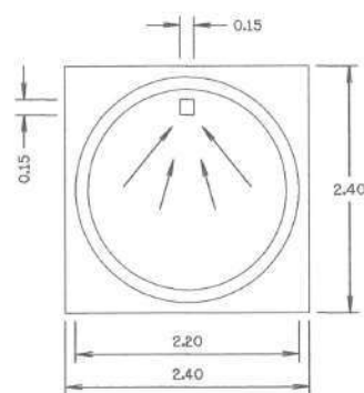
แสดงมิติโดยรวมตะกอน
