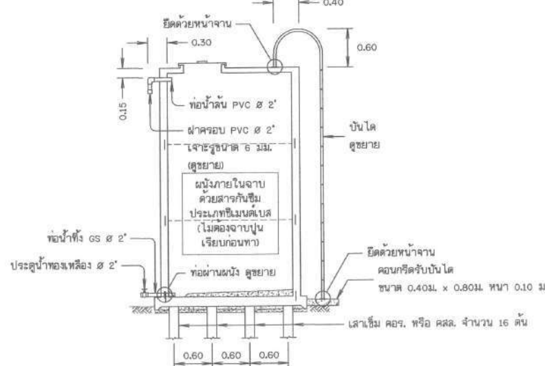
รูปตัด (2)
