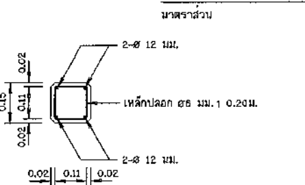
รายละเอียดการติดตั้งเสาป้าย
