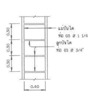
ขยายบันได
