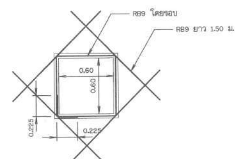
ขยายการเสริมเหล็กช่องคนลง
