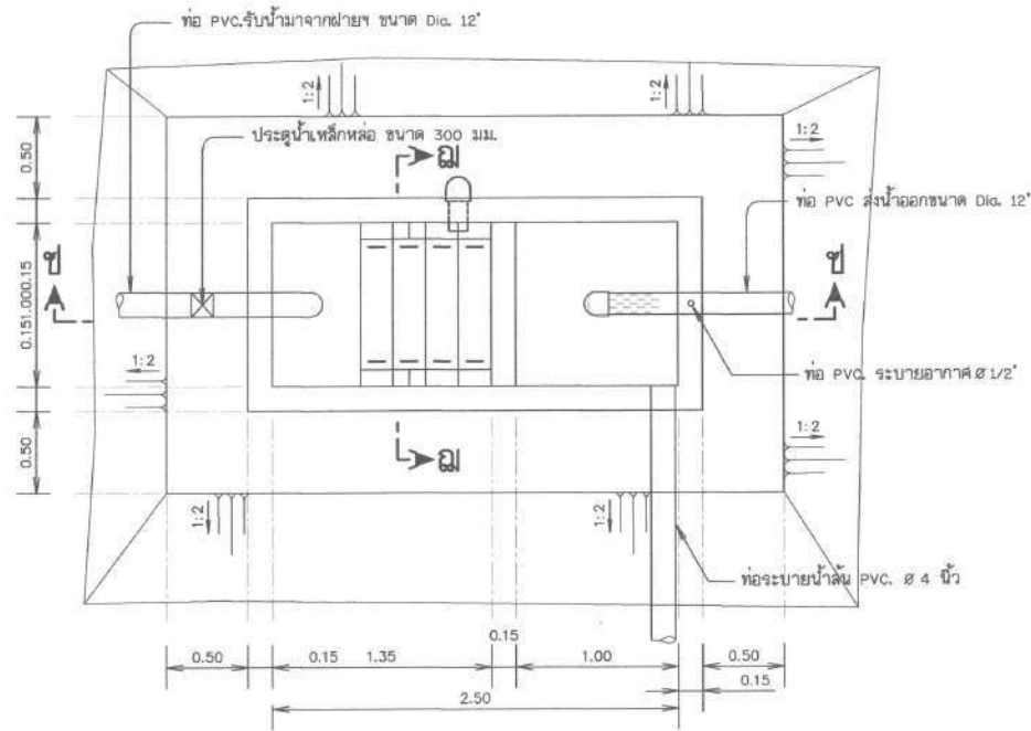
แปลนบ่อดักตะกอน
