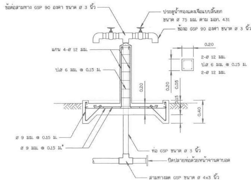
รูปตัด ก - ก
