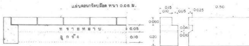
ขยายดินคอนกรีต 1810
