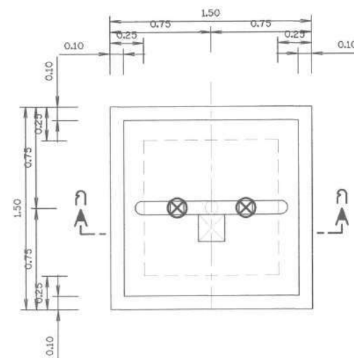
แปลนอาคารจุดปล่อยน้ำ 2 ทาง
