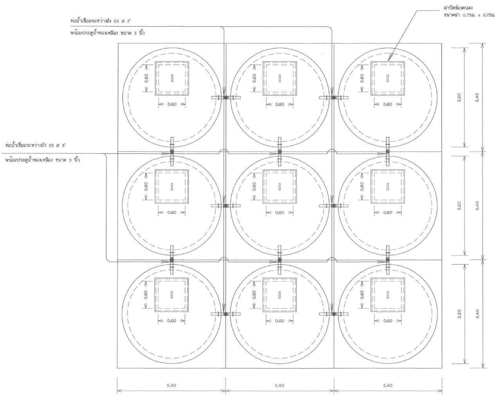
แปลนแบบ 9 ถึง มาตราส่วน 1:100
