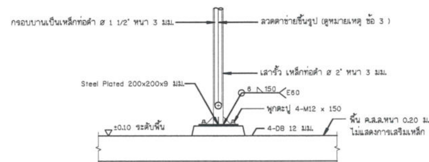
แบบขยายรายละเอียดแสดงการยึด ไม่แสดงขนาดราลวัน
