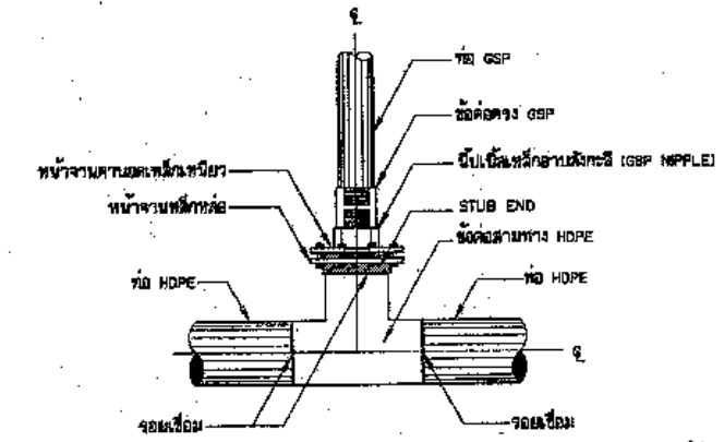
การบรรจุท่อสามทาง HDPE กับท่อ GSP แบบข้อต่อ สำหรับอาคารรูปกล่องน้ำ อาคารประจวบคีรีขันธ์ อาคารท่าเรือระยอง กรณีท่อส่งน้ำขนาดเส้นผ่าศูนย์กลางมากกว่า 315 มม.
