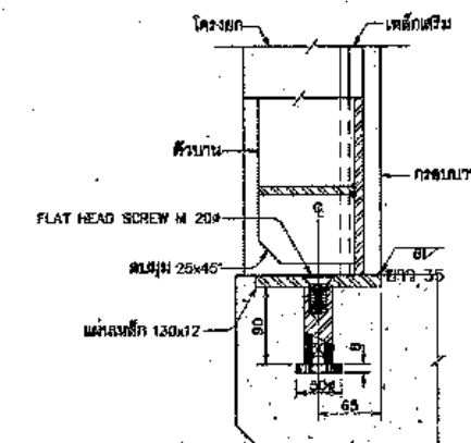
รูปขยาย 2
