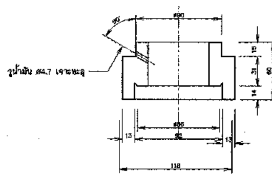
แผ่นปิด
