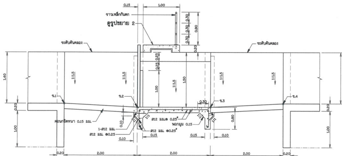
รูปตัด ก-ก
