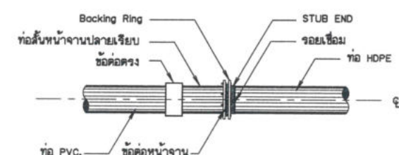
การบรรจุท่อพีวีซี (PVC) กับท่อ HDPE.
