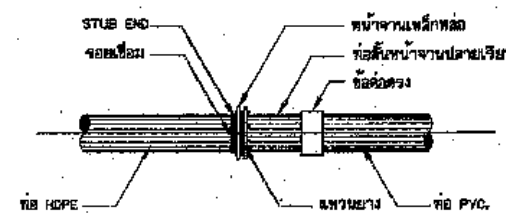
การบรรจุท่อ HDPE กับท่อ PVC. ไม่แสดงขนาดส่วน
