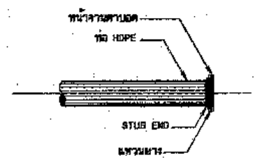
การปิดปลายท่อ ไม่แสดงขนาดส่วน
