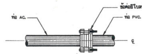
การบรรจบท่อ AC. กับท่อ PVC. ไม่แสดงมาตราส่วน
