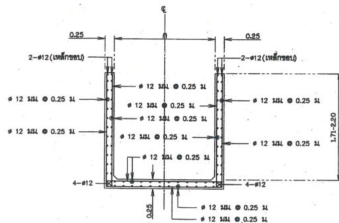
รูปแสดงการเสริมเหล็ก ความสูง 1.51-2.00 ม. ไม่แสดงมาตราส่วน
