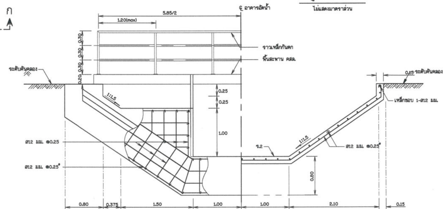
รูปตัด ค-ค
