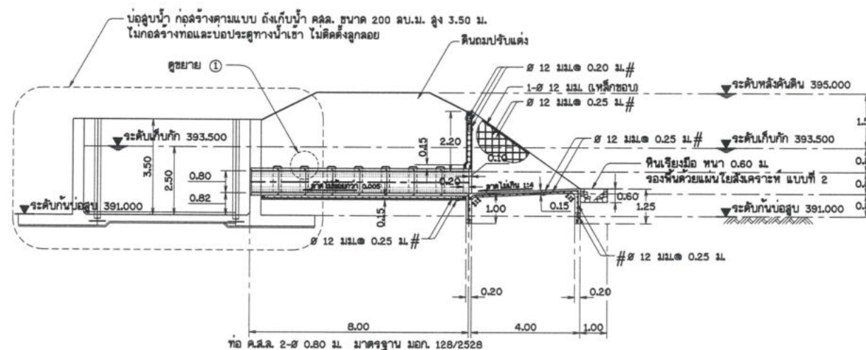
รูปตัดแนว ก - ก
