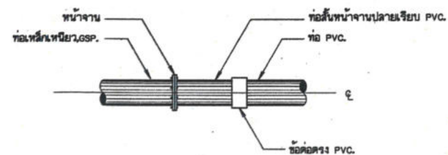
การบรรจบท่อเหล็กเหนียวหรือ GSP. กับท่อ PVC. ไม่แสดงมาตราส่วน
