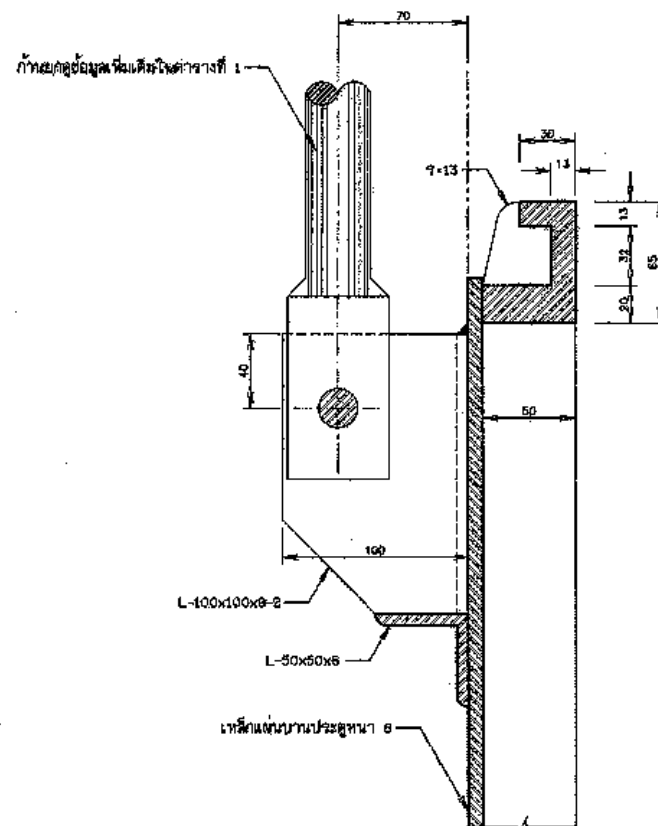
รูปตัด ข - ข มาตราส่วน 1:2
