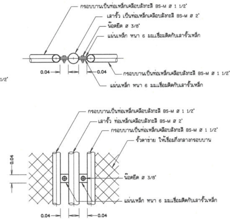
แบบขยายรายละเอียดแสดงการยึดระหว่างรื้อกับเสา ไม่แสดงมาตราส่วน
