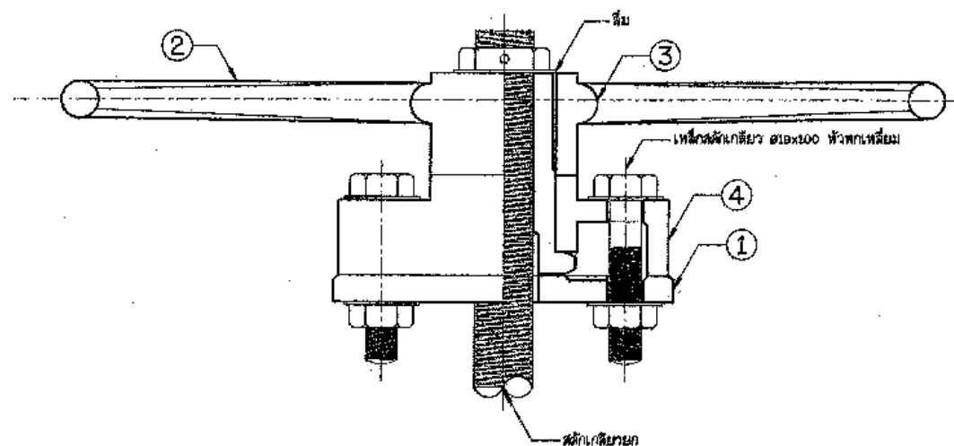
แสดงการติดตั้ง
