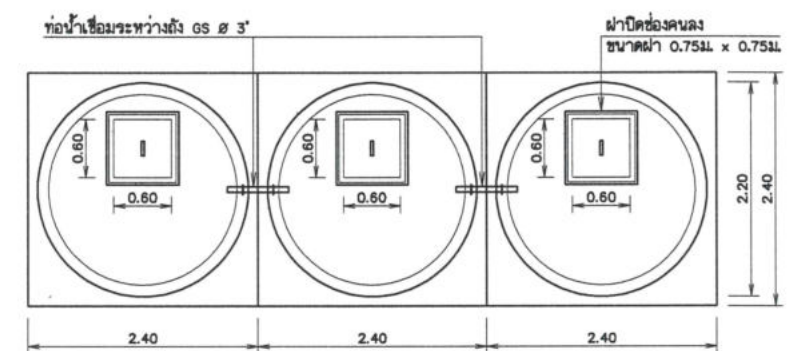
แปลนแบบ 3 ถึง มาตราส่วน 1:40
