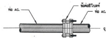
การบรรจบท่อ AC. กับท่อ AC. ไม่แสดงมาตราส่วน
