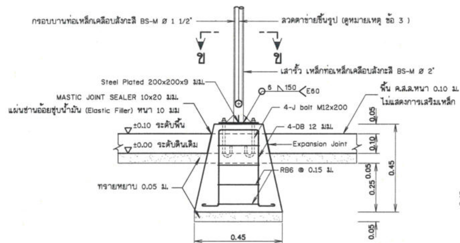
รูปขยายฐานรากโครงสร้างรับแผง F1 (ต่อมา คสล. หล่อสำเร็จรูปพร้อมติดตั้ง)
