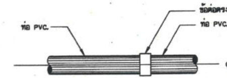
การบรรจบท่อ PVC. กับท่อ PVC. ไม่แสดงมาตราส่วน
