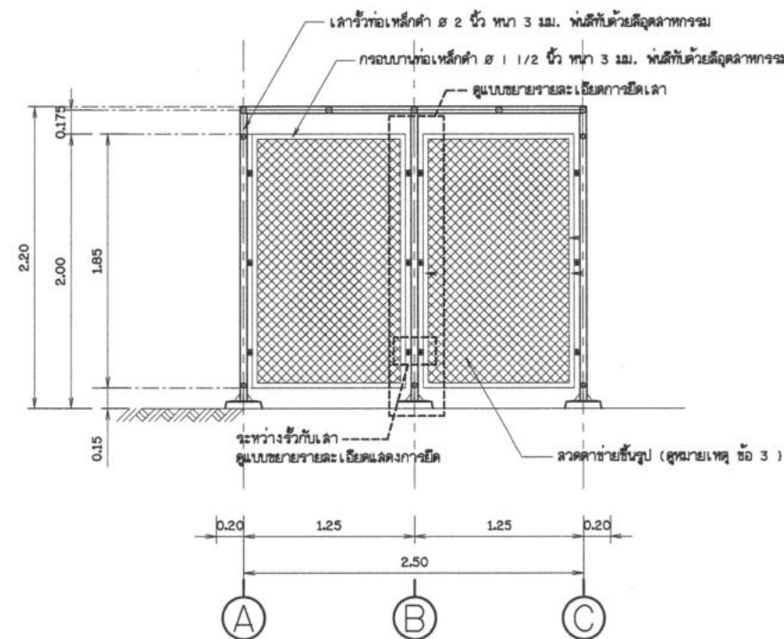
แบบขยายรั้ว 2 ไม่แสดงขนาดราลวัน
