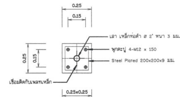
ฐานรากโครงสร้างอาคารคลุม ไม่แสดงขนาดราลวัน
