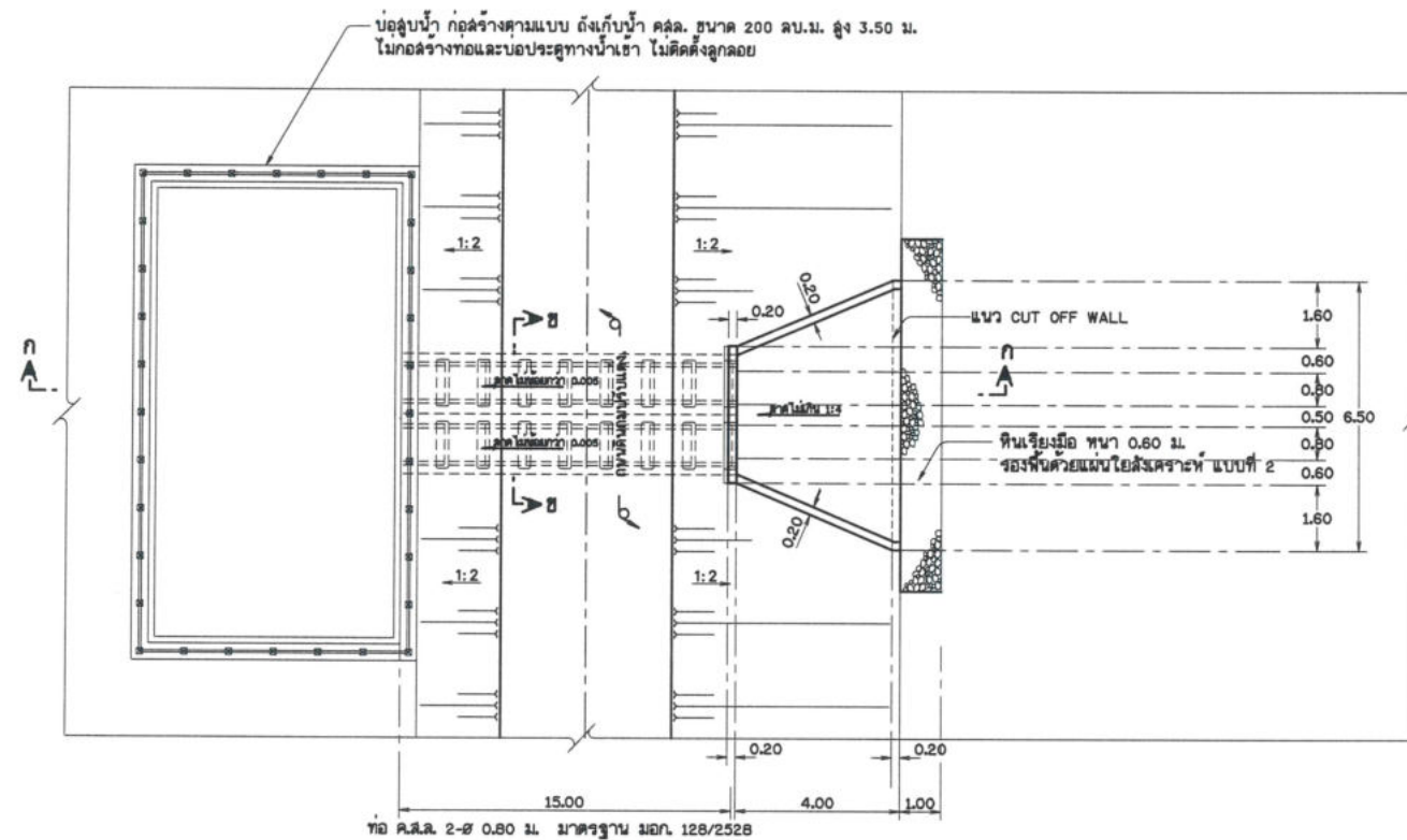
แปลนอาคารท่อทางน้ำเข้าบ่อสูบน้ำ
