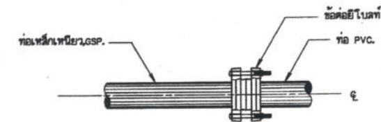
การบรรจบท่อเหล็กเหนียวหรือ GSP. กับท่อ PVC. ไม่แสดงมาตราส่วน
