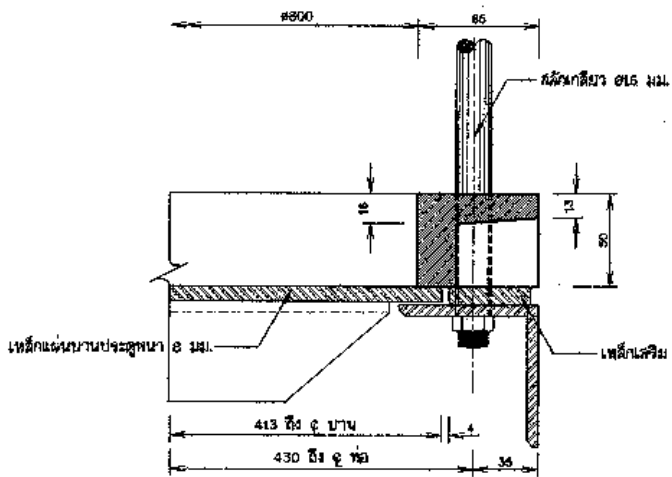
รูปตัด ก - ก มาตราส่วน 1:2
