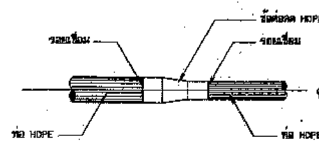
การบรรจุท่อ HDPE กับข้อต่อท่อ HDPE ไม่แสดงขนาดส่วน
