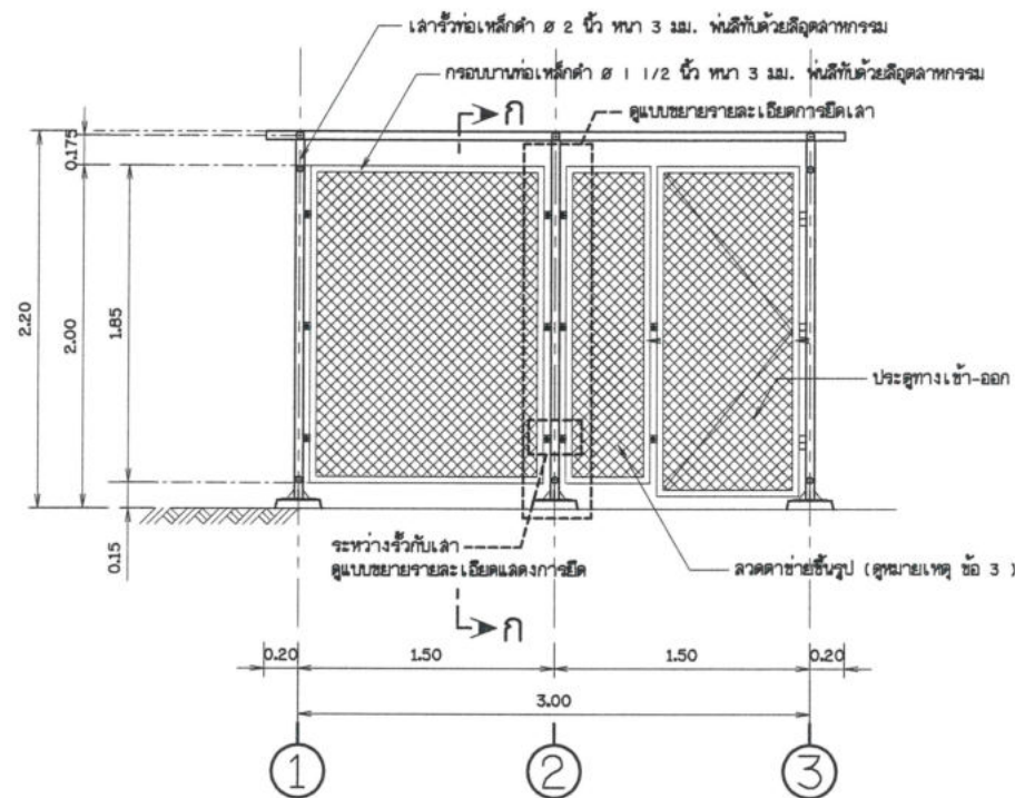
แบบขยายรั้ว 1 ไม่แสดงขนาดราลวัน
