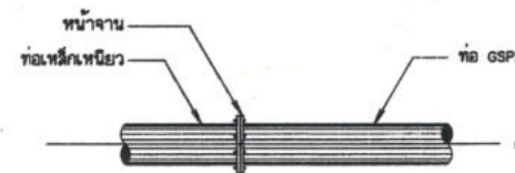
การบรรจบท่อเหล็กเหนียวกับท่อ GSP. ไม่แสดงมาตราส่วน
