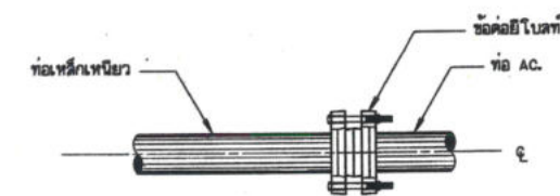
การบรรจบท่อเหล็กเหนียวกับท่อ AC. ไม่แสดงมาตราส่วน
