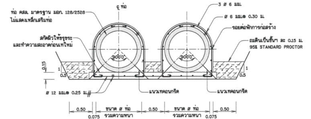
รูปตัดแนว ข - ข
