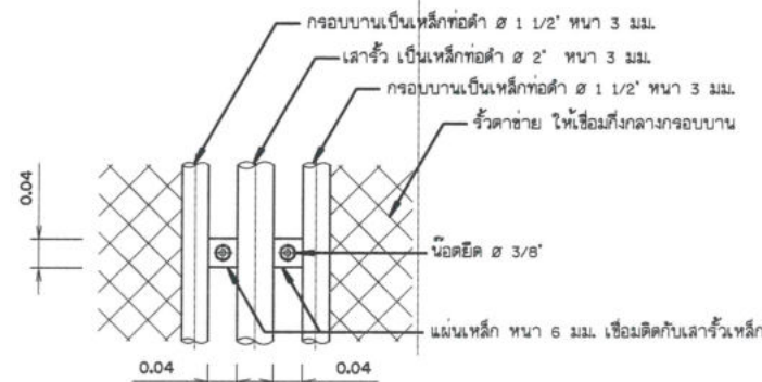
แบบขยายรายละเอียดแสดงการยึดระหว่างรั้วกับเสา ไม่แสดงขนาดราลวัน
