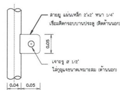
แบบขยายสายยู่ ไม่แสดงขนาดราลวัน
