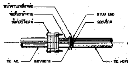
การบรรจุท่อ AC. กับท่อ HDPE ไม่แสดงขนาดส่วน
