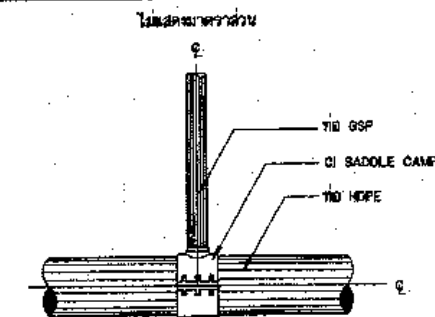
การบรรจุท่อสามทาง HDPE กับท่อ GSP แบบ CI SADDLE CLAMP สำหรับอาคารรูปกล่องน้ำ อาคารประจวบคีรีขันธ์ อาคารท่าเรือระยอง กรณีท่อส่งน้ำขนาดเส้นผ่าศูนย์กลางน้อยกว่าหรือเท่ากับ 315 มม.
