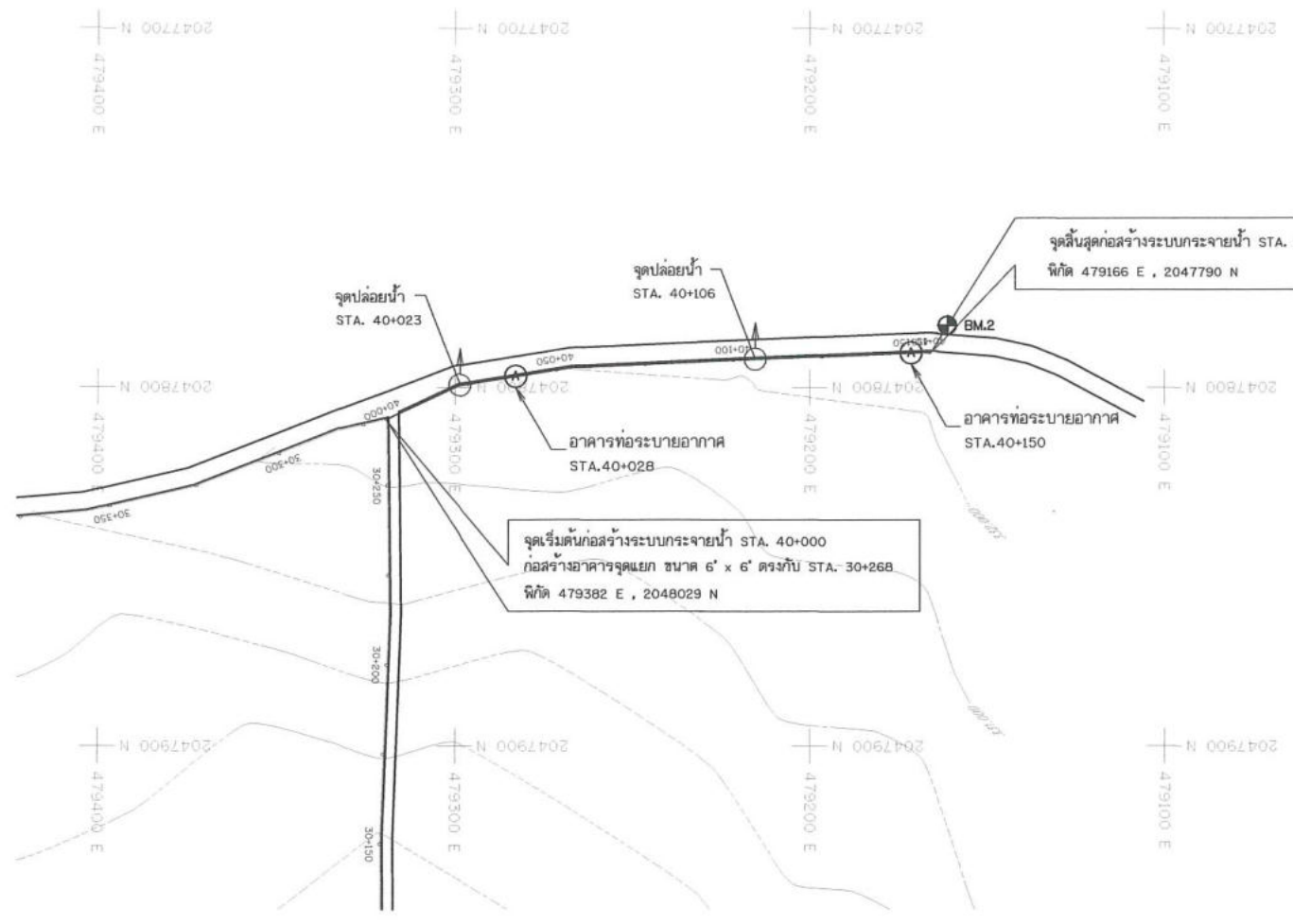
แปลนระบบส่งน้ำ
