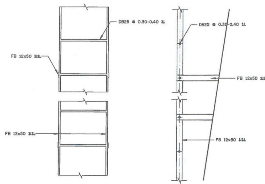
แบบขยายบันได ภายในท่อถึงสูง ไม่แสดงมาตราส่วน
