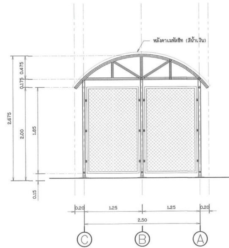
รูปด้าน 2 โมเดลตามตราส่วน
