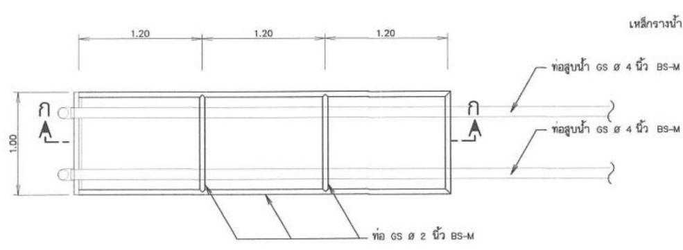
แปลนโครงสร้างรับท่อสูบน้ำ มาตราส่วน 1:25
