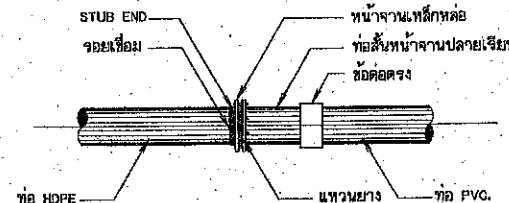
การบรรจุบ่อท่อ HDPE กับท่อ PVC.
