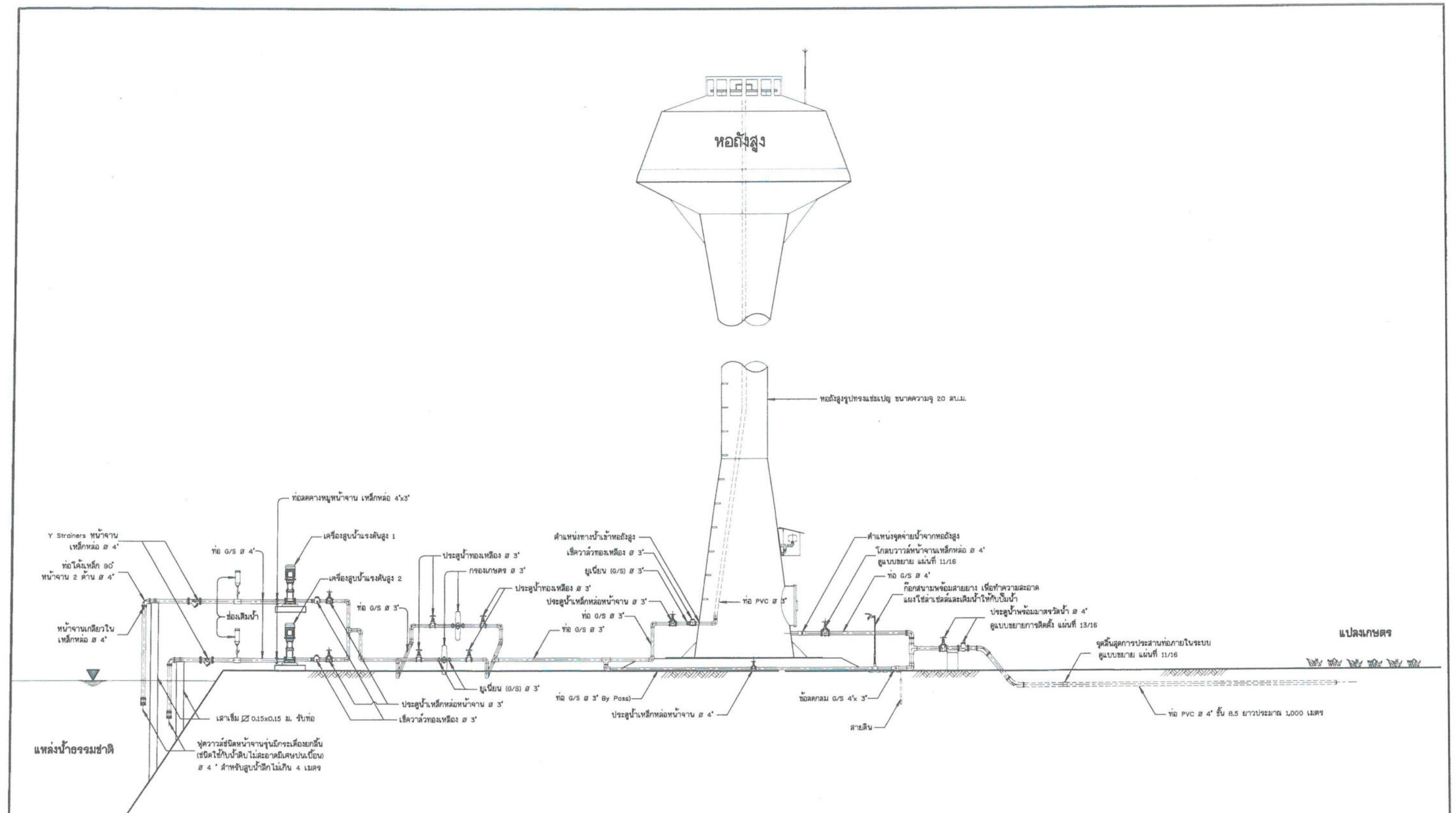
รูปแสดงรายละเอียดท่อและอุปกรณ์ระบบสูบน้ำพลังงานแสงอาทิตย์ ไม่แสดงขนาดตัว
