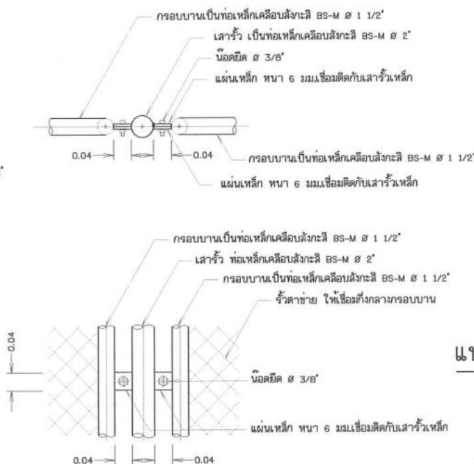
แบบขยายรายละเอียดแสดงการยึดระหว่างรื้อกับเสา ไม่แสดงมาตราส่วน
