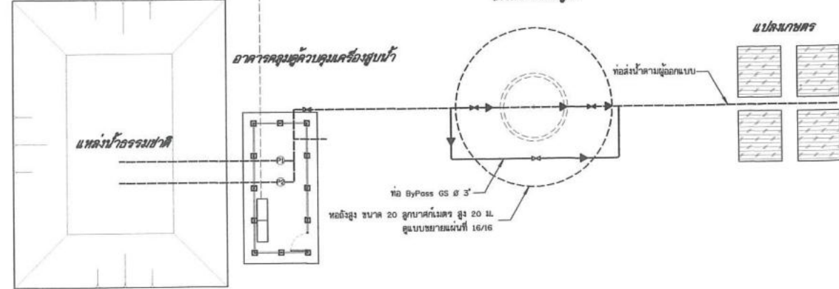
แผนผังระบบกระจายน้ำด้วยพลังงานแสงอาทิตย์ ขนาด 4 กิโลวัตต์
