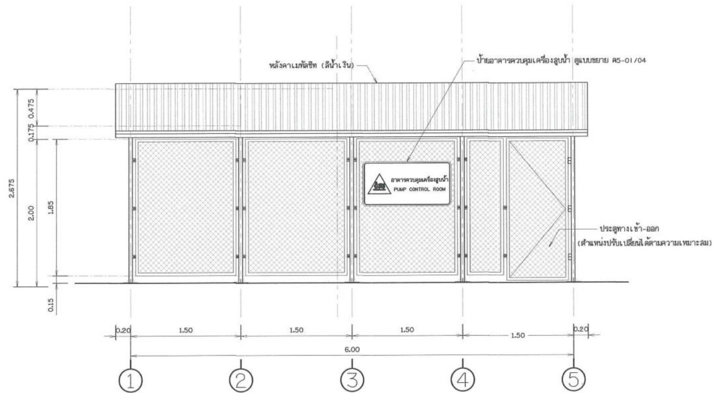
รูปด้าน 1 โมเดลตามตราส่วน
