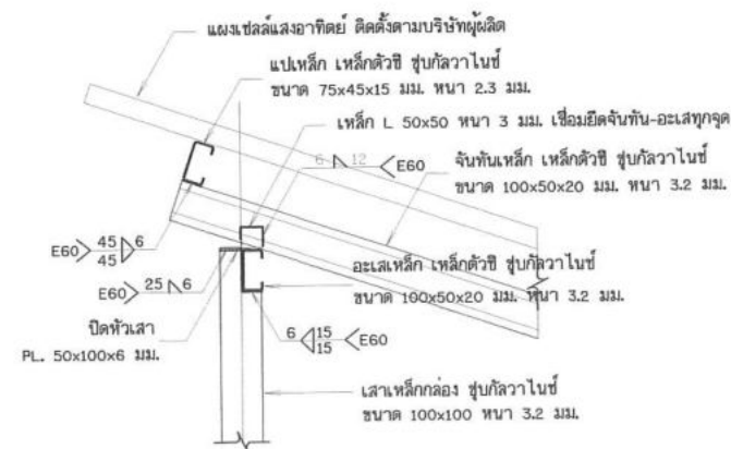
รูปขยาย การติดตั้งโครงหลังคา ไม่แสดงขนาดราส่วน
