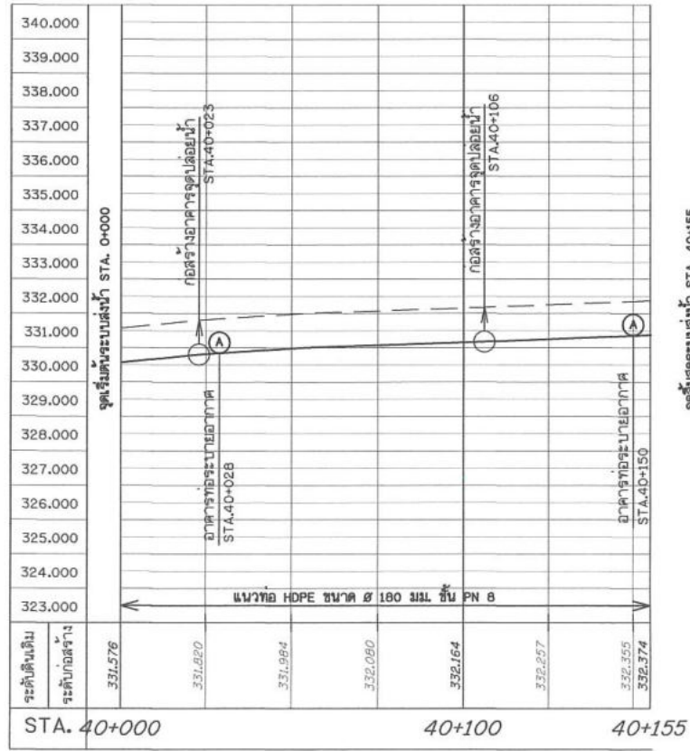
รูปตัดตามแนวยาว
