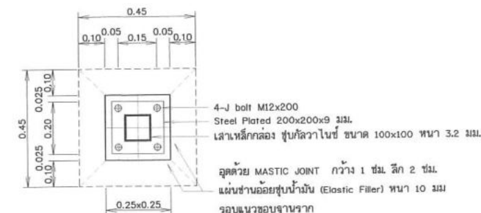
รูปตัด ก-ก ไม่แสดงขนาดราส่วน
