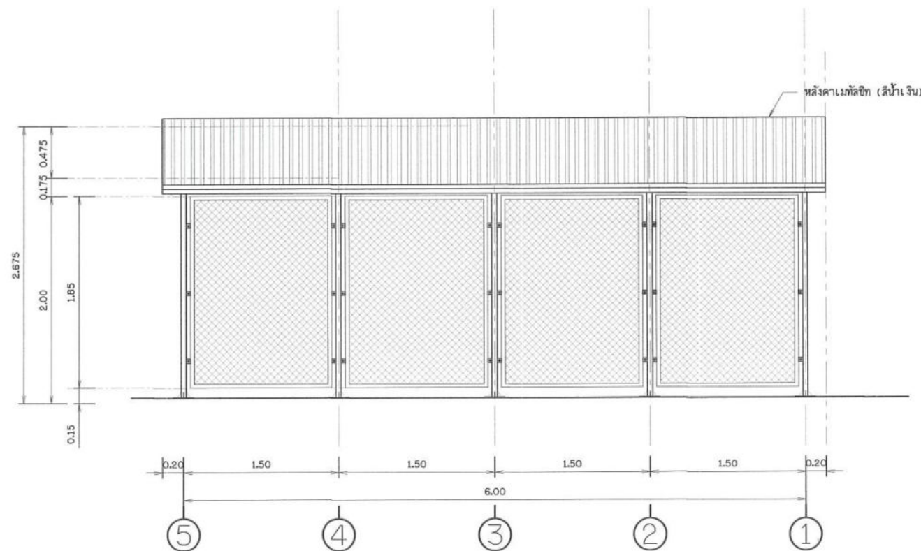
รูปด้าน 1 โมเดลตามตราส่วน
