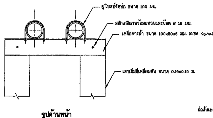
13. เสาคอมม่อนรับท่อชุด และแบบขยายอุปกรณ์รัดท่อ ไม่แสดงขนาดราส่วน
