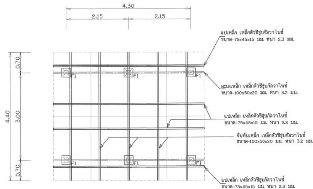
แปลนฐานรากและโครงหลังคา ไม่แสดงขนาดราส่วน
