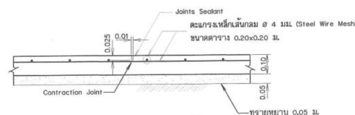
แบบขยายรอยต่อพื้น (Contraction Joint) ไม่แสดงขนาดราส่วน
