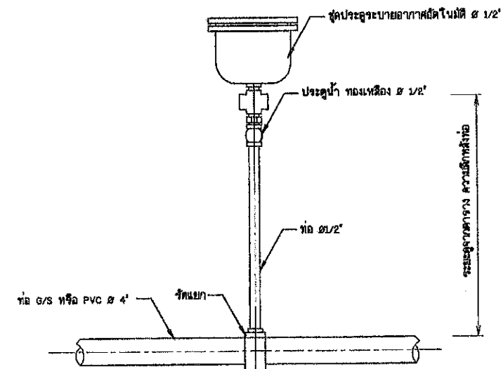
12. การติดตั้งประตูละบายอากาศอัด โนมมิติ ไม่แสดงขนาดราส่วน
