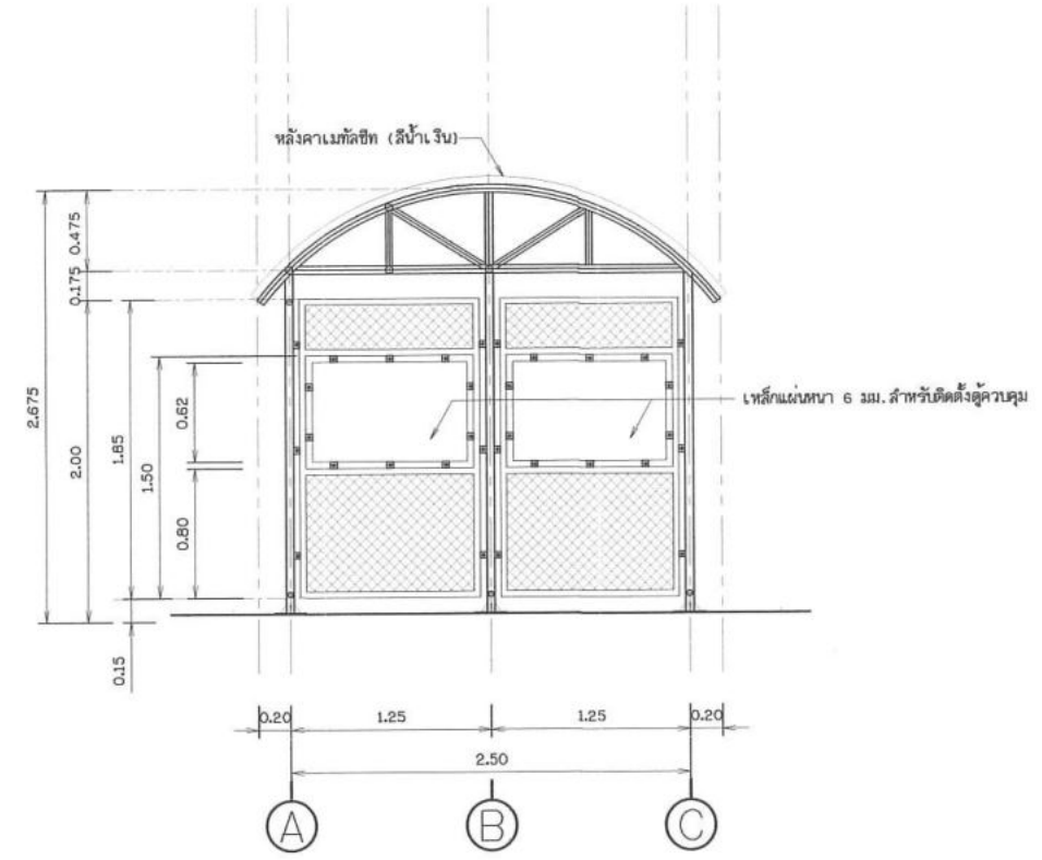
รูปด้าน 2 โมเดลตามตราส่วน
