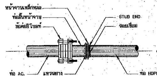
การบรรจุบ่อท่อ AC กับท่อ HDPE
