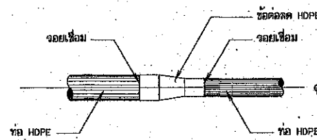
การบรรจุบ่อท่อ HDPE กับข้อลดท่อ HDPE
