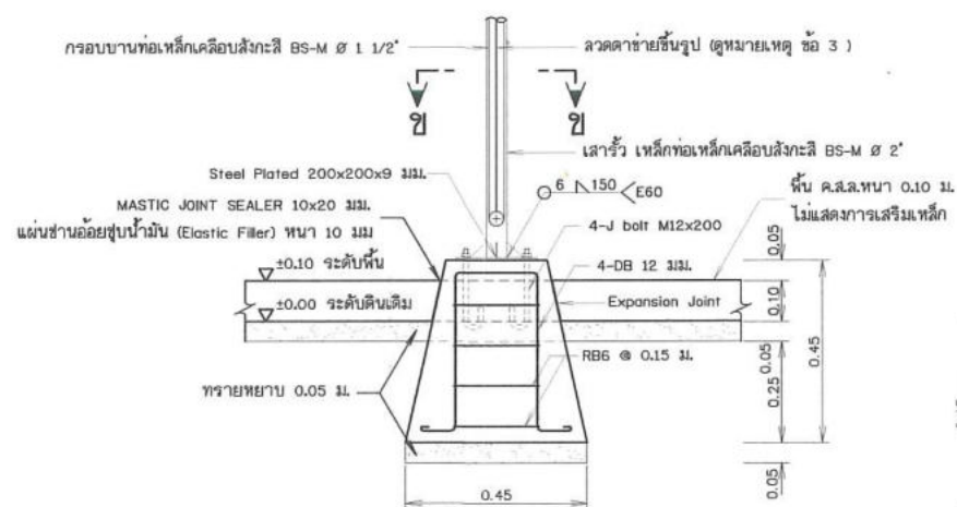
รูปขยายฐานรากโครงสร้างรับแรง F1 (คอม่อ คสล. หล่อสำเร็จรูปพร้อมติดตั้ง) ไม่แสดงมาตราส่วน
