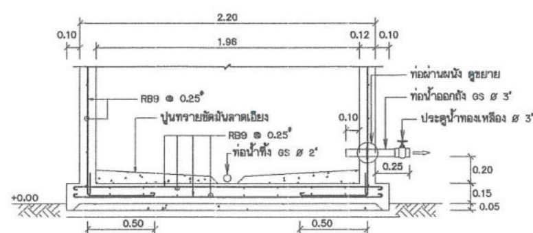
แสดงการเสริมเหล็กพื้นถึง มาตราส่วน 1:20
