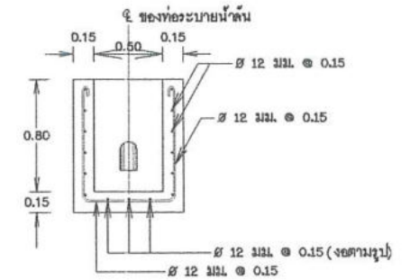
รูปตัดแนว 1 - 1 มาตราส่วน 1:25
