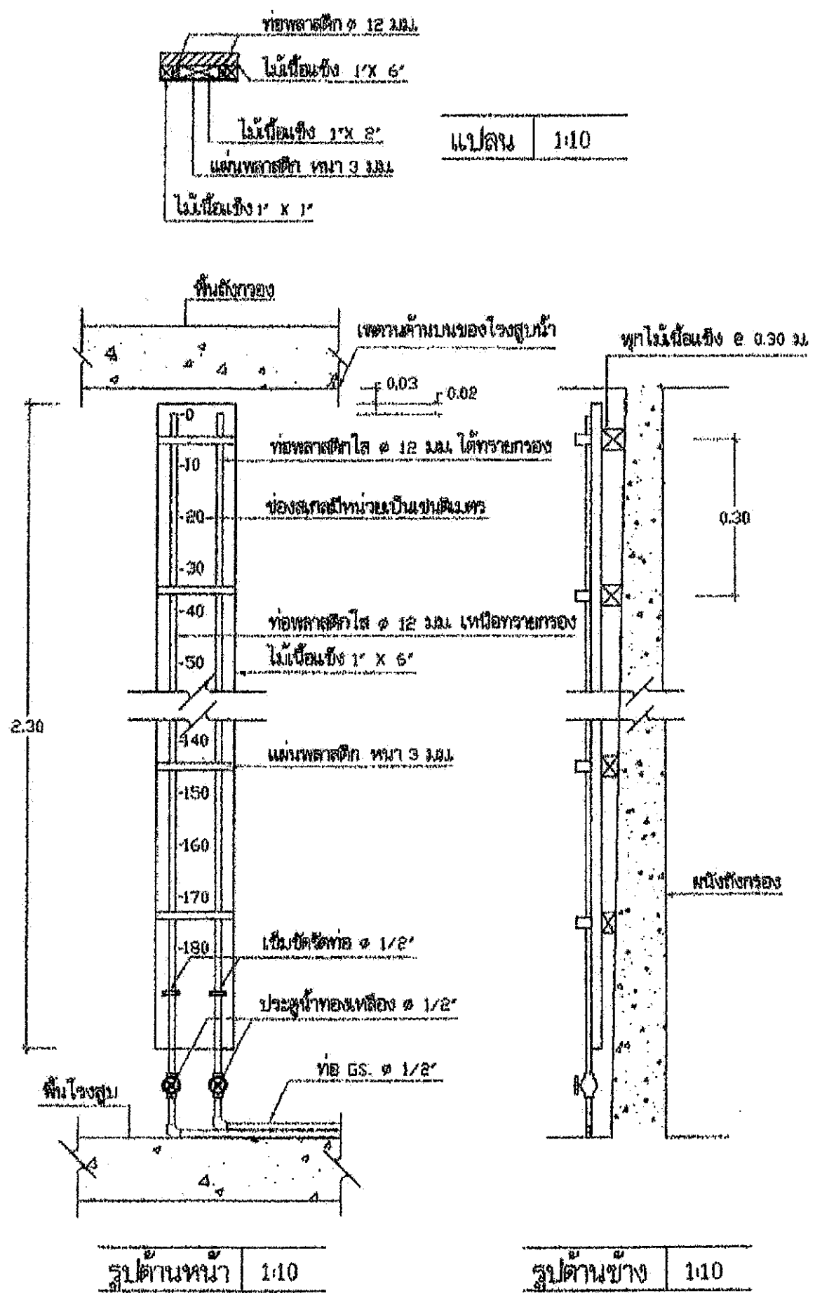
แบบขยาย บัญชีบ่อระดับน้ำเหนือและใต้ทรายกรอง 1:10
