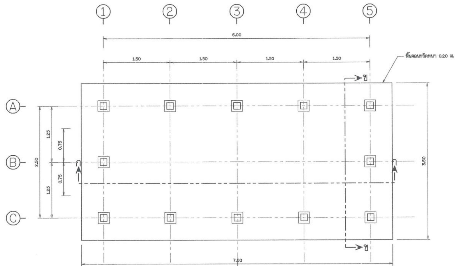
แบบแปลน ไม้แดงขนาดจั่วส่วน
