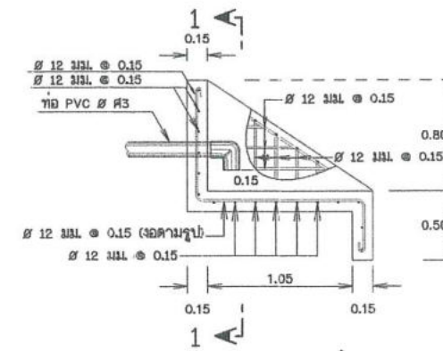
ขยายอาคารปลายท่อระบายน้ำ มาตราส่วน 1:25
