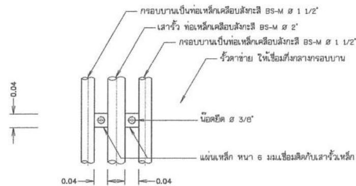
แบบขยายรายละเอียดการยึดระหว่างรั้วกับเสา
