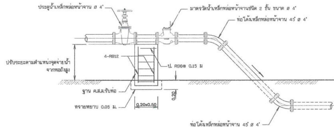
13. การติดตั้งมาตรวัดน้ำบนพื้นดิน 4" ไม่แสดงมาตราส่วน
