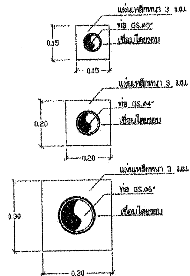
แบบขยายท่อจุดที่ตามผนัง
