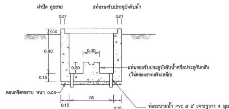
รูปตัด 1 - 1
