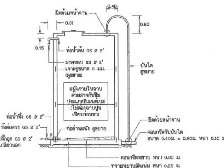
รูปตัด (2) มาตราส่วน 1:40
