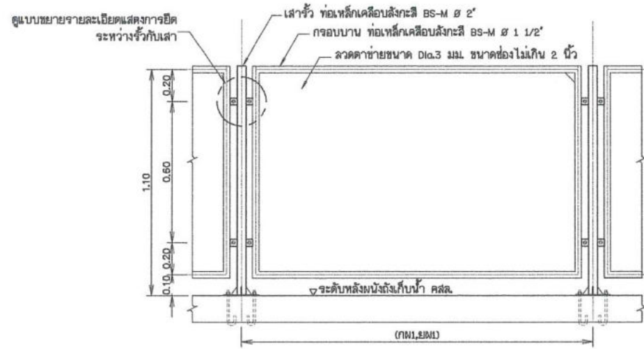
แบบขยายราวกันตก (สำหรับถังเก็บน้ำ คสล. แบบไม่มีฝาด)
