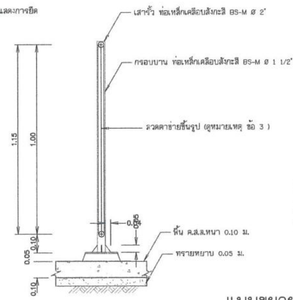
รูปตัด ก-ก ไม่แสดงขนาดจริง
