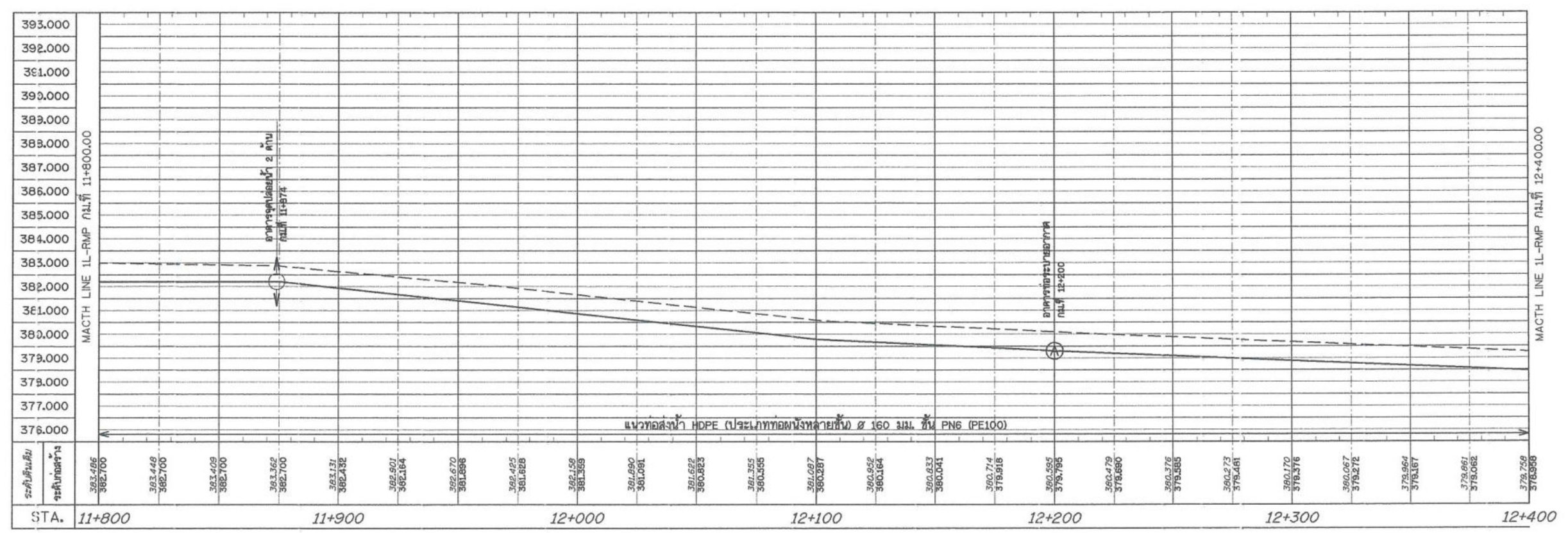
แปลนระบบส่งน้ำ สาย 1L-RMP. STA. 11+800 - 12+400 มาตราส่วน 1:1,000
