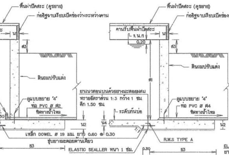
รูปตัดท่อส่งน้ำ มาตราส่วน 1:50
