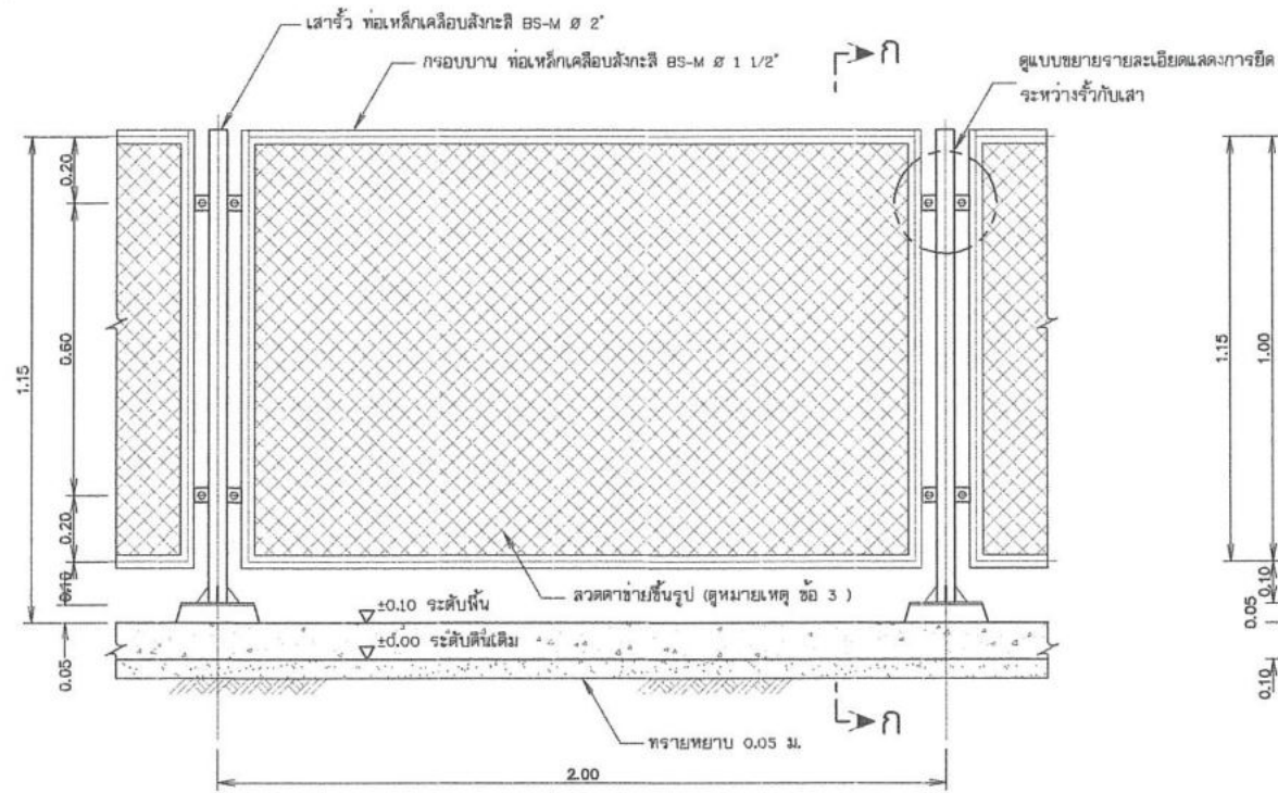
แบบขยายรั้วลวดตาข่าย ไม่แสดงขนาดจริง
