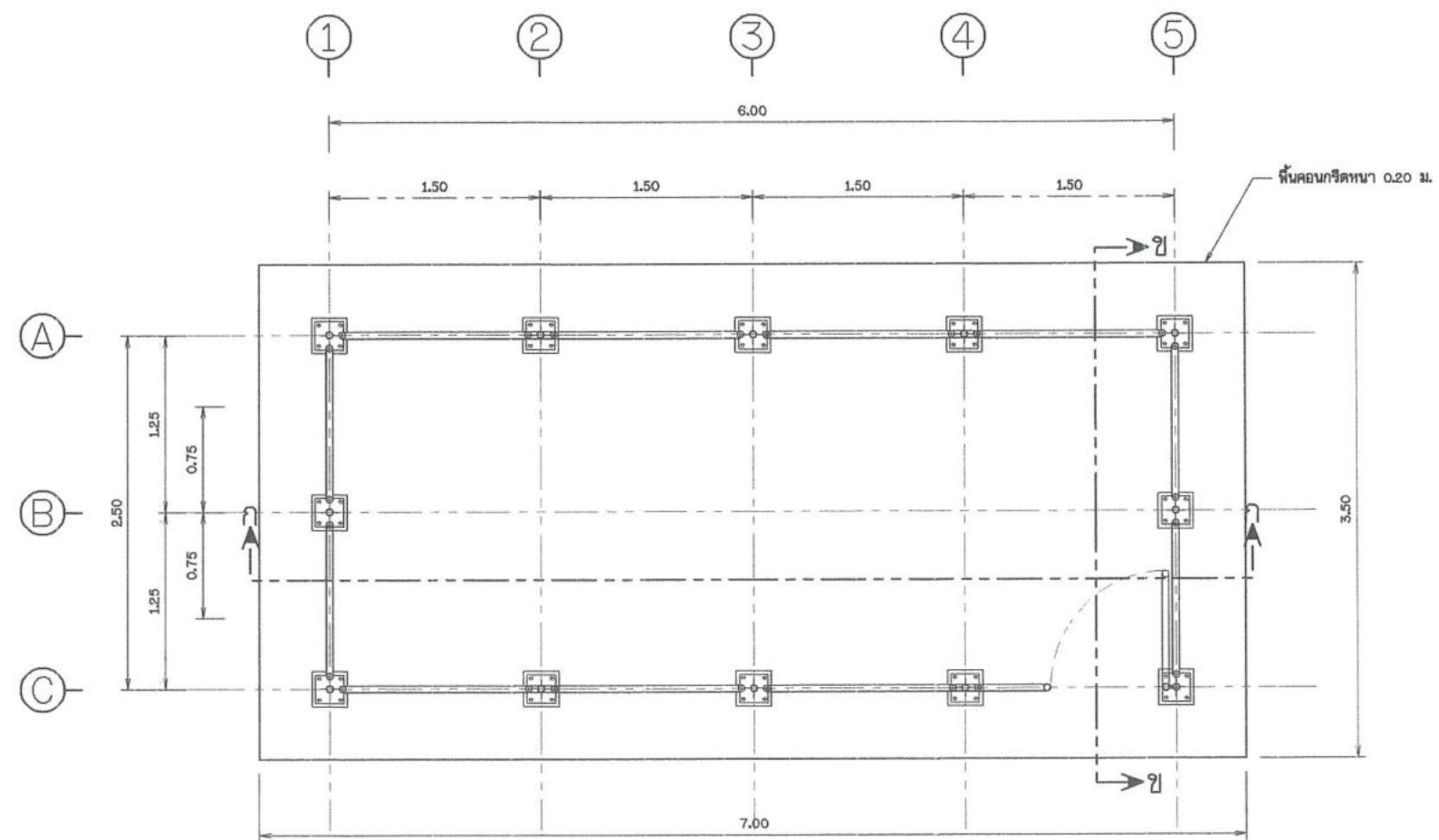
แปลนเสาและรื้อ ไม้แดงขนาดจั่วส่วน
