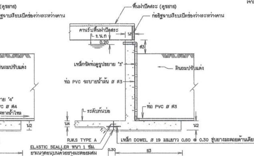
รูปตัดท่อรับน้ำหรือท่อระบายน้ำ มาตราส่วน 1:50
