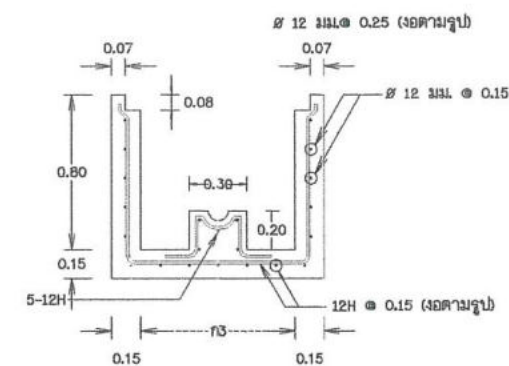
เหล็กเสริมบ่อประตูปังคับน้ำ
