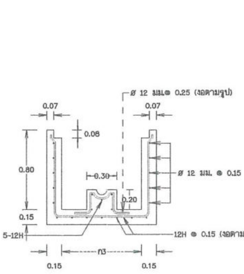
เหล็กเสริมบ่อประตูปรับคันน้ำ มาตราส่วน 1:20
