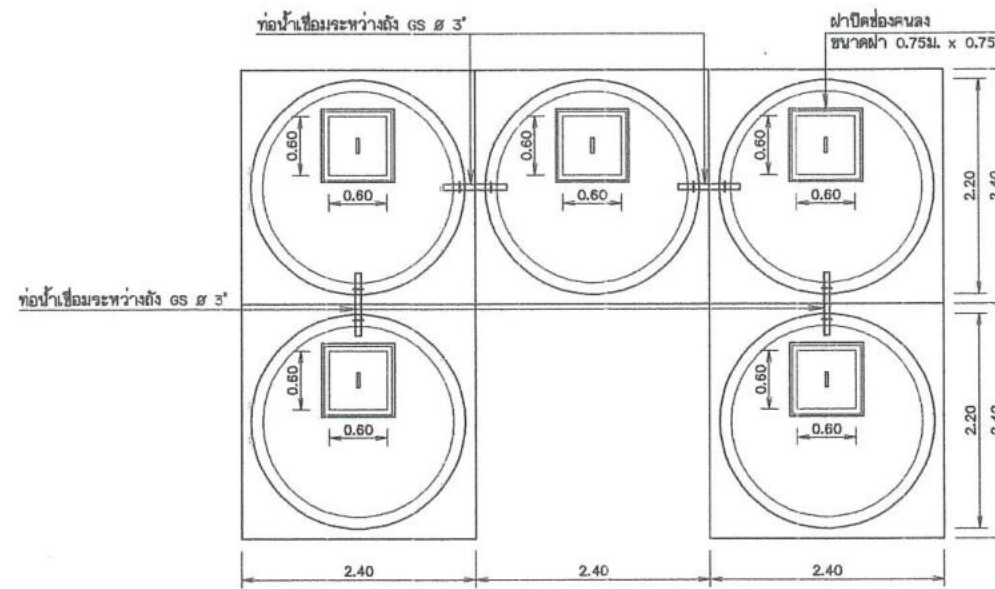
แปลนแบบ 5 ถึง มาตราส่วน 1:40
