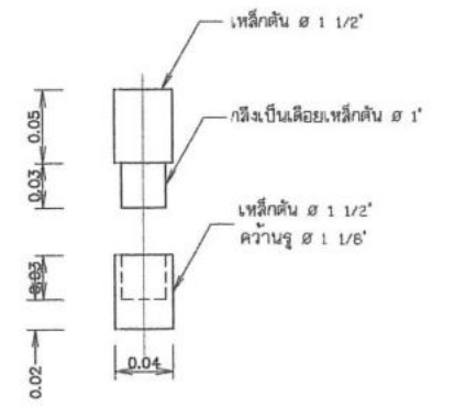
แบบขยายบานพับหัวเหล็ก ไม่แสดงขนาดจริง
