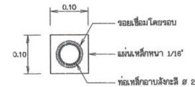
ขยายท่อผ่านผนัง มาตราส่วน 1:5
