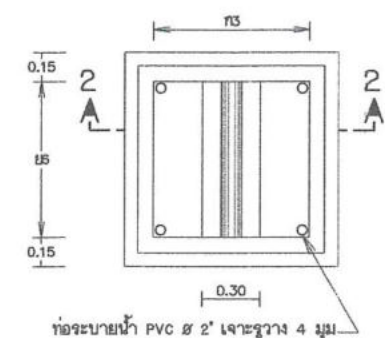
แปลนบ่อประตูปรับคันน้ำ มาตราส่วน 1:20
