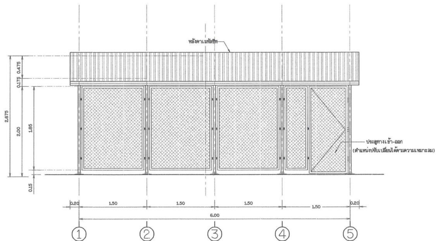
รูปด้าน 1 ไม่แสดงมาตราส่วน
