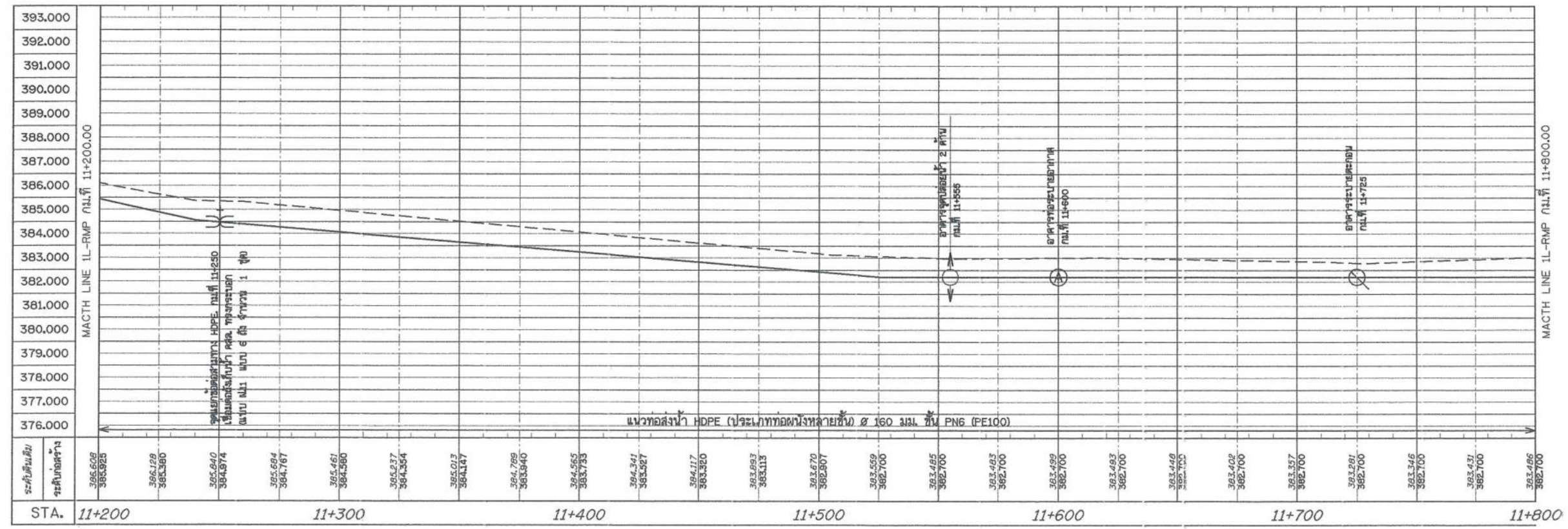
แปลนระบบส่งน้ำ สาย 1L-RMP. STA. 11+200 - 11+800 มาตราส่วน 1:1,000
