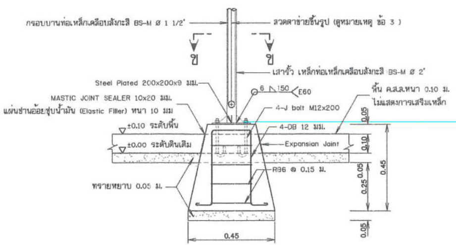
รูปขยายฐานรากโครงสร้างรับแผง F1 (ต่อม่อ คสส. หล่อสำเร็จรูปพร้อมติดตั้ง) ไม่แสดงขนาดจริง
