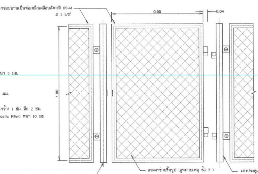
แบบขยายรายละเอียดประตู ไม่แสดงขนาดจริง
