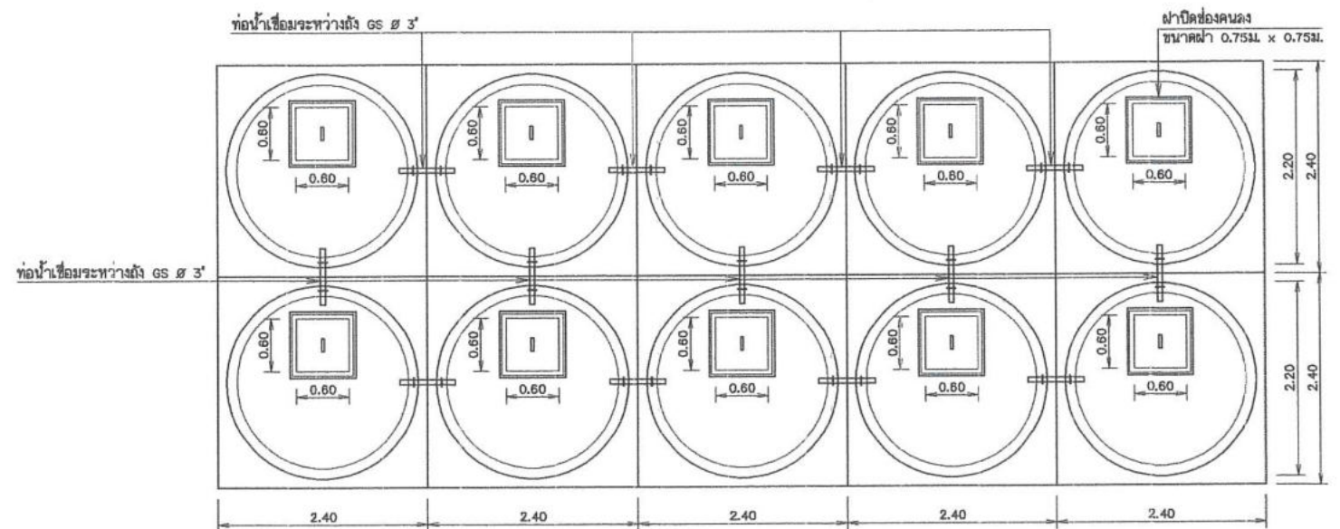
แปลนแบบ 10 ถึง มาตราส่วน 1:40
