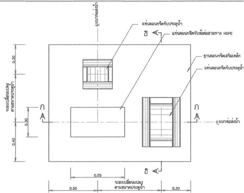
แปลนฐานคอนกรีตเสริมเหล็ก
