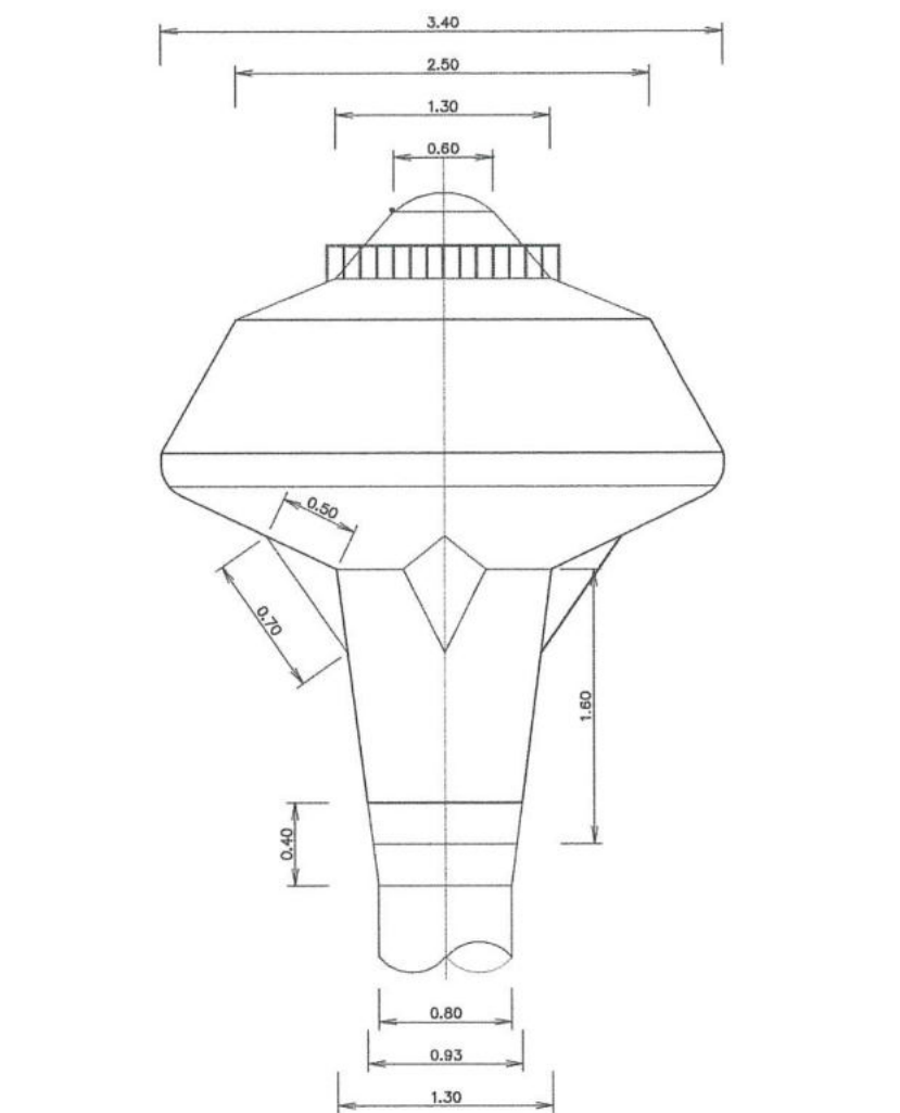
แบบขยายแมนโฮลบนหอถึงสูง
