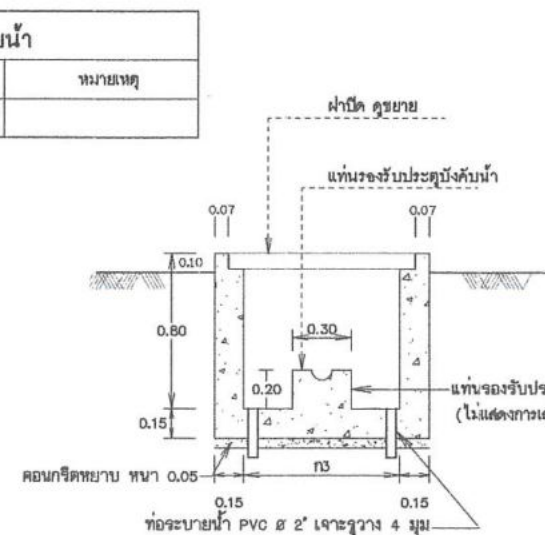
รูปตัด 2 - 2 มาตราส่วน 1:20
