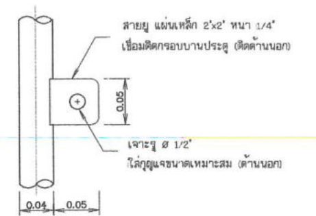
แบบขยายสายยู ไม่แสดงขนาดจริง
