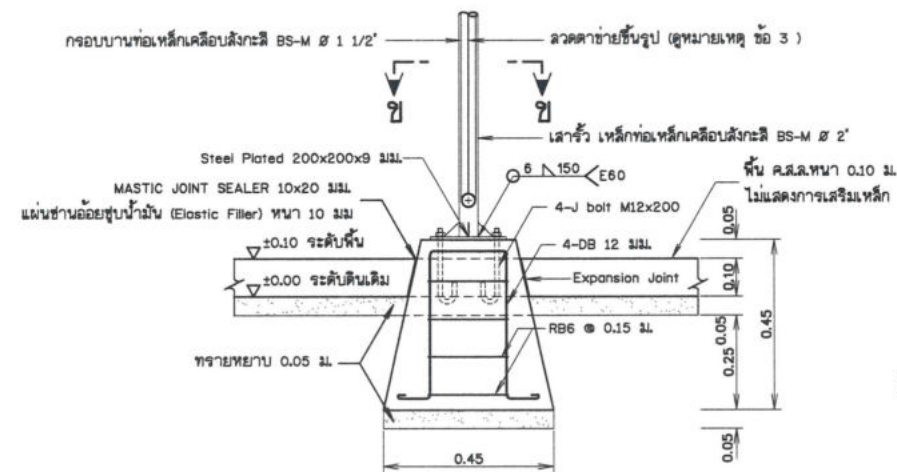
รูปขยายฐานรากโครงสร้างรับแผง F1 (ต่อม่อ คสล. ท่อส่วร้วรูปพร้อมติดตั้ง) ไม่แสดงขนาดจั่วส่วน
