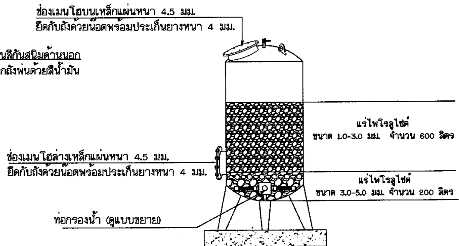
แบบแสดงส่วนประกอบสารกรองถังน้ำ , เมนโฮ Scale 1 : 25
