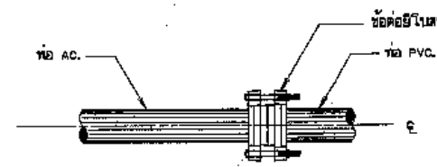
การบรรจุท่อ AC. กับท่อ PVC.
