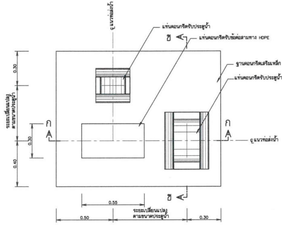
แปลนฐานคอนกรีตเสริมเหล็ก มาตราส่วน 1:10
