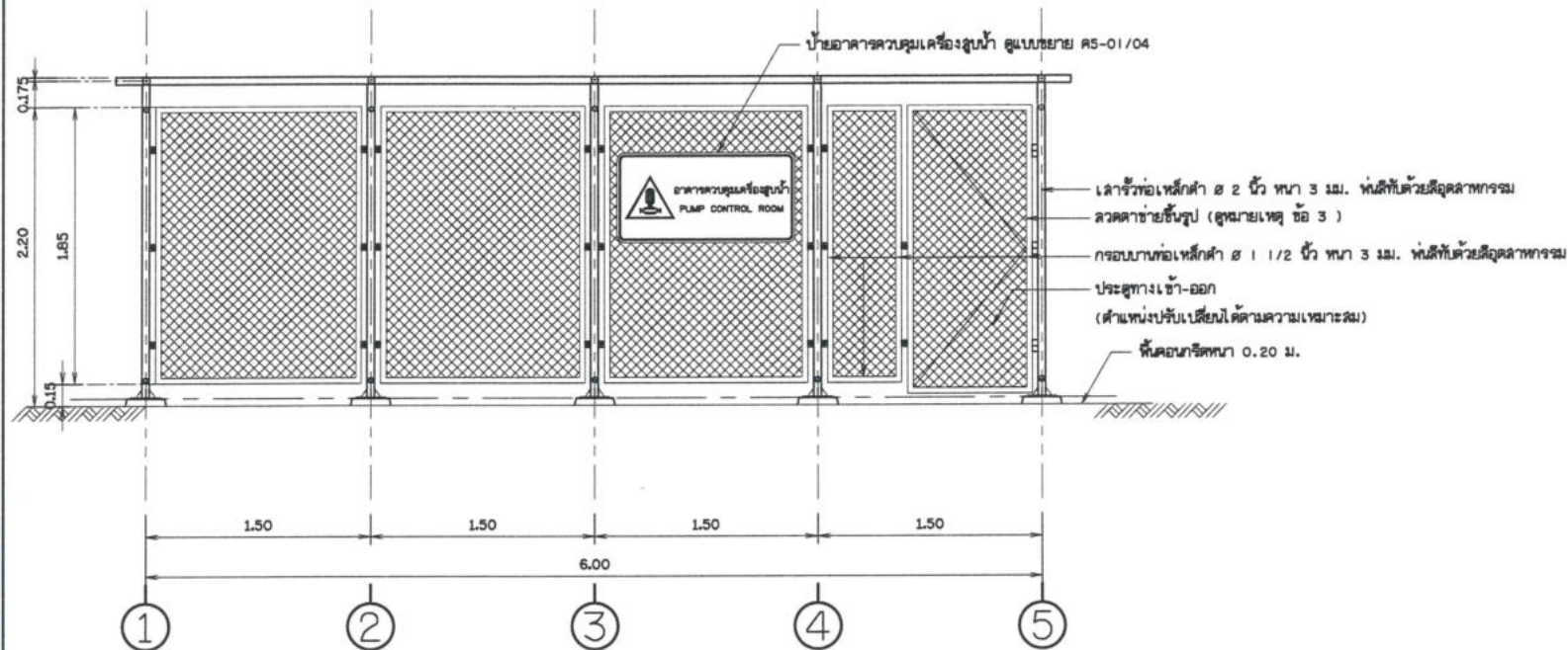
แบบขยายรั้ว 1 ไม่แสดงมาตราส่วน
