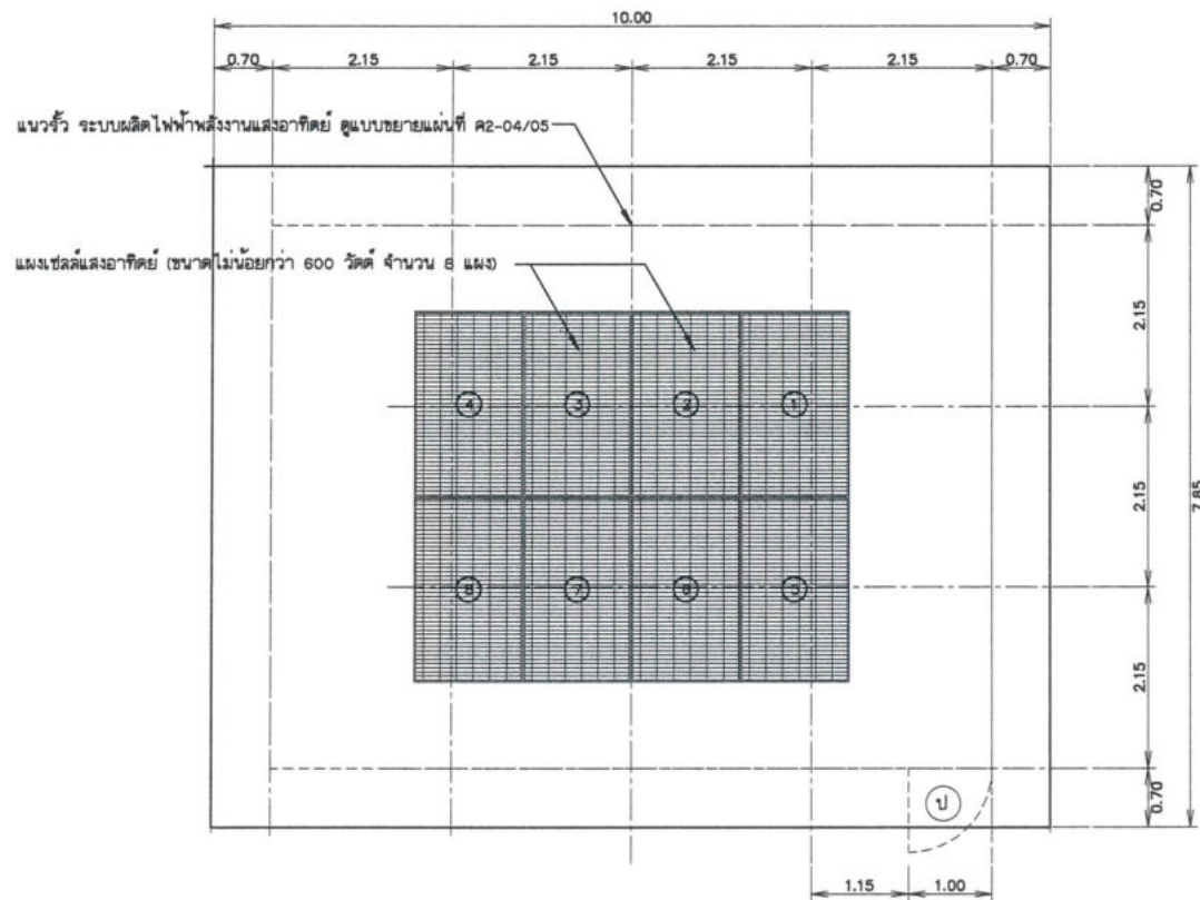
แปลนการติดตั้งแผงเซลล์แสงอาทิตย์ พร้อมรั้ว จำนวน 4 ชุด
