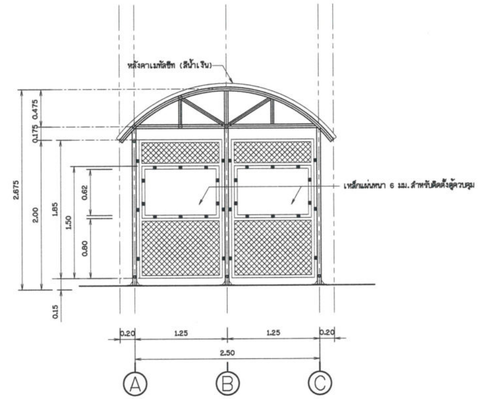
รูปด้าน 2 ไม่แสดงขนาดราวกว
