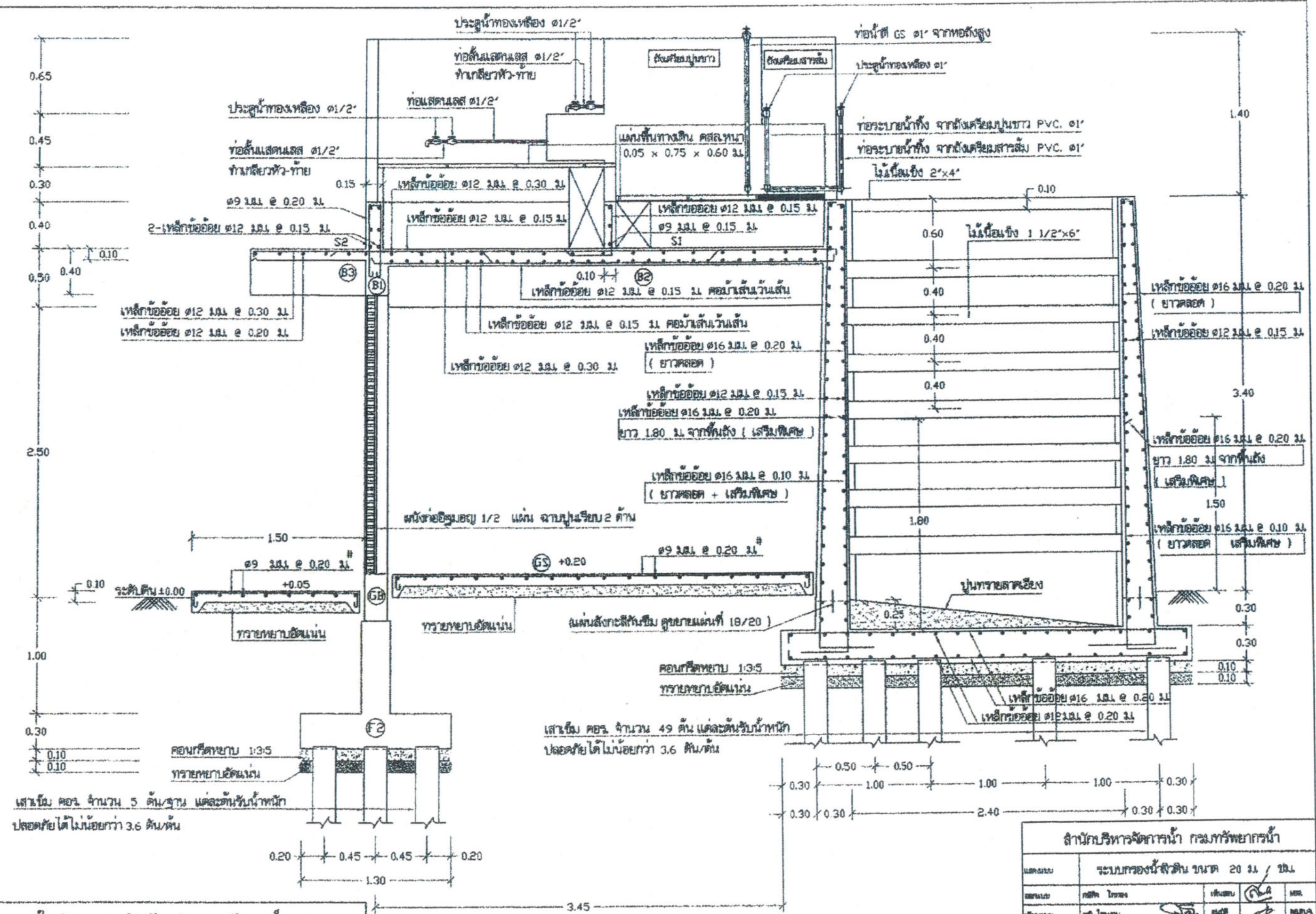
รูปตัด ก - ก 1:30
