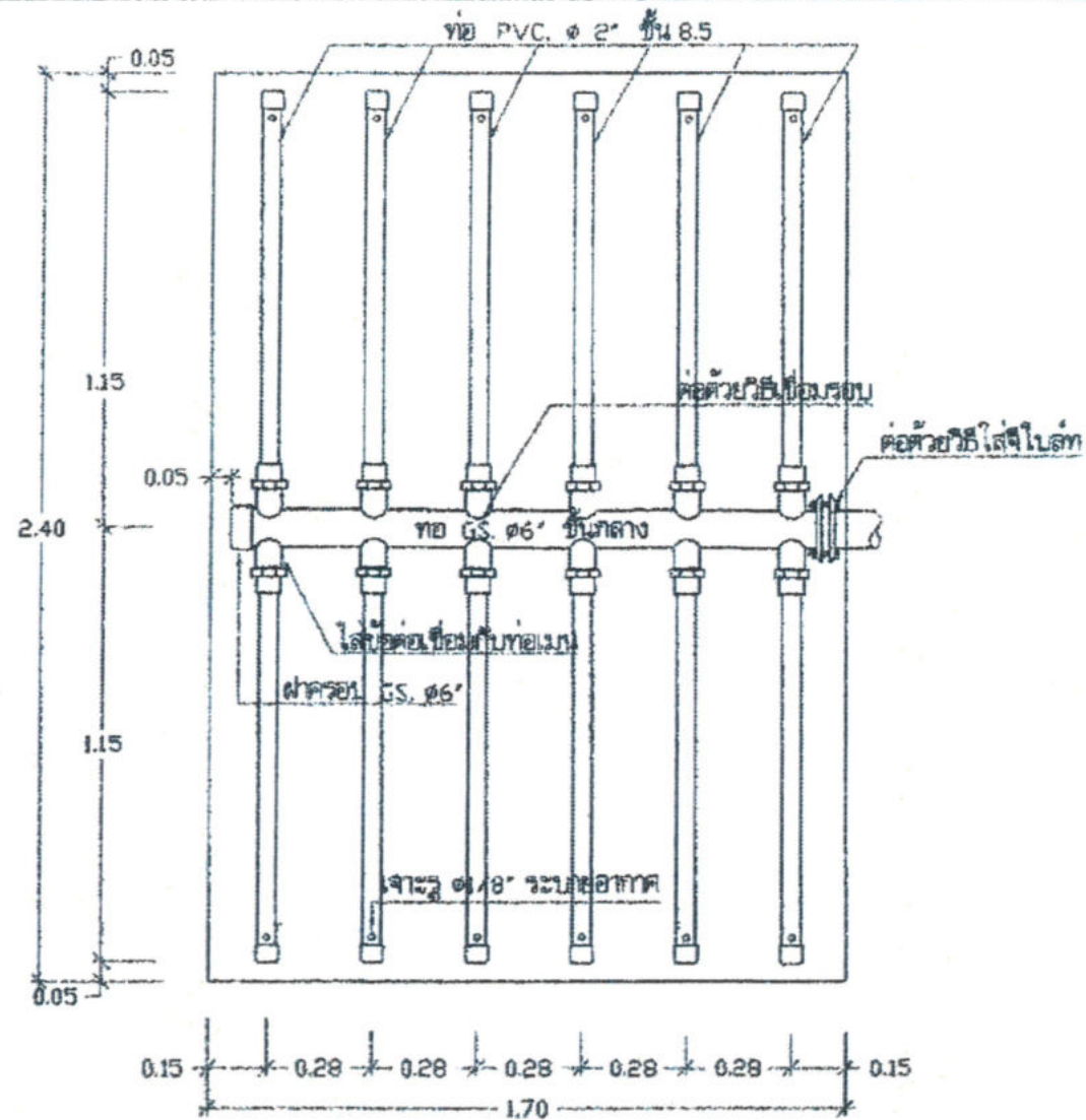
แบบขยายท่อถังปลา 1:20
