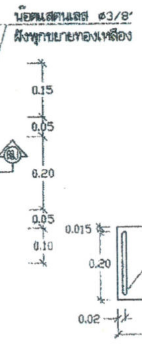
แบบขยายแผ่นอุดรูในแบบปรับระดับ 1 : 10
