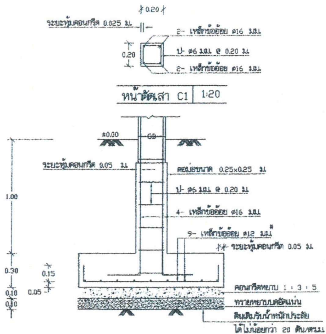
รูปตัด ฉ - ฉ 1:20
