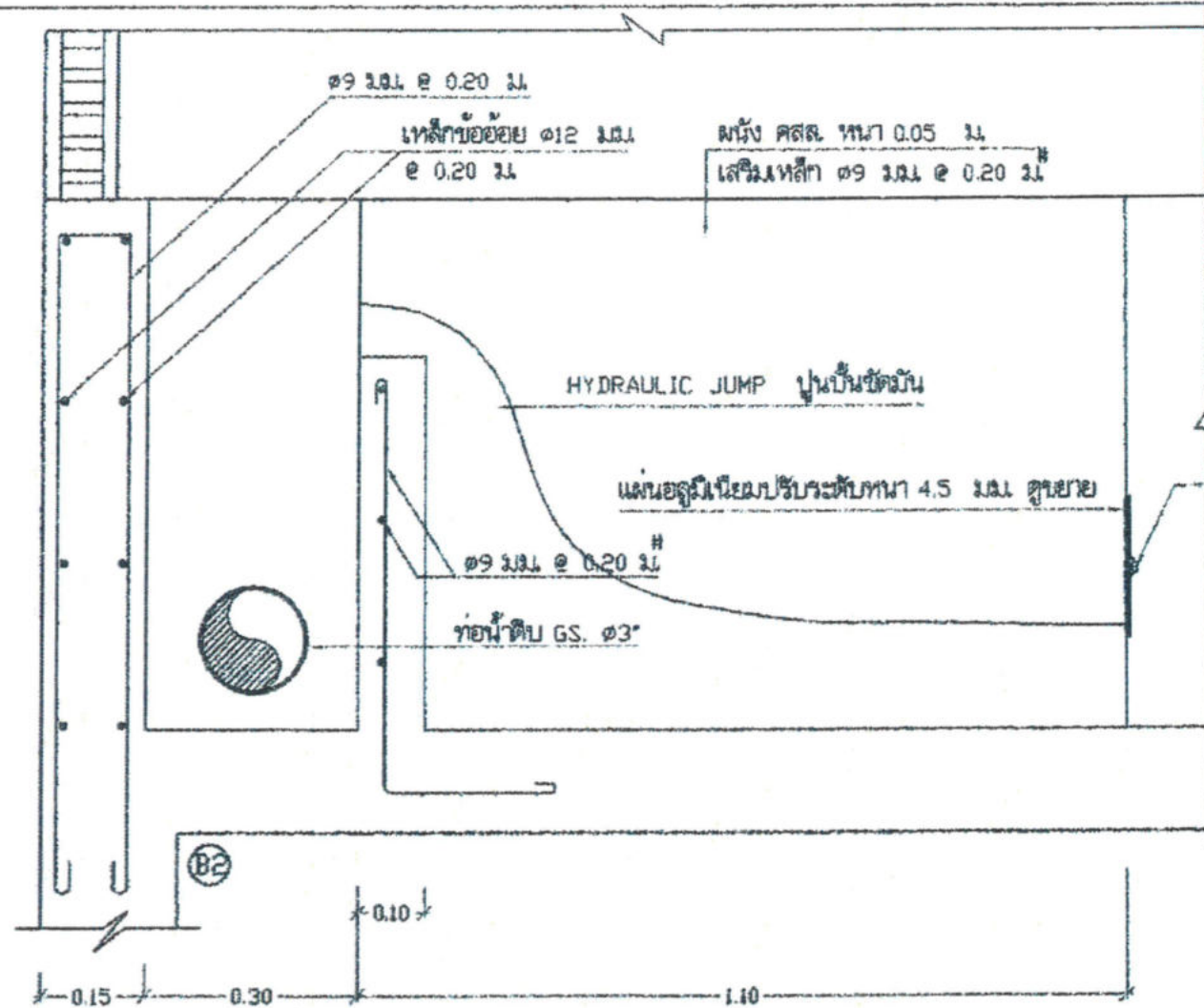
รูปตัด (A) - (B) 1 : 10
