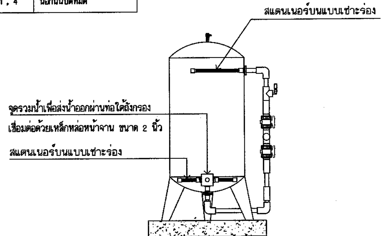
แบบแสดงอุปกรณ์ประกอบถังกรองน้ำภายใน
