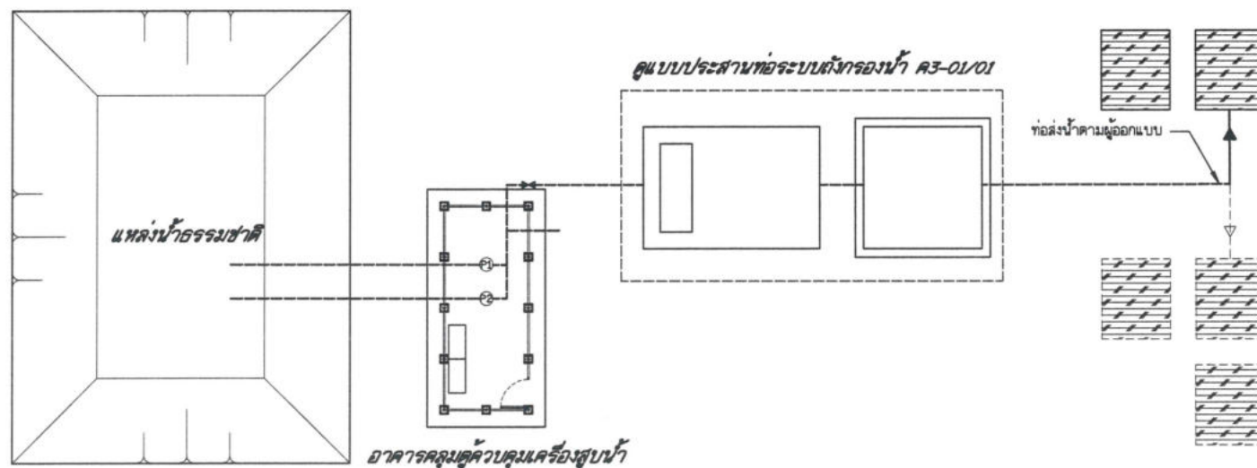
แผนผังระบบกระจายน้ำด้วยพลังงานแสงอาทิตย์ ขนาด 11 กิโลวัตต์
