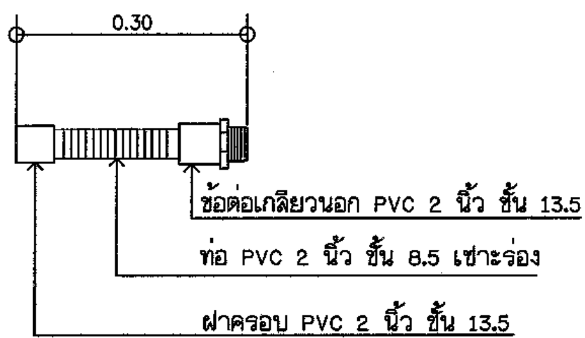
สแตนด์แนวล่างแบบเชาะร่อง
