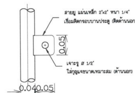
แบบขยายสายรัด ไม่แสดงขนาดจั่วส่วน
