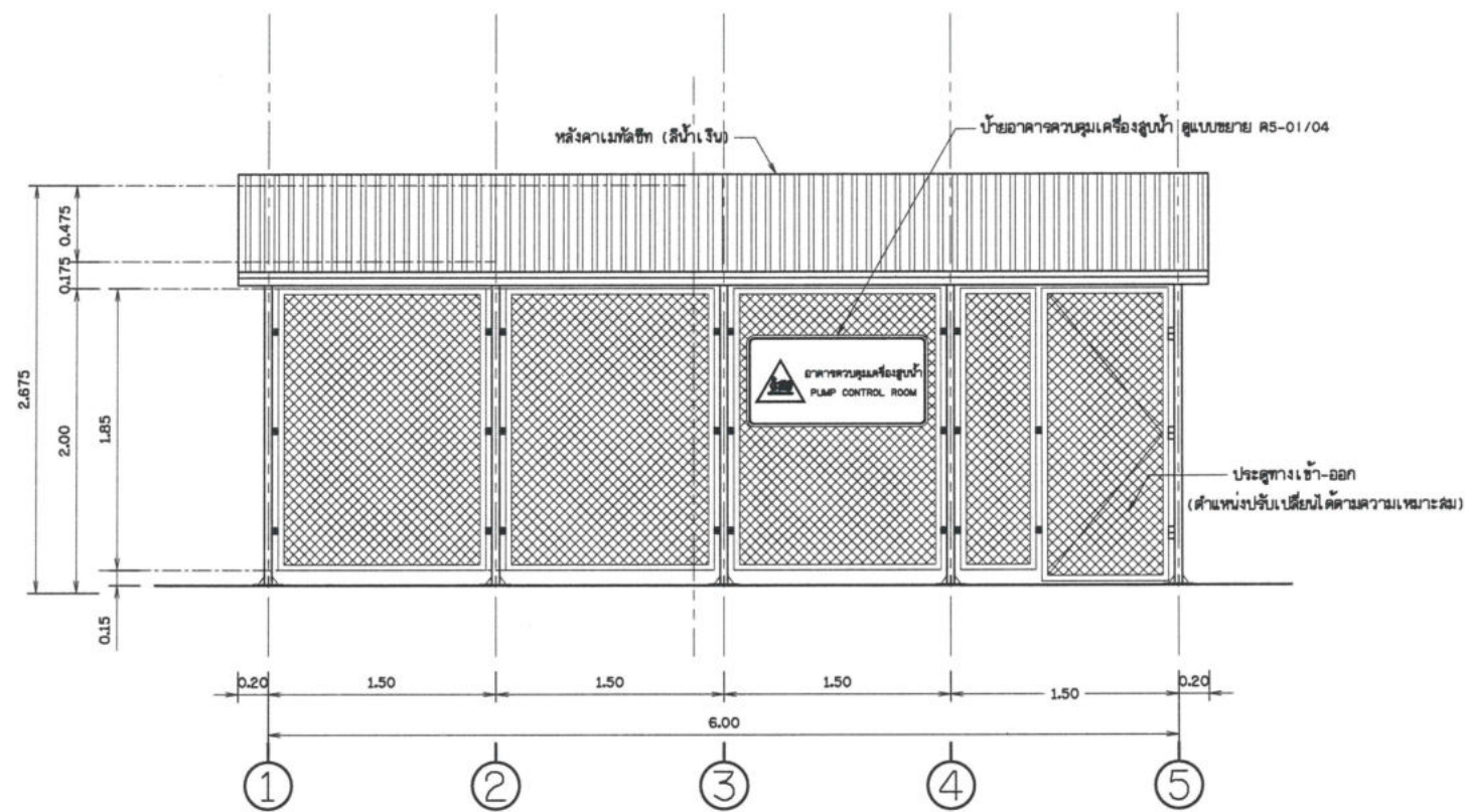
รูปด้าน 1 ไม่แสดงขนาดราวกว
