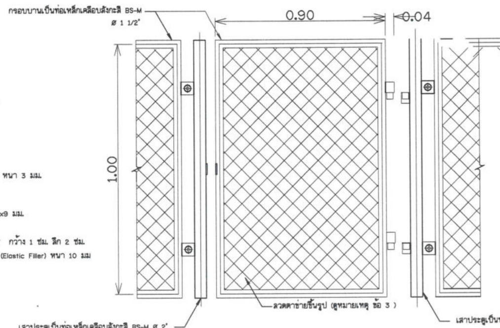
แบบขยายรายละเอียดประตู ไม่แสดงขนาดจั่วส่วน
