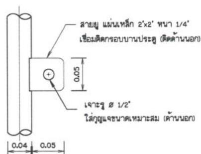
แบบขยายสายโยง ไม่แสดงมาตราส่วน
