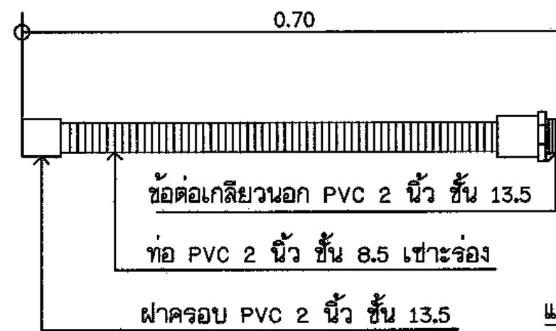
สแตนด์แนวล่างแบบเชาะร่อง
