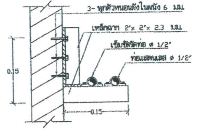
ขยายเหล็กรับท่อสารส้มลงของไฮดรอลิค 1:5
