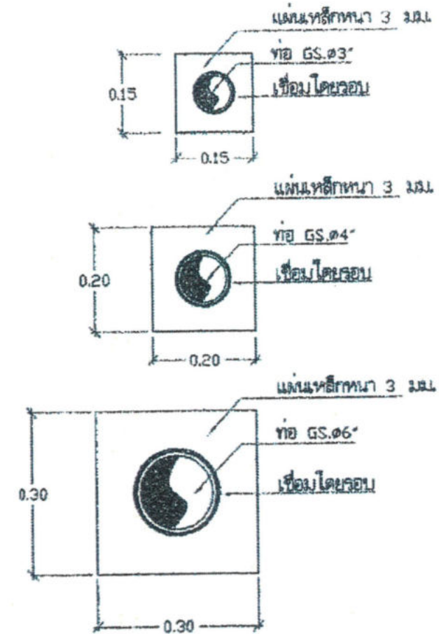
แบบขยายท่อนจุดที่ผ่านผนัง
