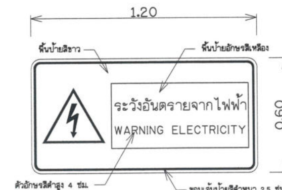
ป้ายเตือนกระแสไฟฟ้า ไม่แสดงขนาดจั่วส่วน
