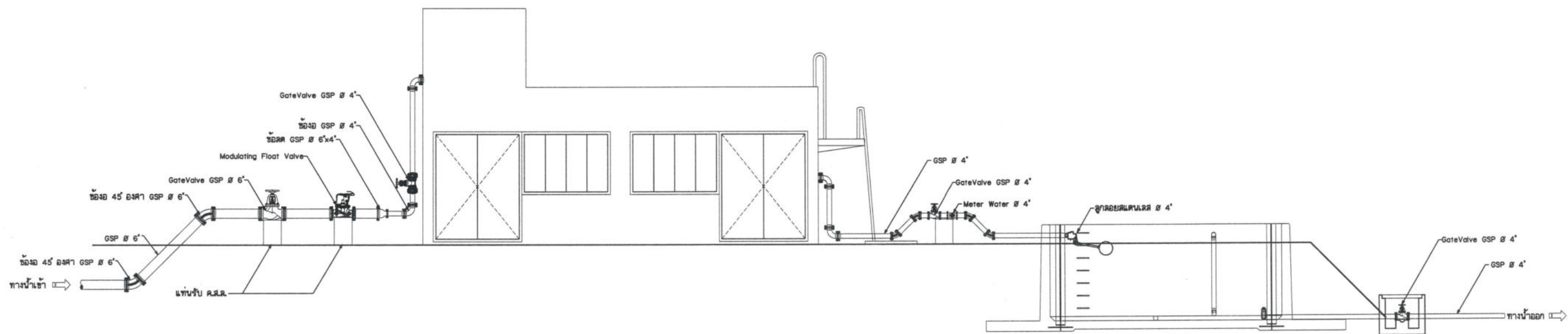
งานประสาณท่อระบบถึงกรองน้ำผิวดิน มาตราส่วน 1 : 100
