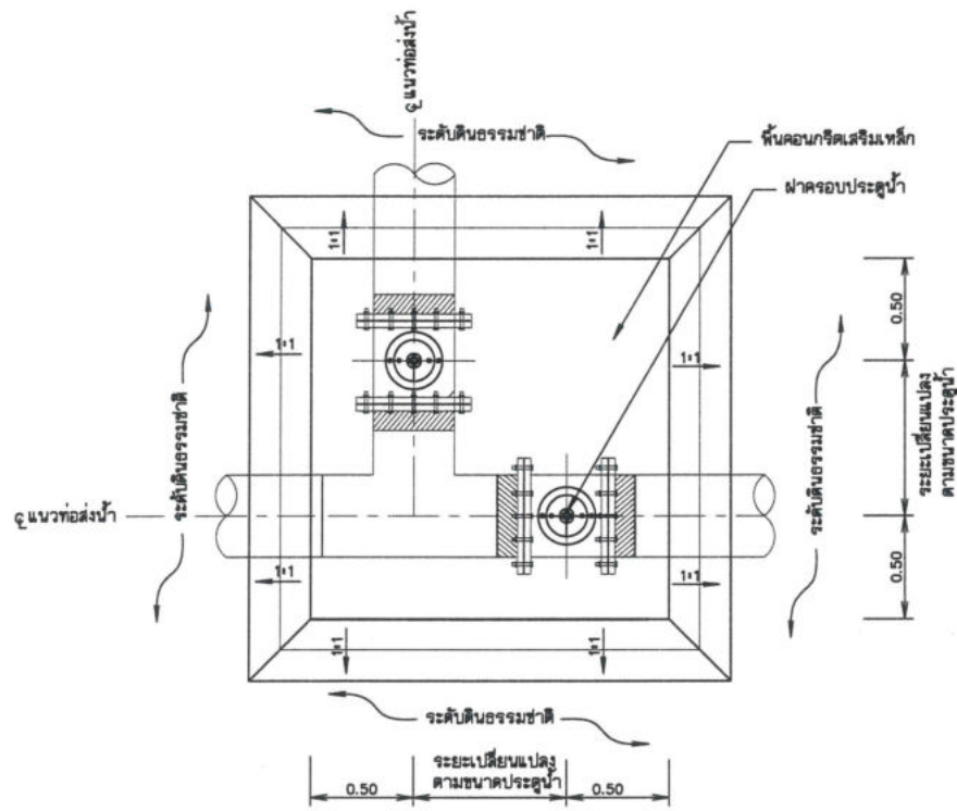
แปลนอาคารจุดแยก มาตราส่วน 1:20
