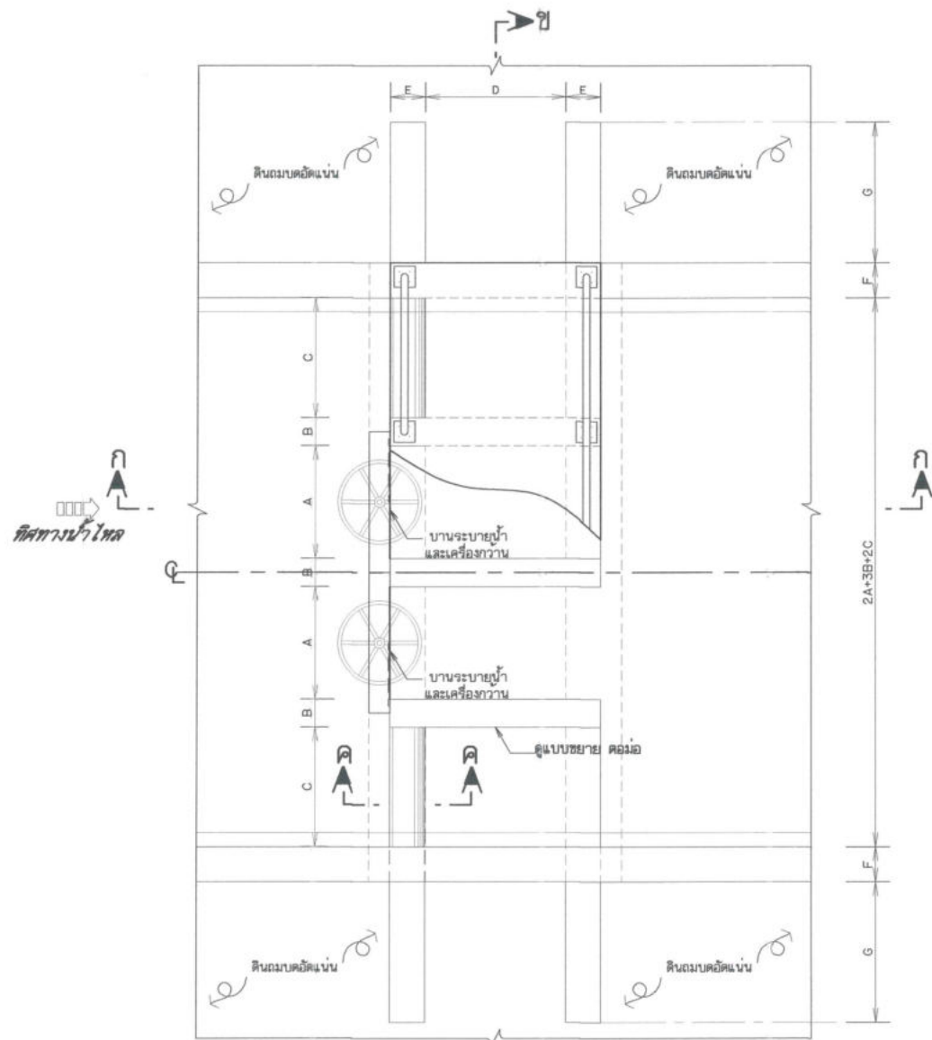
แปลนอาคารอัดน้ำ ไม่แสดงมาตราส่วน
