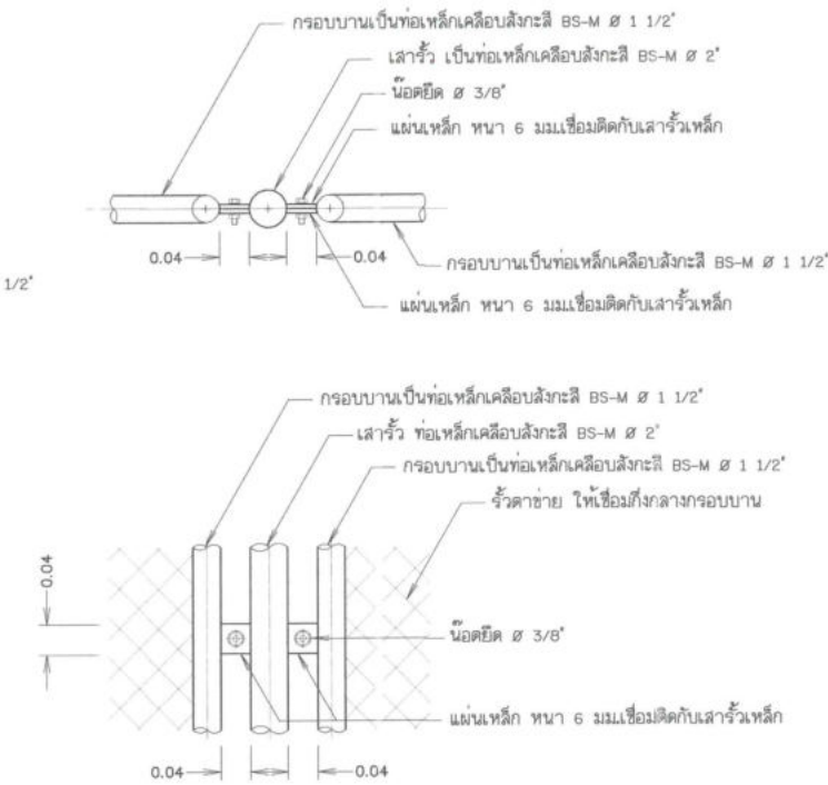
แบบขยายรายละเอียดแสดงการยึดระหว่างหัวกับเสา
