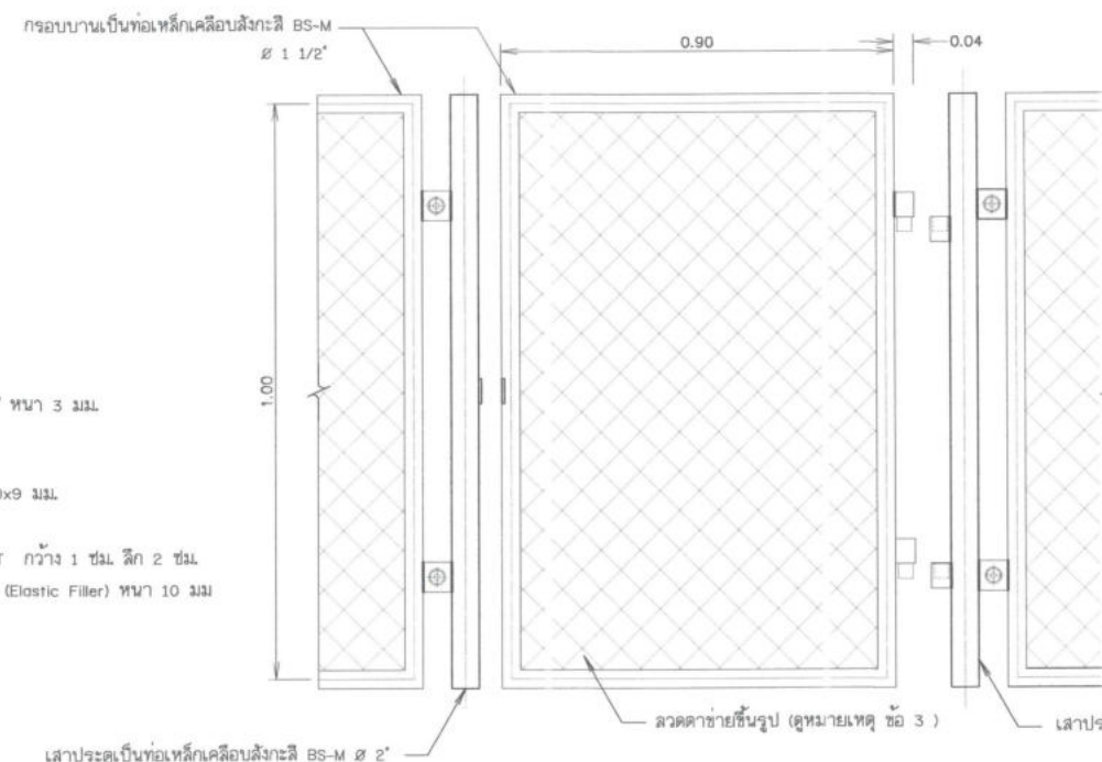
แบบขยายรายละเอียดประตู
