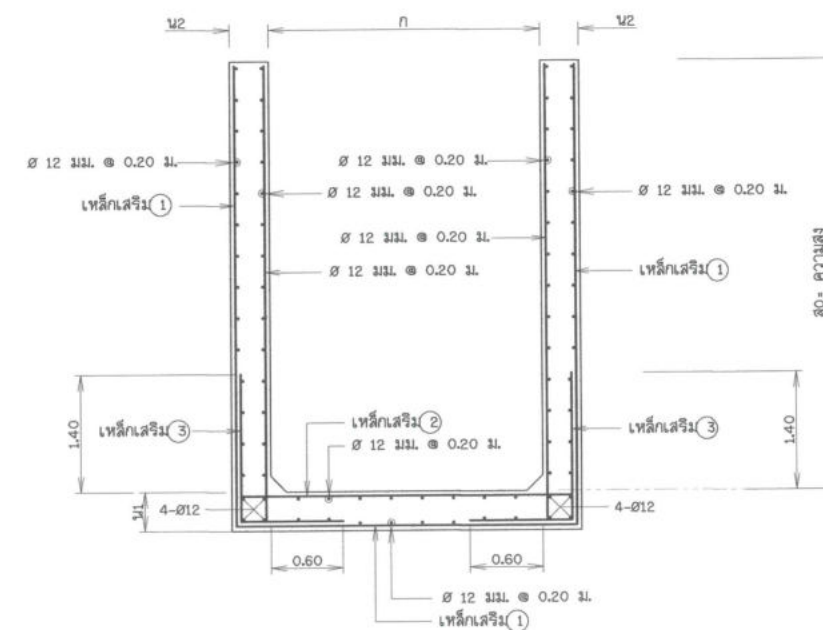
รูปแสดงการเสริมเหล็ก
