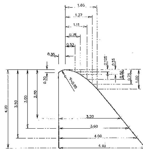
รูปขยายลัดส่วนฝาย ค2 มาตราส่วน 1:50
