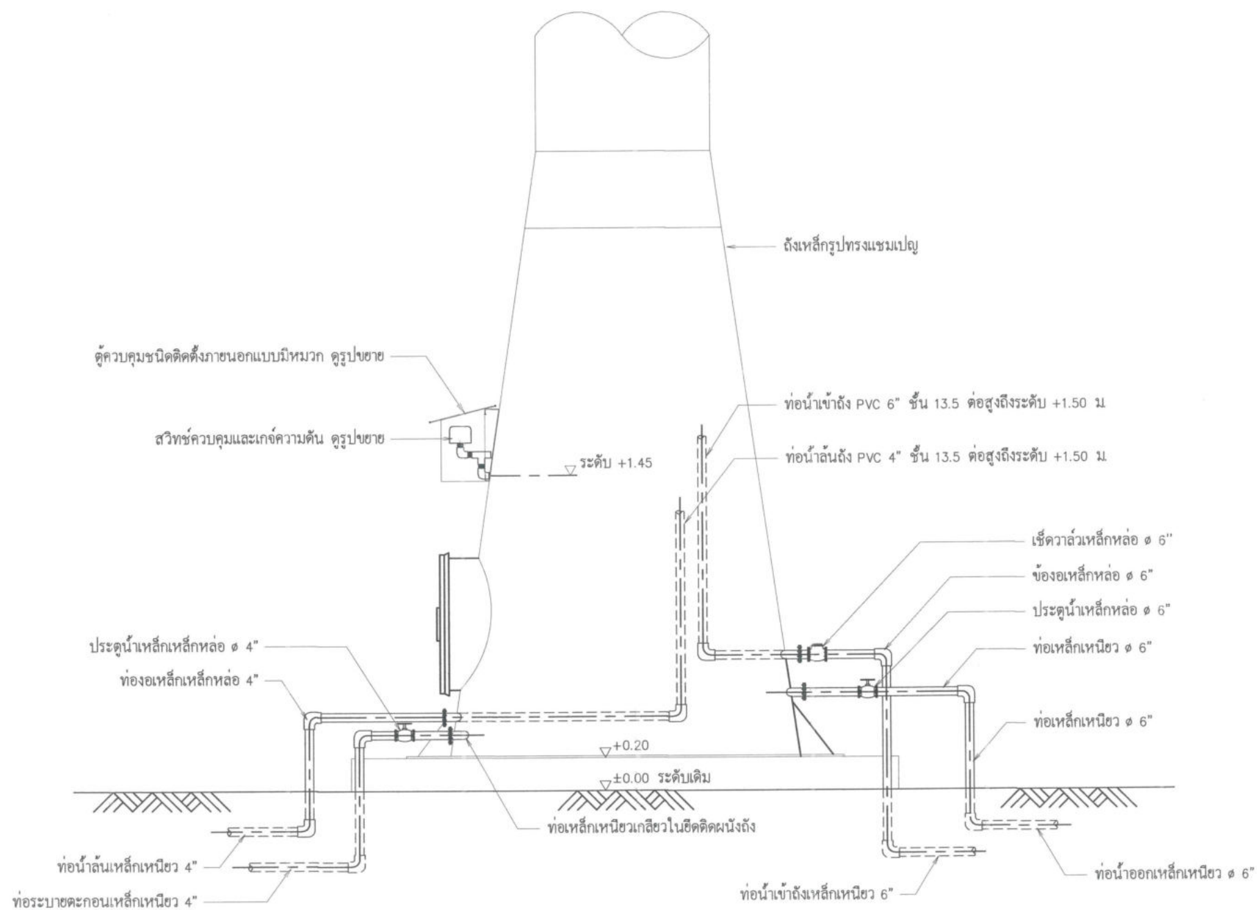
แบบแสดงการเดินท่อในหอถังสูง
