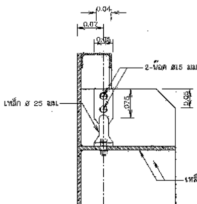
รูปขยาย ตำแหน่งจุดยึดตรอกโซ่กับบานระบาย
