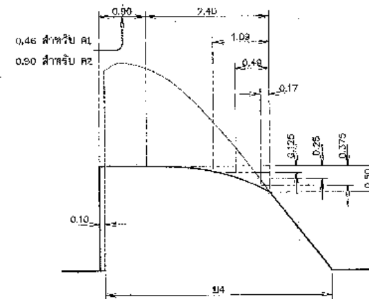
รูปขยายลัดส่วนสันช่องระบายทราย มาตราส่วน 1:50
