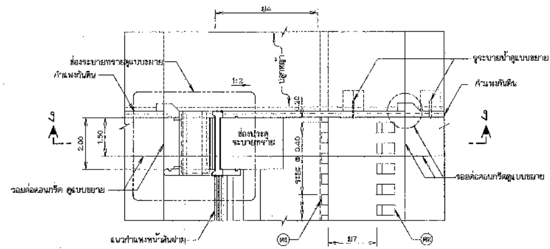
รูปขยาย 1 มาตราส่วน 1:75
