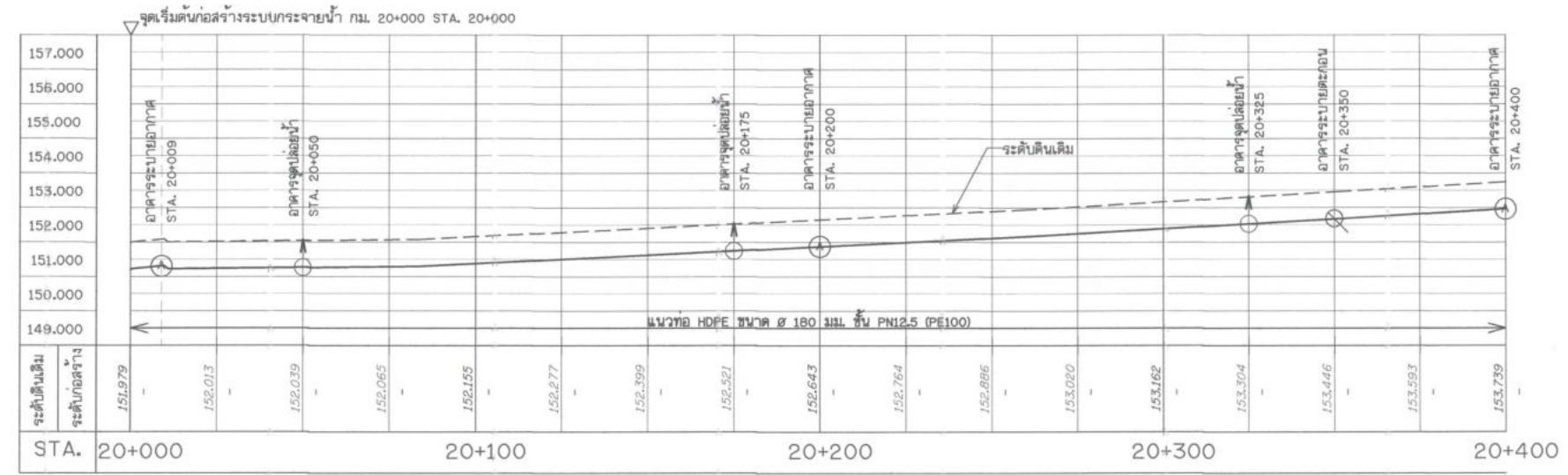
รูปตัดตามแนวยาวท่อส่งน้ำ กม. 20+000 STA. 20+000 - 20+400 มาตราส่วน 1:1,000 แนวนอน 1:1,000 แนวตั้ง 1:100
