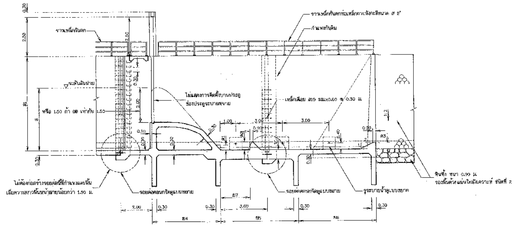
รูปขยาย 2 ตามแนว ก-ง มาตราส่วน 1:75
