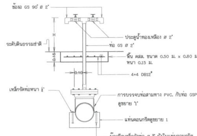
รูปตัดอาคารจุดปล่อยน้ำ 2 ด้าน
