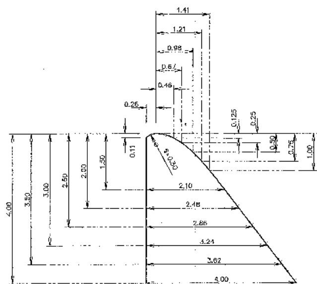
รูปขยายลัดส่วนฝาย ค1 มาตราส่วน 1:50
