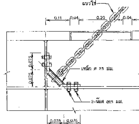
รูปขยาย ตำแหน่งจุดยึดตรอกโซ่กับบานระบาย
