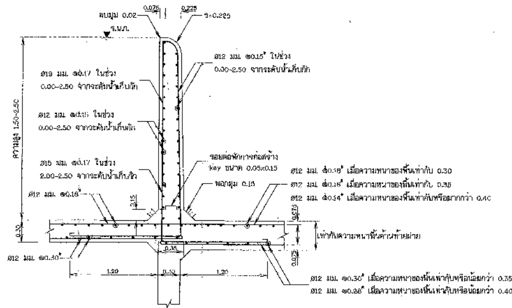
รูปขยายฝายทดน้ำแบบคดตรงความสูงระหว่าง 1.50-2.50
