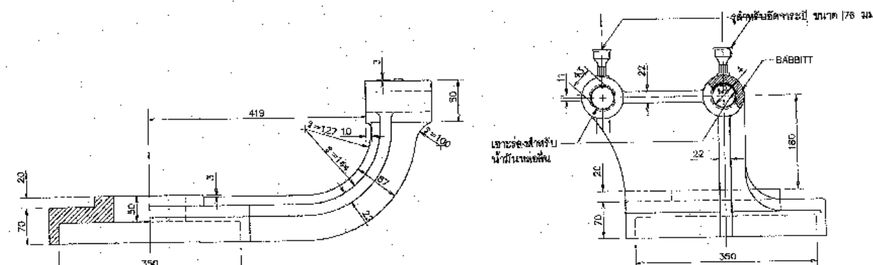
ผ่าครอบและตักดา (เหล็กหล่อ) มาตราส่วน 1:5
