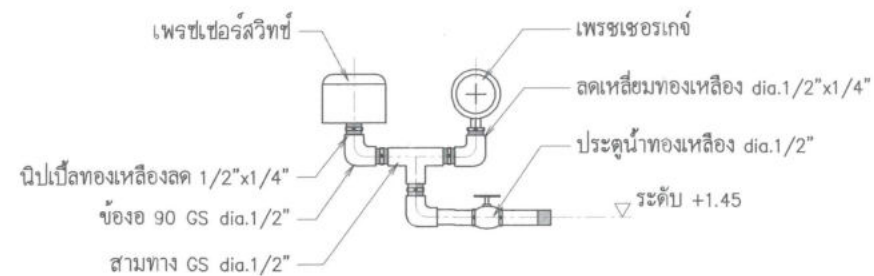
แบบขยายสวิตช์ควบคุมและแก้้ความดัน
