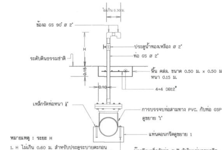
รูปตัดอาคารประตูปะบายตะกอนและอาคารจุดปล่อยน้ำ
