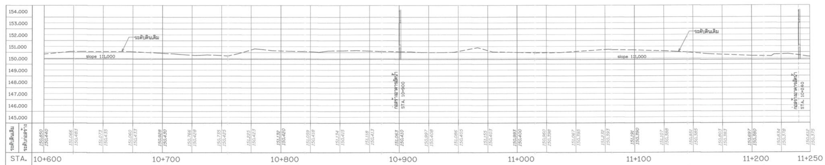
รูปตัดตามแนวยาวคลองส่งน้ำ คสล. กม. 10+000 STA. 10+600 - 11+250
