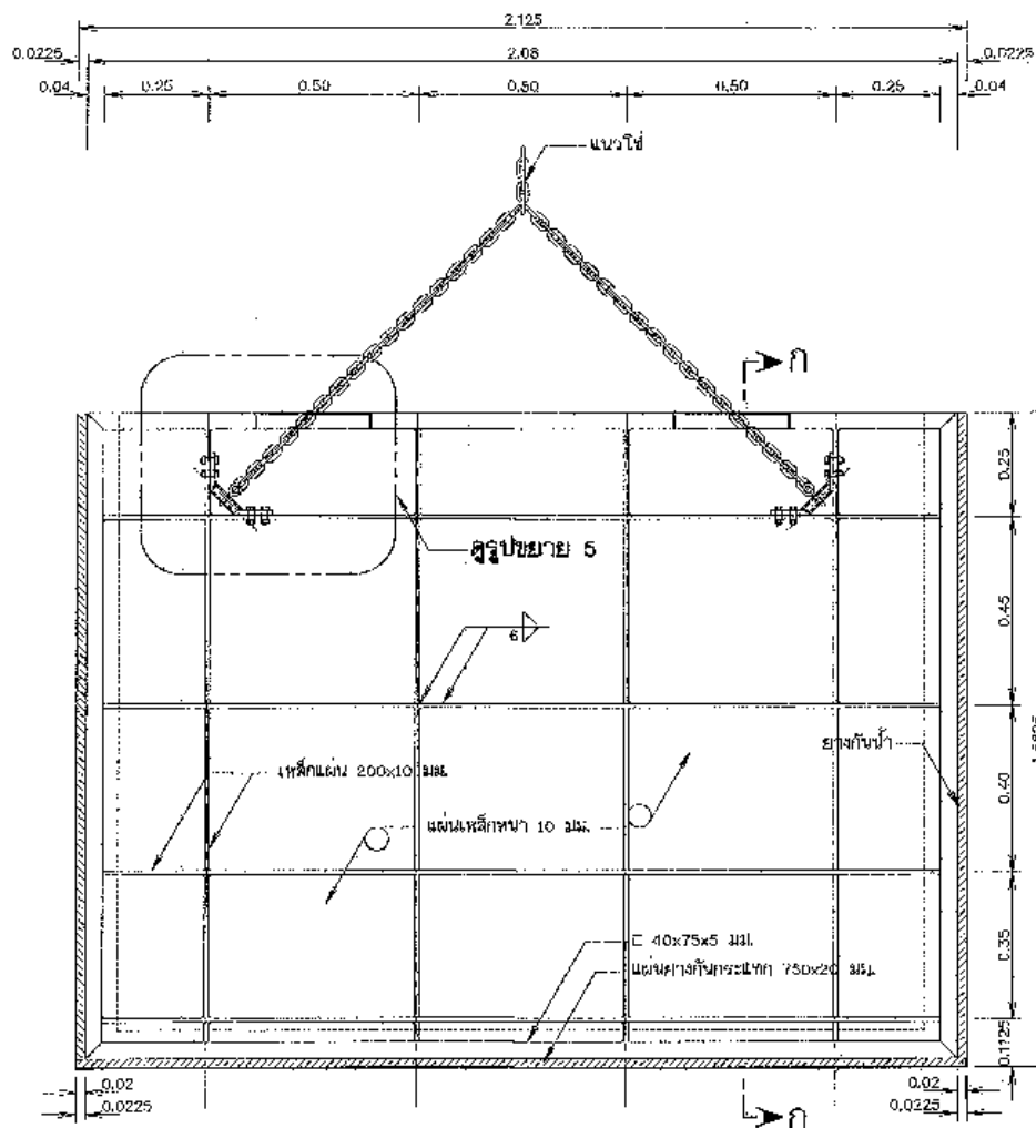
รูปด้านหลังบานประตูประบายทราย
