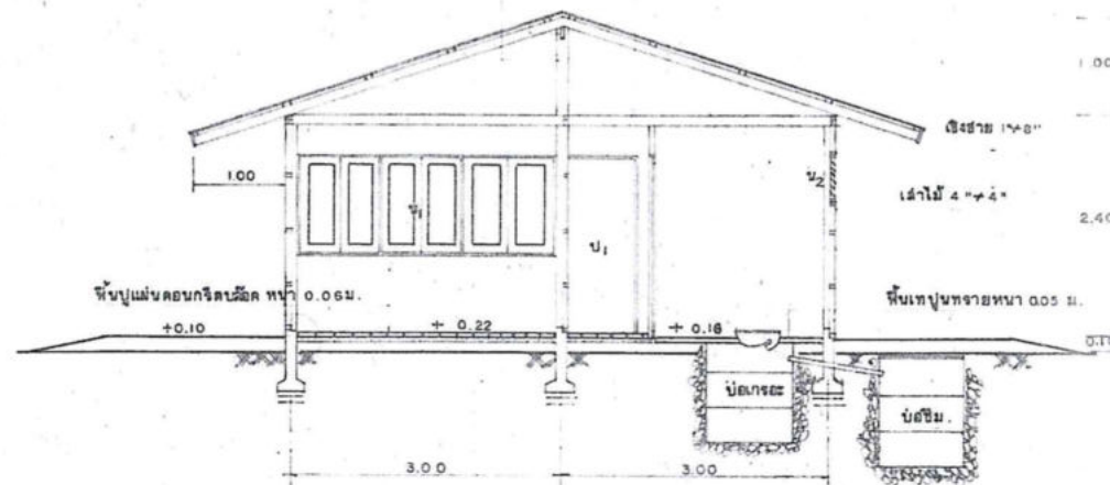
รูปตัด 1850
