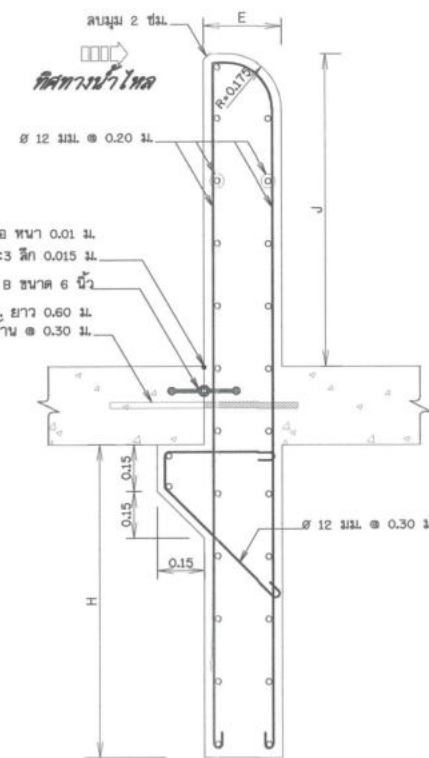
รูปตัด ค - ค ขยายสันฝ้าย ไม่แสดงมาตราส่วน
