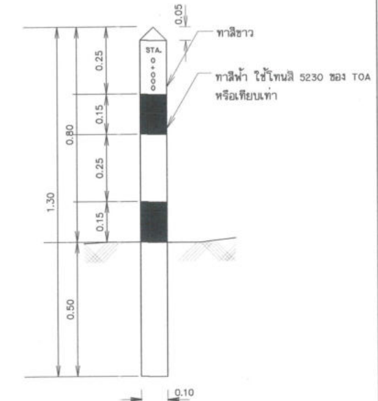
แสดงลัดส่วนหลักบ่อแกวท่อ
