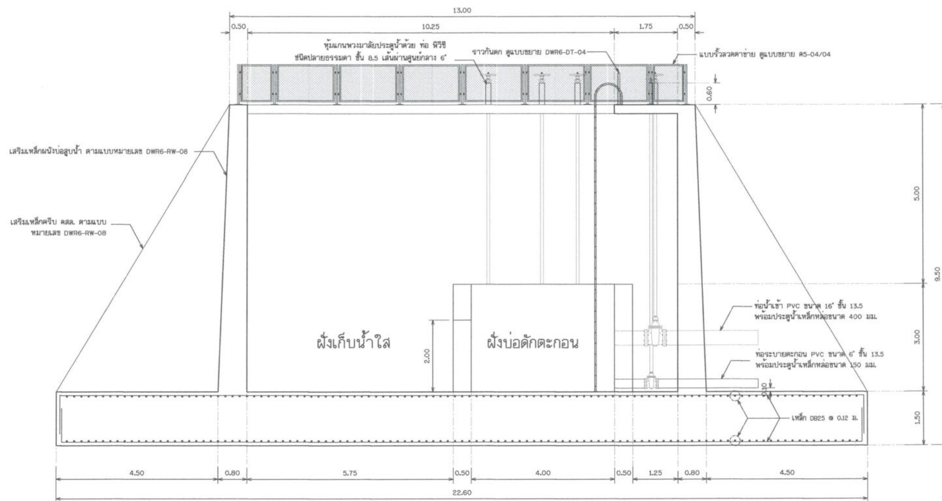
รูปตัด ข - ข ไม่แสดงขนาดบางส่วน
