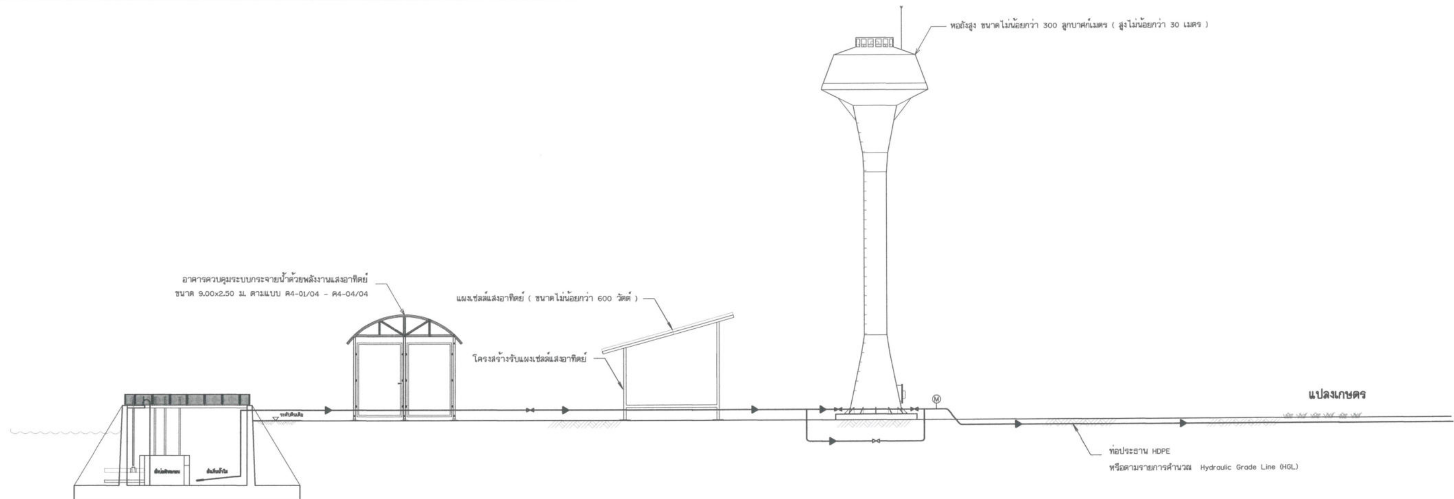
รูปด้านแผนผังระบบกระจายน้ำด้วยพลังงานแสงอาทิตย์ ขนาดไม่น้อยกว่า 75 กิโลวัตต์ (แบบก่อสร้างหอถังสูง)
