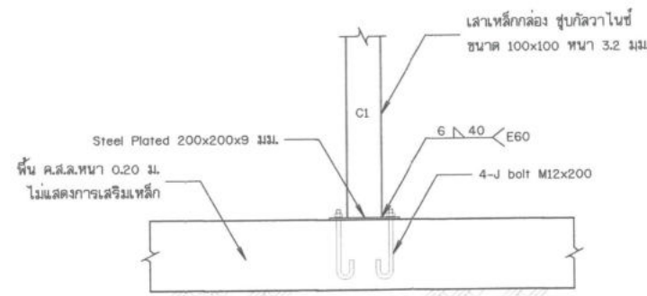
รูปขยายฐานรากโครงสร้างรับแผง C1
