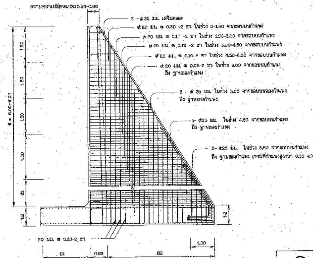
รูปตัด 5-ก (ด้านติดดิน)
