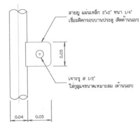
แบบขยายสายยู
