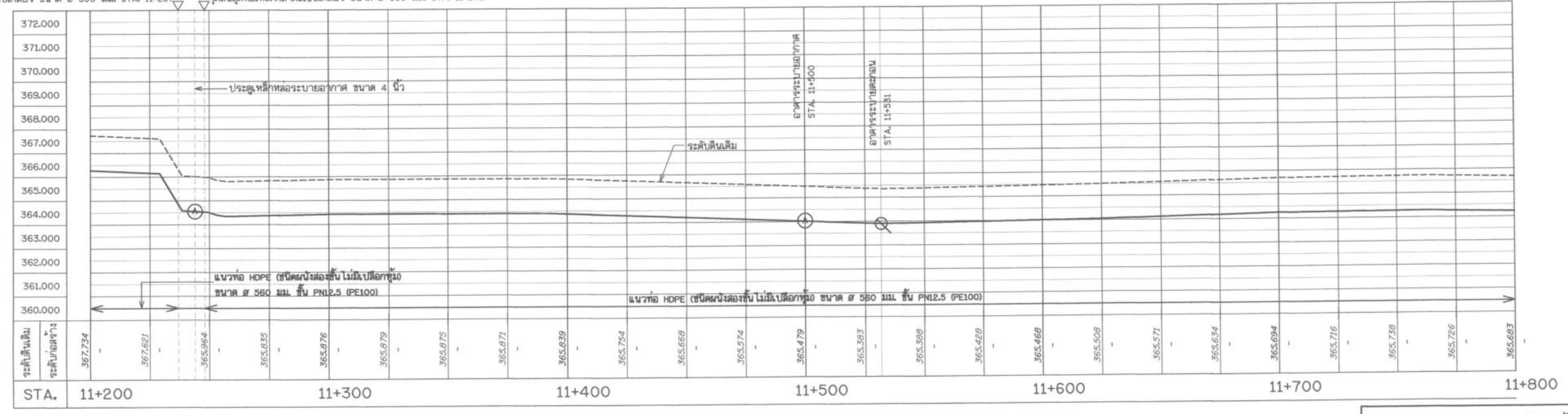
รูปตัดตามแนวยาว สาย LMP STA. 11+200 - 11+800
