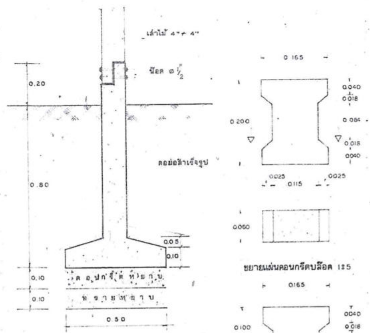
รูปขยายคอเมื่อ 1:10
