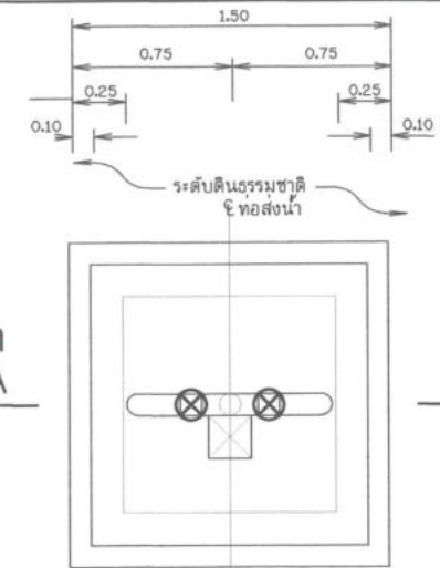
แปลนอาคารจุดปล่อยน้ำ 2 ด้าน
