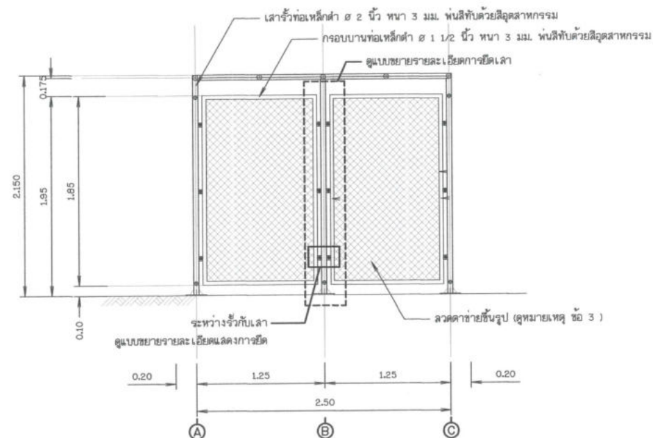
แบบขยายรั้ว 2
