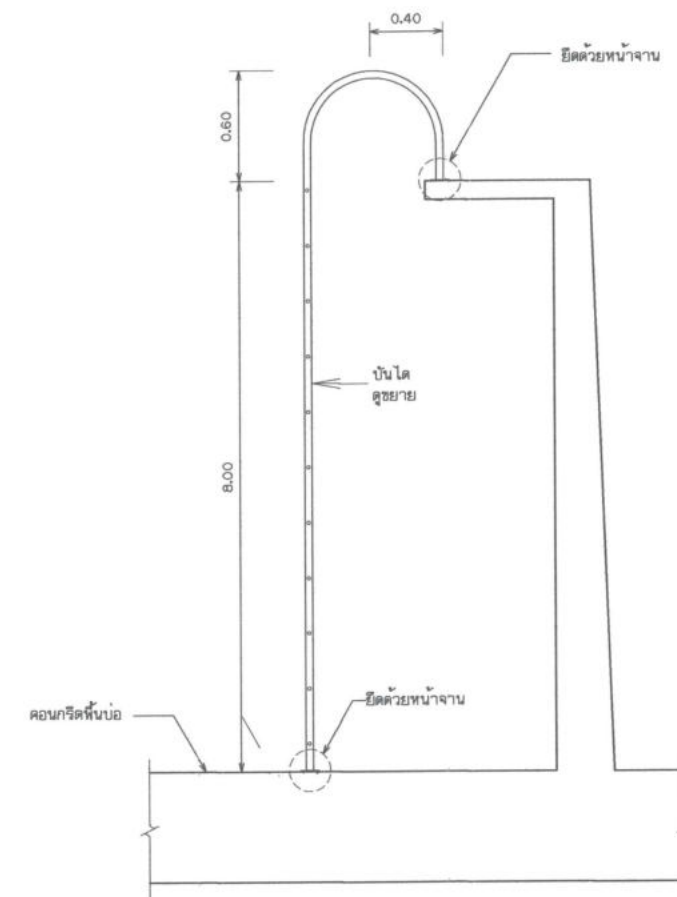
บันไดเหล็ก ไม่แสดงขนาดบางส่วน
