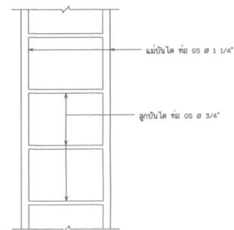
ขยายบันไดเหล็ก ไม่แสดงขนาดบางส่วน
