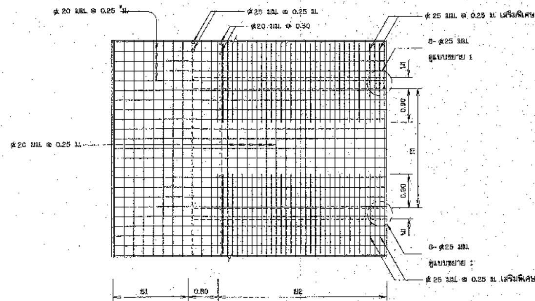
รูปตัด 4-ก (พื้นด้านบน)
