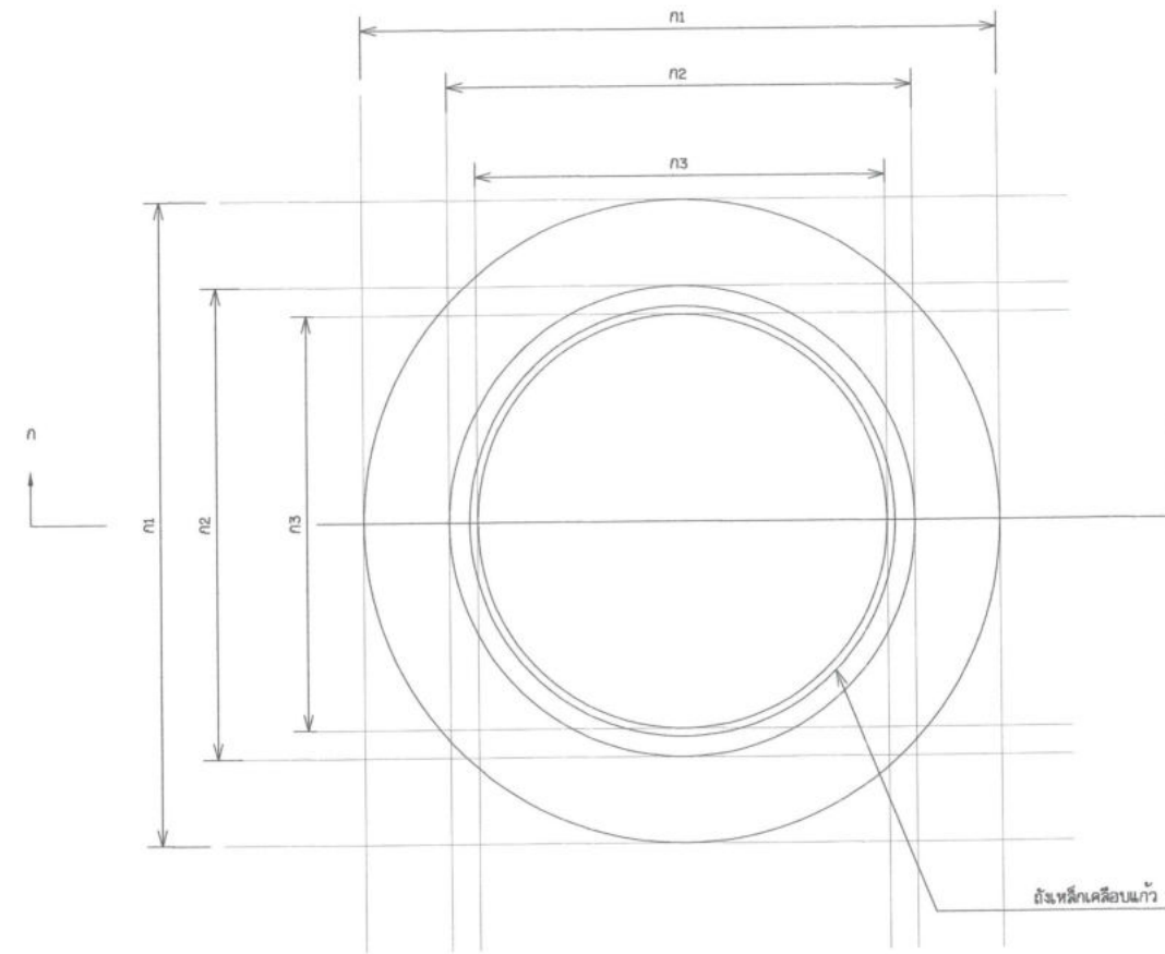
แปลนฐานรับถังเก็บน้ำ Fusion Bonded Epoxy (FBE) มาตราส่วน 1:100
