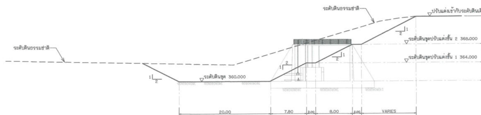
รูปตัดงานดิน
