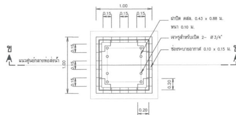
แปลนอาคารท่อระบายอากาศ
