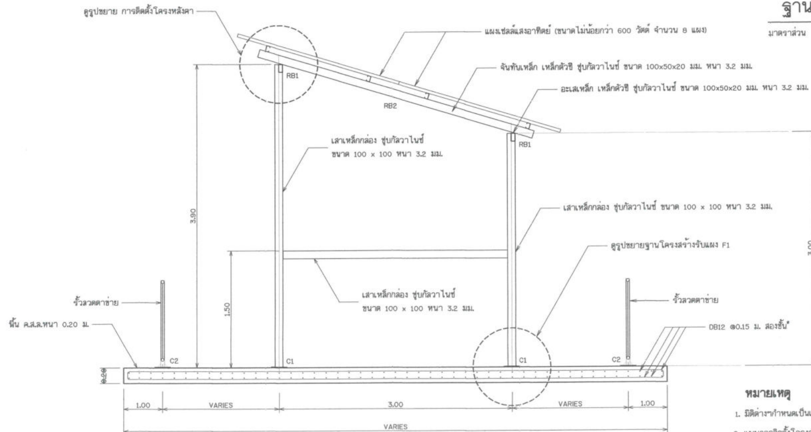
รูปด้านข้าง
