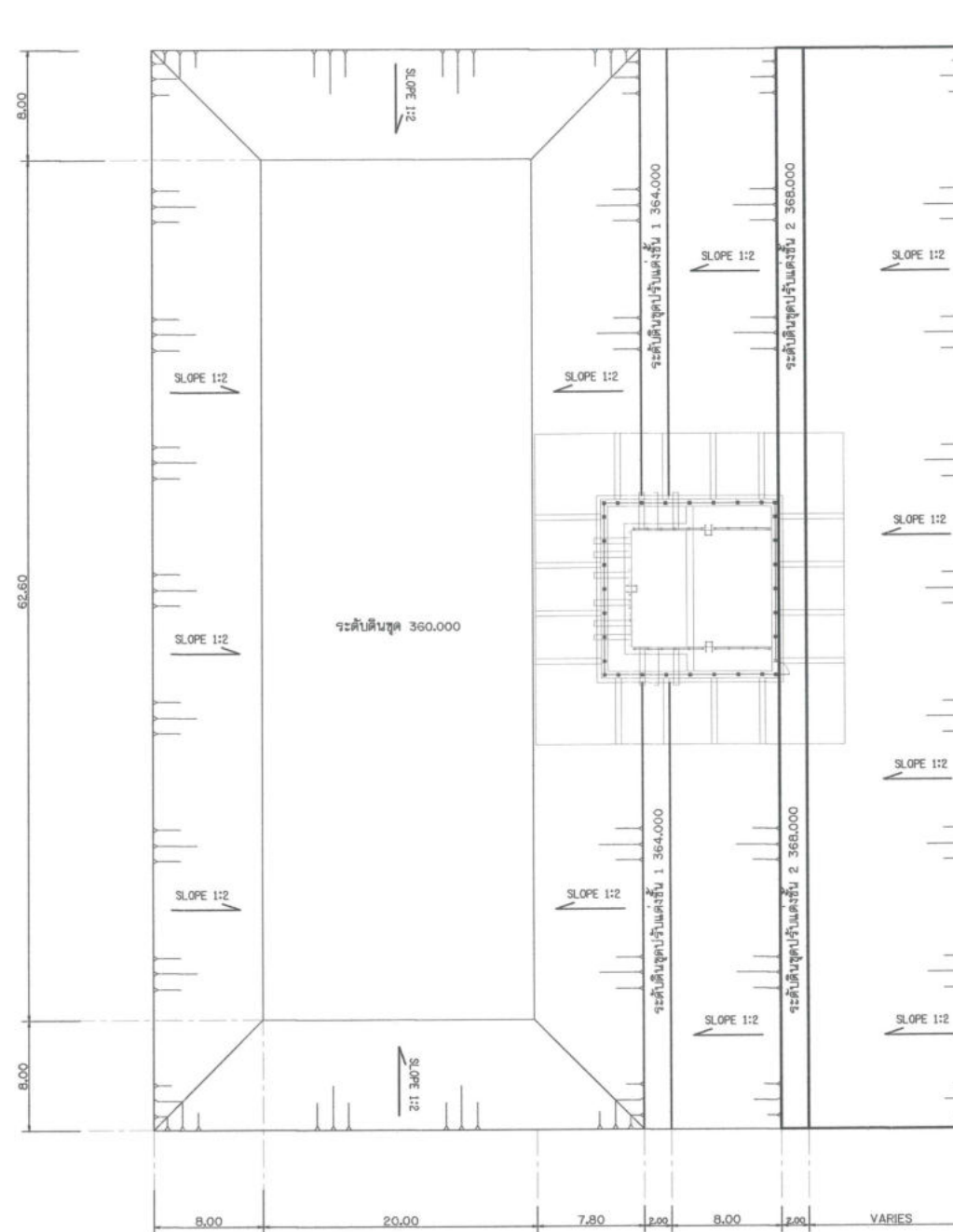
แปลนงานดินชุดบ่อสูบน้ำ คสล.
