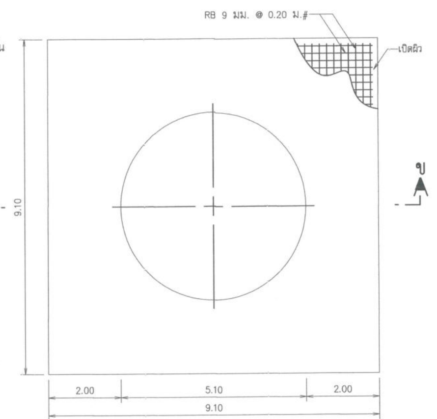
แปลนพื้นคอนกรีตเสริมเหล็ก ไม่แสดงมาตราส่วน
