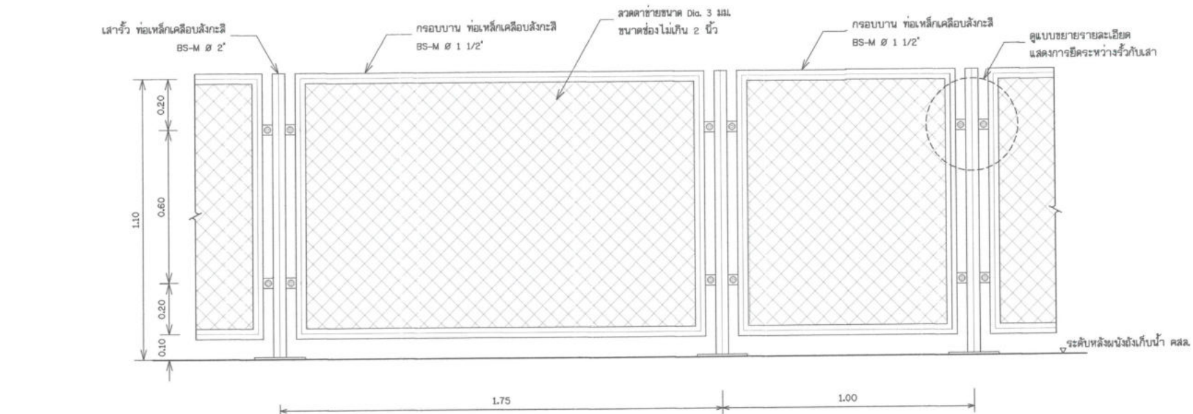
แบบขยายราวกันตก
