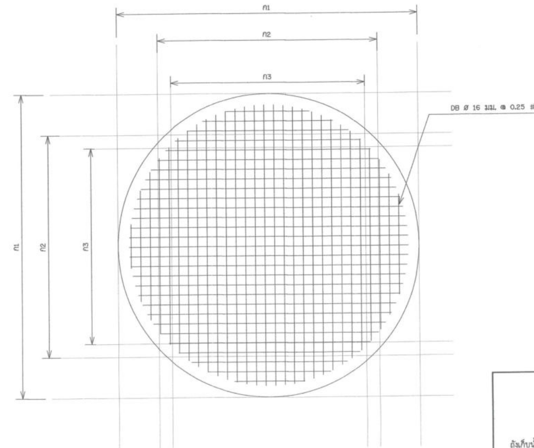
แปลนฐานรับถังเก็บน้ำ Fusion Bonded Epoxy (FBE) มาตราส่วน 1:100
