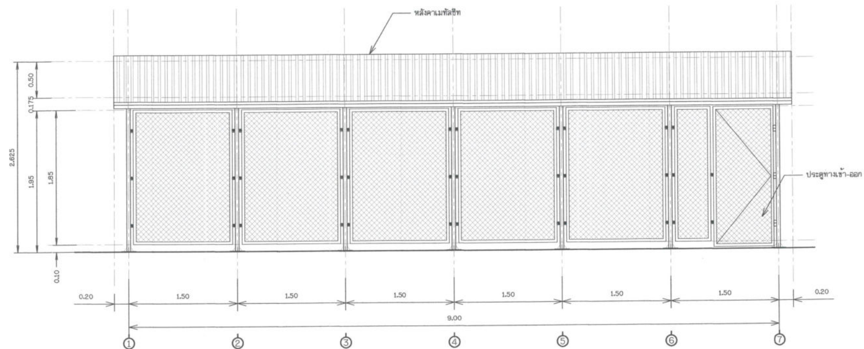
รูปด้าน 1
