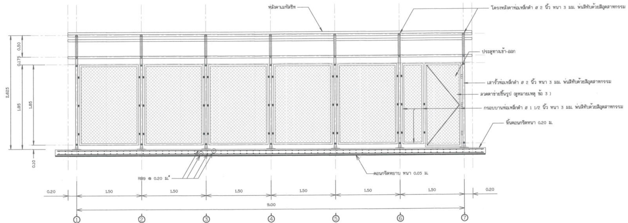
รูปตัด ก - ก
