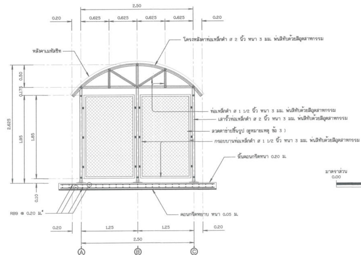
รูปตัด ข - ข
