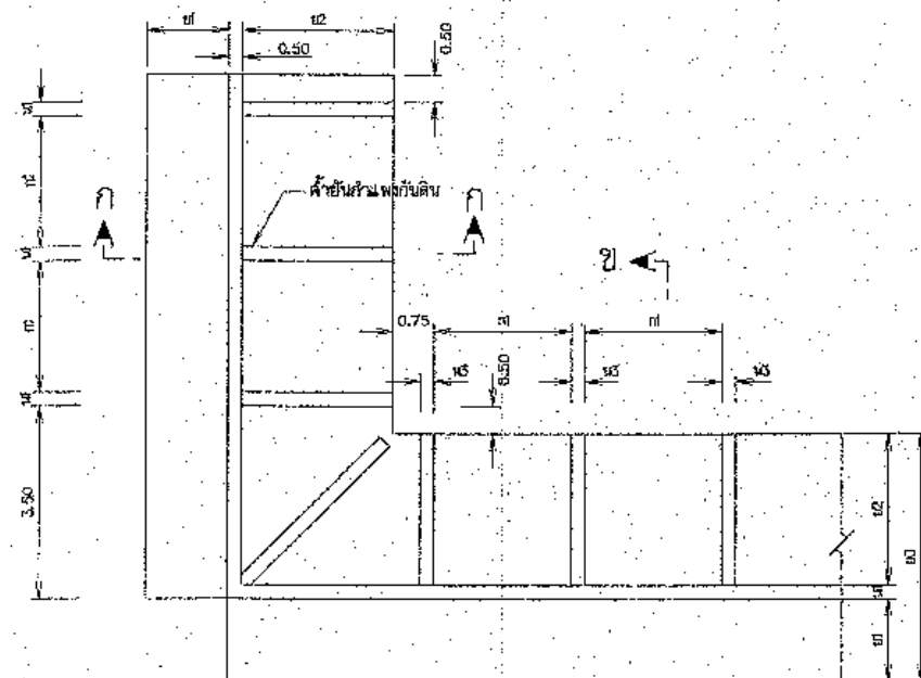
แปลน ไม่แสดงมาตราส่วน
