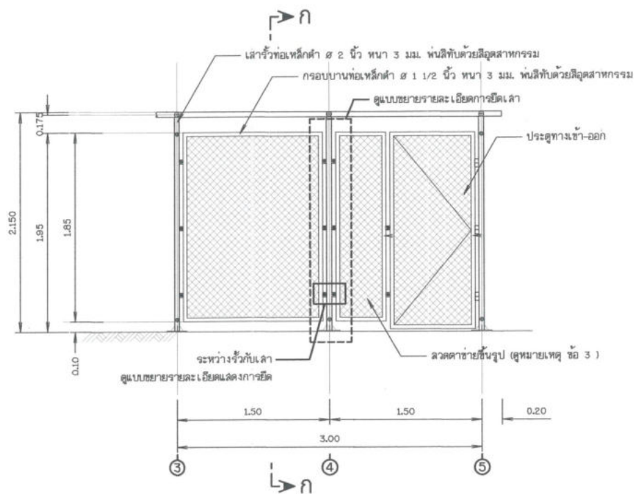
แบบขยายรั้ว 1
