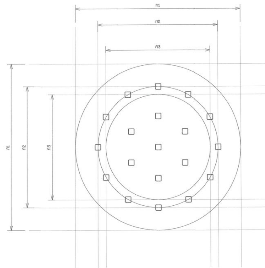
แปลนเสาเข็ม ถังเก็บน้ำ Fusion Bonded Epoxy (FBE) ขนาด 300 ลบ.ม. มาตราส่วน 1:100
