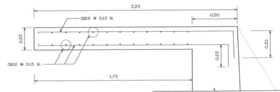
รูปขยายเหล็กเสริม 2
