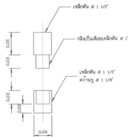
แบบขยายบานพับเหล็ก
