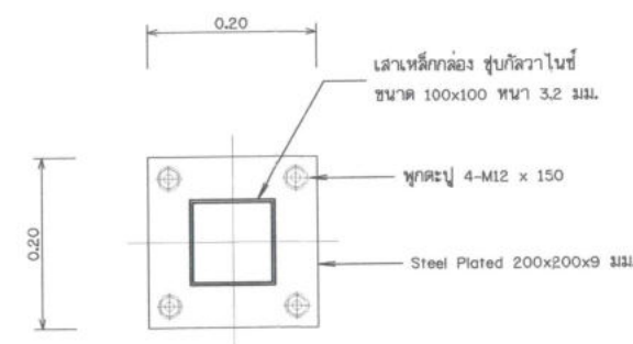
ฐานรากโครงสร้างเสา C1
