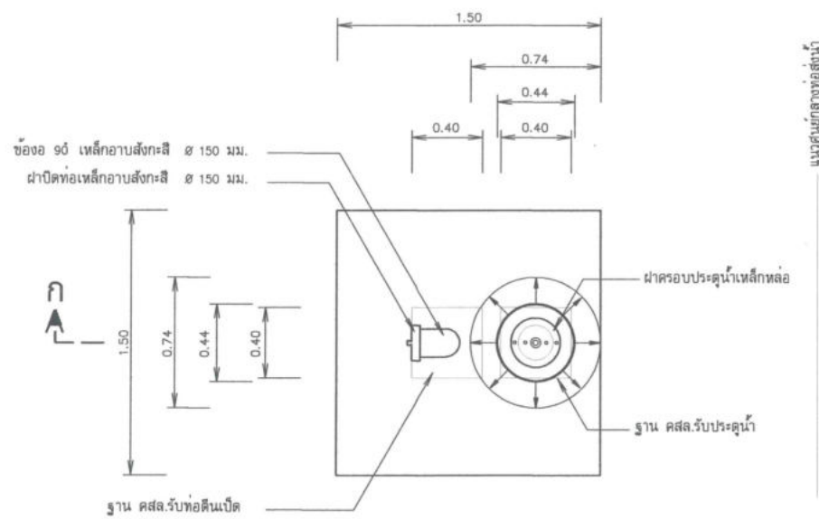
แปลนอาคารประตูปะบายตะกอน
