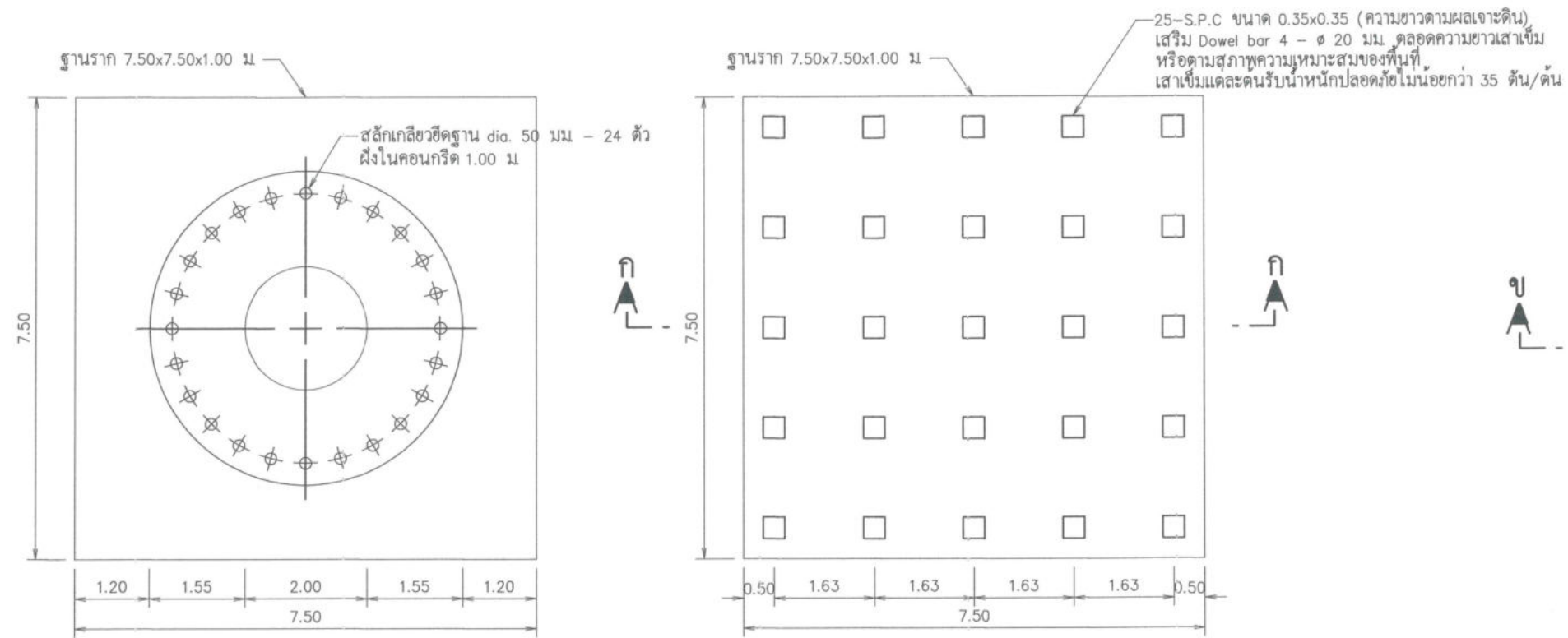
แปลนฐานรากหอดังสูง (แบบเสาเข็ม) ไม่แสดงมาตราส่วน
