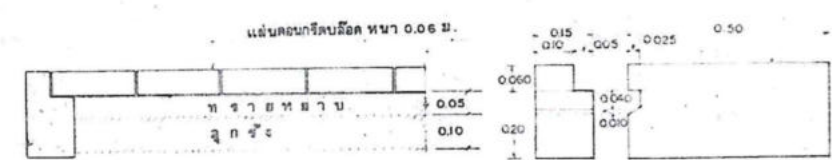
ขยายคันท่อนก 1:10
