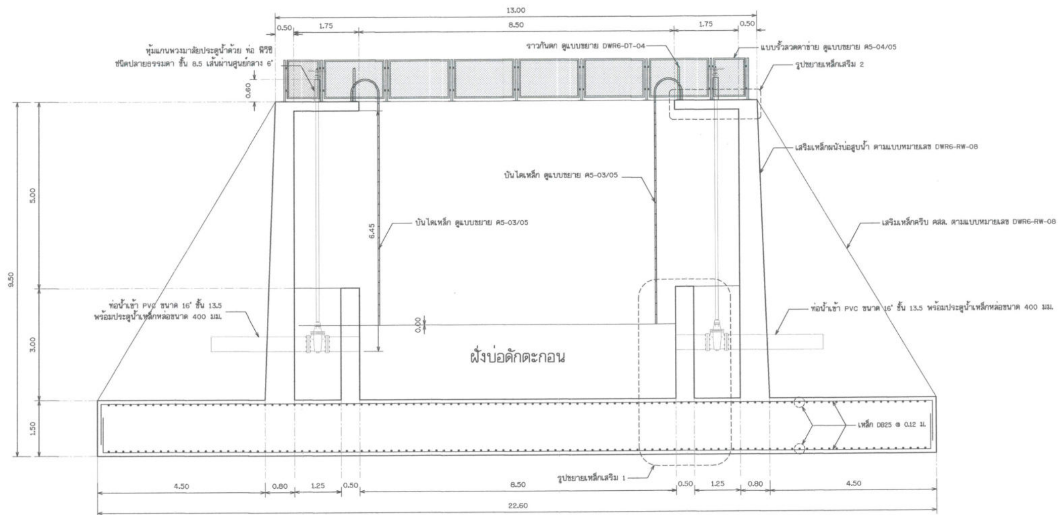
รูปตัด ก - ก
