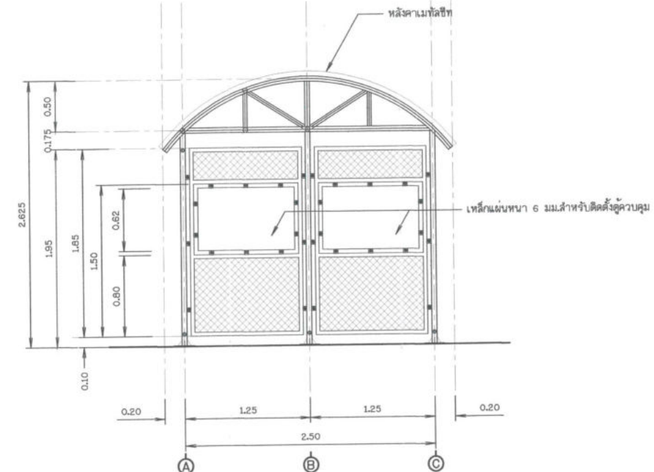
รูปด้าน 2
