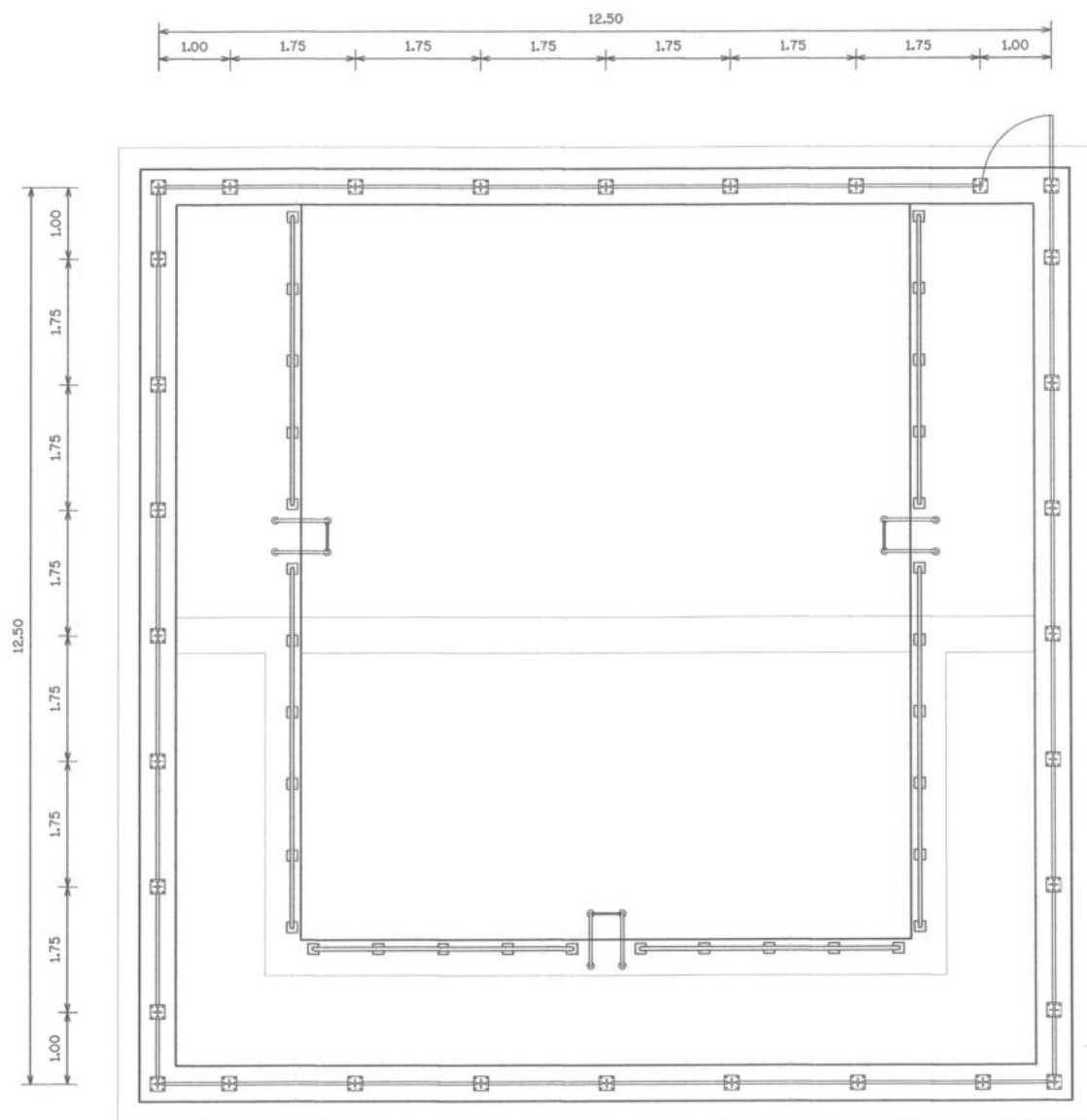
แบบแปลนรั้วลวดตาข่าย (บ่อสูบน้ำ คสล.)
