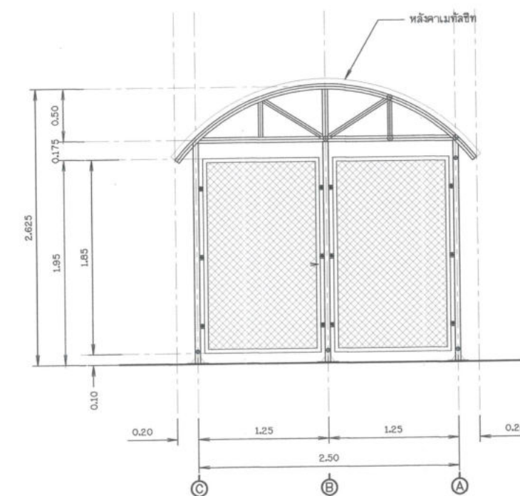
รูปด้าน 4
