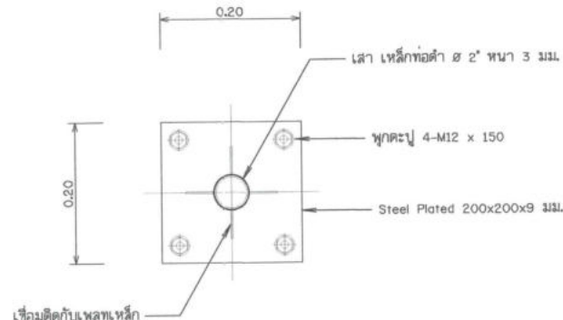
ฐานรากโครงสร้างเสาหัว C2
