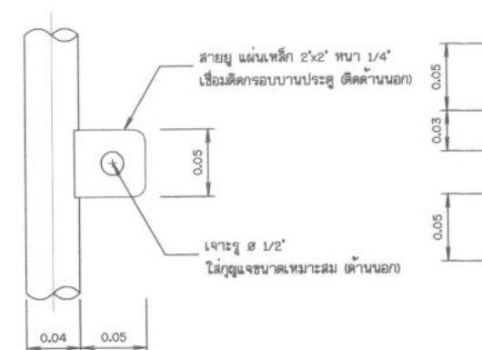
แบบขยายสายยู่
