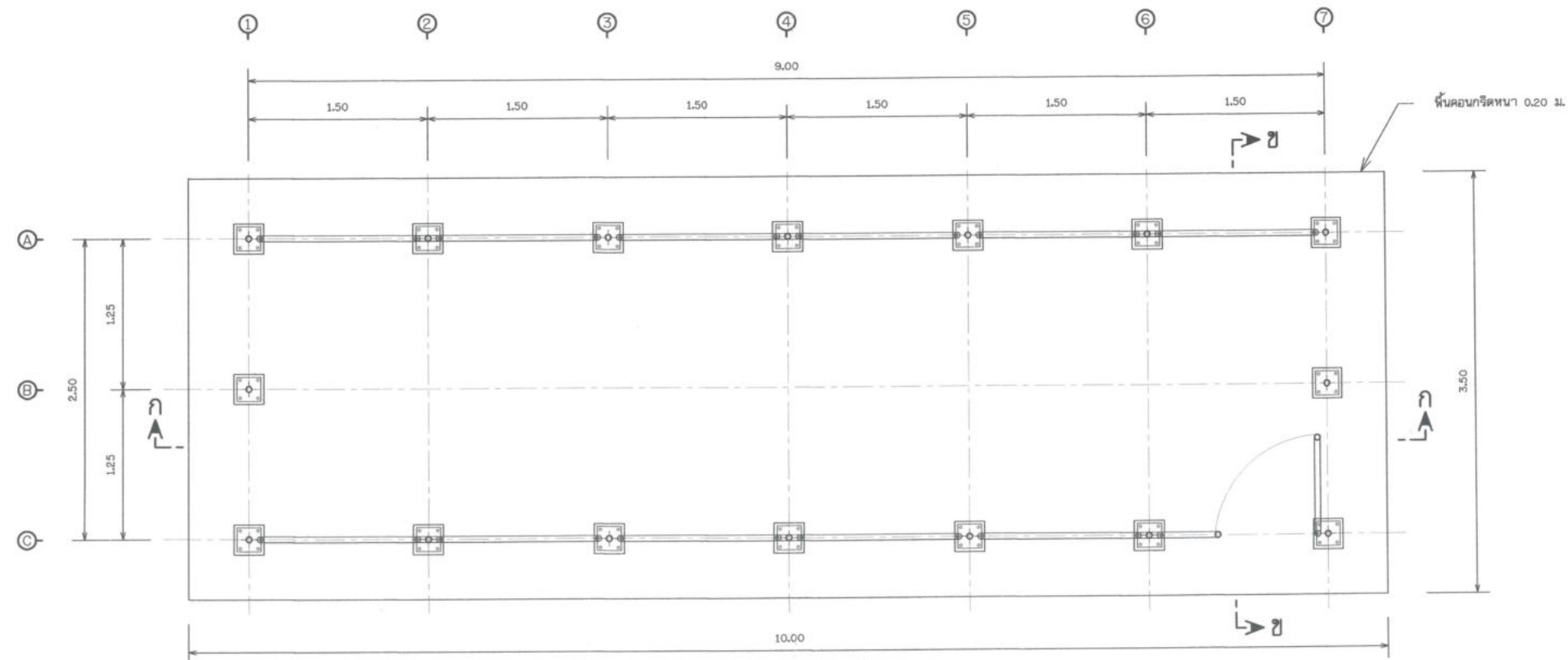
แปลนเสาและรั้ว
