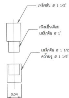
แบบขยายบานพับปีกเหล็ก
