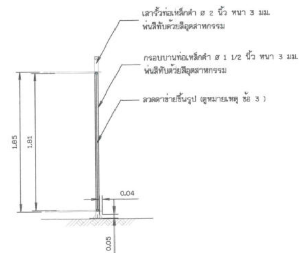
รูปตัด ก - ก
