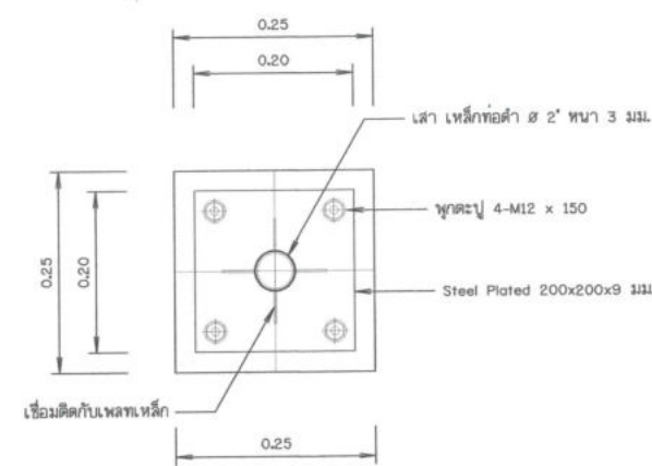
ฐานรากโครงสร้างอาคารคลุม
