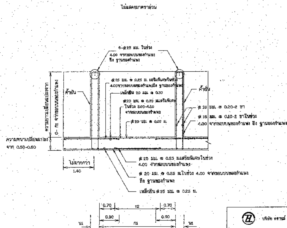
รูปตัด 4-ก (พื้นคานล่าง)
