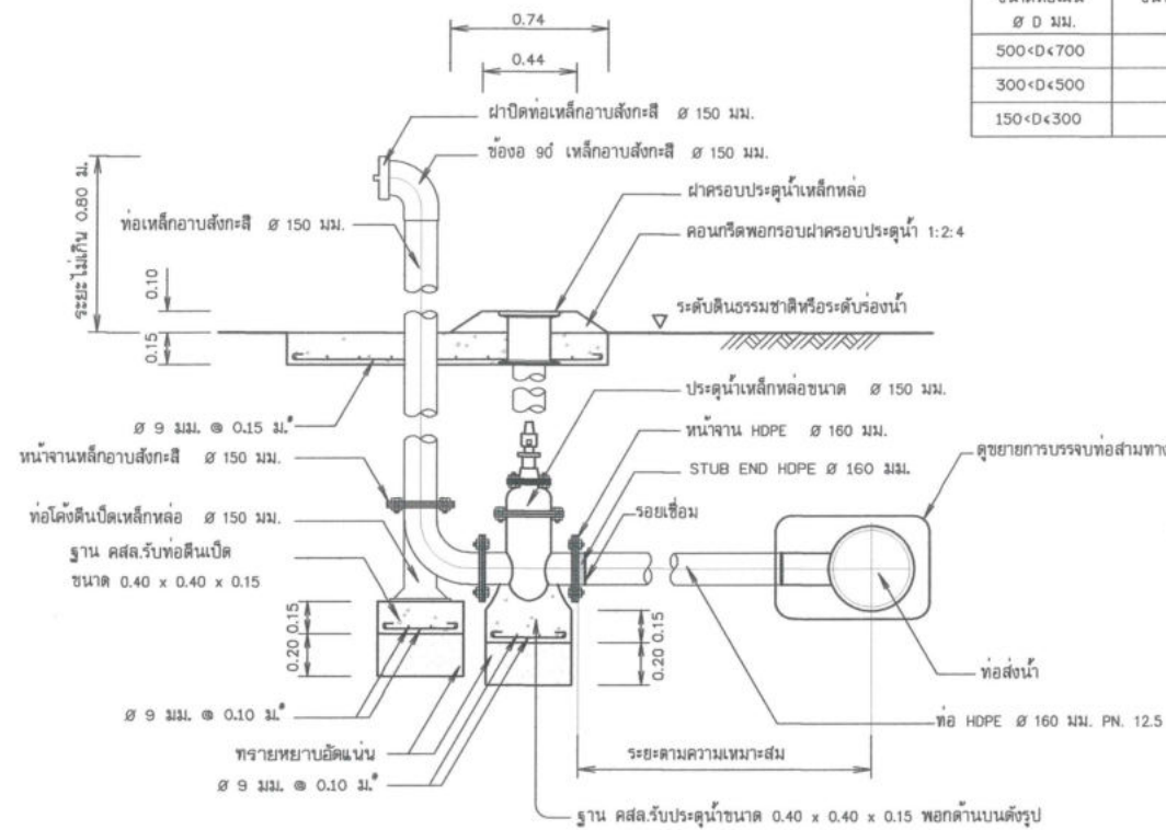
รูปตัด ก - ก แสดงการติดตั้งประตูปะบายตะกอน
