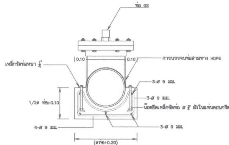
รูปตัดอากาศท่อระบายอากาศ Ø 50 มม. (ใช้สำหรับท่อส่งน้ำที่มีขนาดไม่เกินกว่า 150 มม.) มาตราส่วน 1:20
