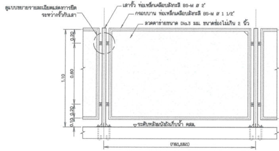
แบบขยายราวกันตก
