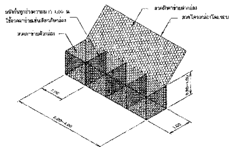
กล่องวัดคานาแบบ GABION
