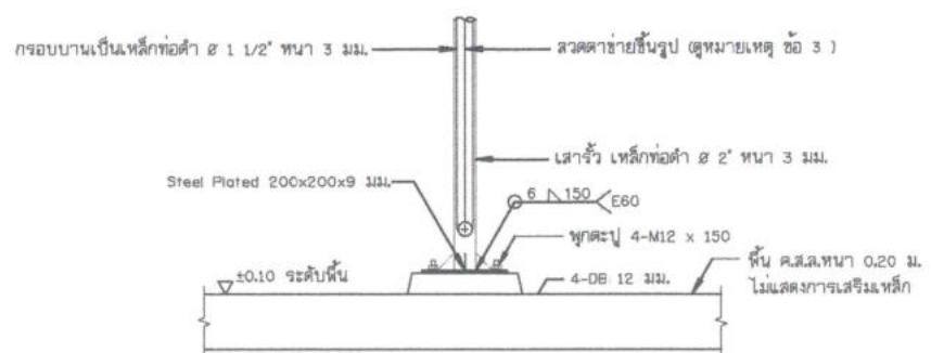
แบบขยายรายละเอียดแสดงการยึด ไม่แสดงขนาดราส่วน
