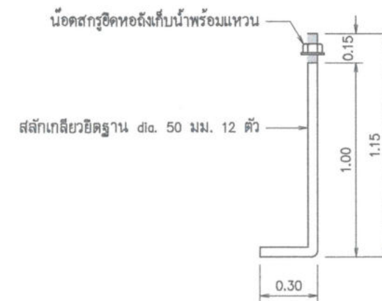
แบบขยายสลักเกลียวยึดฐาน ไม่แสดงมาตราส่วน
