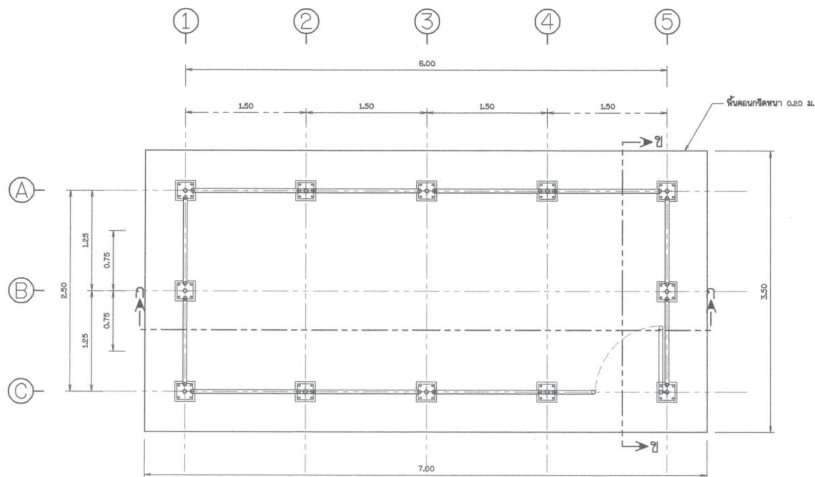
แปลนเสาและรั้ว โรงแสดงขนาดจริง
