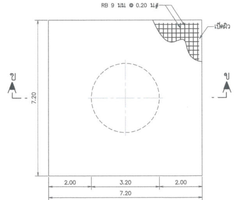
แปลนพื้นคอนกรีตเสริมเหล็ก ไม่แสดงมาตราส่วน
