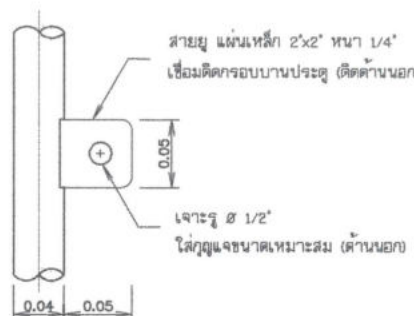
แบบขยายสายยู
