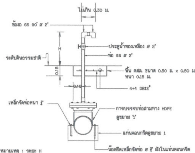
รูปตัดอากาศท่อระบายอากาศ Ø 50 มม. (ใช้สำหรับท่อส่งน้ำที่มีขนาดไม่เกินกว่า 150 มม.) มาตราส่วน 1:20
