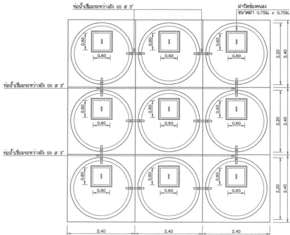
แปลนแบบ ๙ ถัง มาตราส่วน 1:40
