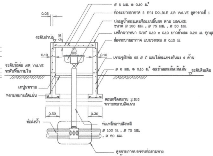
รูปตัด ข - ข แสดงการติดตั้งท่อระบายอากาศ
