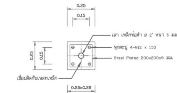
ฐานรากโครงสร้างอาคารคลุม ไม่แสดงขนาดราส่วน
