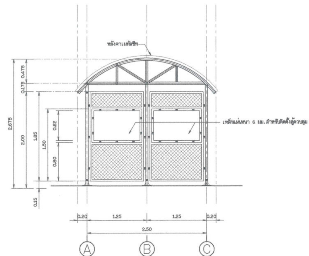
รูปด้าน 2 ไม่แสดงขนาดตัวหนังสือ
