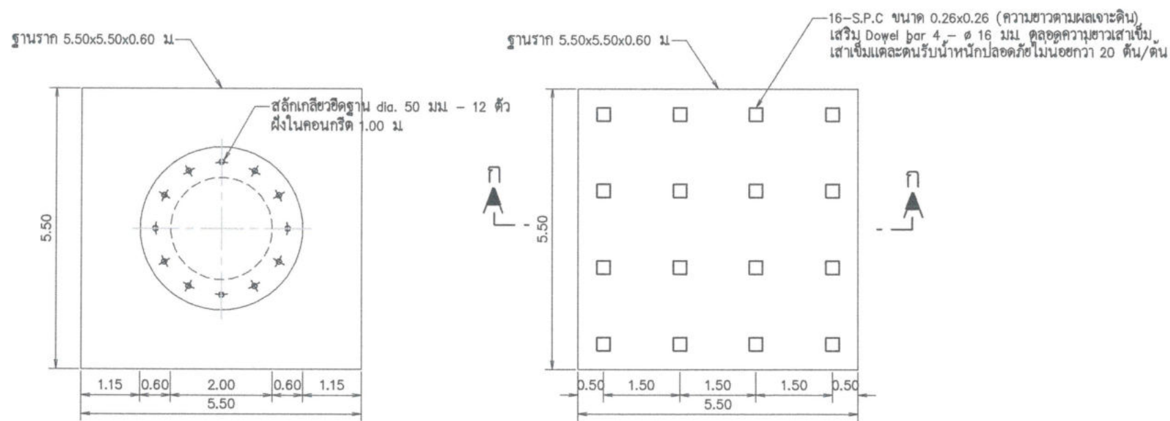
แปลนฐานรากหอดังสูง (แบบเสาเข็ม) ไม่แสดงมาตราส่วน
