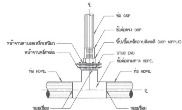
การบรรจุท่อสามทาง HDPE.
