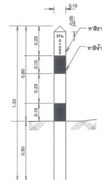
แสดงสัดส่วนหลักบอกแนวท่อ มาตราส่วน 1:10
