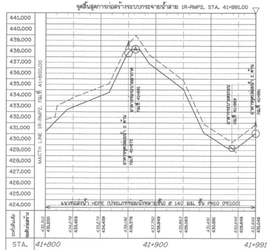
รูปตัดตามแนวยาว มาตราส่วน แนวตั้ง 1:500 แนวนอน 1:1,000
