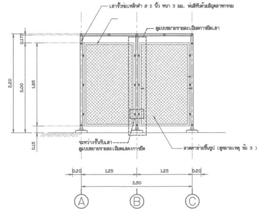
แบบขยายรั้ว 2 ไม่แสดงขนาดราส่วน
