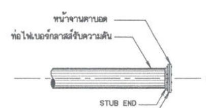
การปิดปลายท่อ
