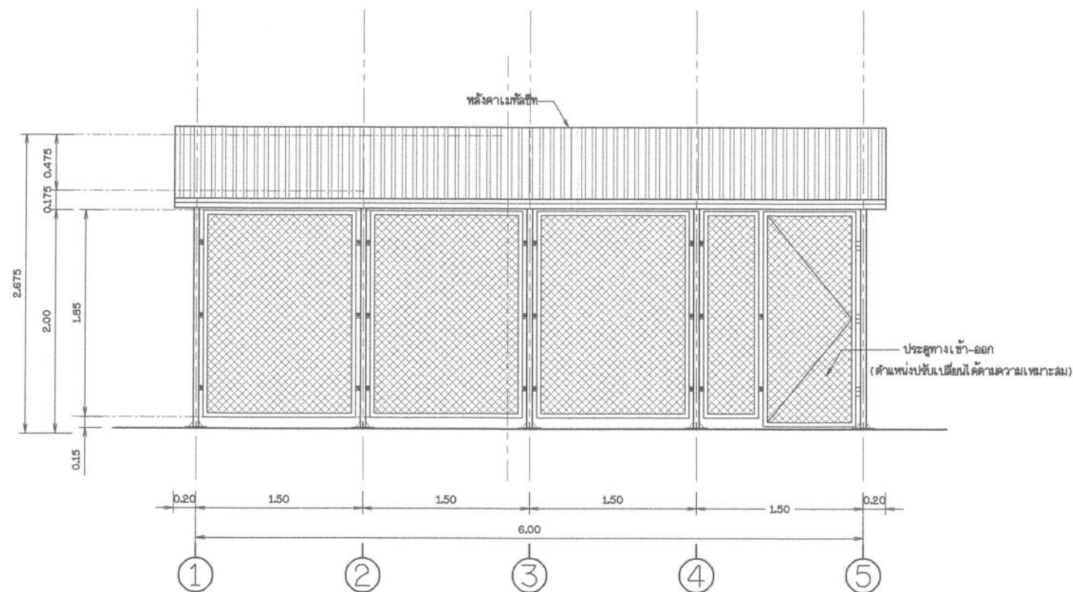
รูปด้าน 1 ไม่แสดงขนาดตัวหนังสือ
