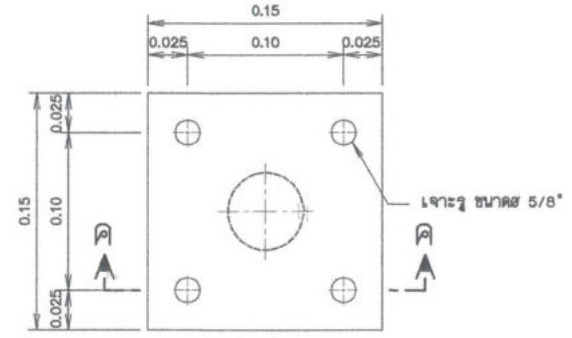
รูปขยายแผ่นเหล็กหน้าแปลน
