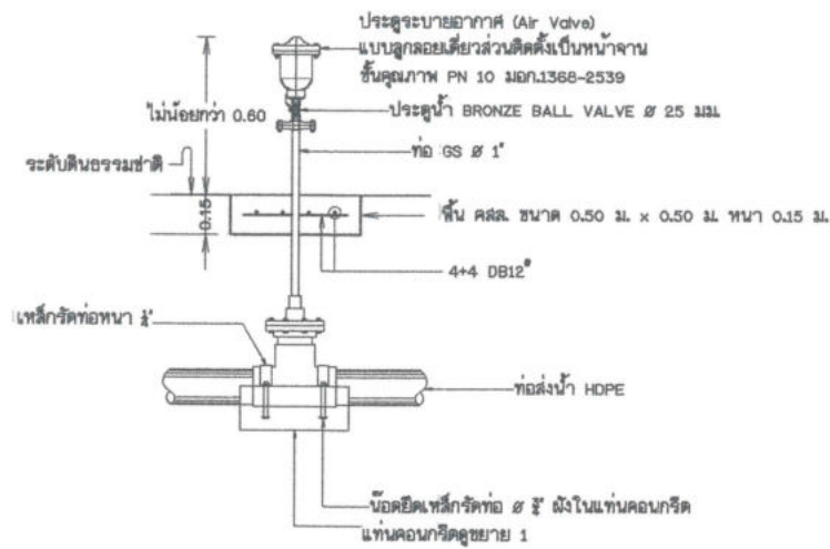
รูปตัดอากาศท่อระบายอากาศ Ø 25 มม. (ใช้สำหรับท่อส่งน้ำที่มีขนาดไม่เกินกว่า 150 มม.) มาตราส่วน 1:20
