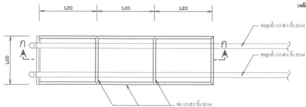
แปลนโครงสร้างรับท่อส่งน้ำ มาตราส่วน 1:25
