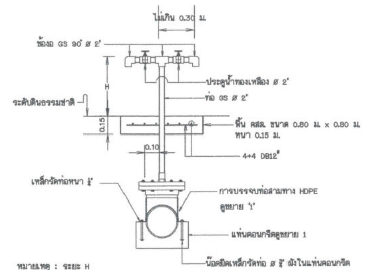
รูปตัดอากาศจุดปล่อยน้ำ 2 ด้าน (ใช้สำหรับท่อส่งน้ำที่มีขนาดไม่เกินกว่า 150 มม.) มาตราส่วน 1:20
