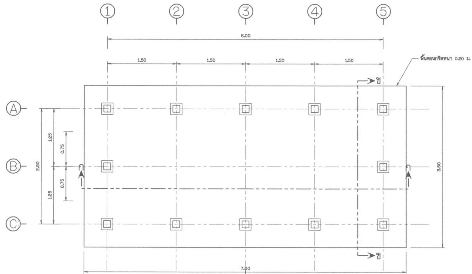
แบบแปลน โรงแสดงขนาดจริง
