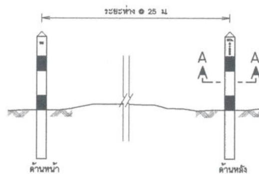
แสดงการวางหลักบอกแนวท่อ มาตราส่วน 1:20
