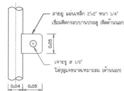
แบบขยายสายยู ไม่แสดงขนาดราส่วน
