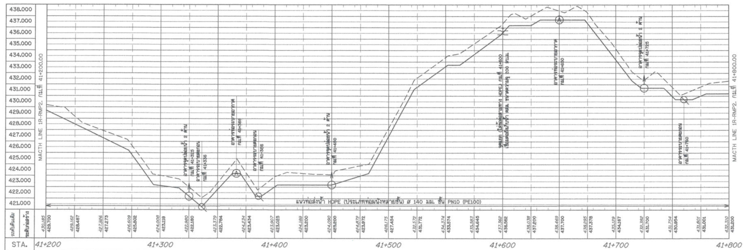
แผนระบบส่งน้ำ สาย 1R-RMP2. STA. 41+200 - 41+800 มาตราส่วน 1:1,000
