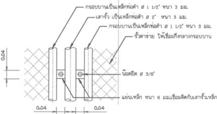
แบบขยายรายละเอียดแสดงการยึดระหว่างรั้วกับเสา ไม่แสดงขนาดราส่วน
