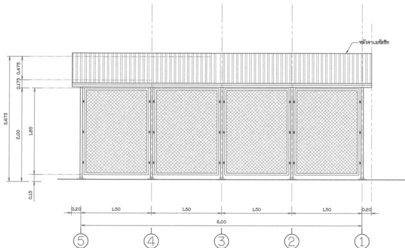
รูปด้าน 1 ไม่แสดงขนาดตัวหนังสือ
