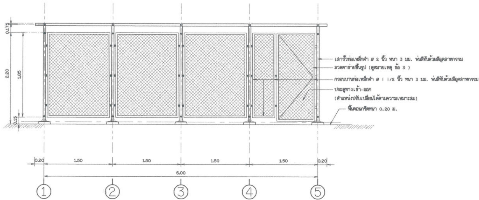
แบบขยายรั้ว 1 ไม่แสดงขนาดราส่วน
