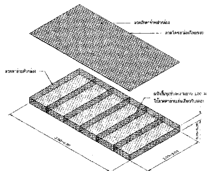
กล่องใส่ตุ๊กตาชายแบบ MATTRESS
