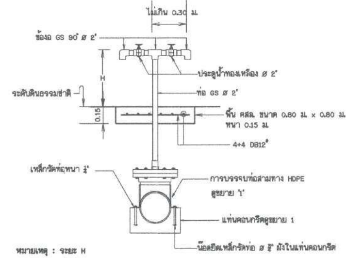
หมายเหตุ : ระยะ H H ไม่เกิน 0.60 ม. สำหรับจุดปล่อยน้ำ รูปตัดอาคารจุดปล่อยน้ำ 2 ด้าน มาตรฐาน 1:20
