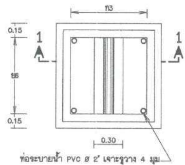
แปลนบ่อประตูปรับระดับน้ำ มาตรฐาน 1:20
