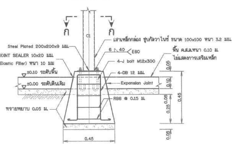
รูปขยายฐานรากโครงสร้างรับแผง F1 (ต่อมอด คลส หล่อสำเร็จรูปพร้อมติดตั้ง) ไม่แสดงมาตราส่วน
