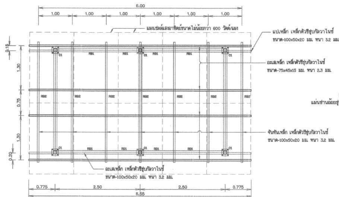
แปลนฐานรากและโครงหลังคารับแผง จำนวน 10 แผง ไม่แสดงมาตราส่วน
