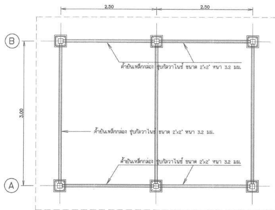
รูปแสดงค้ำยันโครงสร้างรับแผง ชั้น 1 ไม่แสดงมาตราส่วน
