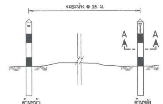
แสดงการวางหลักบ่อแก๊ส มาตรฐาน 1:20
