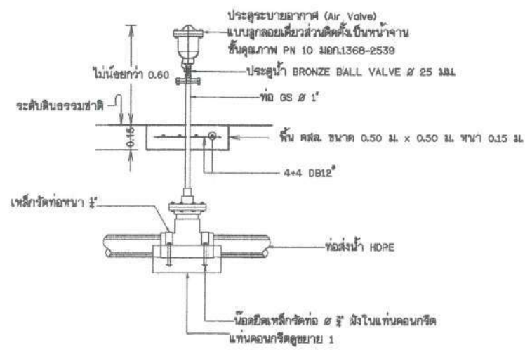
รูปตัดอาคารท่อระบายอากาศ Ø 25 มม. (ใช้สำหรับท่อส่งน้ำที่มีขนาดไม่เกิน 6 นิ้ว) มาตรฐาน 1:20
