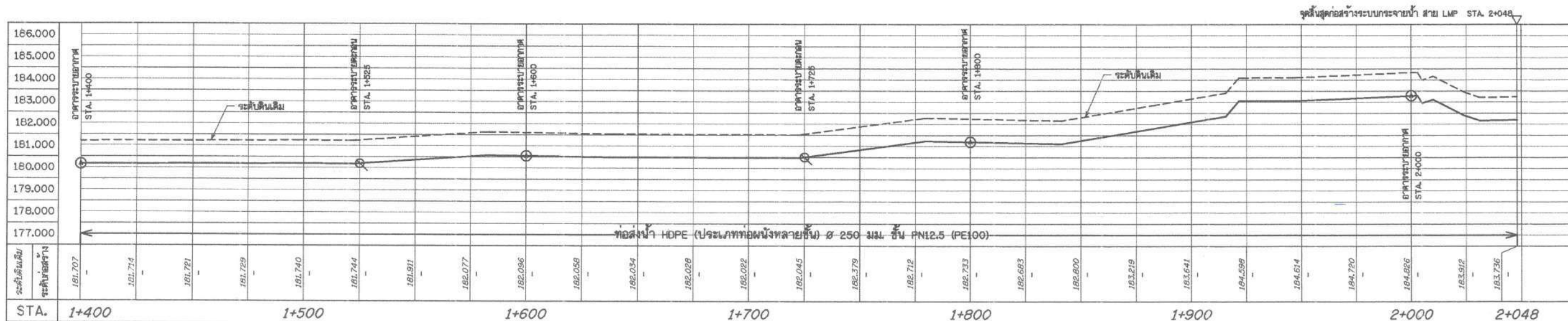
รูปตัดตามแนวยาวระบบกระจายน้ำ สาย LMP มาตราส่วน 1:1,000
