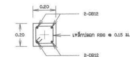
รูปตัด A-A (C1)
