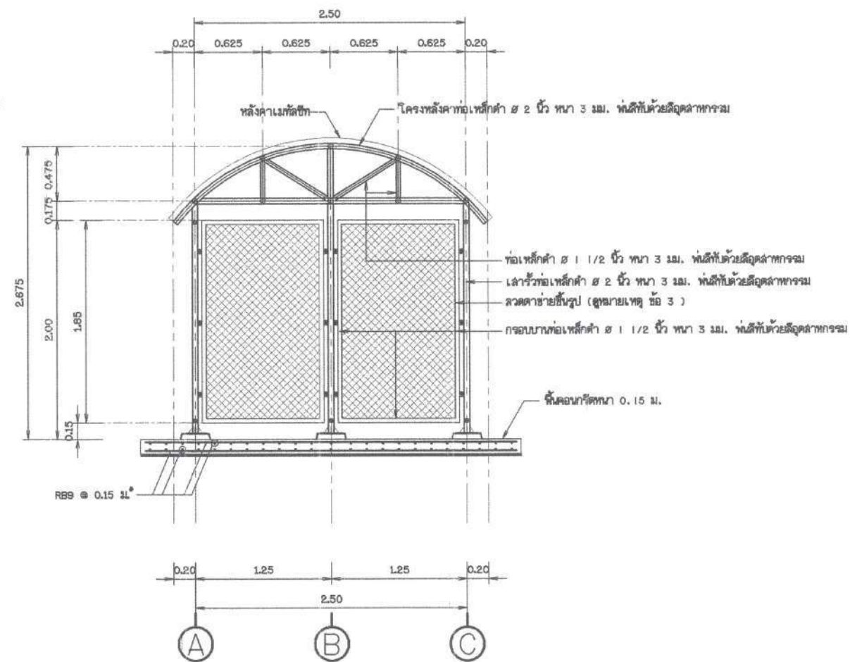
รูปตัด ข - ข ไม้คดงมดจาด่วน
