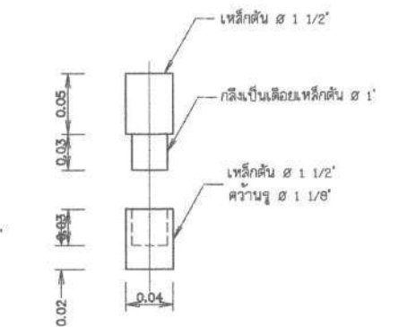
แบบขยายบานพับหัวเหล็ก
