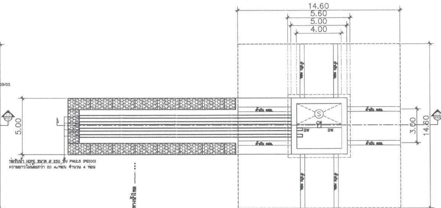
แปลนแสดงโครงสร้างคานและพื้นสำหรับบ่อสูบน้ำ
