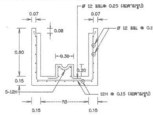
เหล็กเสริมบ่อประตูปรับระดับน้ำ มาตรฐาน 1:20
