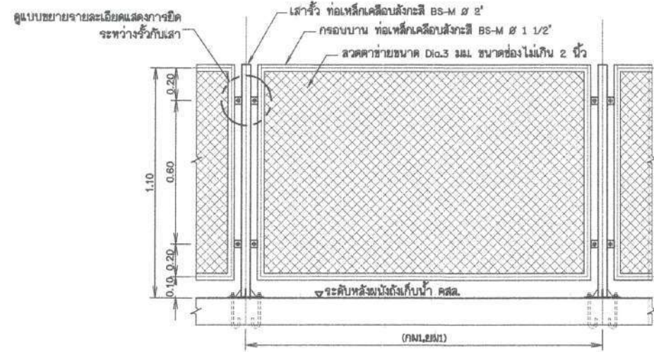
แบบขยายราวกันตก สำหรับบังน้ำ คสล. แบบไม่มีฝ้าปิด
