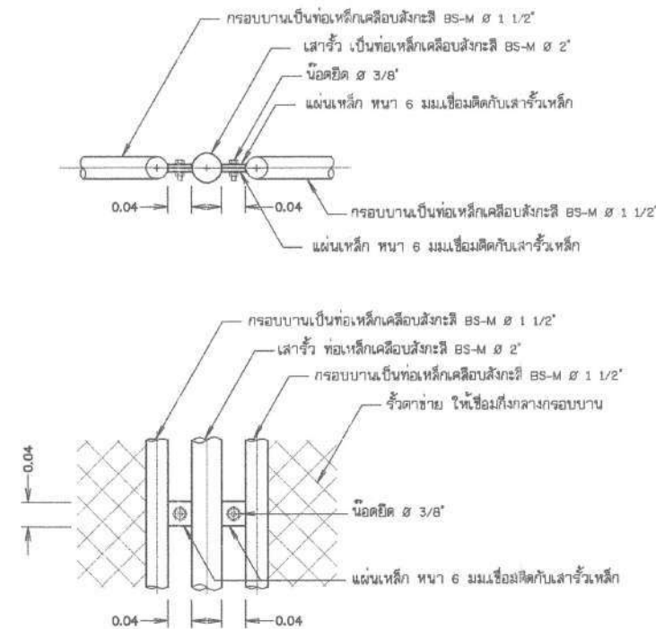
แบบขยายรายละเอียดแสดงการยึดระหว่างรูลกับเสา
