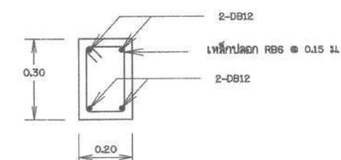
รูปตัด 1-1 (B2)
