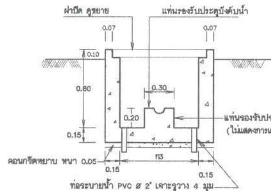
รูปตัด 1 - 1 มาตรฐาน 1:20
