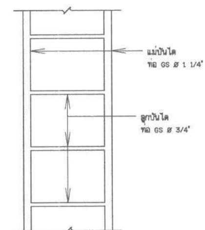
ขยายบันได
