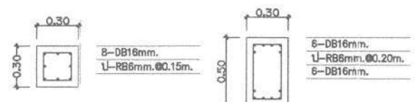
รูปตัดเสา CW
