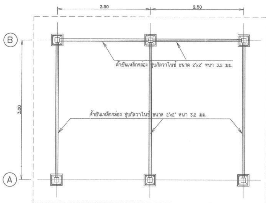
รูปแสดงค้ำยันโครงสร้างรับแผง ชั้น 2 ไม่แสดงมาตราส่วน
