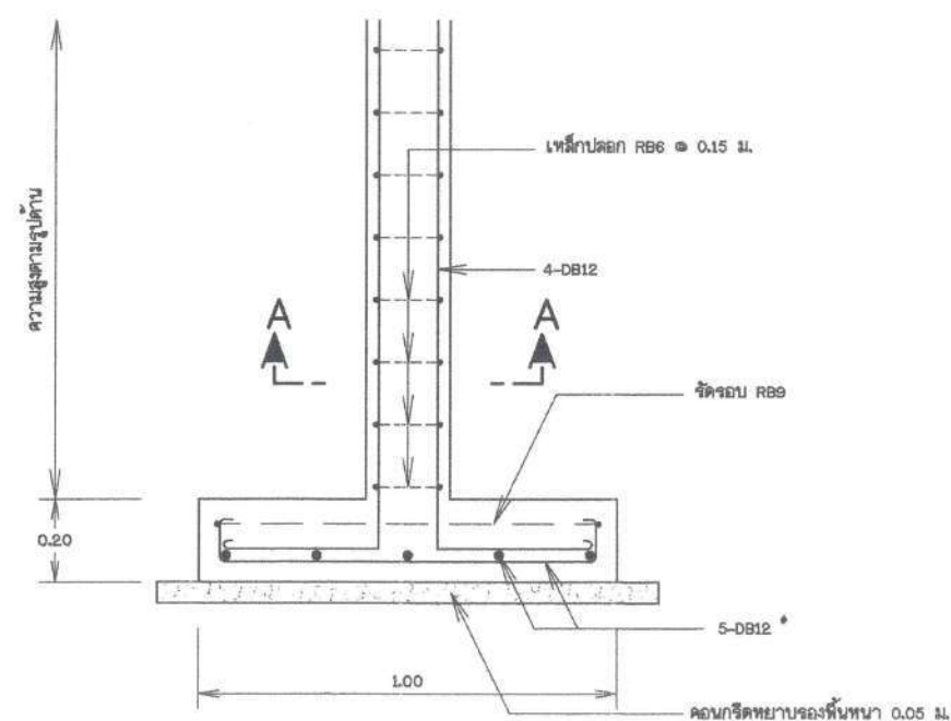
รูปตัดฐานราก F1
