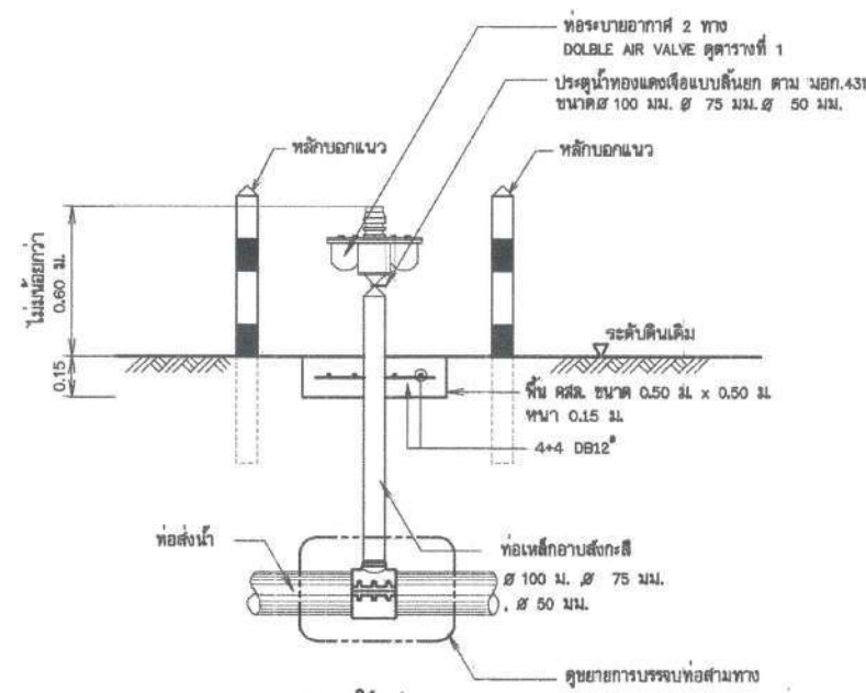
รูปแสดงการติดตั้งท่อระบายอากาศ มาตรฐาน 1:20
