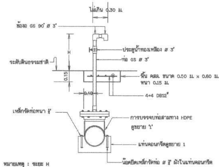
หมายเหตุ : ระยะ H H ไม่เกิน 0.60 ม. สำหรับประตูลอยตัว รูปตัดอาคารประตูลอยตัว Ø 75 มม. มาตรฐาน 1:20
