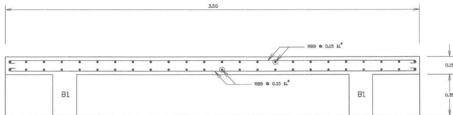
พื้น S1
