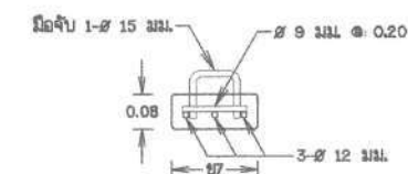
รูปตัดแนว 2 - 2 มาตรฐาน 1:10
