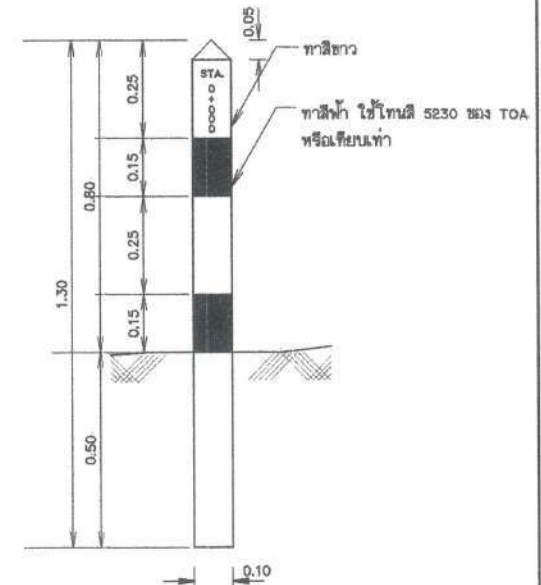
แสดงสัดส่วนหลักบ่อแก๊ส มาตรฐาน 1:10
