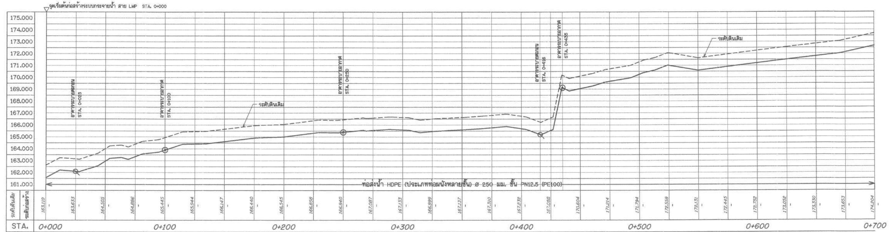
รูปตัดตามแนวาวระบบกระจายน้ำ สาย LMP
