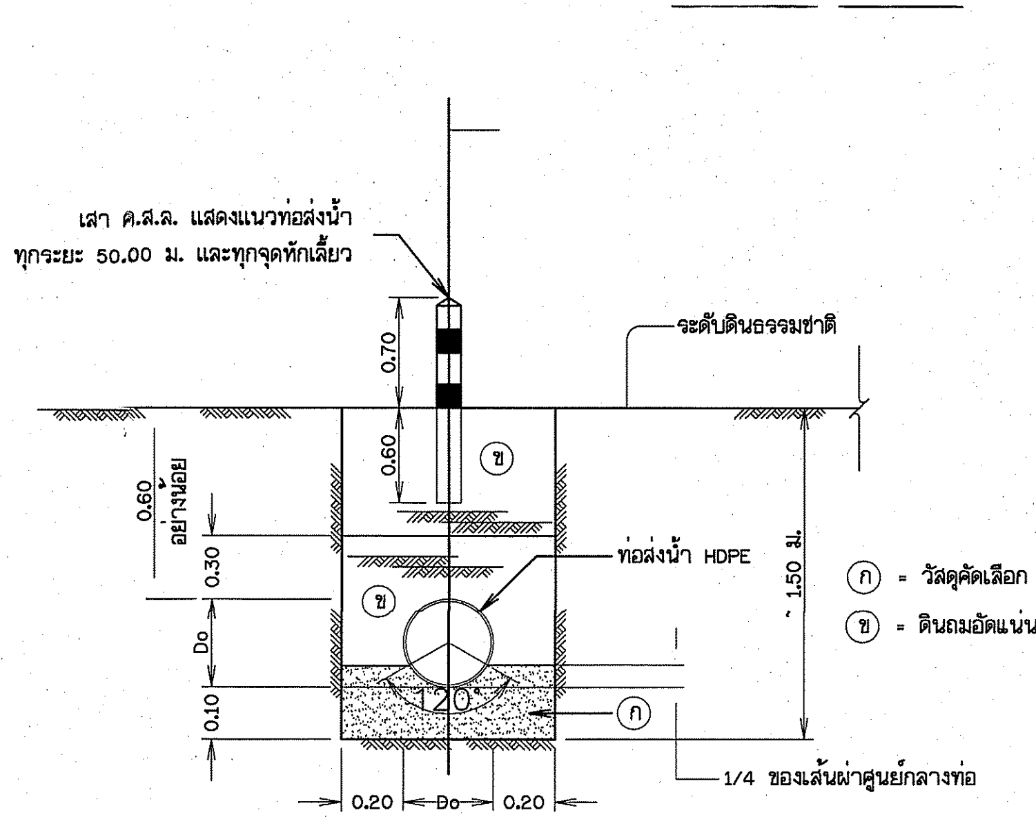
รูปตัดขวางการฝังท่อพีอี (ท่อHDPE)
