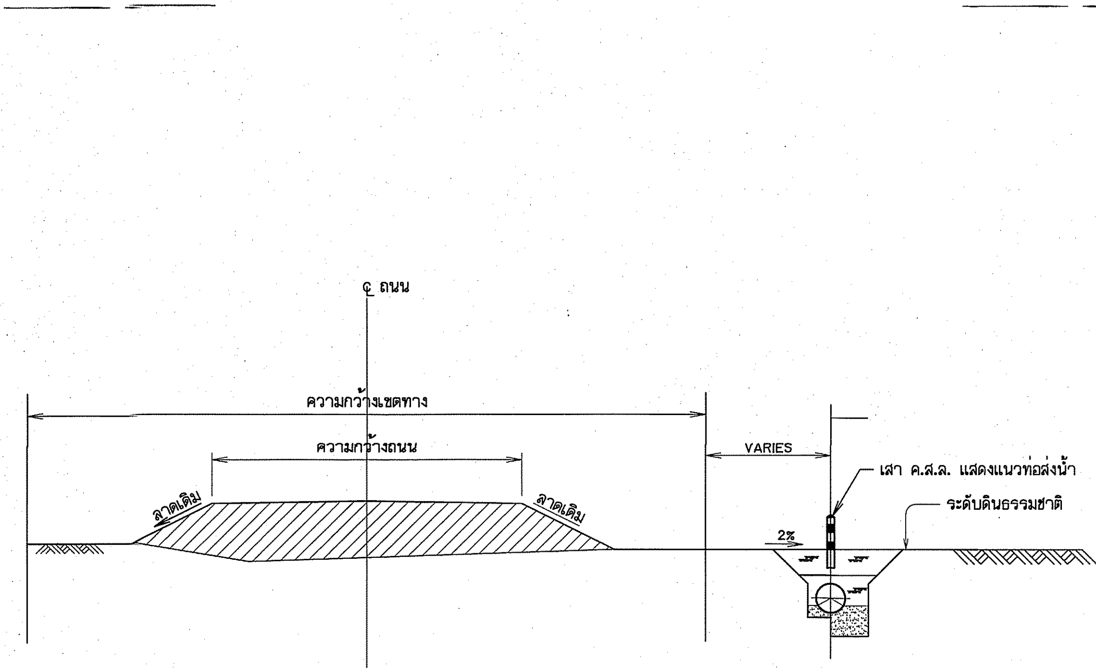
รูปตัดแสดงการวางท่อส่งน้ำ
