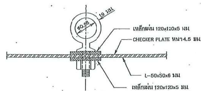
รูปขยายห่วงยึดแปะสูบน้ำ มาตราส่วน 1 : 5
