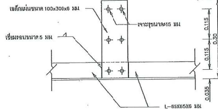
รูปด้านตั้ง (ไม่แสดงเหล็กฉาก)
