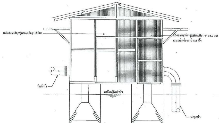
รูปด้าน 3
