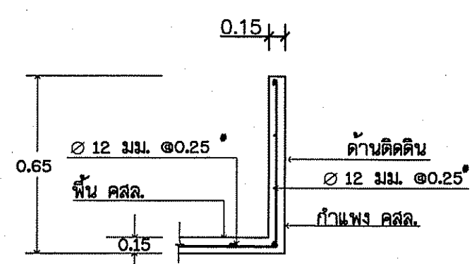
รูปตัด (ค-ค) (ความหนาพื้น 0.15 ม.) ไม่แสดงมาตราส่วน
