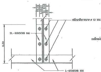
รูปด้านตั้ง
