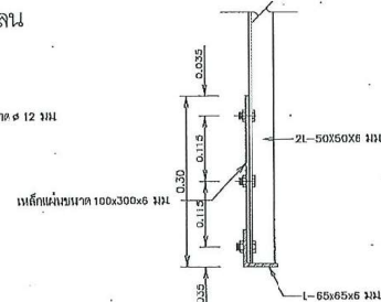
รูปตัด ข-ข
