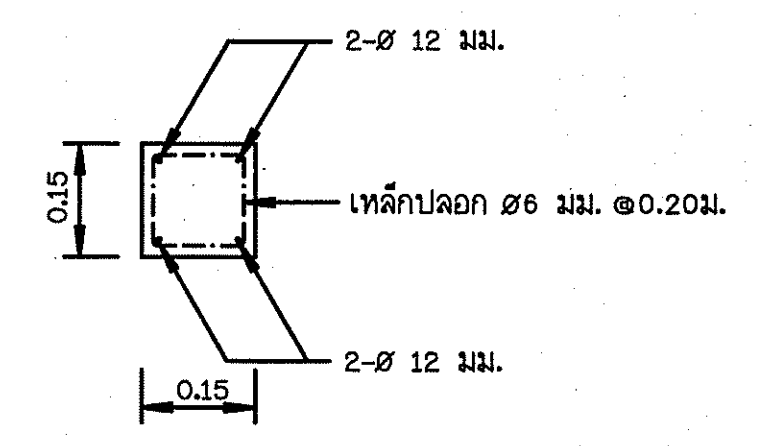
รูปตัด ก - ก มาตรฐาน 1:10
