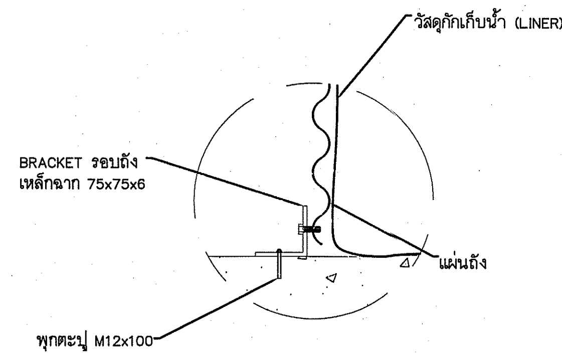
แบบขยาย 11-ติดตั้งผนังกับฐานจาก Scale NTC.
