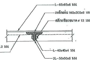
รูปตัด ค-ค
