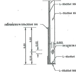
รูปตัด ง-ง
