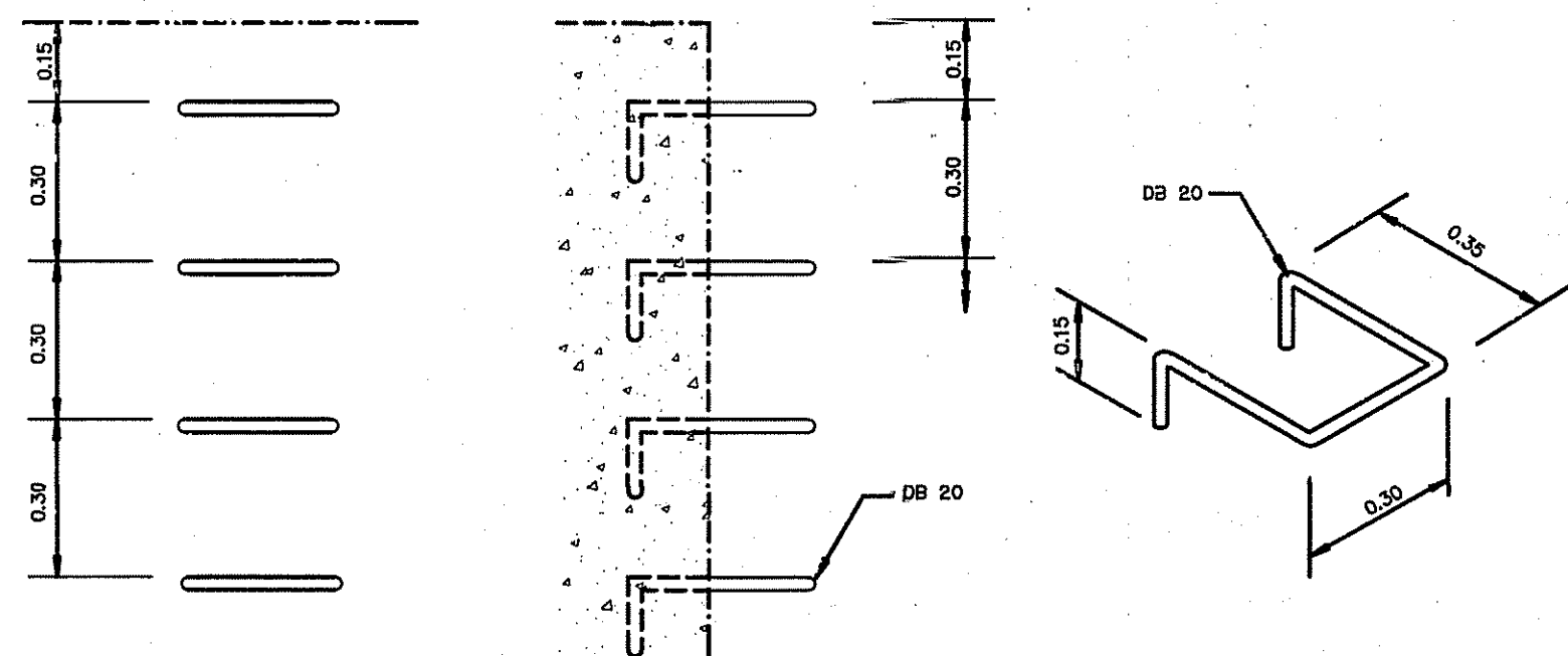
รูปขยายฐานรอง ไม่แสดงมาตราส่วน
