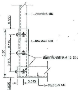
รูปด้านตั้ง
