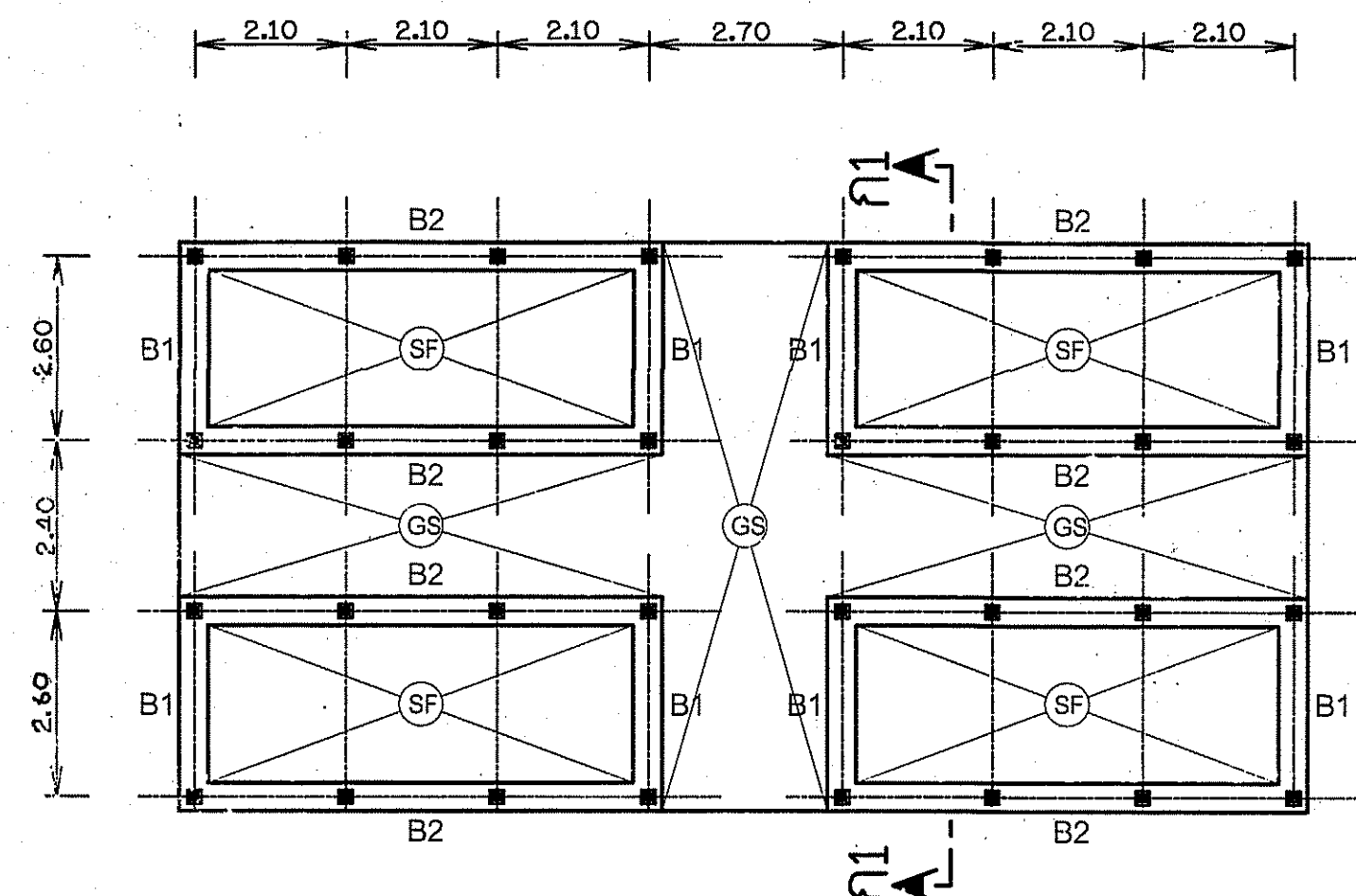
แปลนคานคอดินแฉงเซลล์พลังงานแสงอาทิตย์
