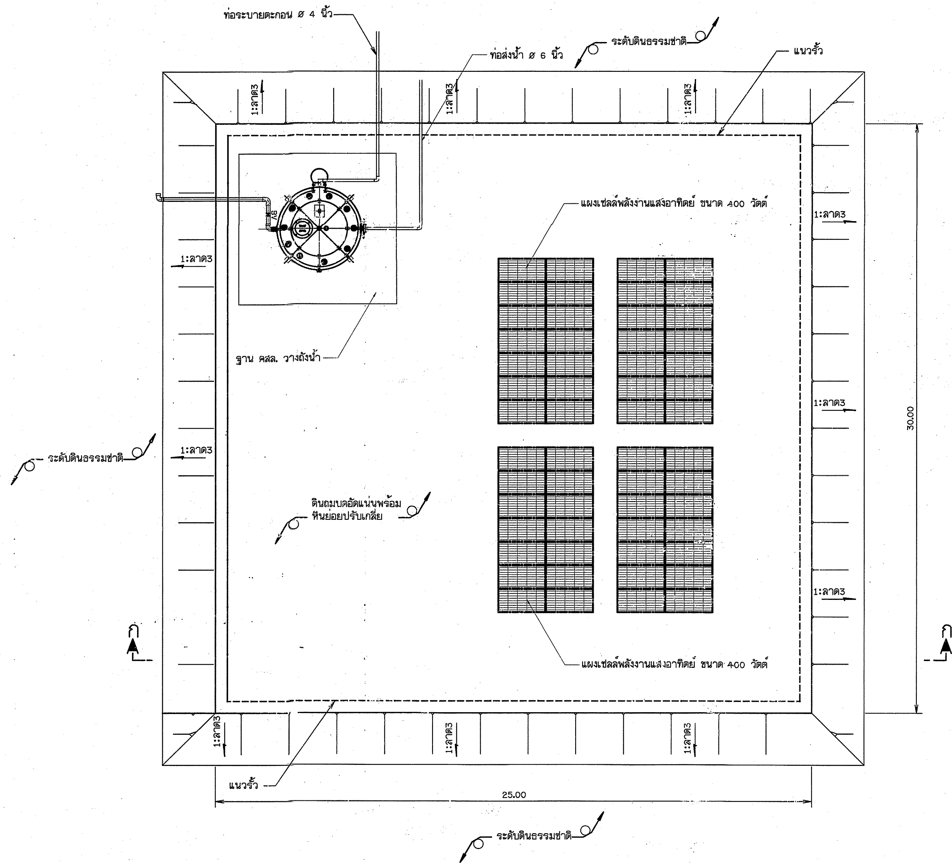
แปลนทั่วไป
