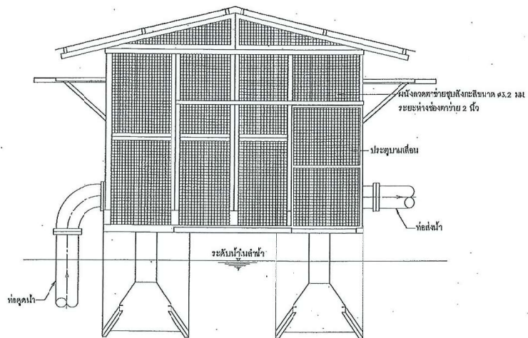
รูปด้าน 1
