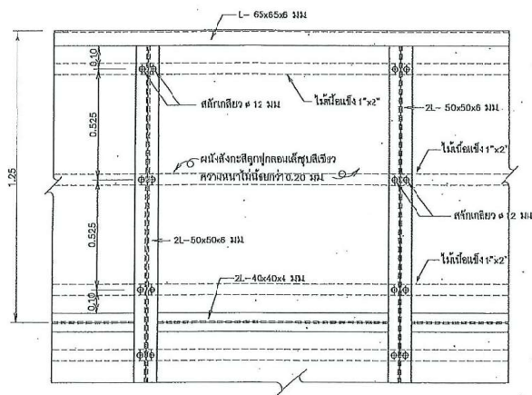
รูปขยายการประกอบติดตั้งผนังหังกะติ
