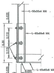
รูปตัด ก-ก
