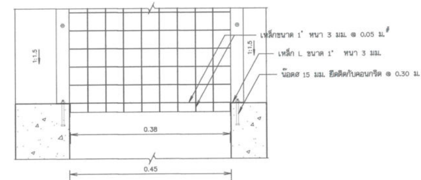
รูปตัด ซ - ซ มาตราส่วน 1 : 5
