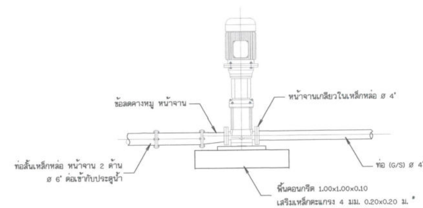
การต่อท่อเครื่องสูบน้ำ ไม่แสดงมาตราส่วน
