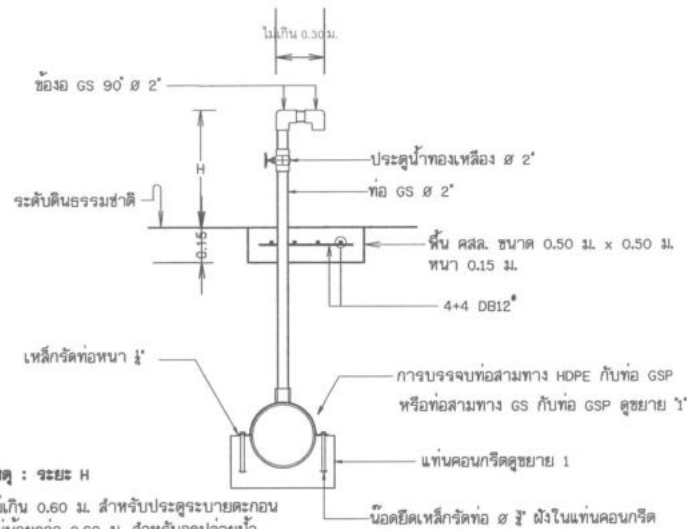
รูปตัดอาคารประตูปน้ำตะกอนและอาคารจุดปล่อยน้ำ
