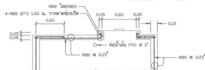
แสดงการเสริมเหล็กฟาด
