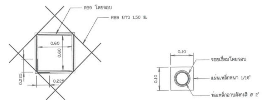
ขยายการเสริมเหล็กช่องคนลง
