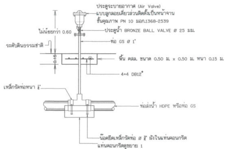
รูปตัดอาคารประตูปน้ำอากาศ (Air Valve)
