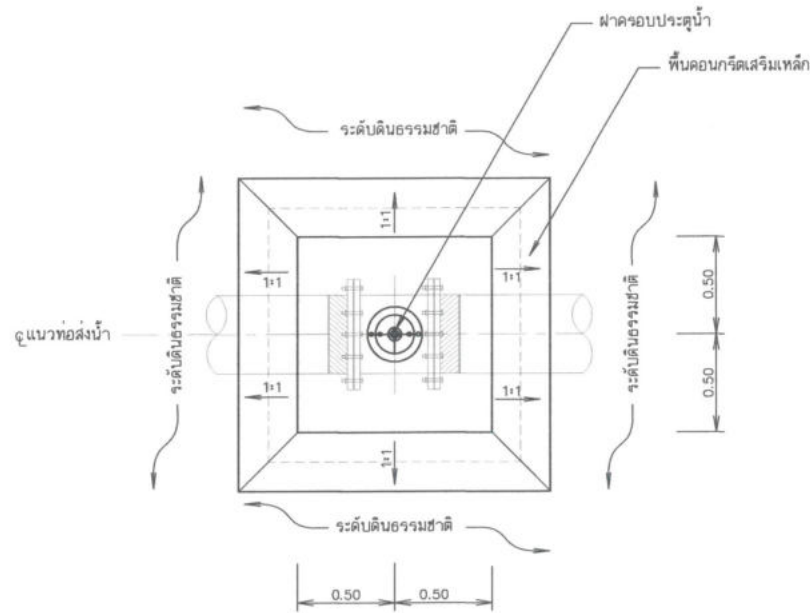
แปลนอาคารควบคุมท่อน้ำ มาตราส่วน 1:20
