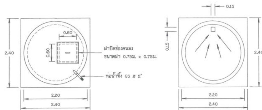
แสดงมิติบ่อรวมตะกอน
