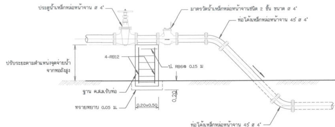
การติดตั้งมาตรวัดน้ำบนพื้นดิน 1/2" ไม่แสดงมาตราส่วน
