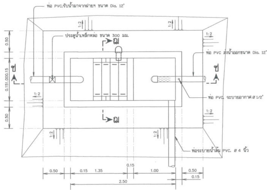
แปลนบ่อตกตะกอน
