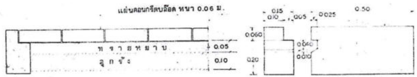
รูปขยายคั่นคอนกรีต 1:10
