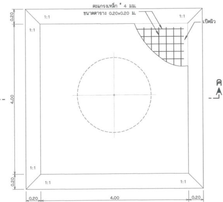
แปลงพื้นคอนกรีตเสริมเหล็ก
