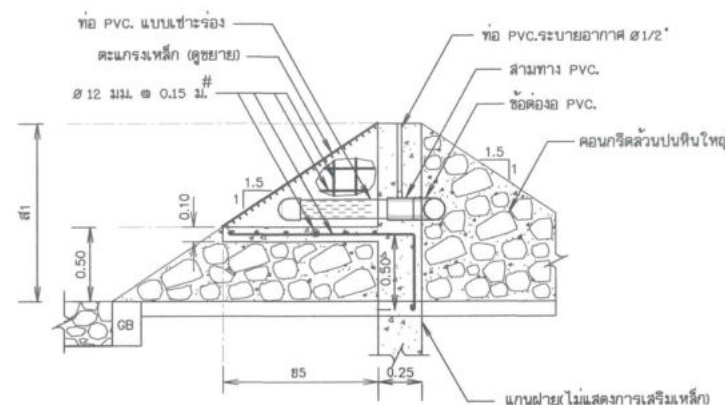
รูปตัด ช - ช มาตราส่วน 1 : 25
