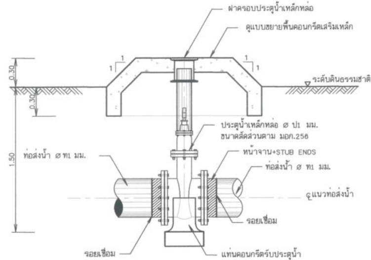
รูปตัดอาคารควบคุมท่อน้ำ มาตราส่วน 1:20
