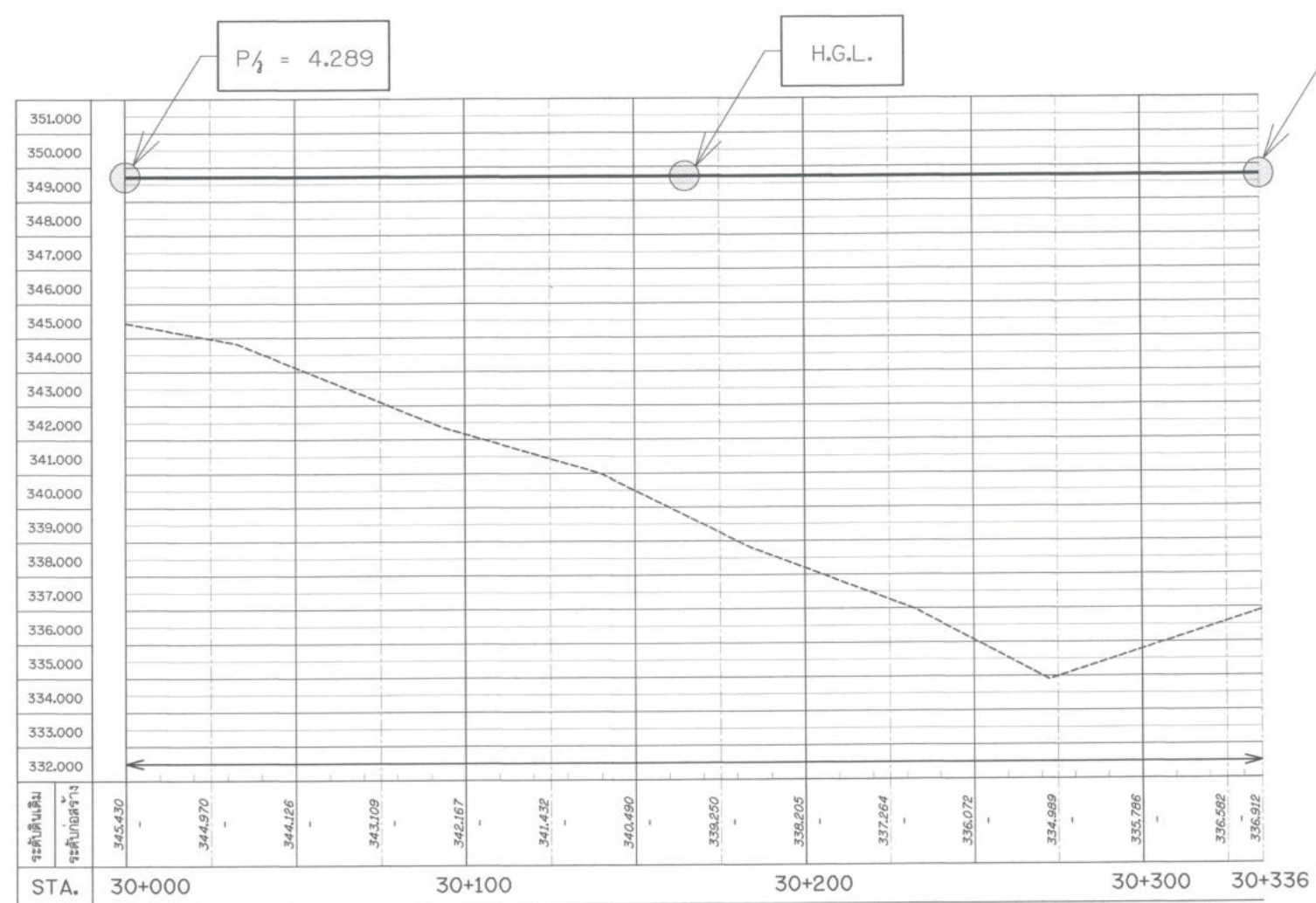
รูปตัดตามแนวยาวแสดง H.G.L. สาย 1L-RMP STA. 30+000 - 30+336
