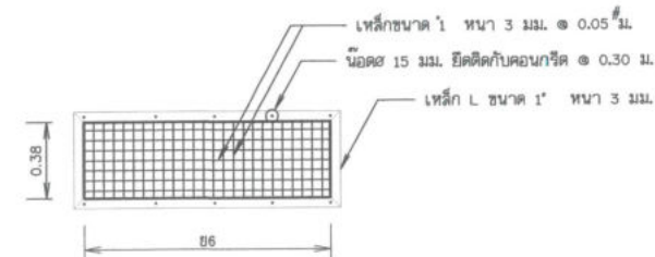
แปลนตะแกรงเหล็กกันสวะ มาตราส่วน 1 : 20
