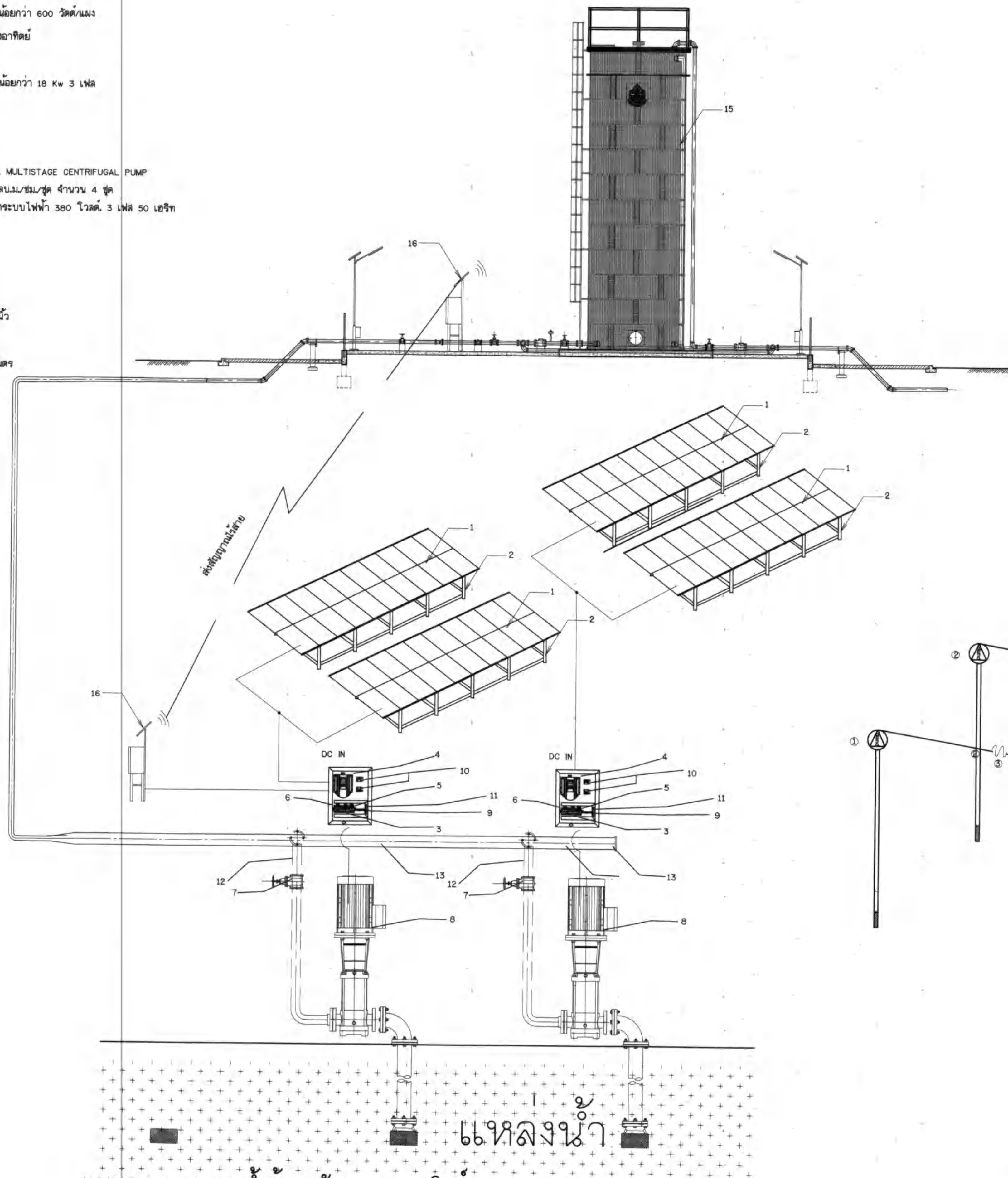
แบบระบบกระจายน้ำด้วยพลังงานแสงอาทิตย์ มาตราส่วน ไม่แสดงมาตราส่วน
