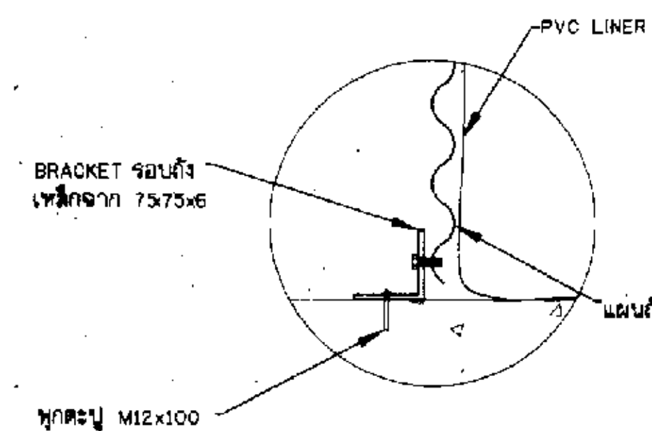
แบบขยาย 11 - ติดตั้งบันไดลอยในถัง Scale NTC.
