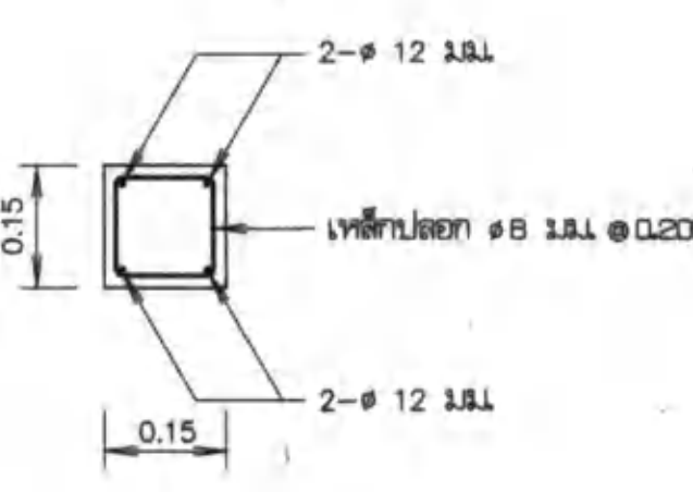
รูปตัด ก - ก มาตราส่วน 1:10
