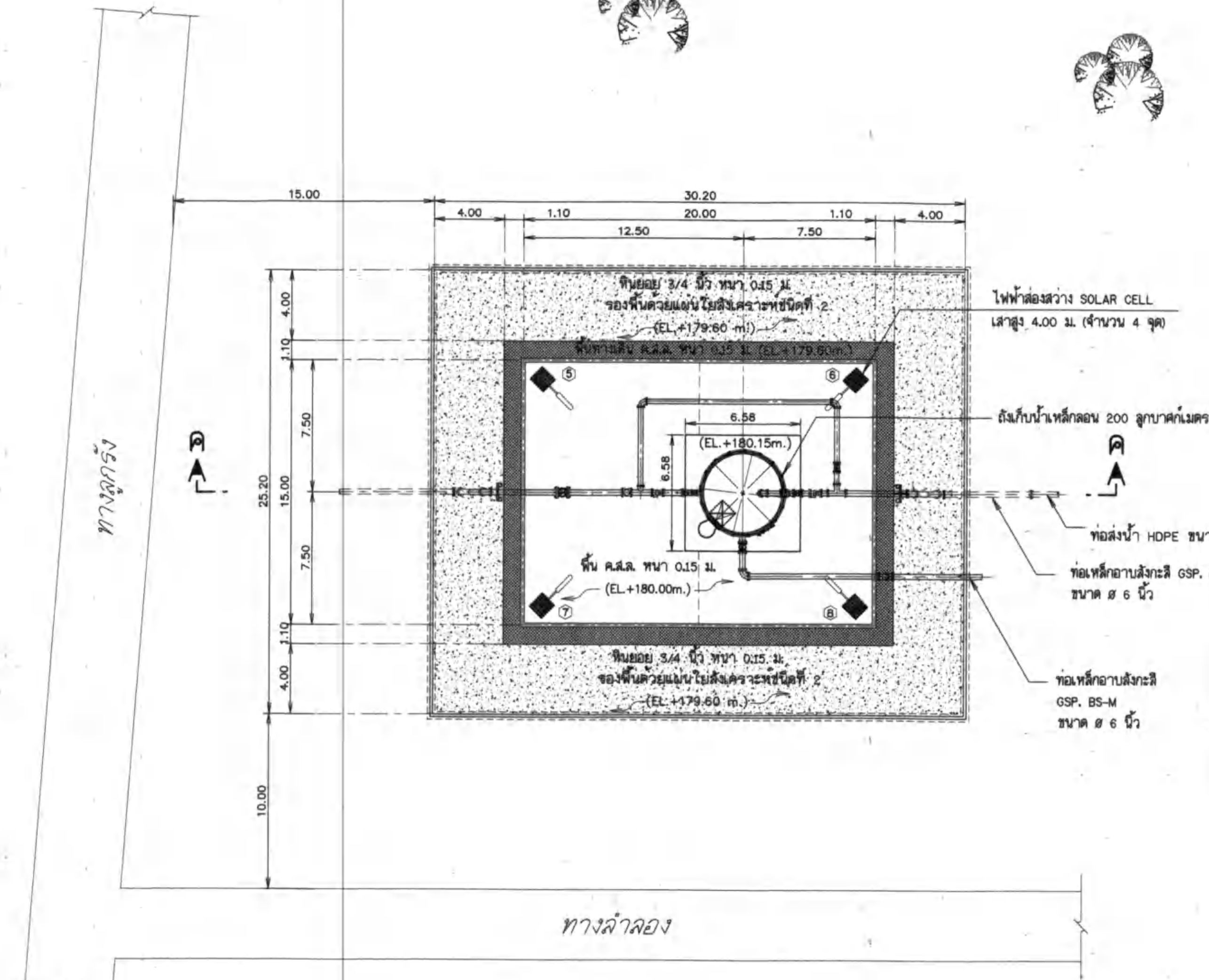
แปลนอาคารหอถังเก็บน้ำ
