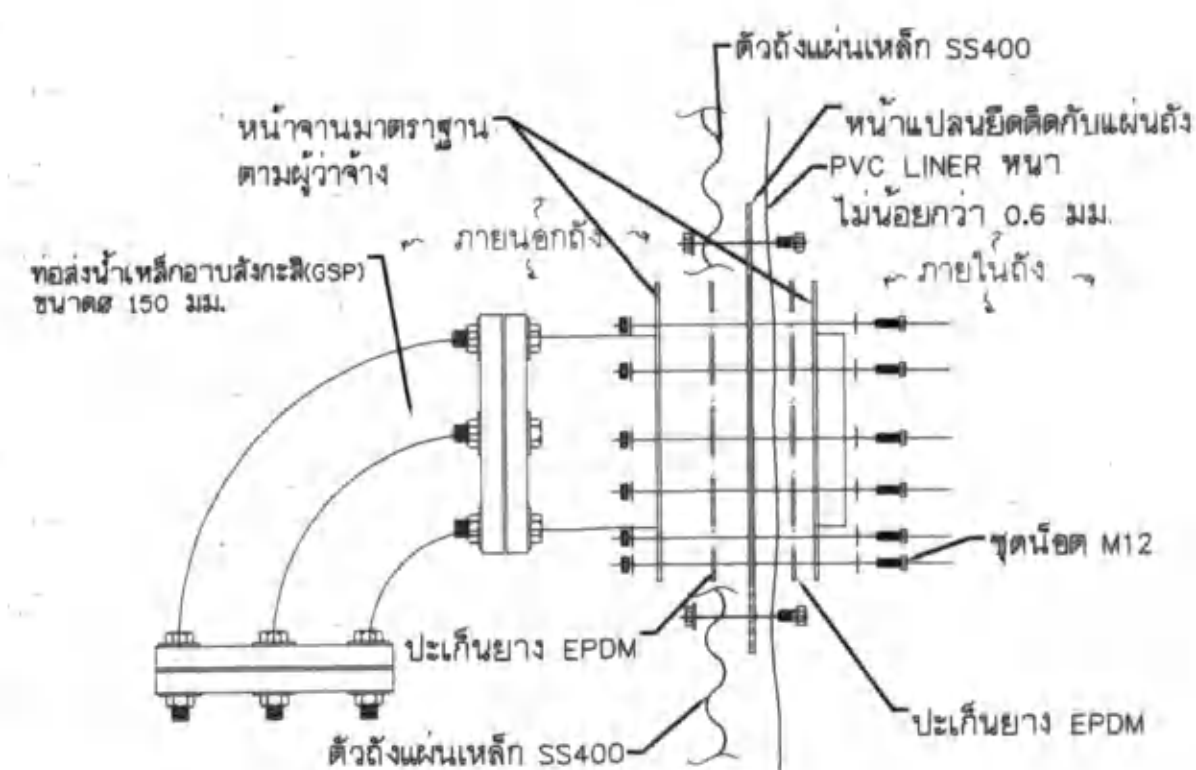
แบบขยาย 5- รูปแบบประกอบหน้าแปลน
