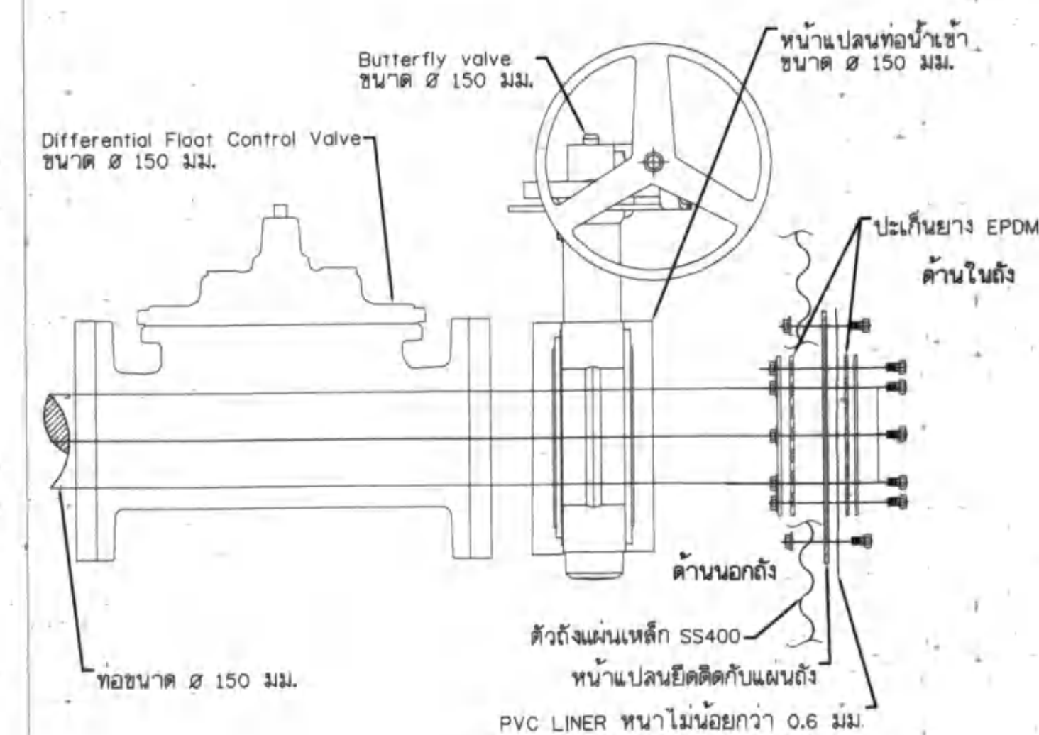
แบบขยาย 4
