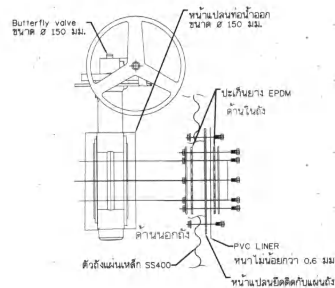
แบบขยาย 7
