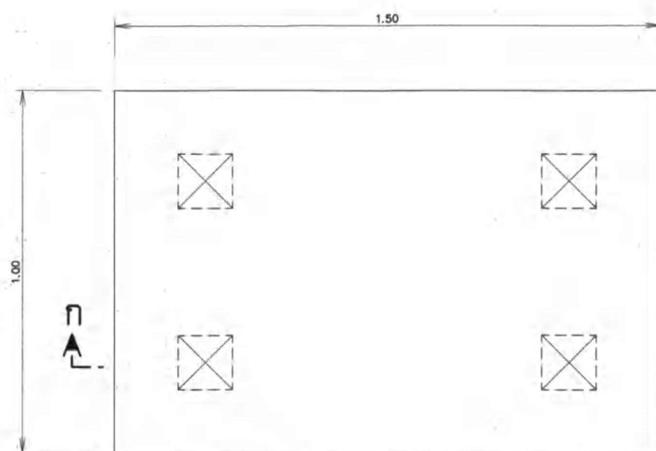
แปลนแท่นเครื่องกว้าน ไม่แสดงมาตราส่วน
