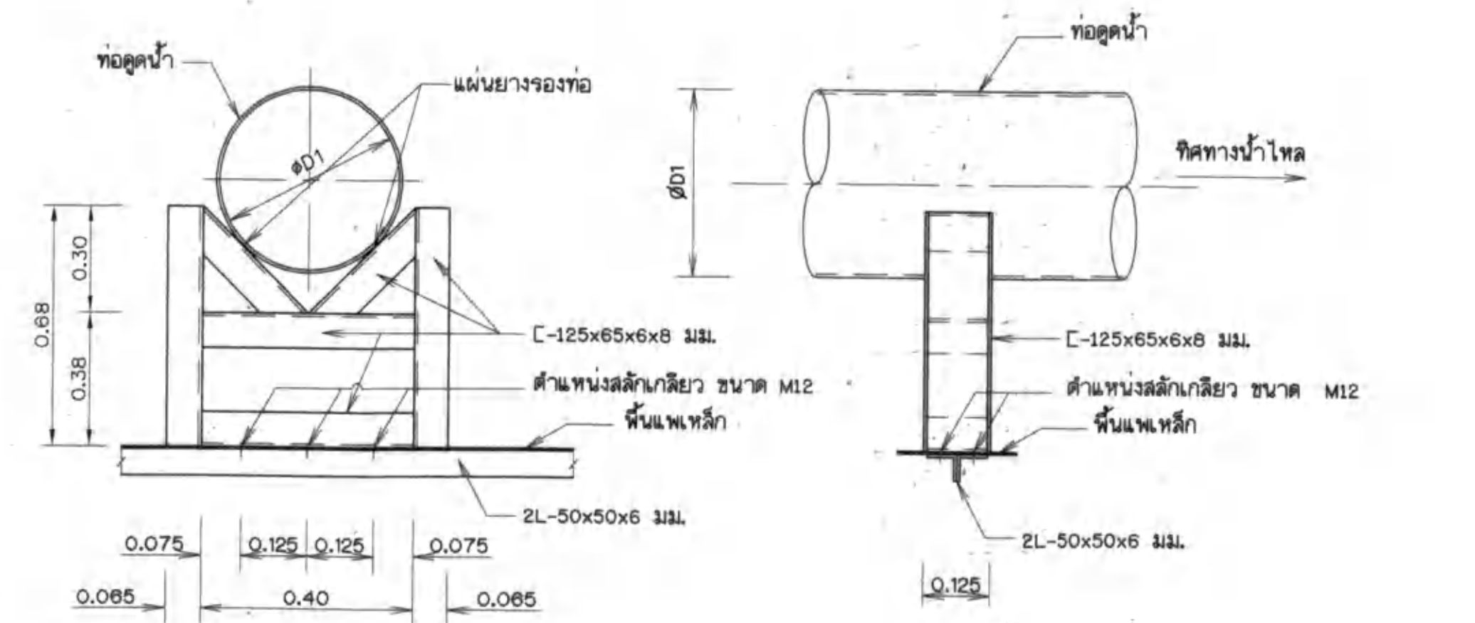
รูปขยาย SUPPORT "A" ไม่แสดงมาตราส่วน
