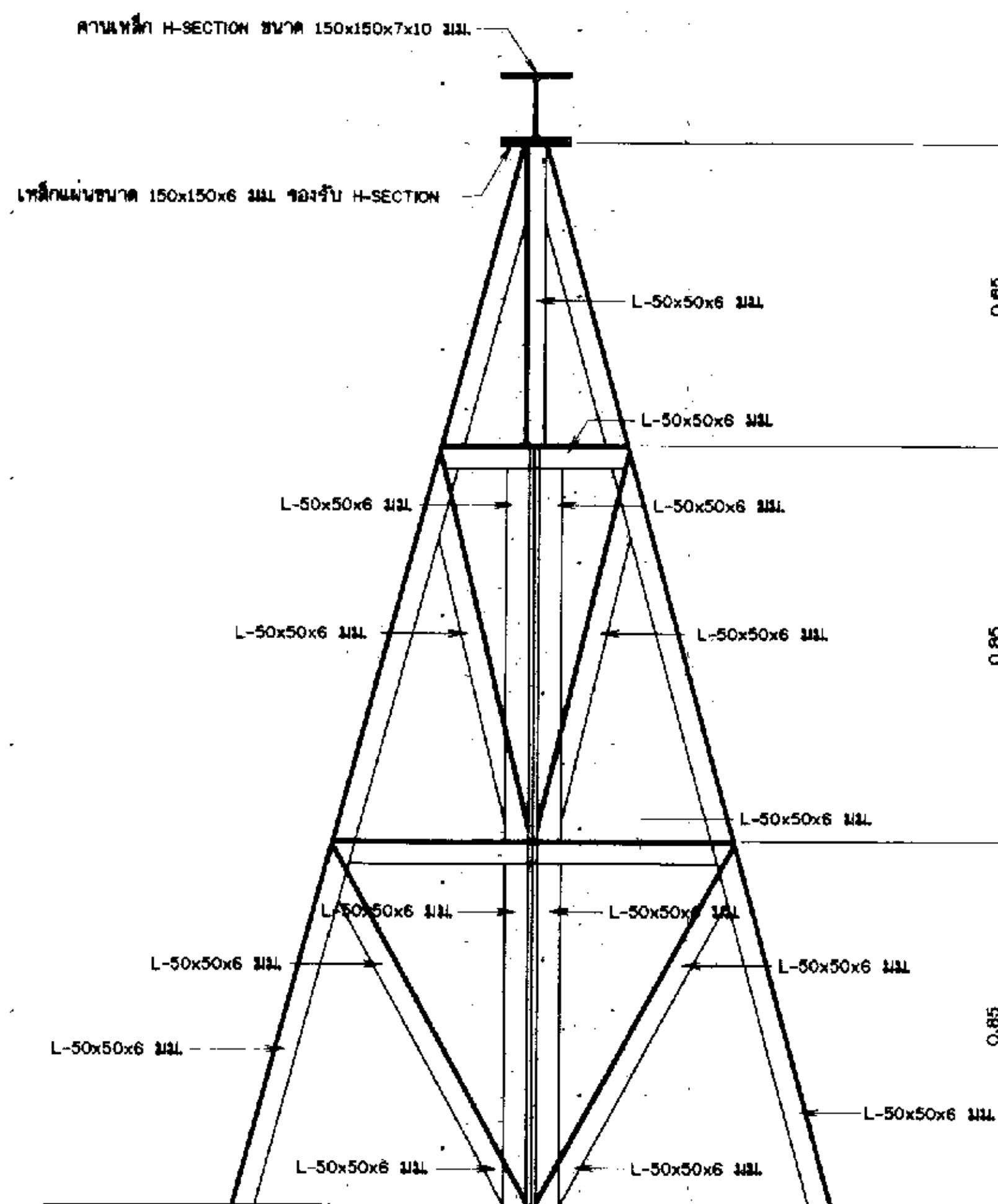
รูปขยายขาดังรูปตัว A รับคานาเหล็ก มาตราส่วน 1 : 10
