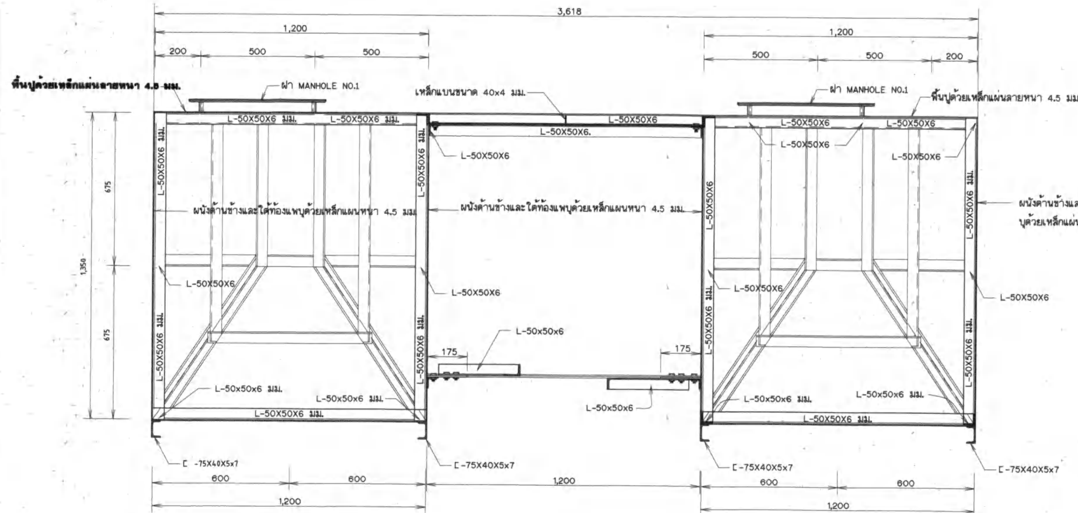
รูปตัด ง - ง
