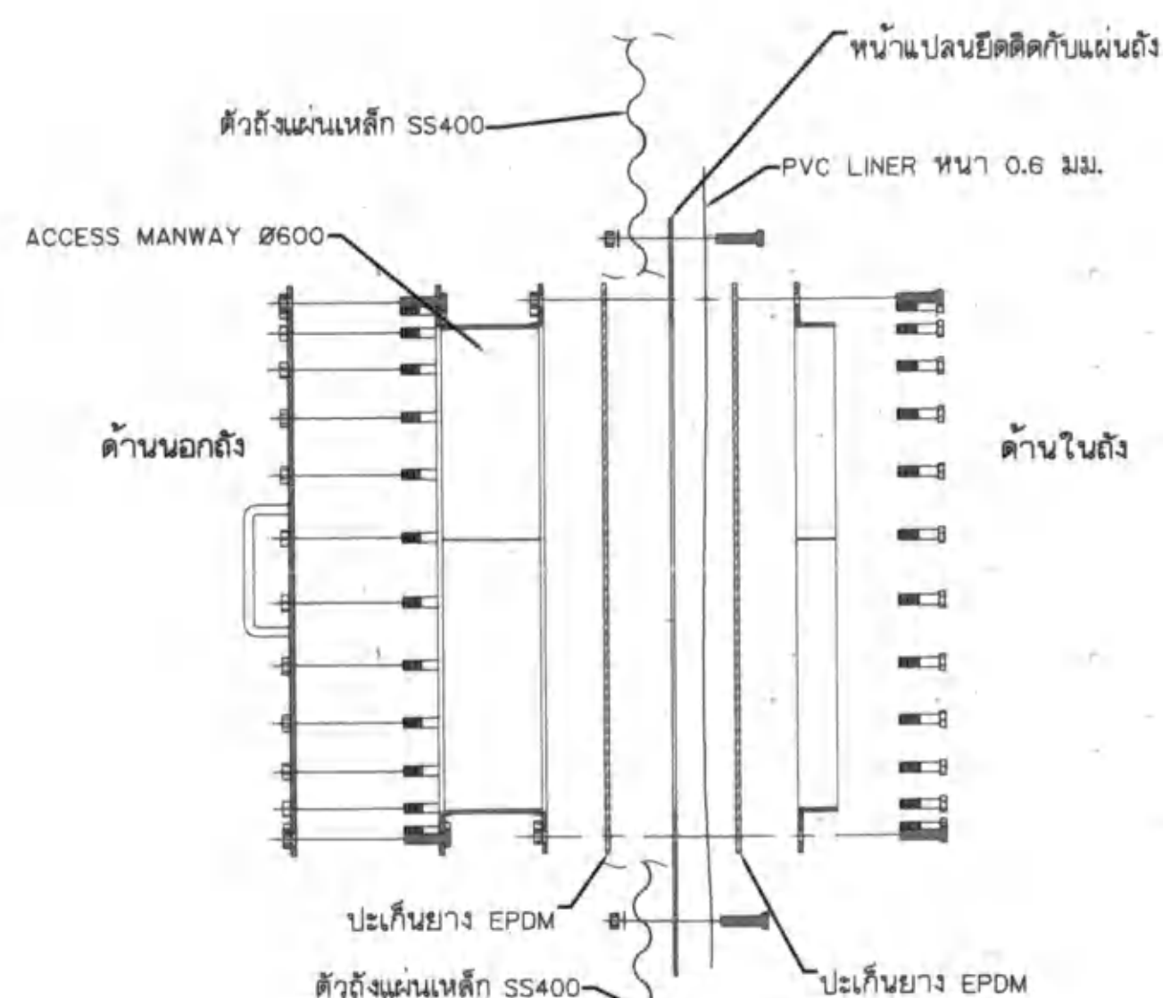
แบบขยายประตูตรวจสอบบำรุงรักษา
