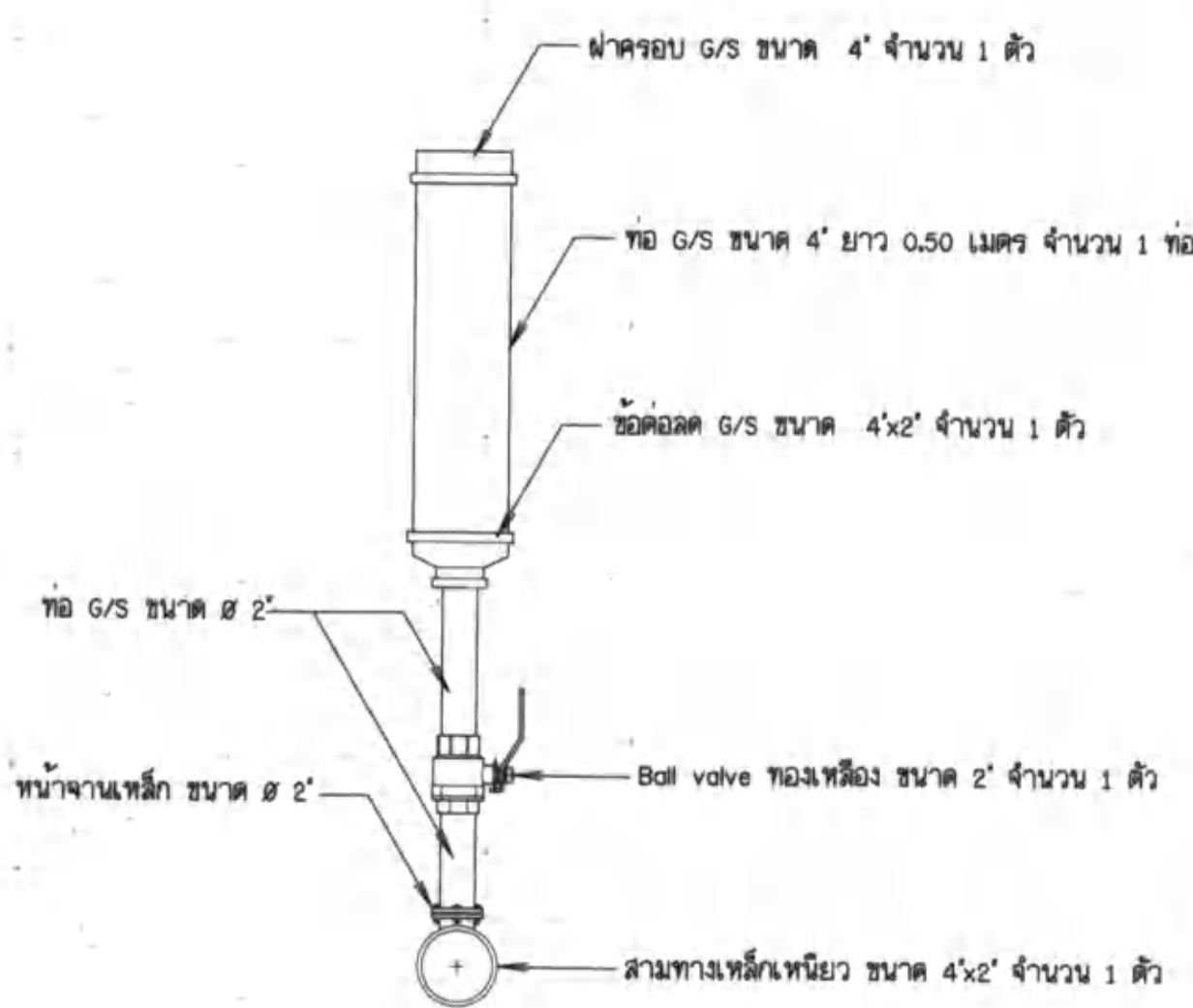
ขยาย 1 ไม่แสดงมาตราส่วน
