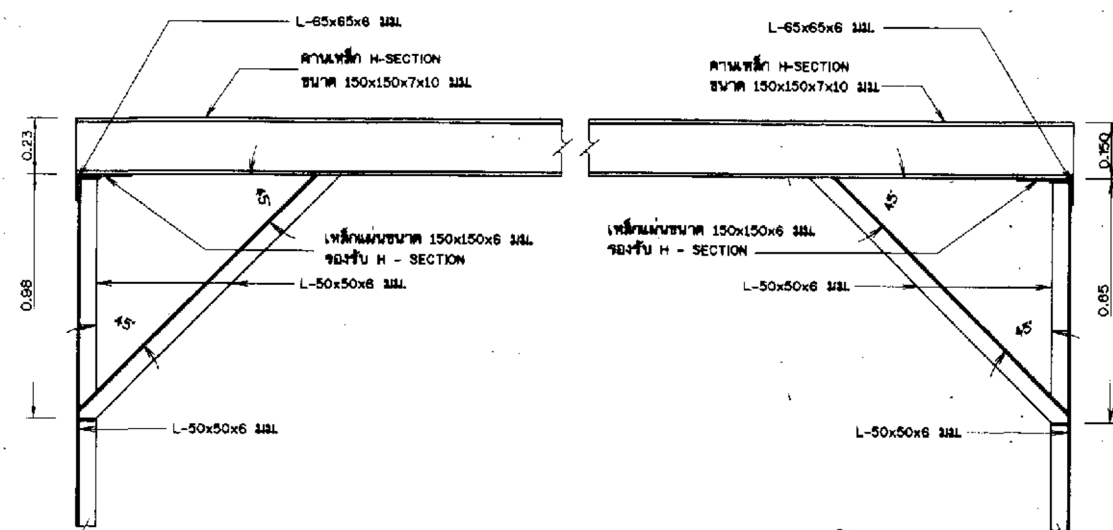
รายละเอียดคานาเหล็กยกเครื่องสูบน้ำ มาตราส่วน 1 : 10
