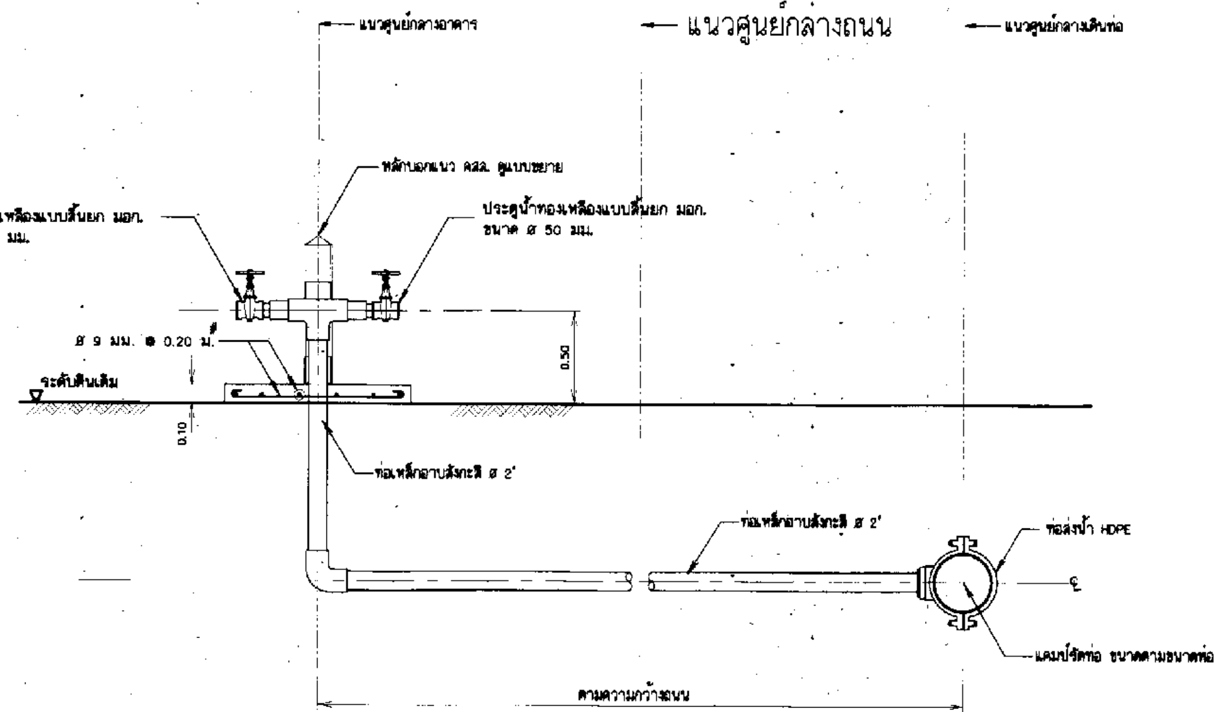
รูปตัด ก - ก (แบบที่ 2 กรณีข้ามถนน)
