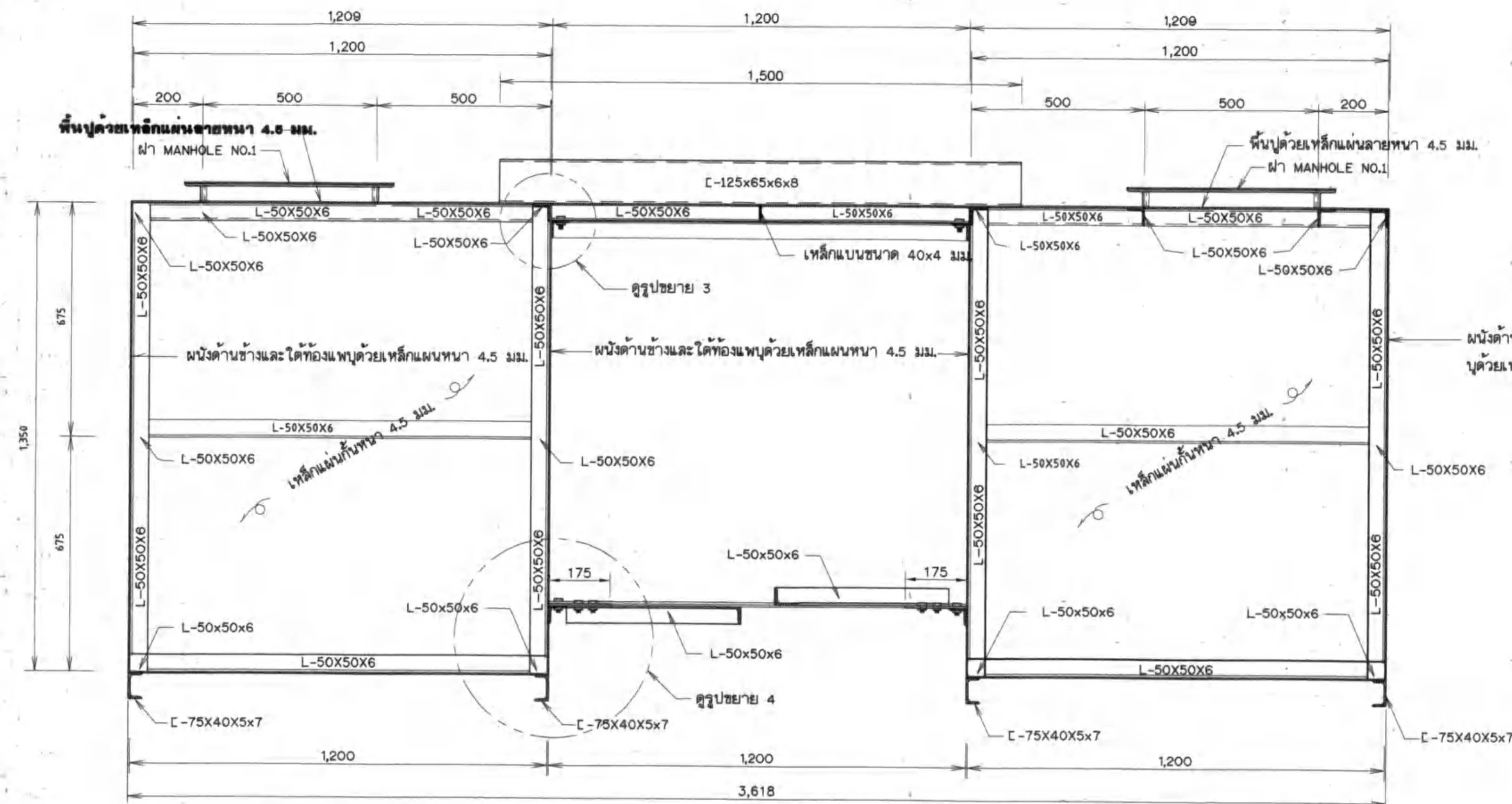
รูปตัด ค - ค
