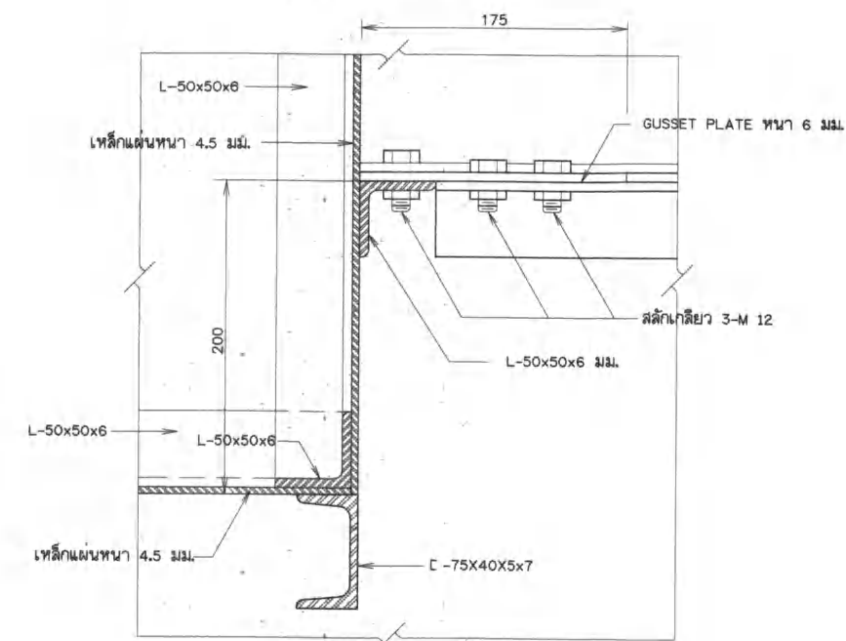
รูปขยาย 4
