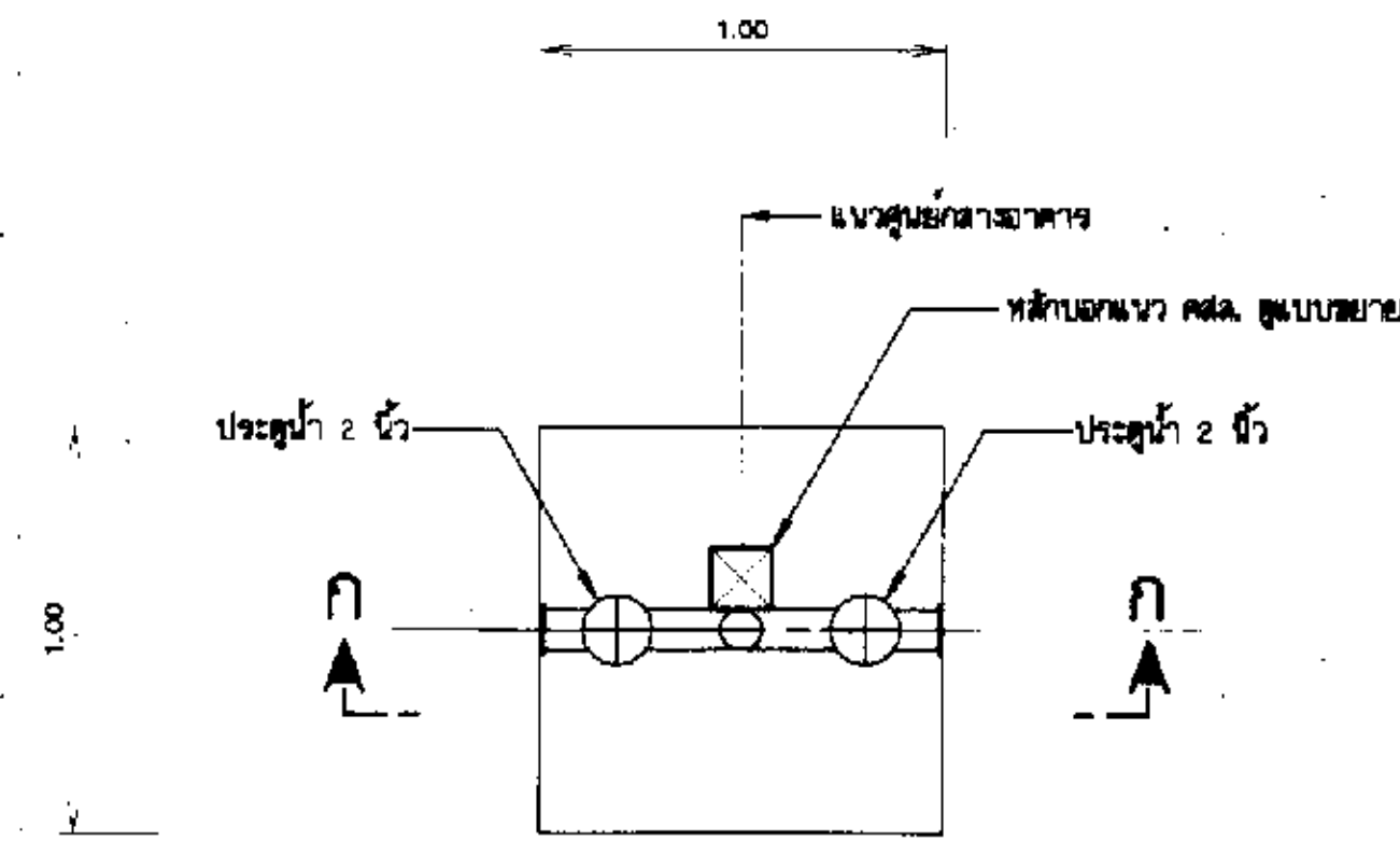
แปลนอาคารจุดปล่อยน้ำ (แบบ ก)
