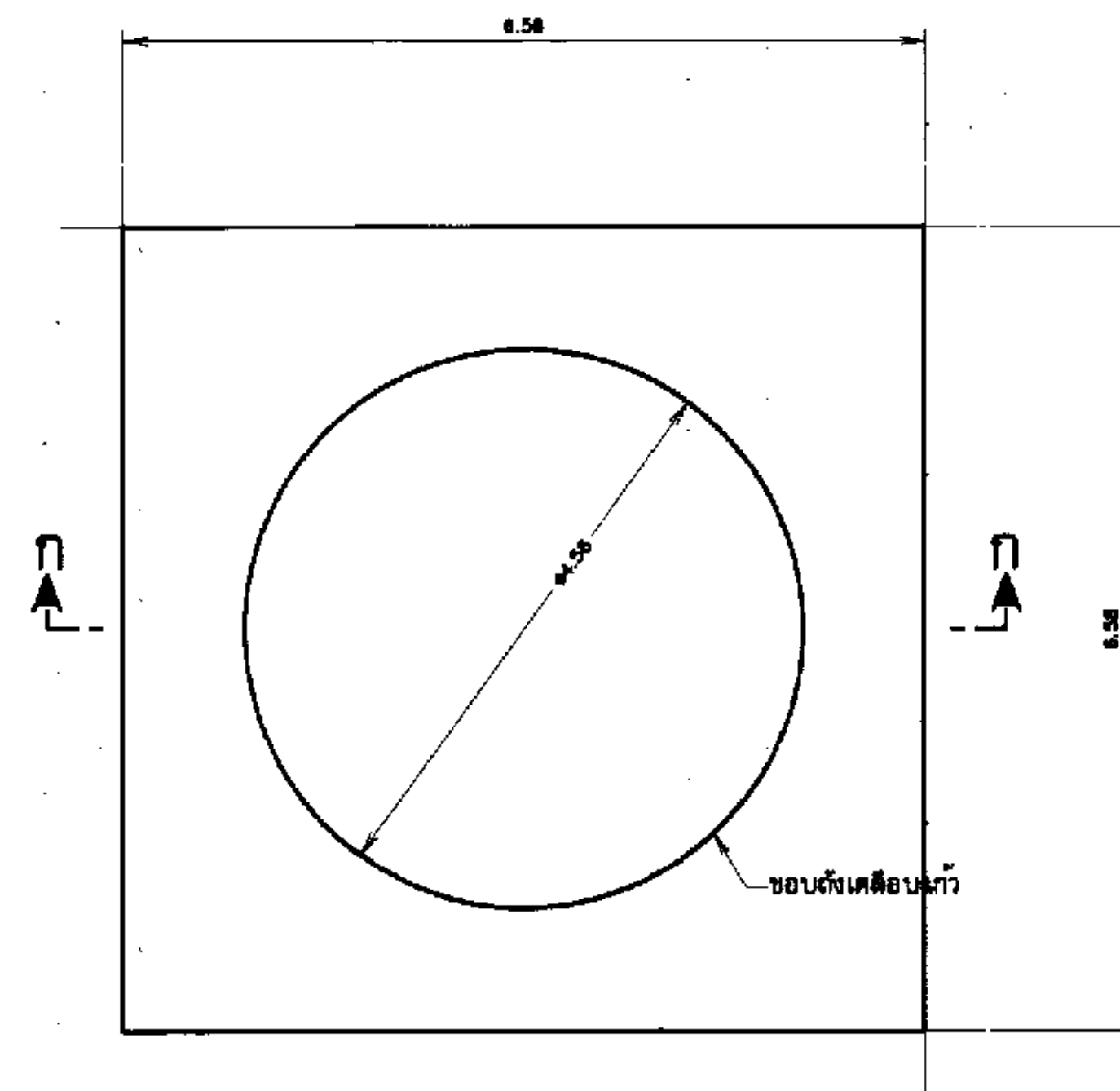
แปลนฐานรากแบบไม่มีเสาเข็ม
