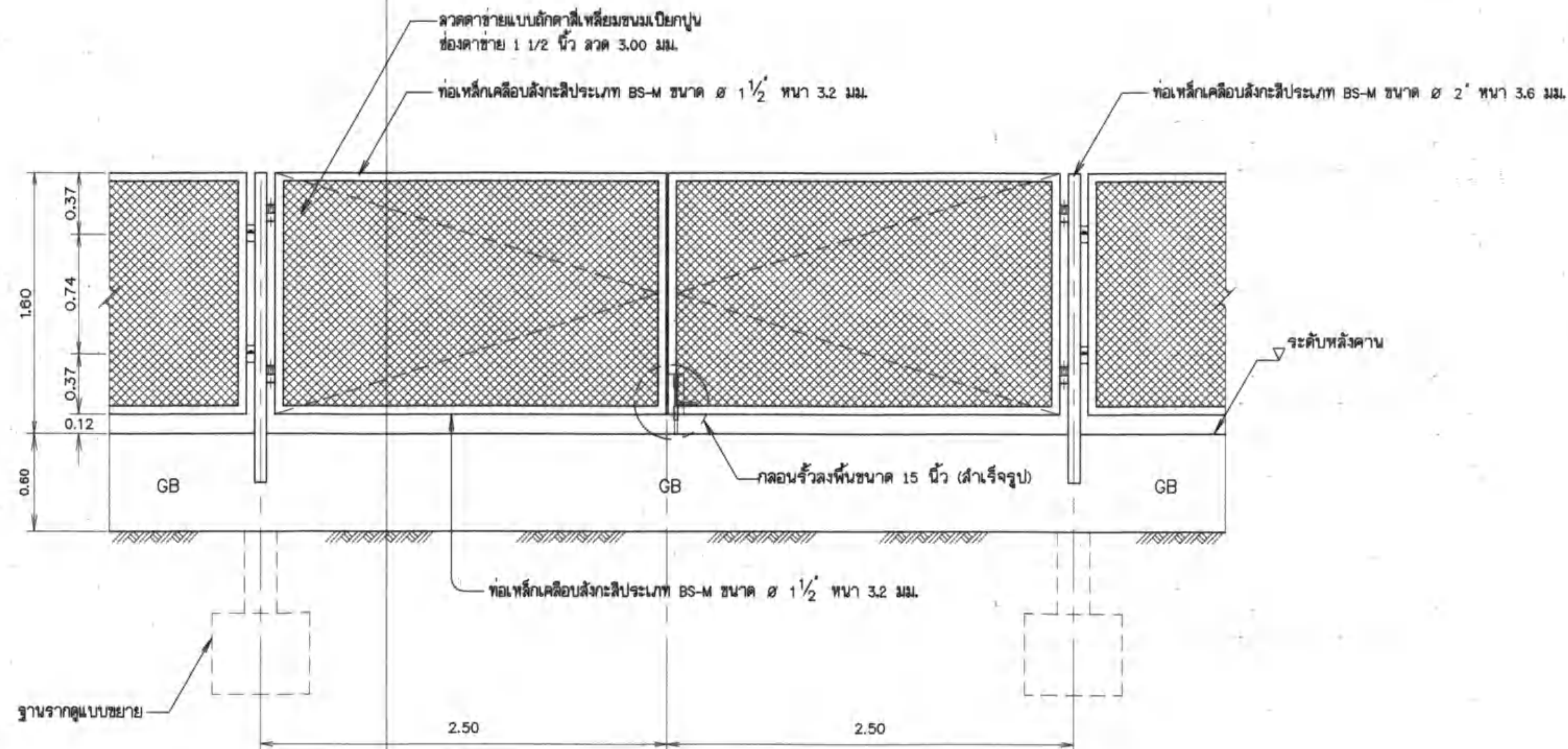
แบบขยายประตูรั้ว
