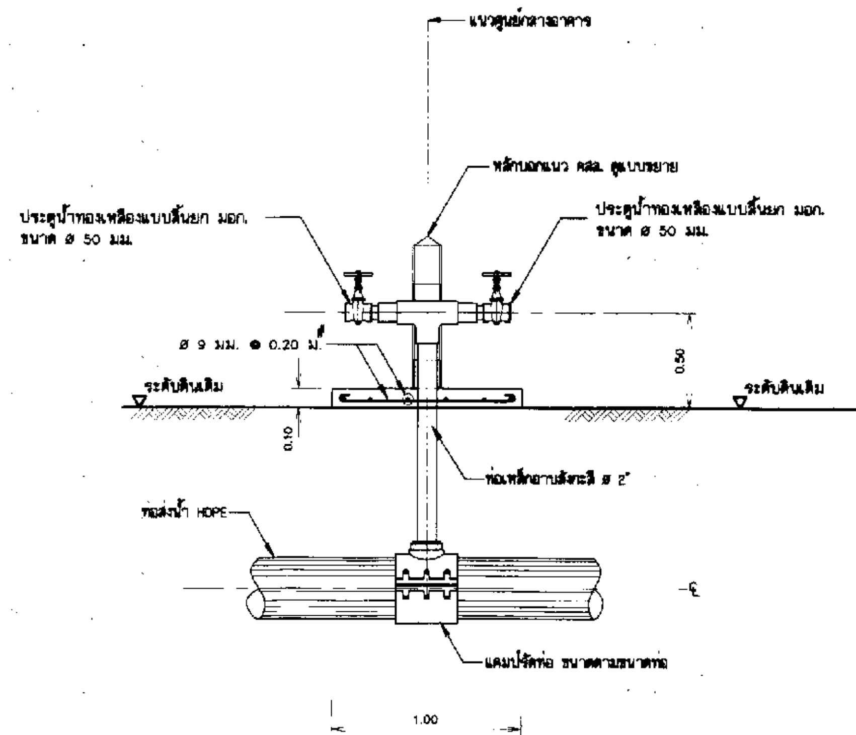
รูปตัด ก - ก (แบบที่ 1)
