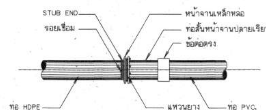
6. การบรรจุท่อ HDPE กับท่อ PVC. ไม่แสดงมาตราส่วน
