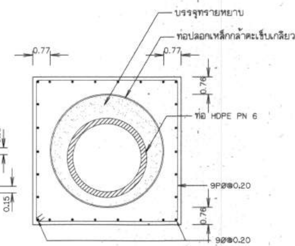
รูปตัด ก-ก มาตราส่วน 1:20
