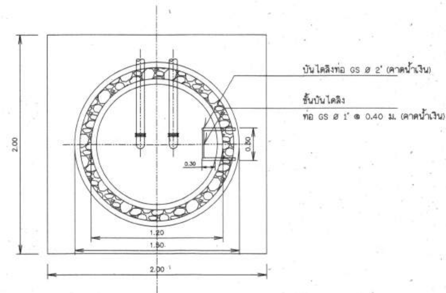
แปลนอาคารบ่อกรองน้ำดิบ คสล.
