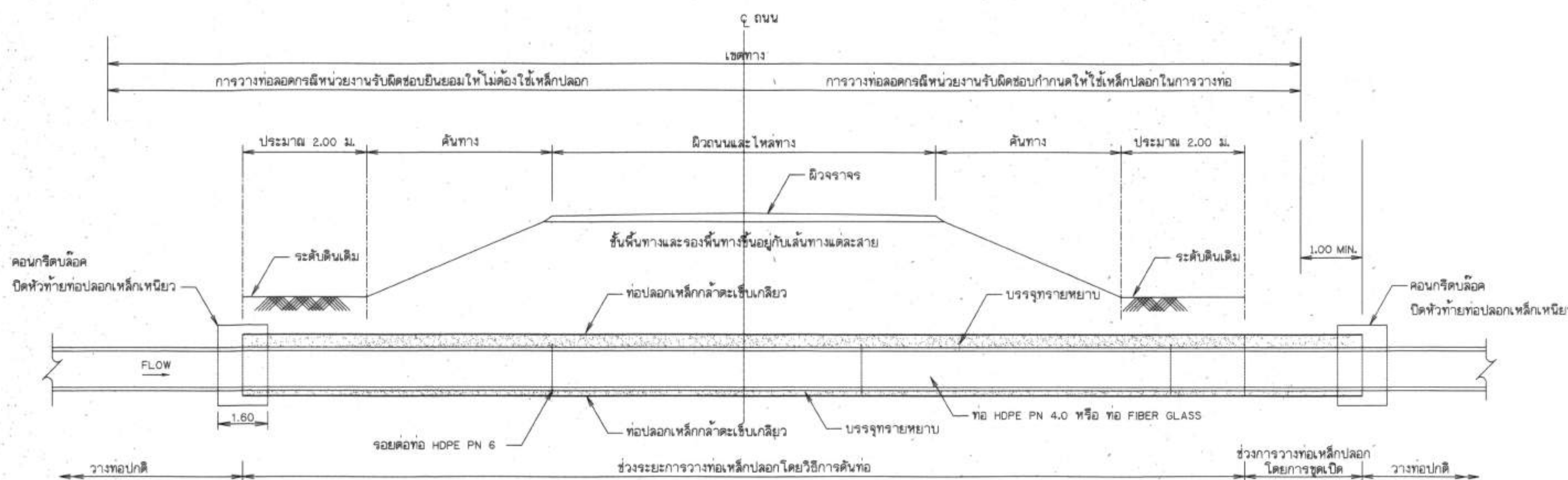
แสดงการวางท่อตลอดใต้ผิวจราจร
