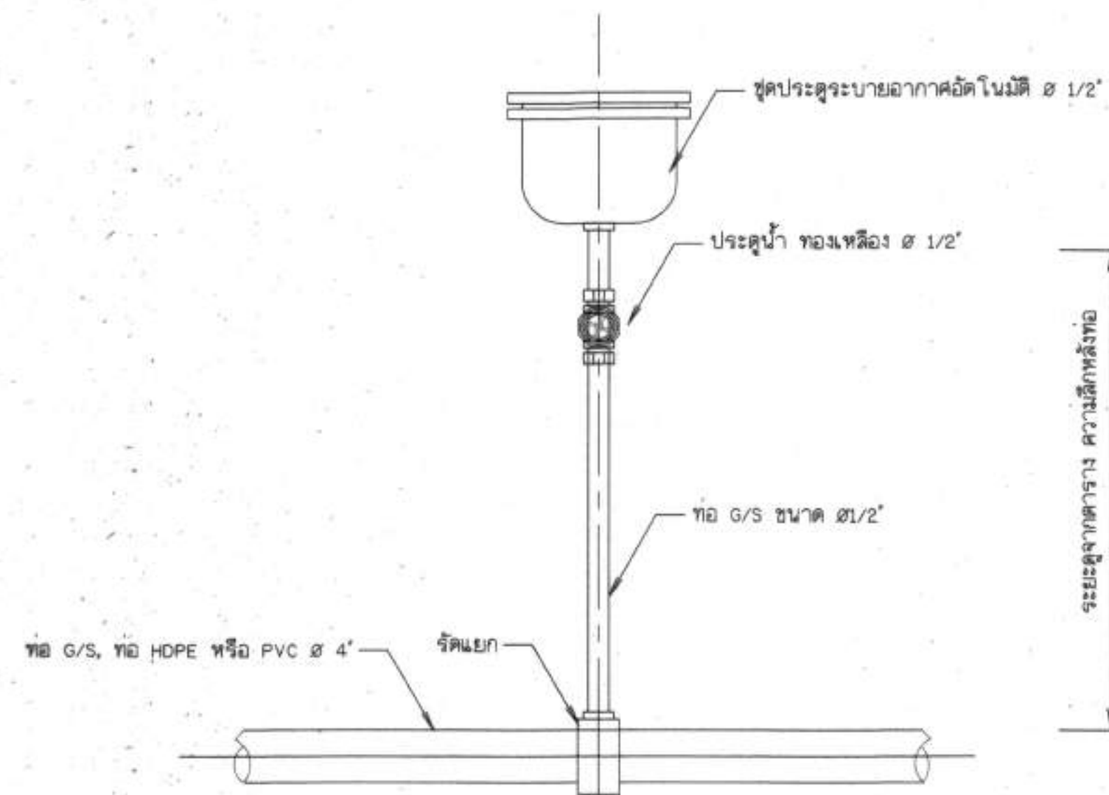
11. การติดตั้งประตูปะบายอากาศอัตโนมัติ ไม่แสดงมาตราส่วน
