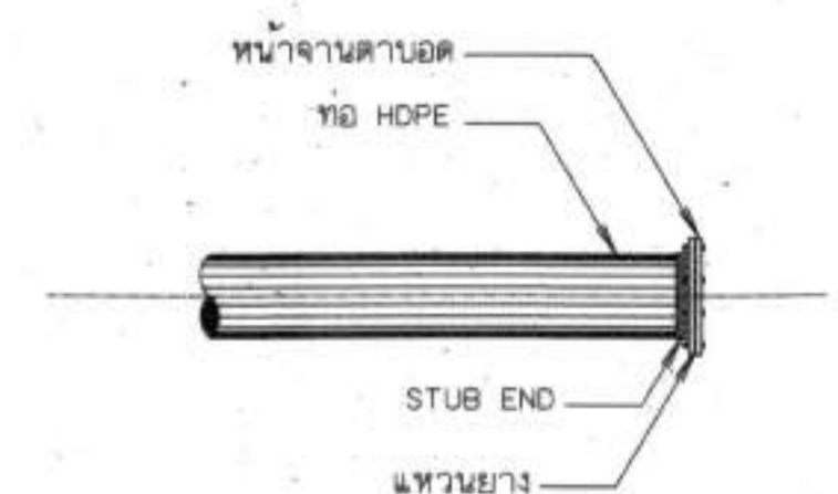
7. การปิดปลายท่อ ไม่แสดงมาตราส่วน
