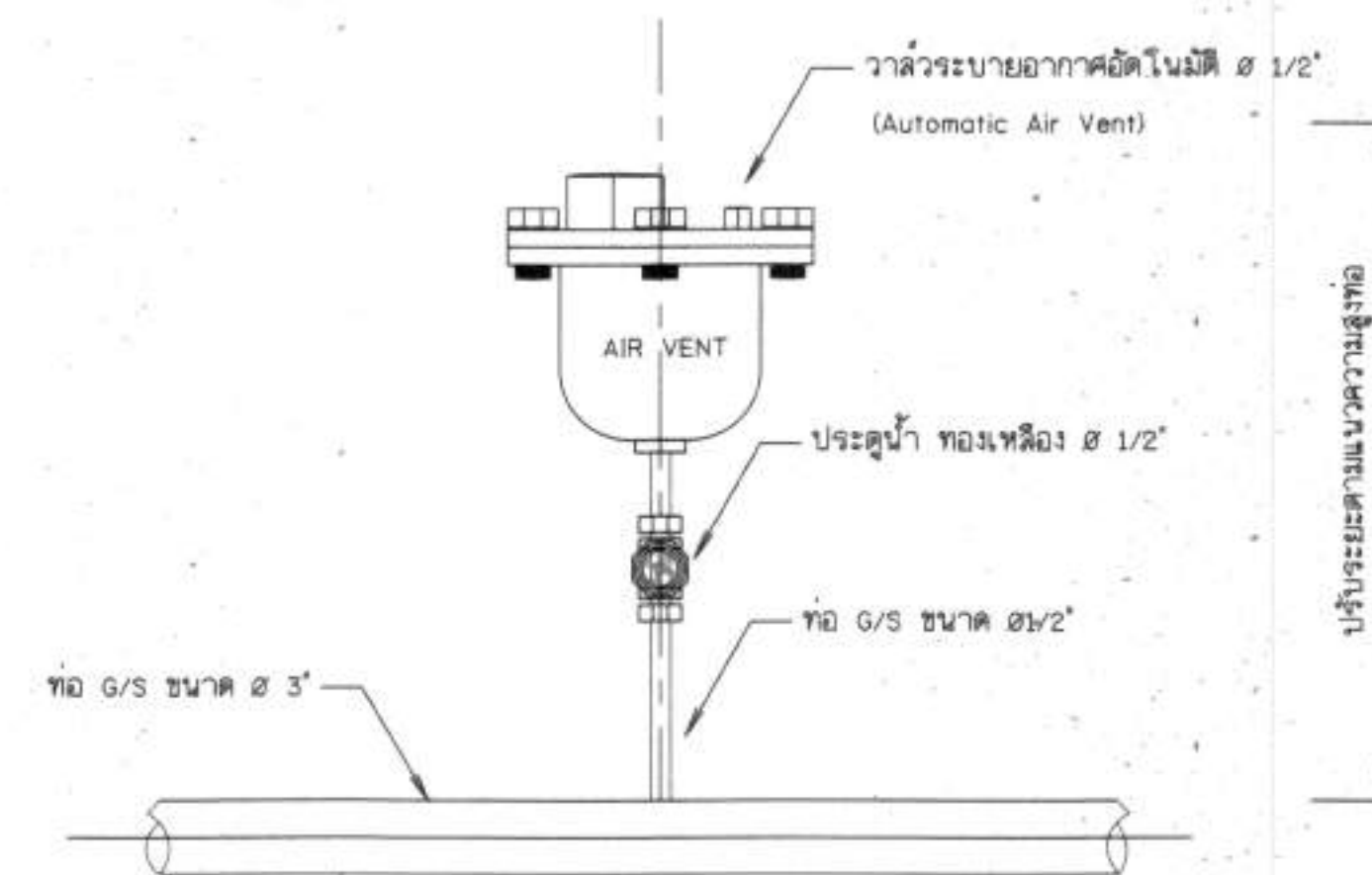
12. การติดตั้งวาล์วระบายอากาศอัตโนมัติ (Automatic Air Vent) ไม่แสดงมาตราส่วน
