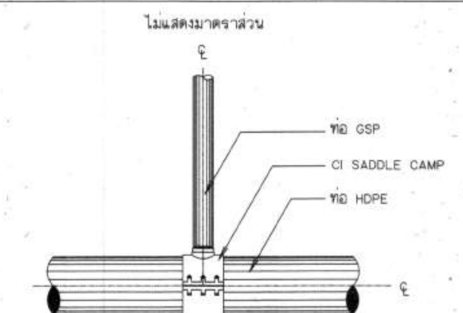
9. การบรรจุท่อสามทาง HDPE กับท่อ GSP แบบ CI SADDLE CLAMP
