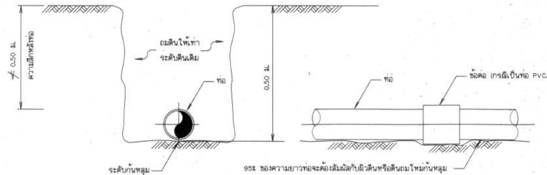
1. แบบการวางท่อทั่วไป ไม่แสดงมาตราส่วน
