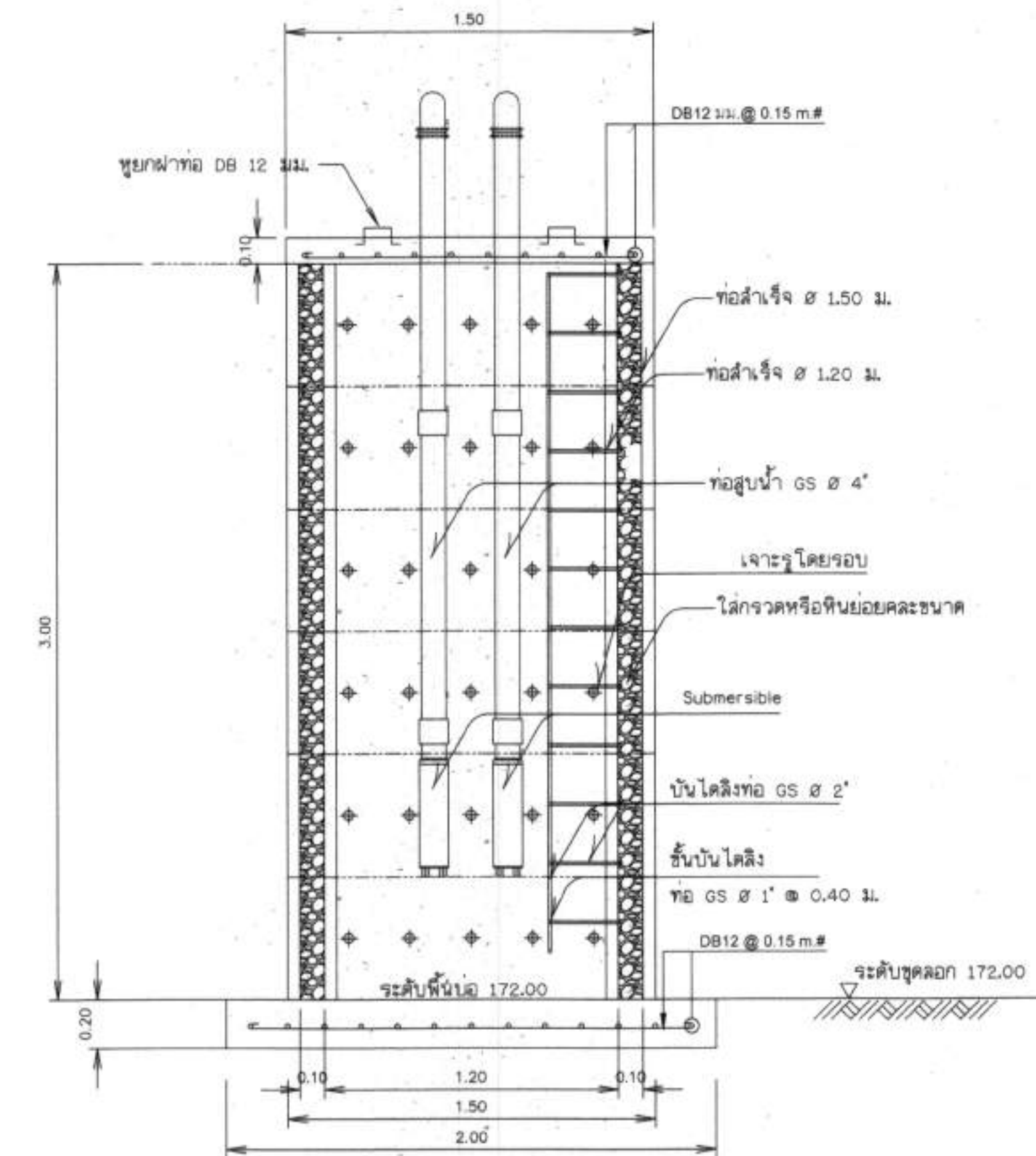
แบบรูปตัดอาคารบ่อกรองน้ำดิบ คสล.
