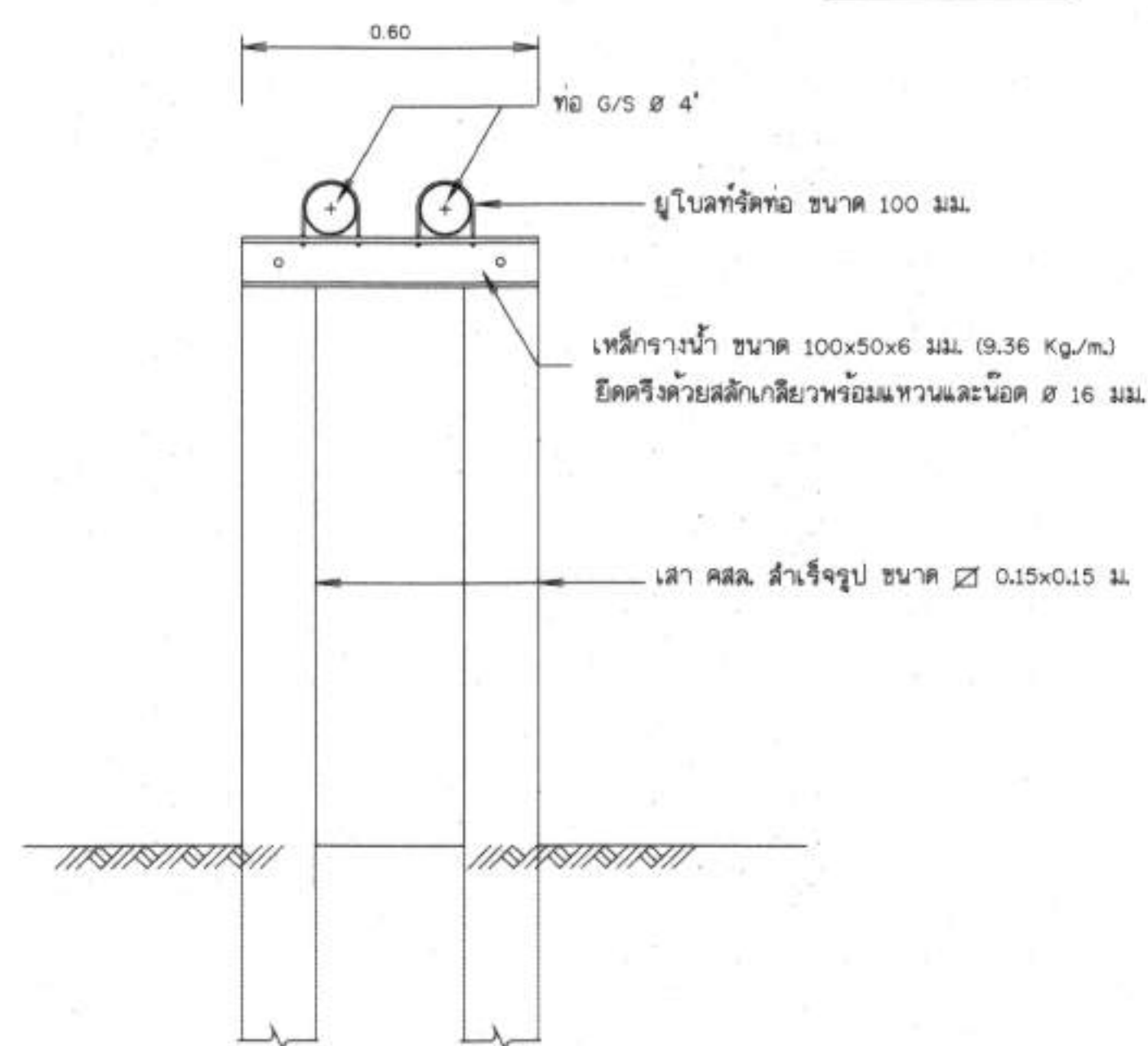
13. เสาดอมรองรับท่ออุด และแบบขยายอุปกรณ์รัดท่อ ไม่แสดงมาตราส่วน
