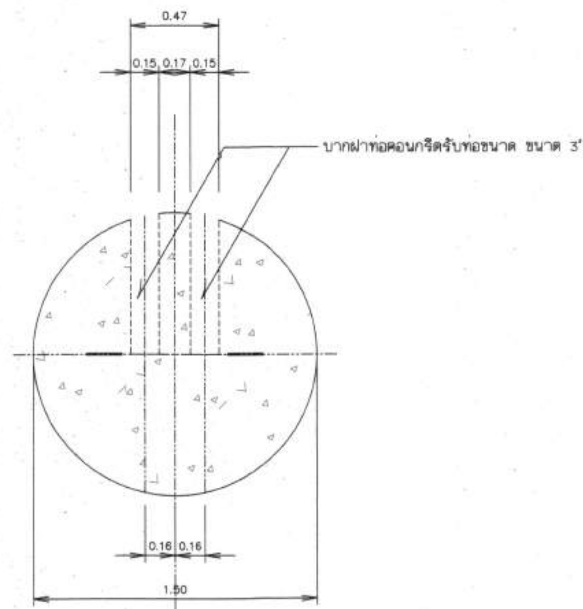
แปลนฝาท่อกรองน้ำดิบ คสล.
