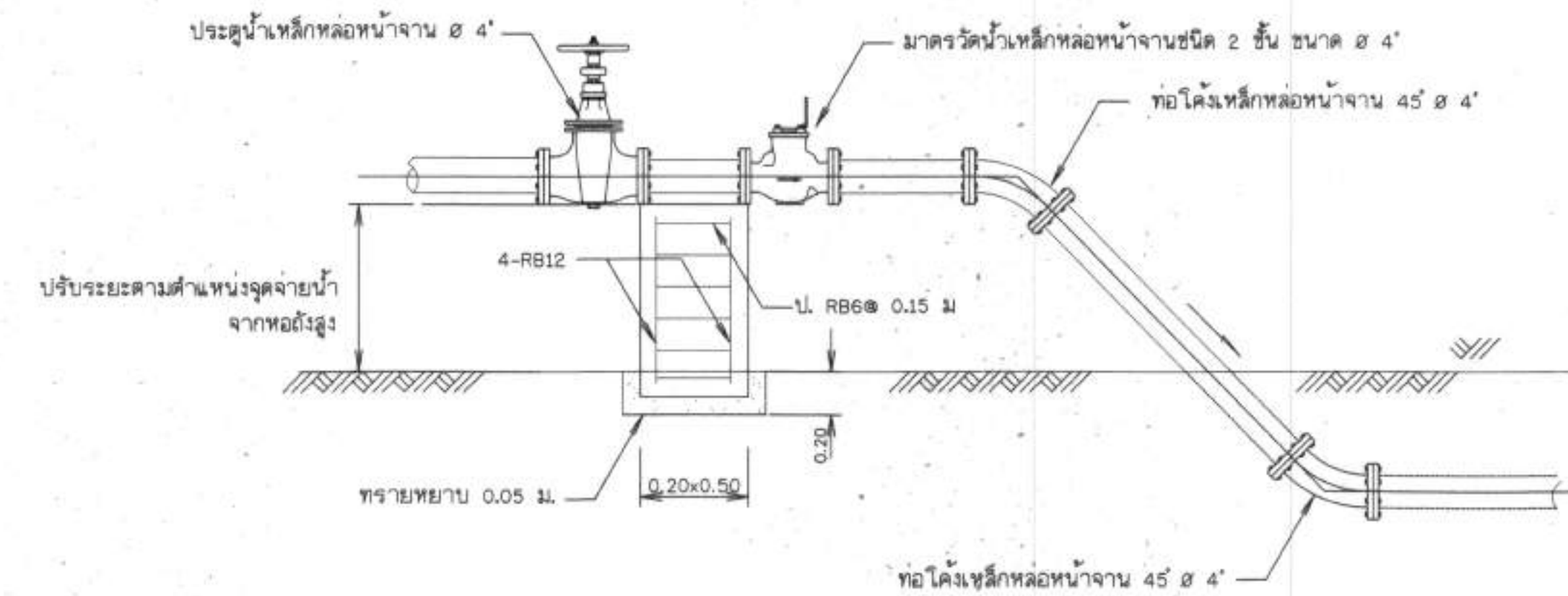
14. การติดตั้งมาตรวัดน้ำบนพื้นดิน 4\"/>
