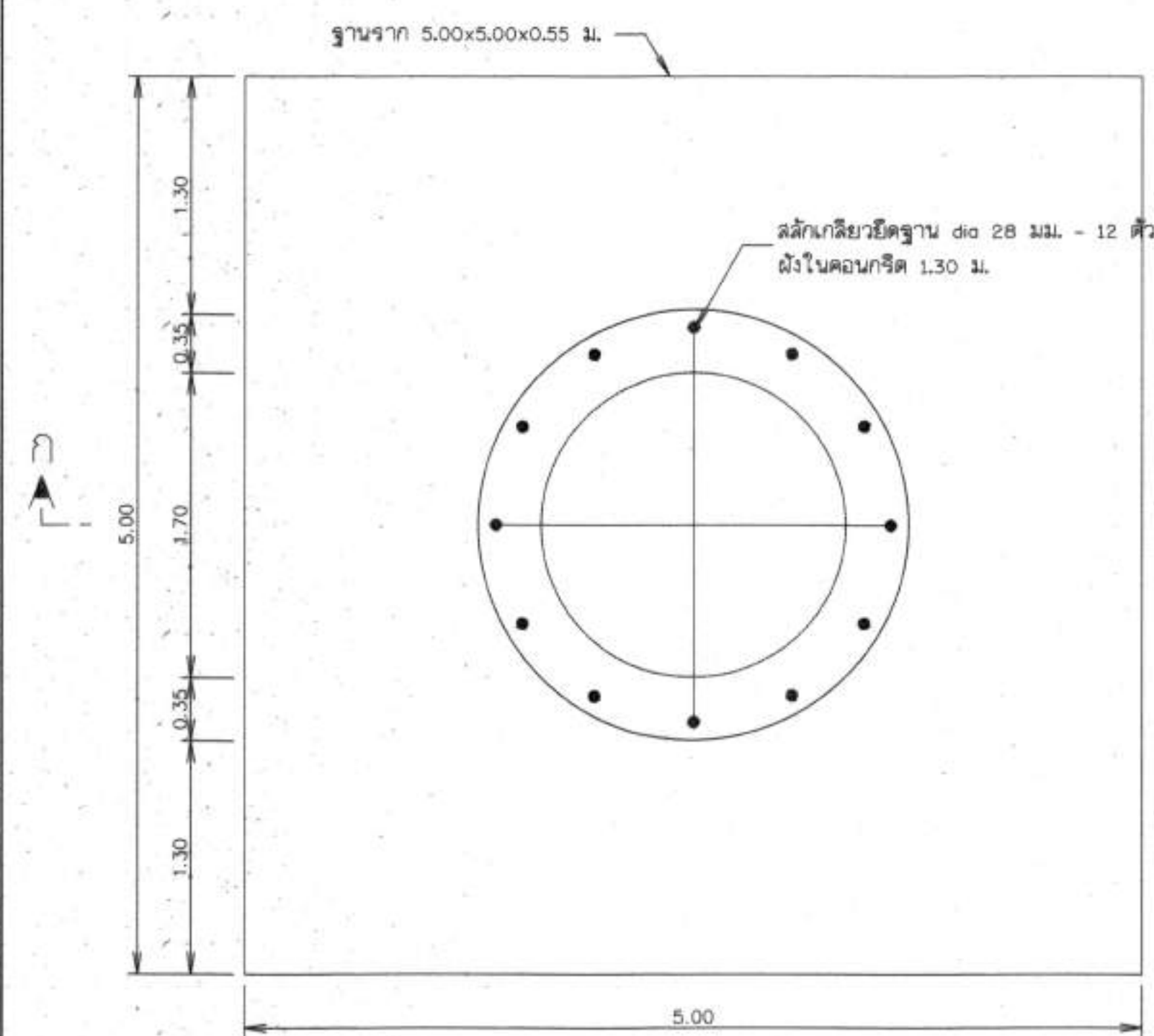
แปลน ฐานรากหอถังสูง (แบบฐานแพ)
