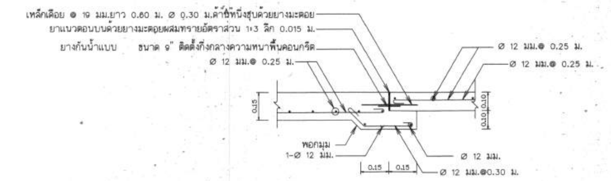
แบบขยาย A-3 มาตราส่วน 1:25
