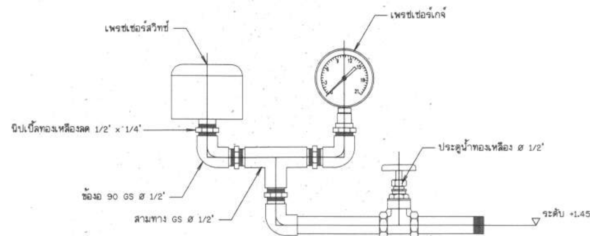
แบบขยายสิทธิ์ควบคุมและกำจัดความดัน
