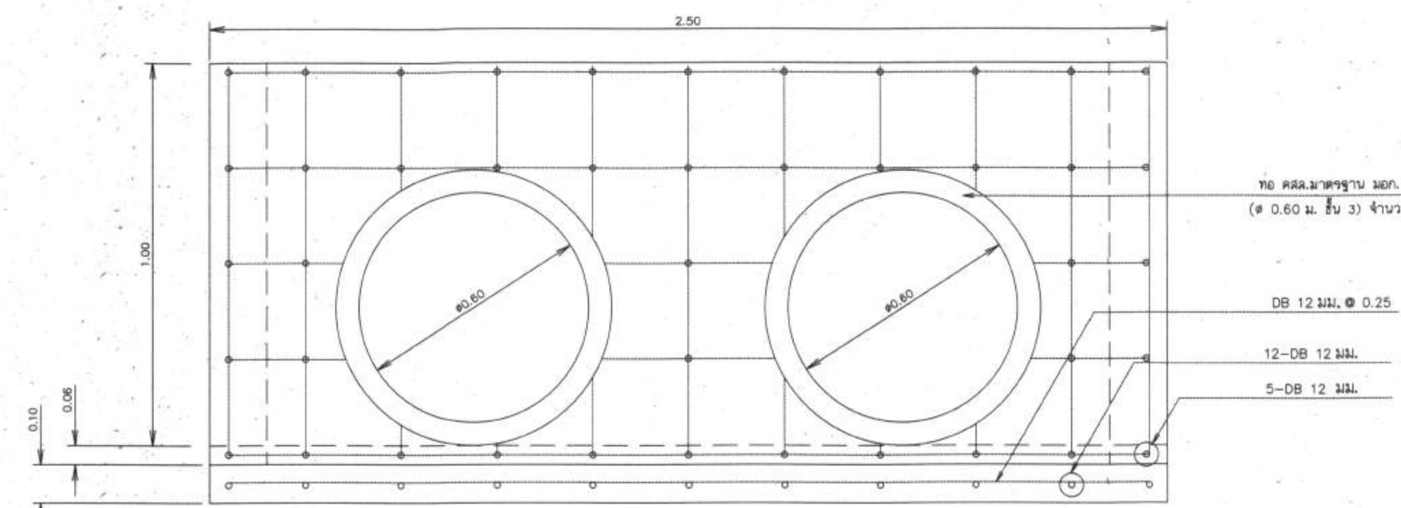
รูปตัด 2 - 2 (+ แผง คลส.) มาตราส่วน 1:10
