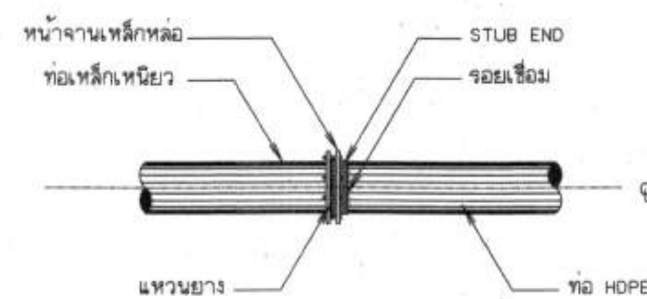
2. การบรรจุท่อเหล็กเหนียวกับท่อ HDPE ไม่แสดงมาตราส่วน
