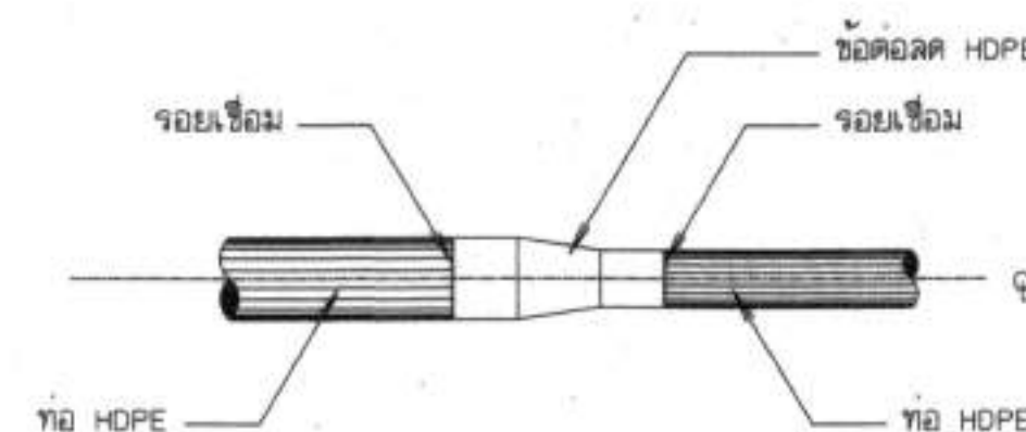
3. การบรรจุท่อ HDPE กับข้อต่อท่อ HDPE ไม่แสดงมาตราส่วน
