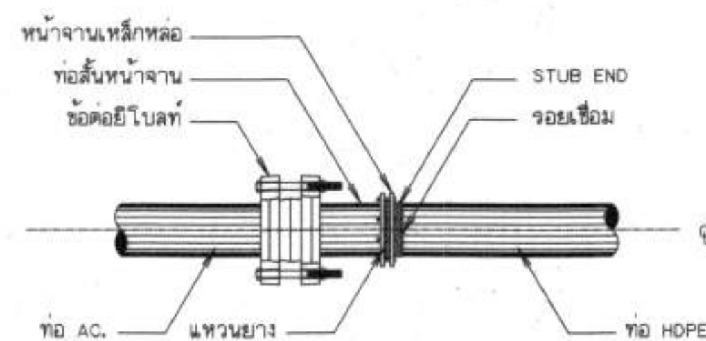
4. การบรรจุท่อ AC. กับท่อ HDPE ไม่แสดงมาตราส่วน
