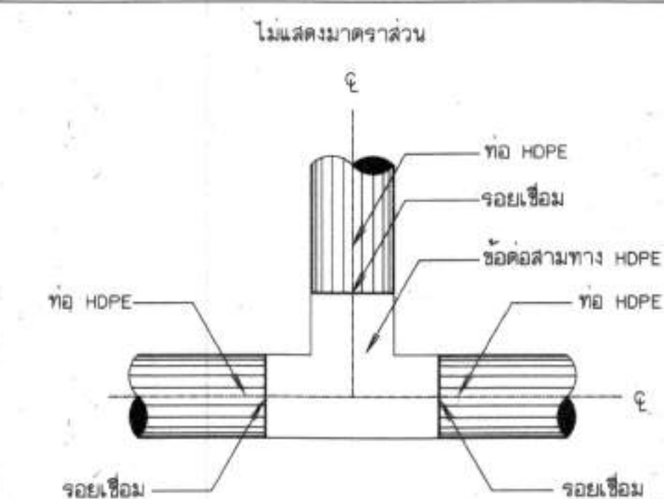
10. การบรรจุท่อสามทาง HDPE กับท่อ HDPE
