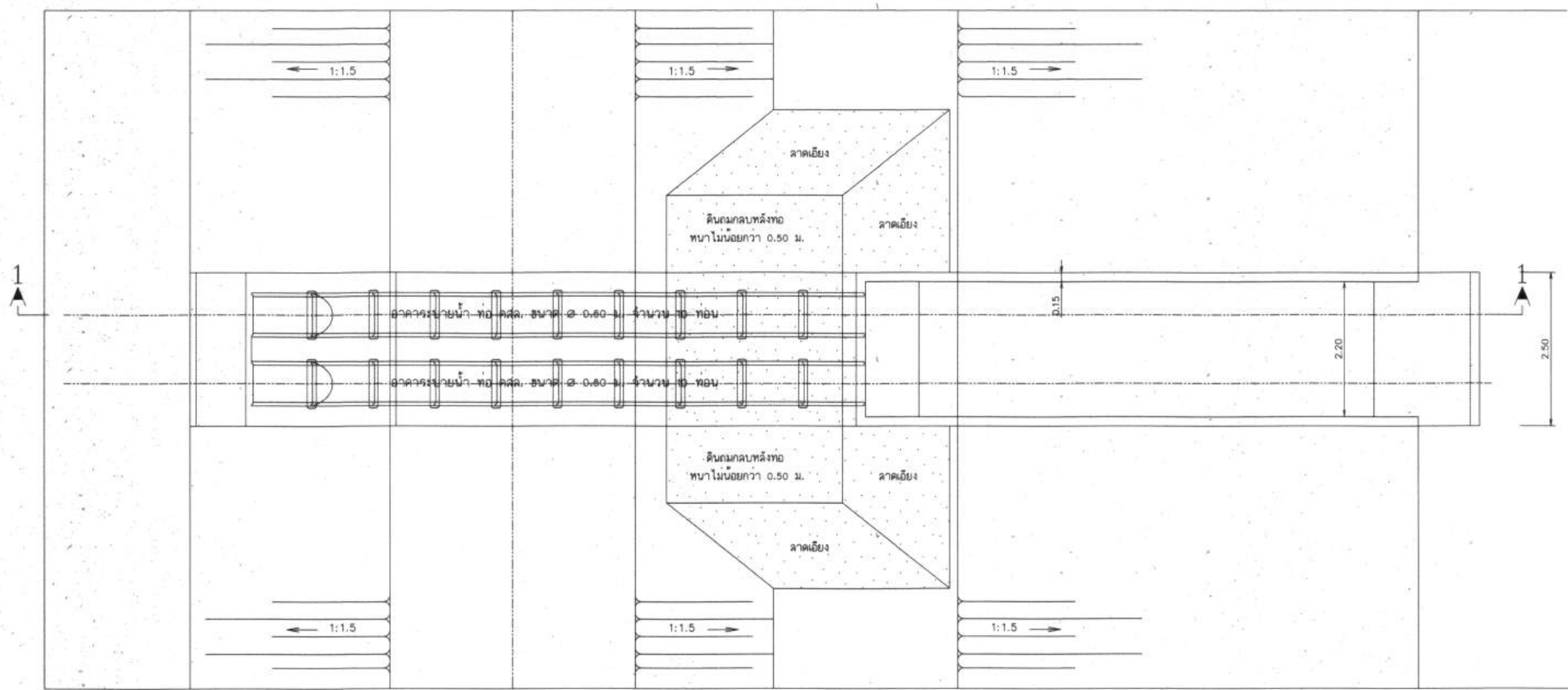
แปลนวางท่อ คล. ขนาด 0.60 ม. มาตราส่วน 1:50
