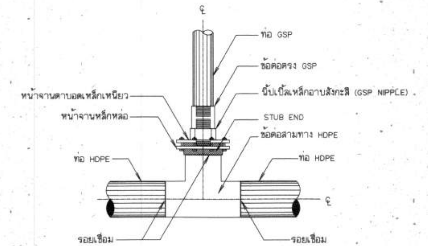
8. การบรรจุท่อสามทาง HDPE กับท่อ GSP แบบข้อต่อ
