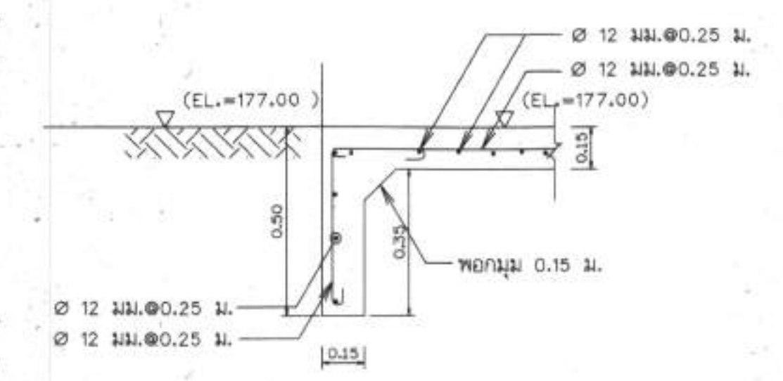
แบบขยาย A-1 มาตราส่วน 1:25
