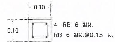
แบบขยายเหล็กเสริมหลักบ่อแนวท่อ มาตราส่วน 1:15
