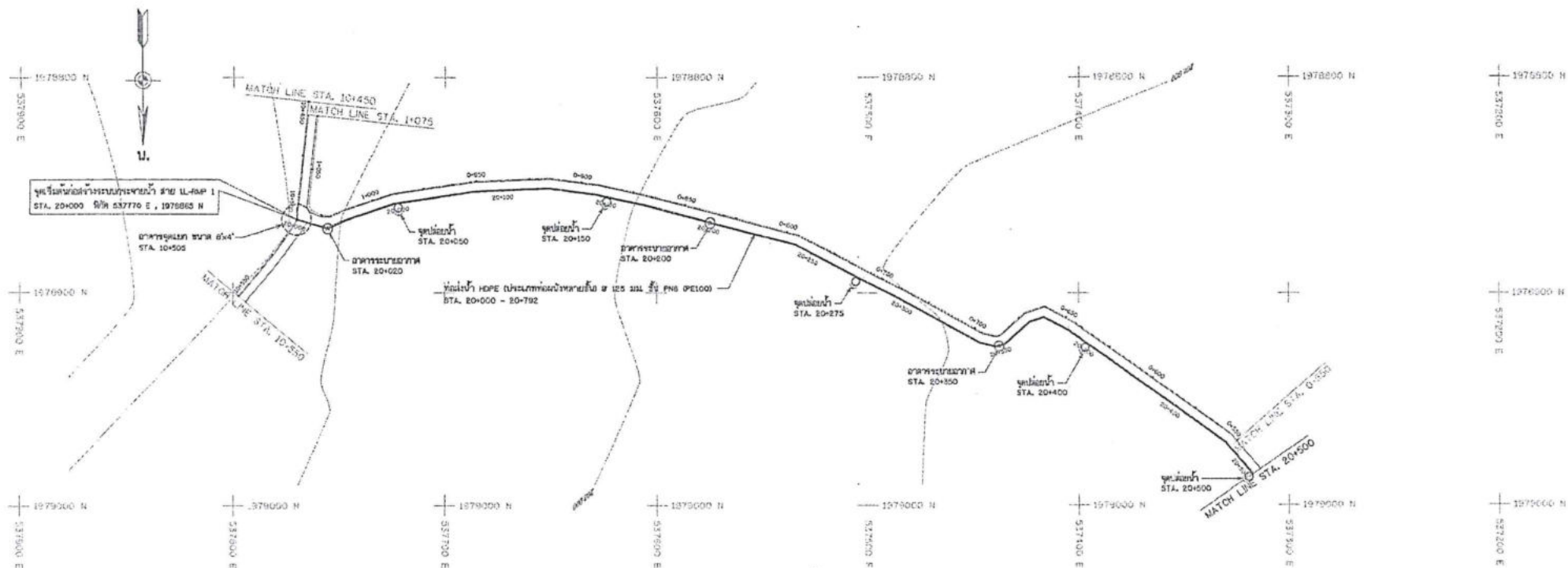
แปลนทั่วไประบบกระจายน้ำ สาย 1L-RMP 1 มาตราส่วน 1:10,000
