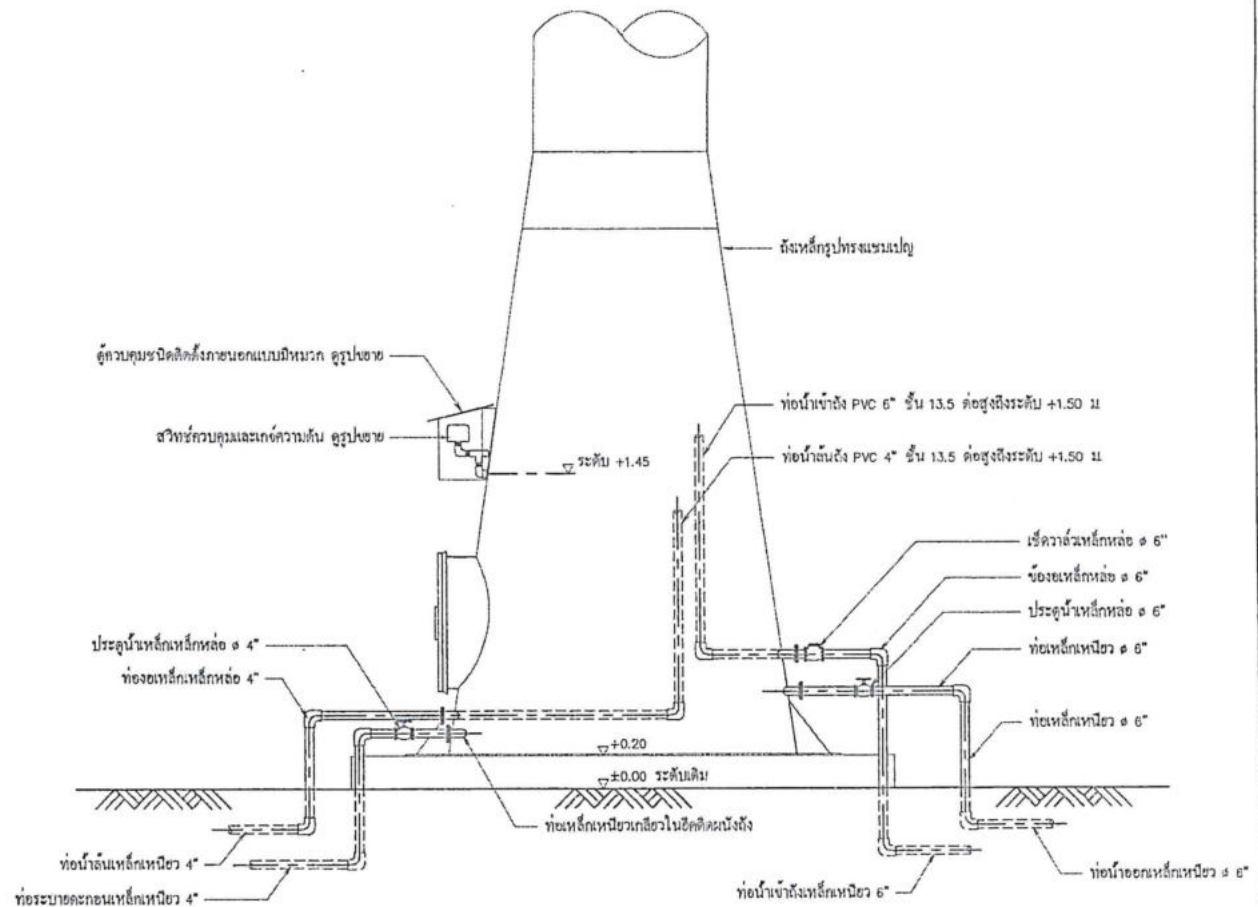
แบบแสดงการเดินท่อในหอดึงสูง ไม่แสดงมาตราส่วน
