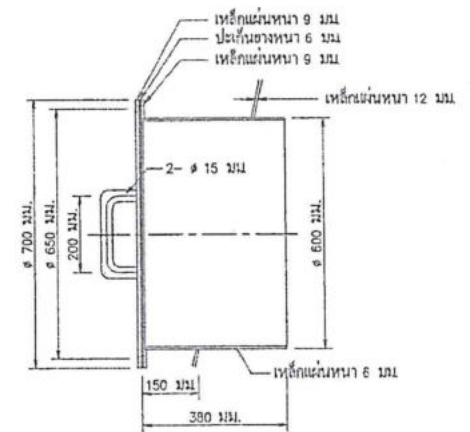
ภาพขยายทางคนเข้า-ออก "2" ไม่แสดงขนาดส่วน
