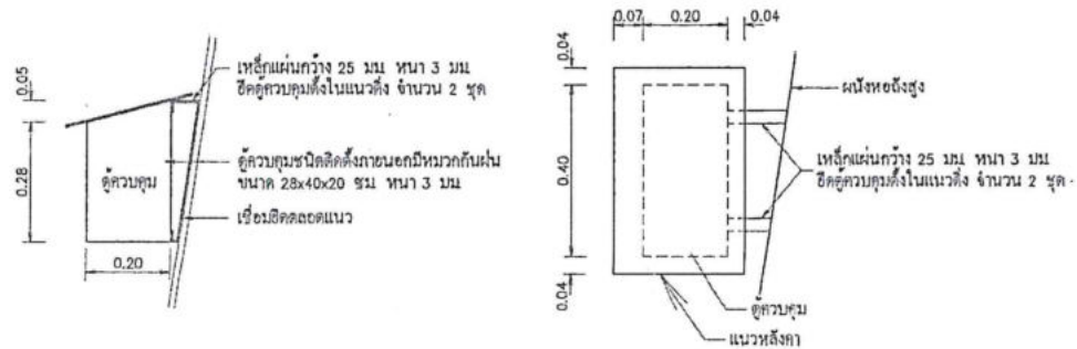
แบบขยายตุ้มนกตึง ไม่แสดงขนาดส่วน
