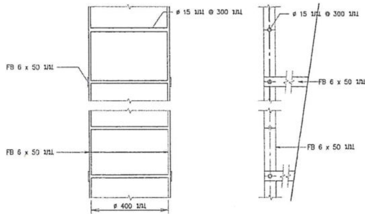
ภาพขยายบันได "1" ภายในห้องถึงเหล็กเก็บน้ำ ไม่แสดงขนาดส่วน
