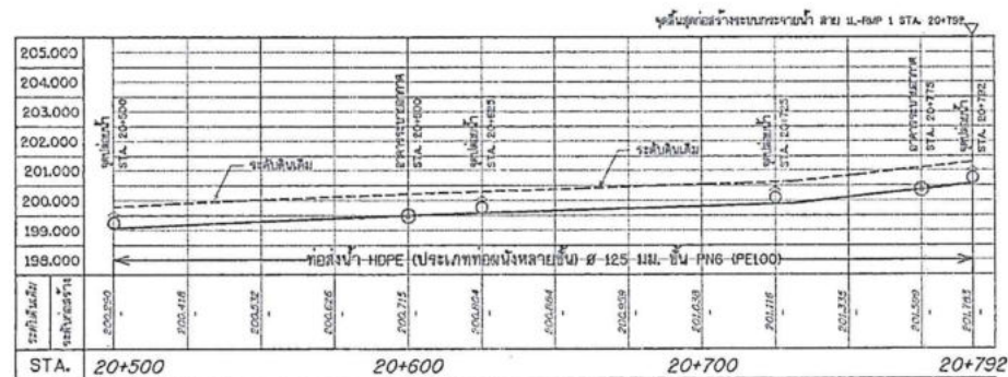
รูปตัดตามแนวาวระบบกระจายน้ำ สาย 1L-RMP 1 มาตราส่วน 1:1,000
