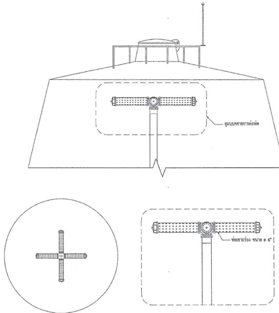
ภาพขยายการติดตั้งท่อกระจายน้ำ HDPE หรือ PVC โมดูลขนาดสามส่วน
