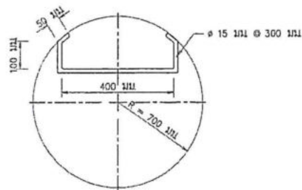
ภาพขยายบันได "2" ภายในส่วน Column ไม่แสดงขนาดส่วน
