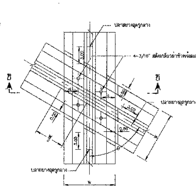
การต่อพาดทับกันไม่ทำมุมฉาก ไม่แสดงขนาดส่วน
