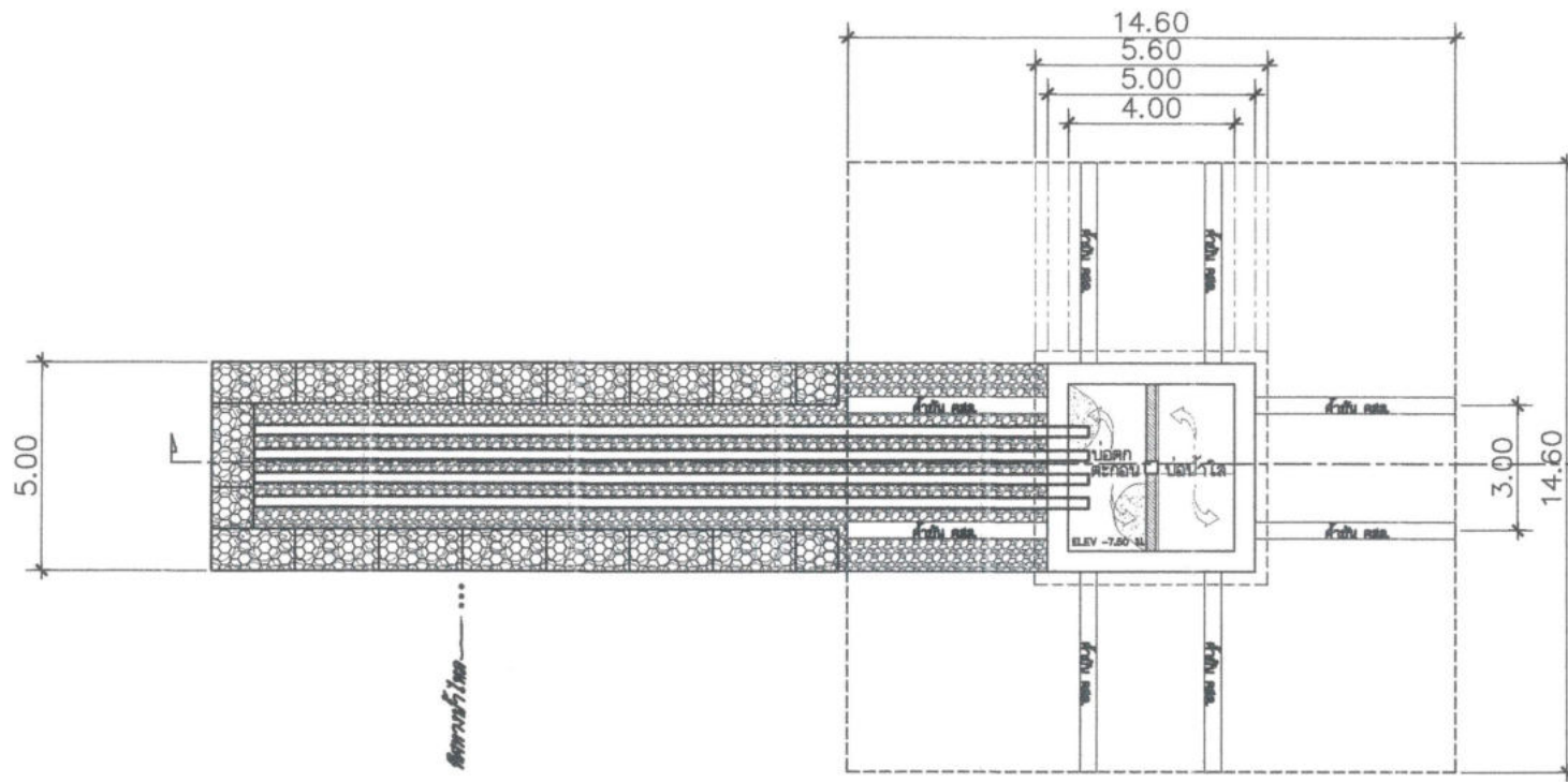
แปลนแสดงทางน้ำเข้าสู่อาคารบ่อสูบล
