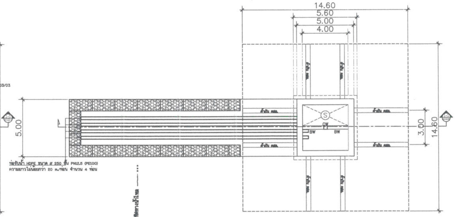
แปลนแสดงโครงสร้างคานและพื้นสำหรับบ่อน้ำ
