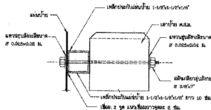
รูปตัดขยายการยึดแผ่นป้ายและเสา
