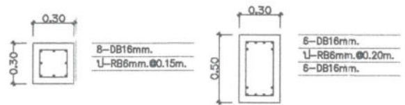
รูปตัดเล้า CW
