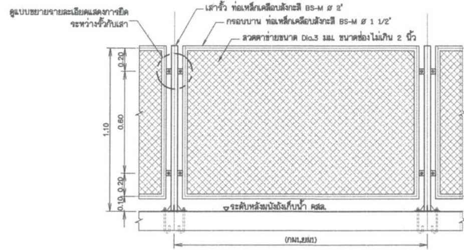
แบบขยายราวกันตก สำหรับบันไดน้ำ คสล. แบบไม่มีฝ้าปิด
