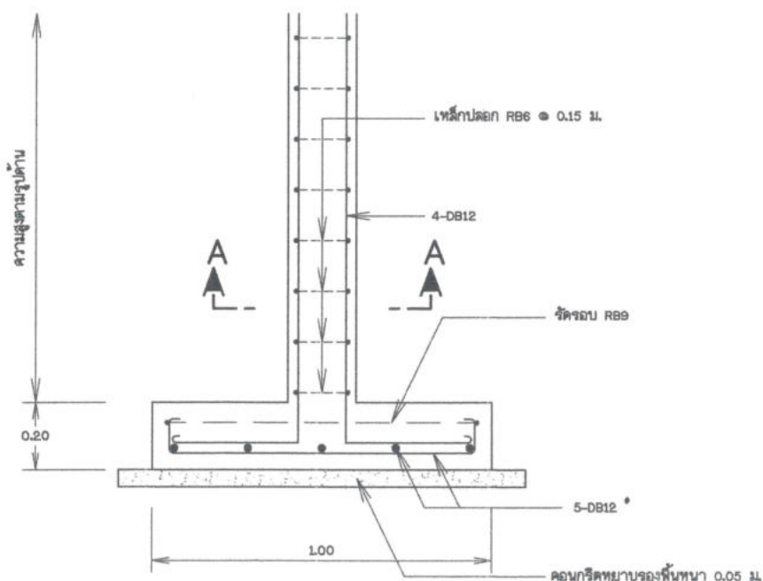
รูปตัดฐานราก F1
