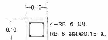
แบบขยายเหล็กเสริมหลักบ่อแก้ว มาตราส่วน 1:15
