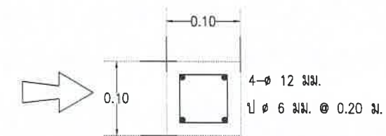
ขยายเสাপ้ายใต้ป้าย - หัวเสา SCALE 1:10
