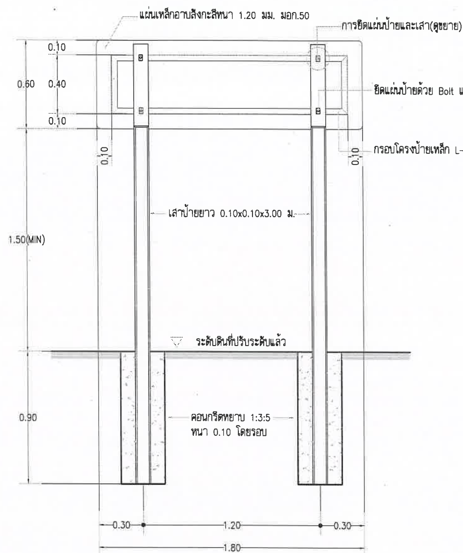
แสดงรูปด้านหลังแนะนำโครงการ SCALE 1:25
