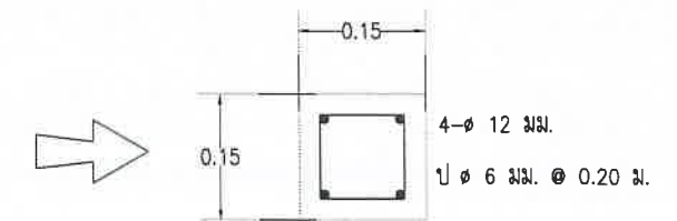
ขยายเส้าป้ายได้ป้าย - หัวเส้า SCALE 1:10
