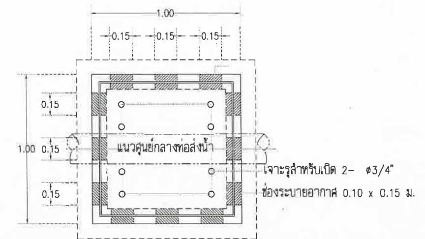
แปลนอาคารท่อระบายอากาศ 1:25
