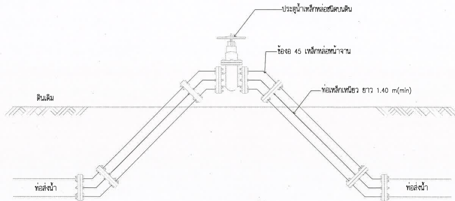
แปลนอาคารประตุน้ำบนดิน SCALE 1:25
