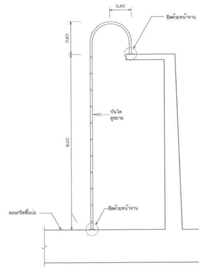
บันไดเหล็ก ไม่แสดงมาตราส่วน
