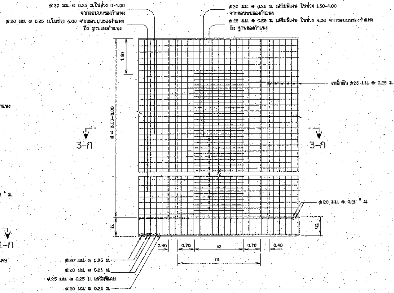
รูปตัด 3-ก (พื้นคานล่าง)
