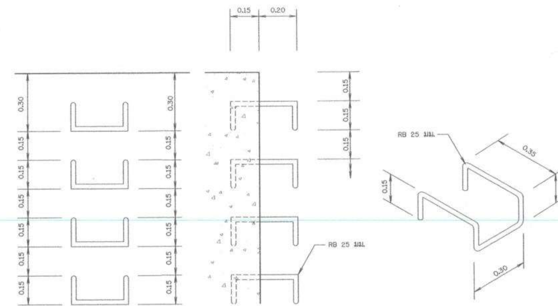
รูปขยายบันไดลิง
