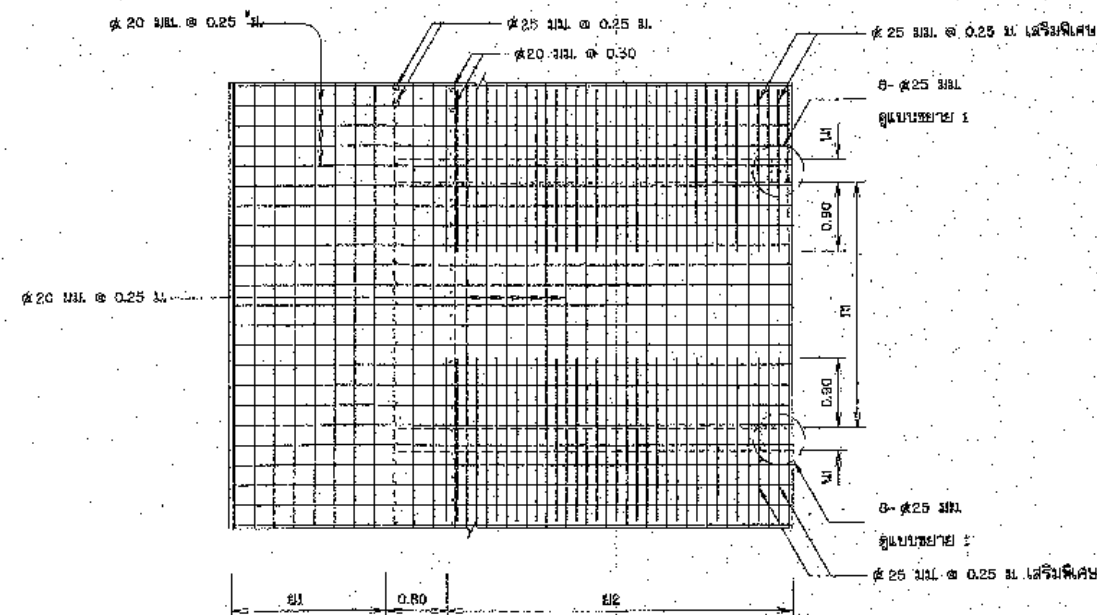
รูปตัด 4-ก (พื้นค้ำยัน)
