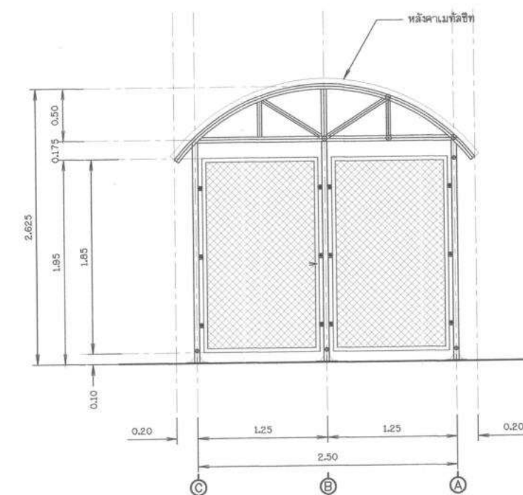
รูปด้าน 4
