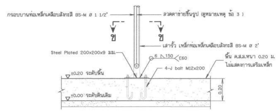
รูปขยายฐานรากโครงสร้างรับแผง F1 (ต่อม่อ คสล. หล่อสำเร็จรูปพร้อมติดตั้ง) ไม่แสดงมาตราส่วน
