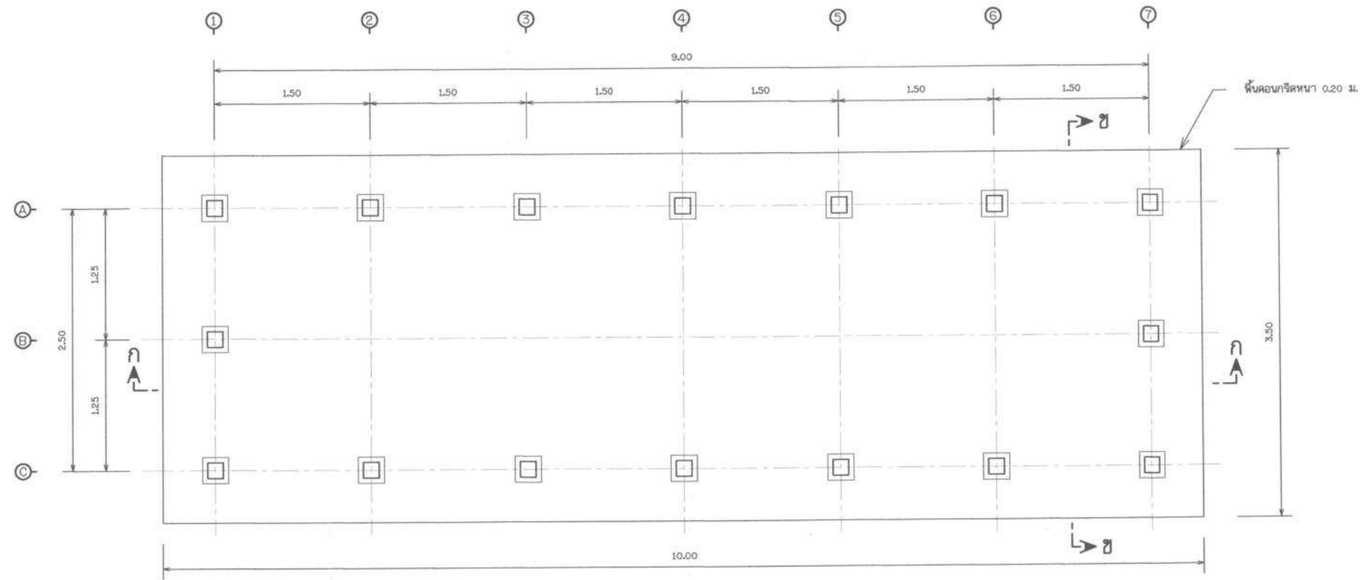
แปลนแบบ
