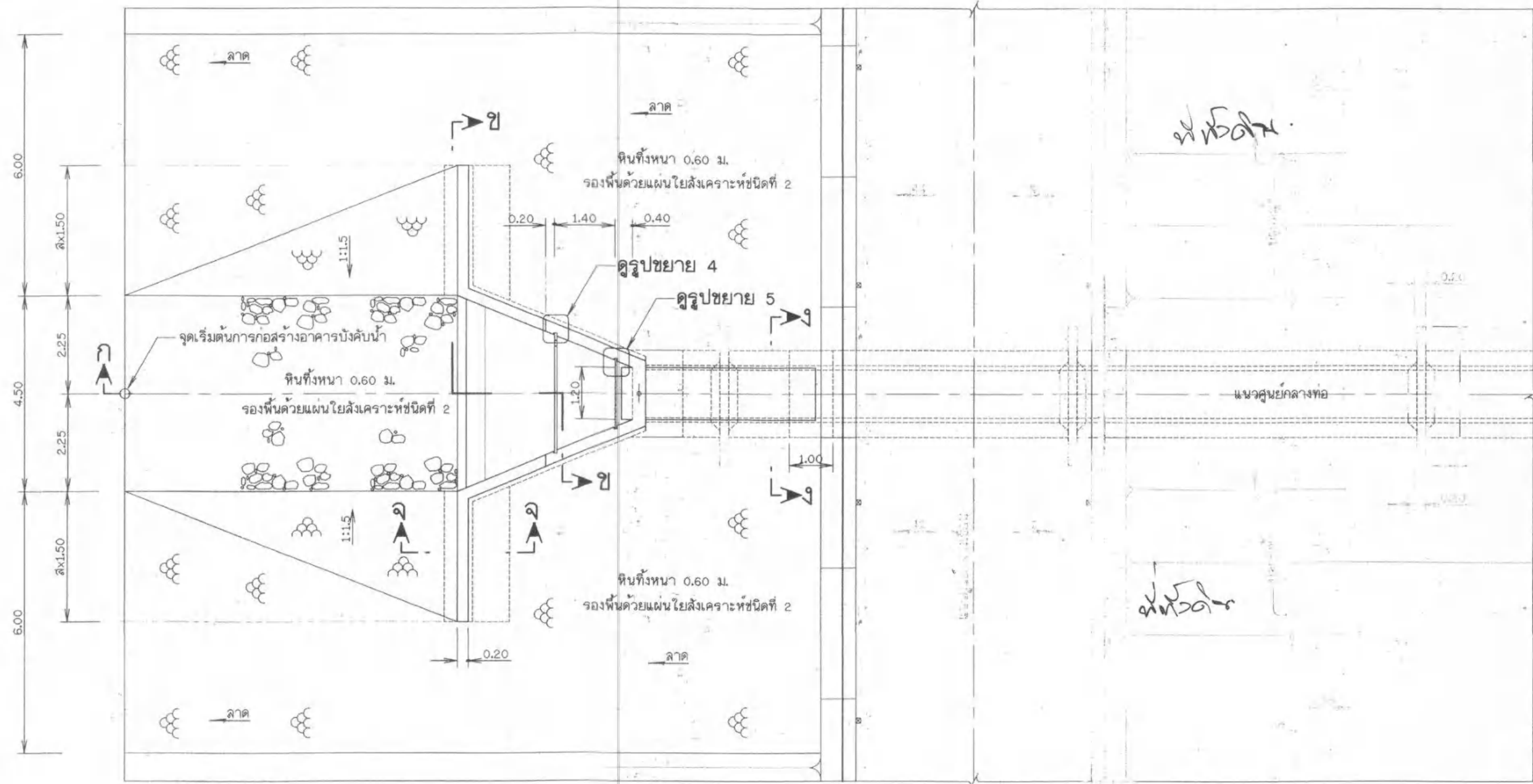
แปลนอาคารบังคับน้ำแบบฝาท่อ มาตรฐาน 1:75
