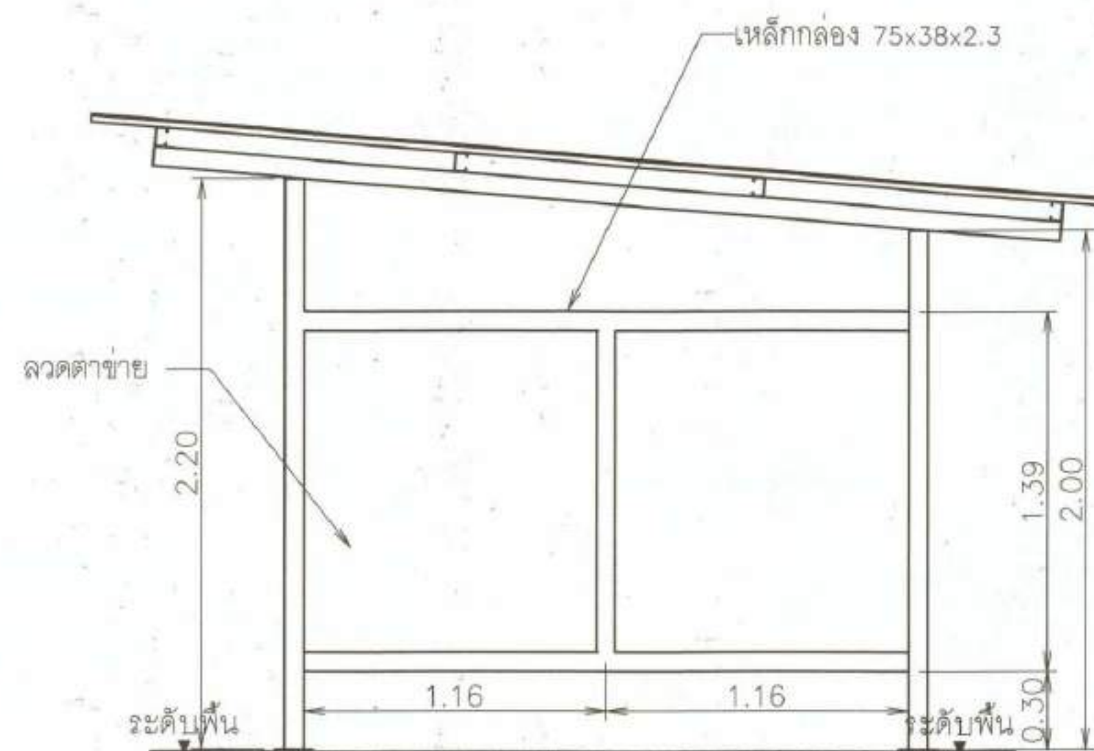
ด้านข้าง 2
