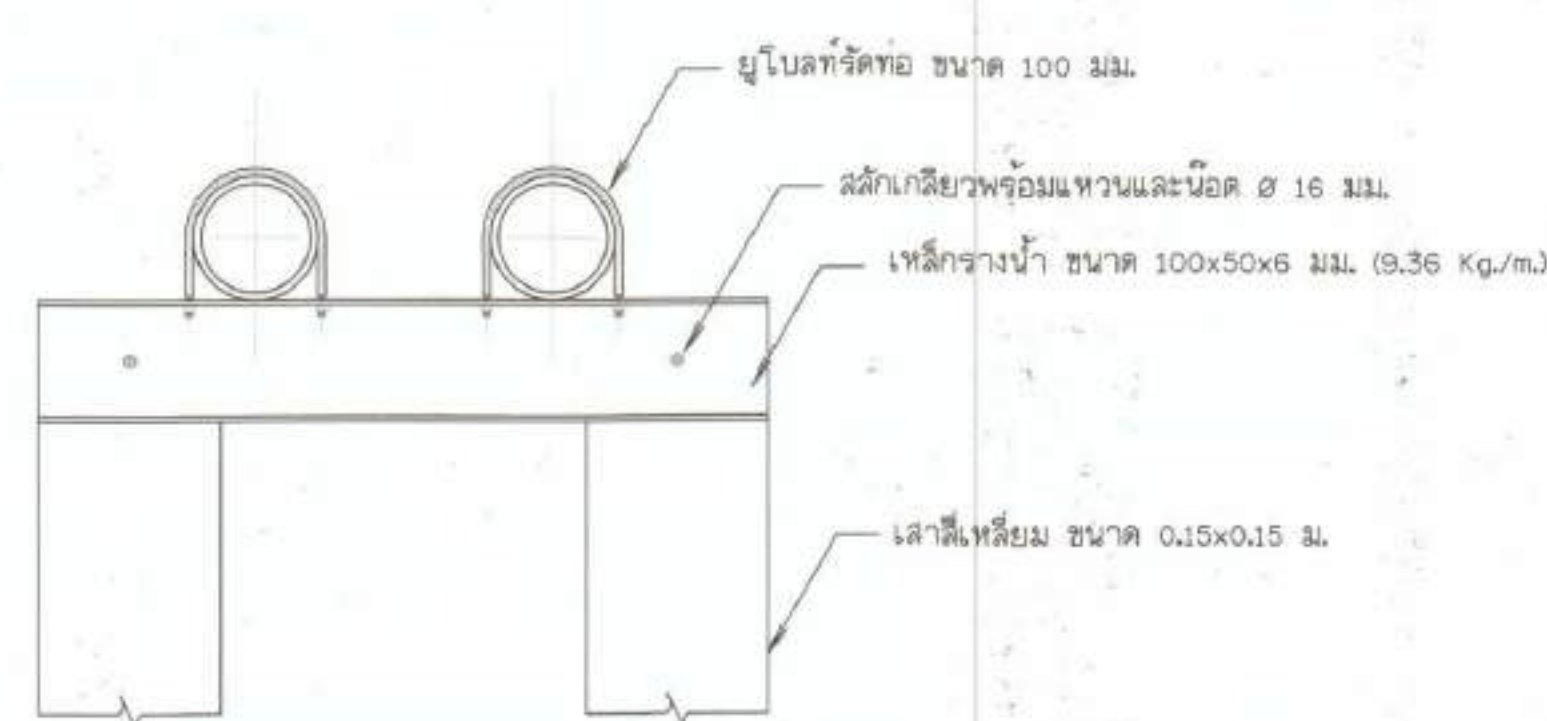
รูปด้านบน
