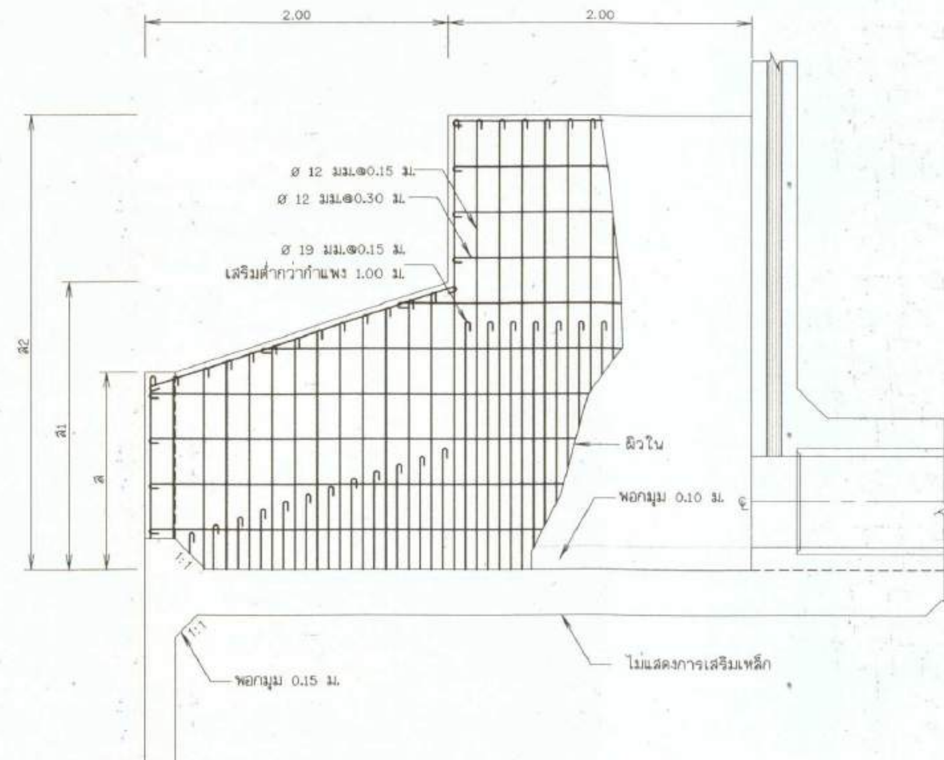
แสดงการเสริมเหล็กด้านข้างอาคารเหนือหน้า มาตราส่วน 1:25
