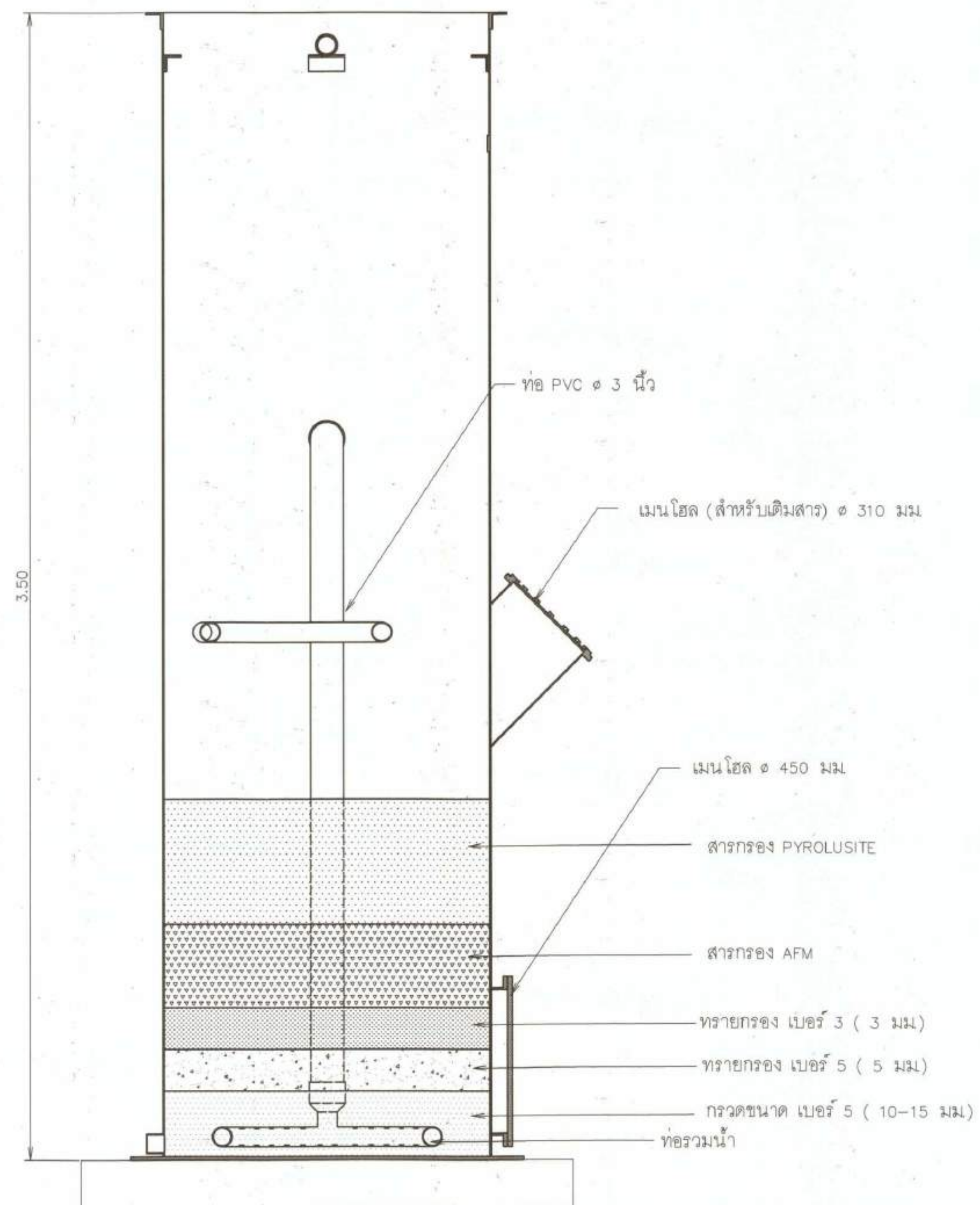
A-A(1:1)
