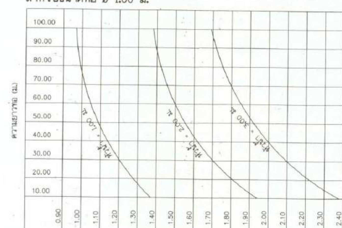
สำหรับขนาดท่อ Ø 1.00 ม.
