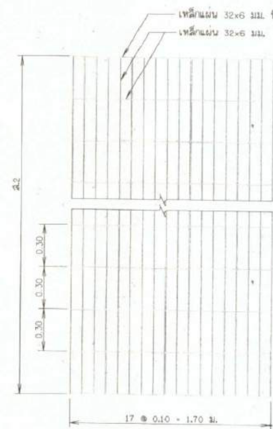
รูปขยายตะแกรงกันสวะ
