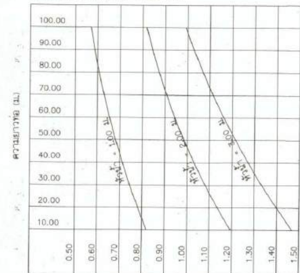
สำหรับขนาดท่อ Ø 0.60 ม.
