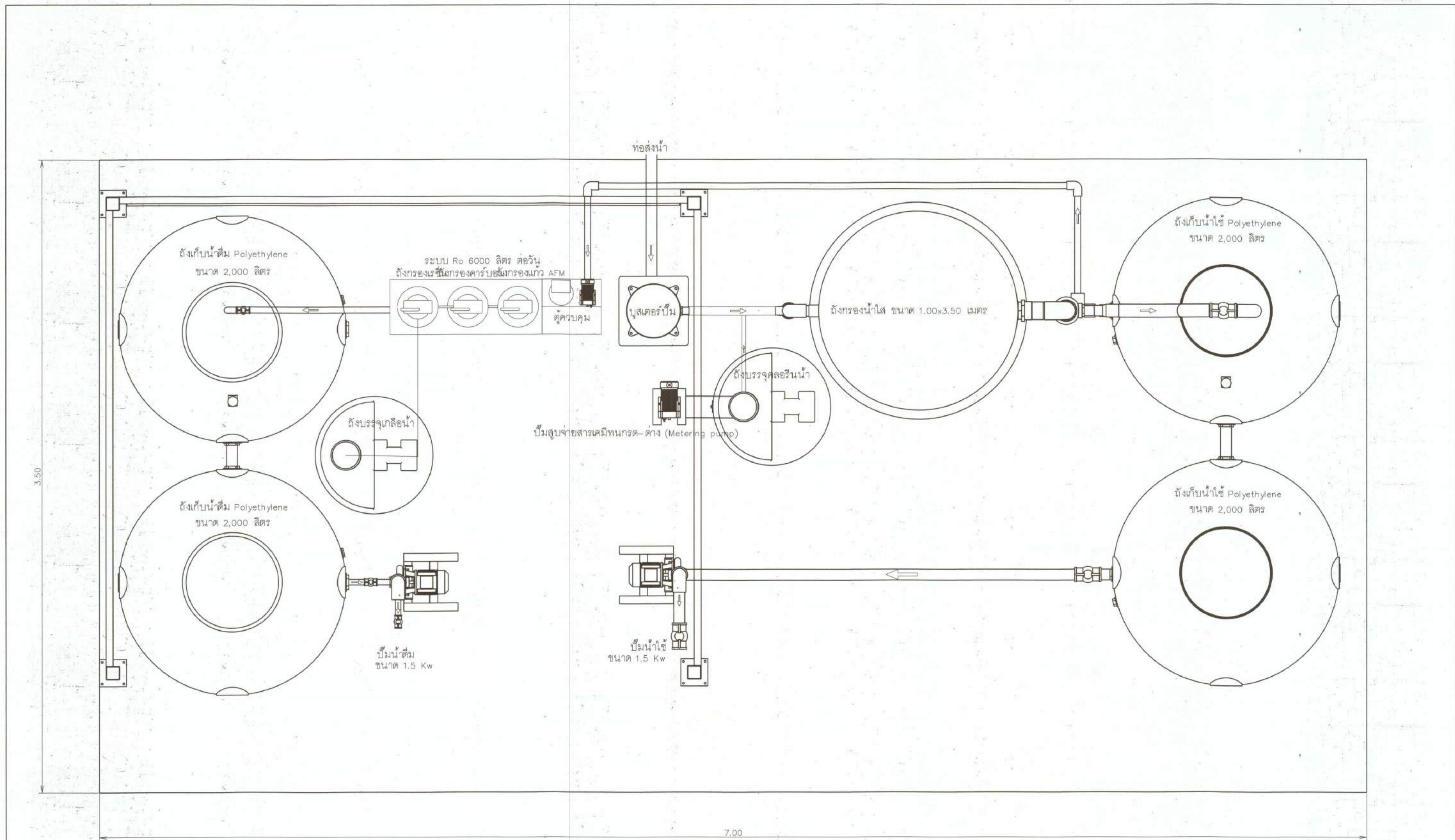
แบบแสดงแผนผังการติดตั้งระบบผลิตน้ำดื่มสะอาด มาตราส่วน 1:10
