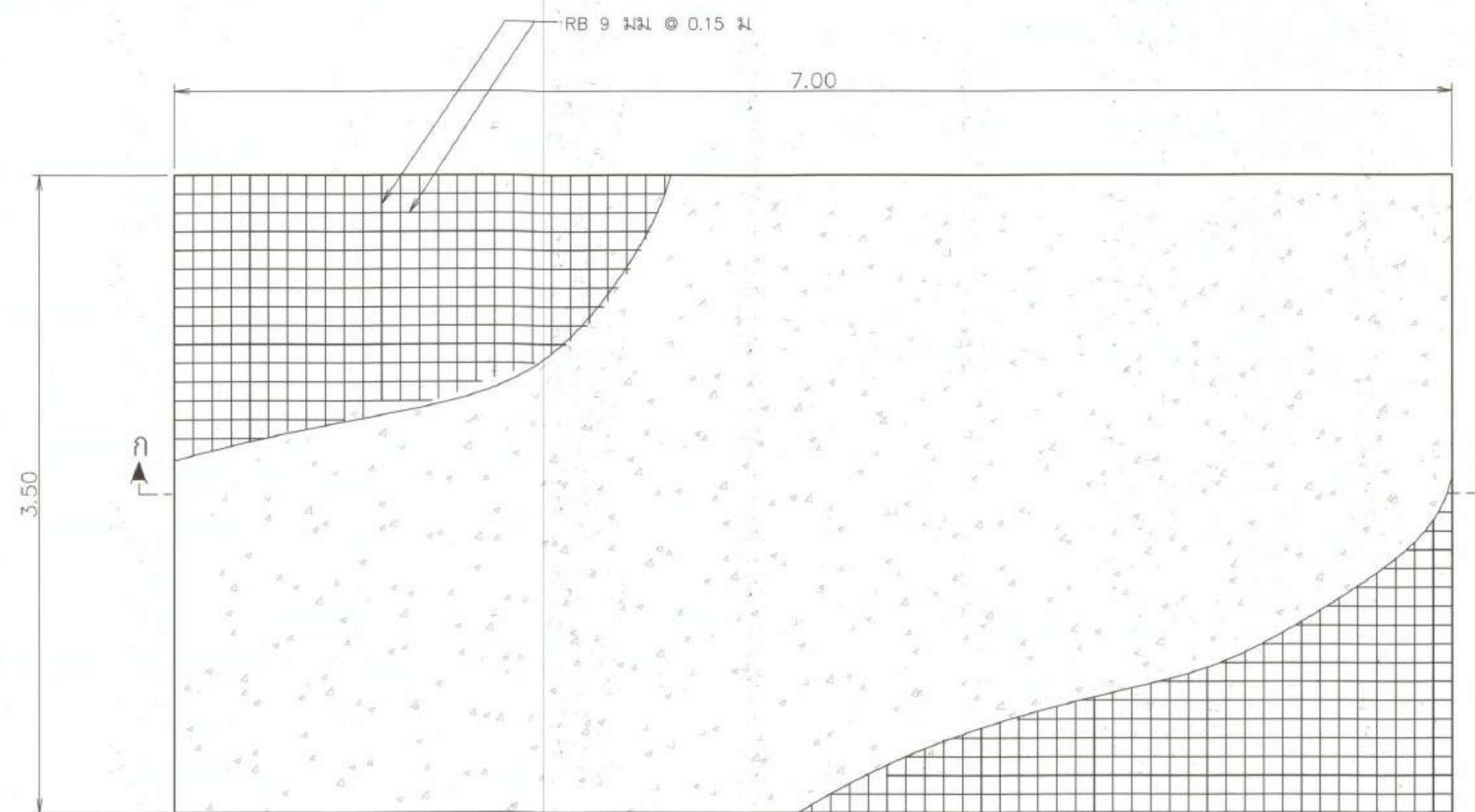
แบบฐานราก มาตราส่วน 1:20
