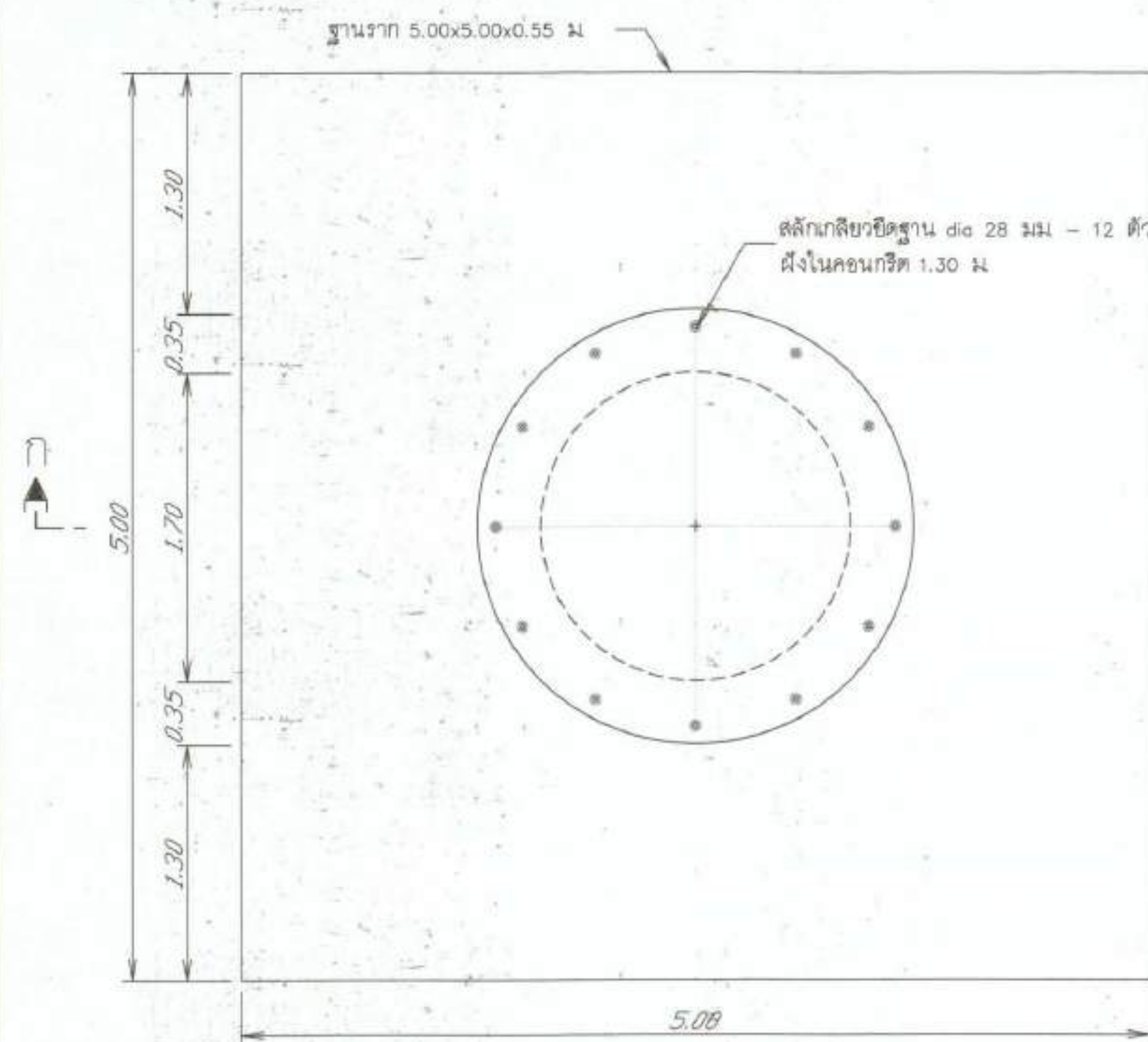
แปลน ฐานรากหอดังสูง (แบบฐานแพ)
