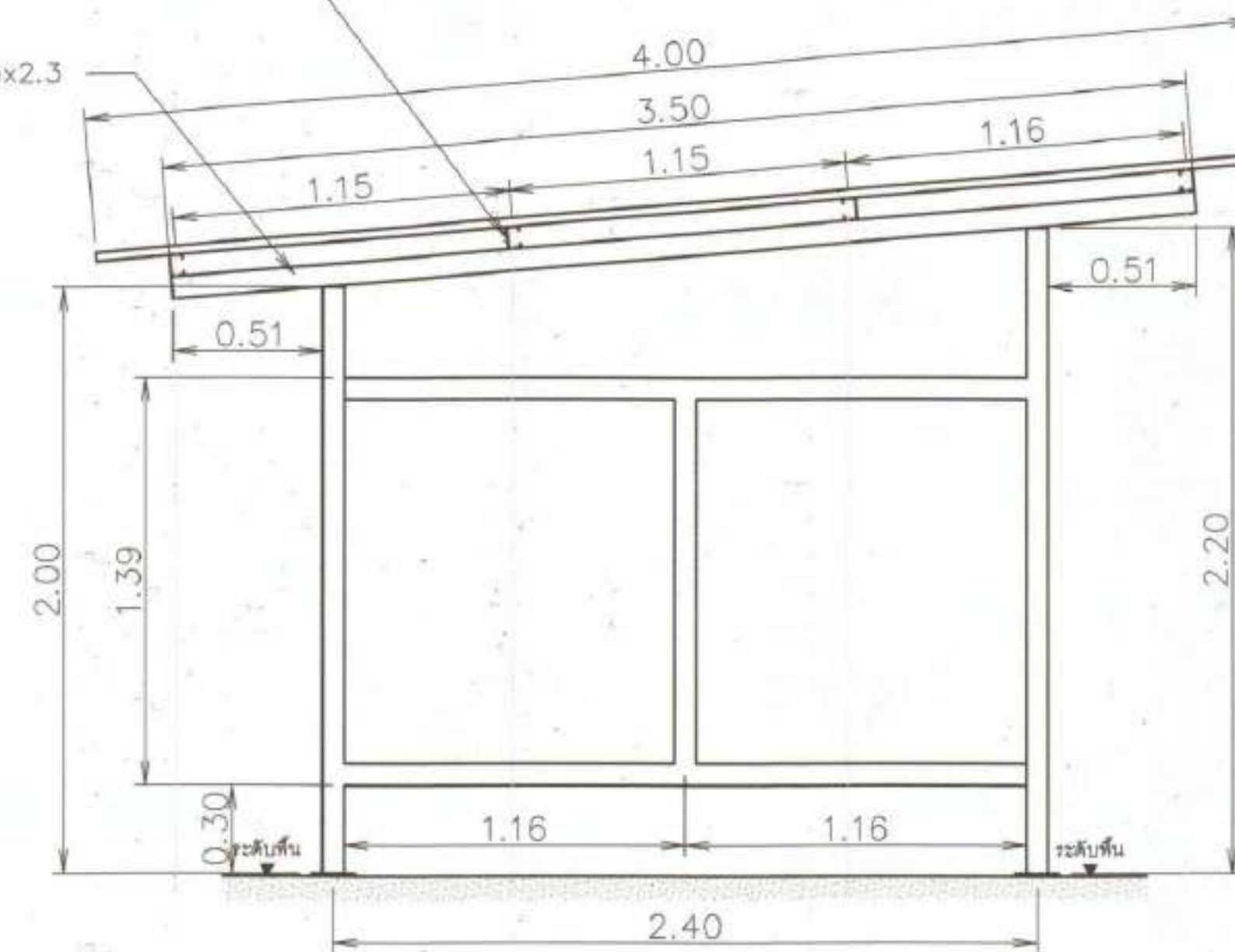
ด้านข้าง 1
