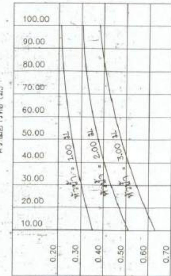
สำหรับขนาดท่อ Ø 0.40 ม.
