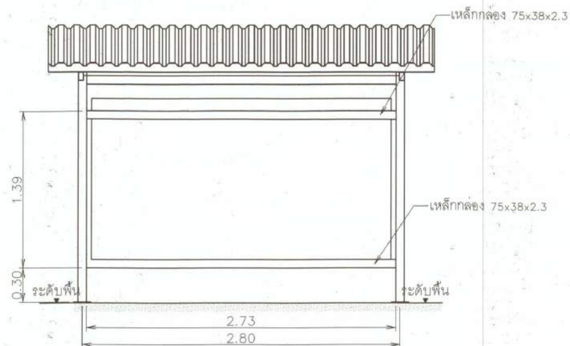
ด้านหลัง
