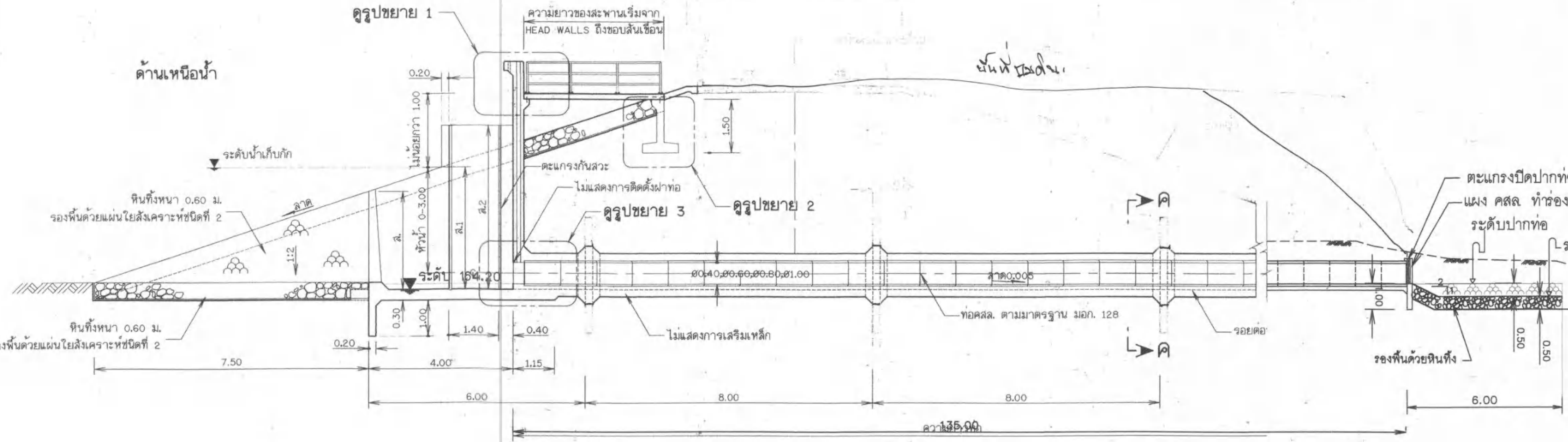
รูปตัด ก - ก มาตรฐาน 1:75
