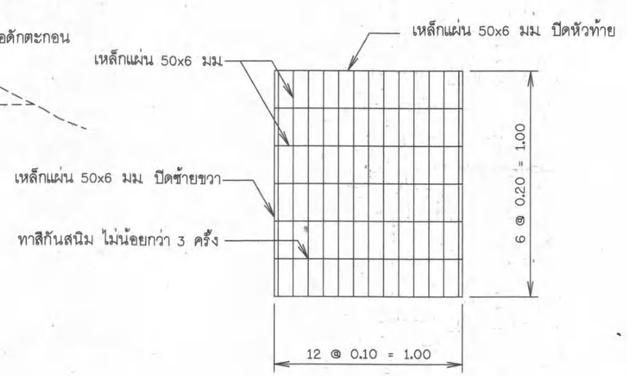
รูปขยายตะแกรงกันสวะ มาตรฐาน 1:25
