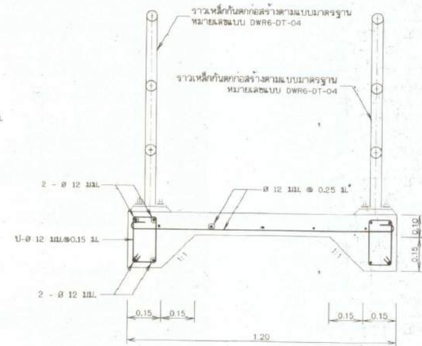
รูปตัด ง - ง
