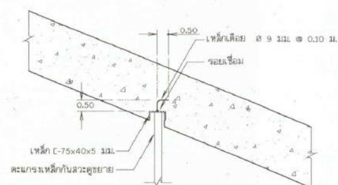
รูปขยาย 5 ร่องใส่ตะแกรงกั้นสวะ มาตราส่วน 1:10
