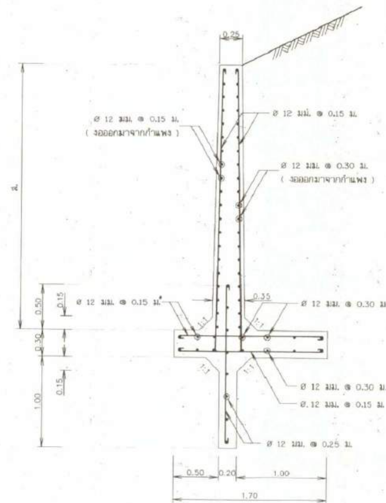
รูปตัด จ - จ
