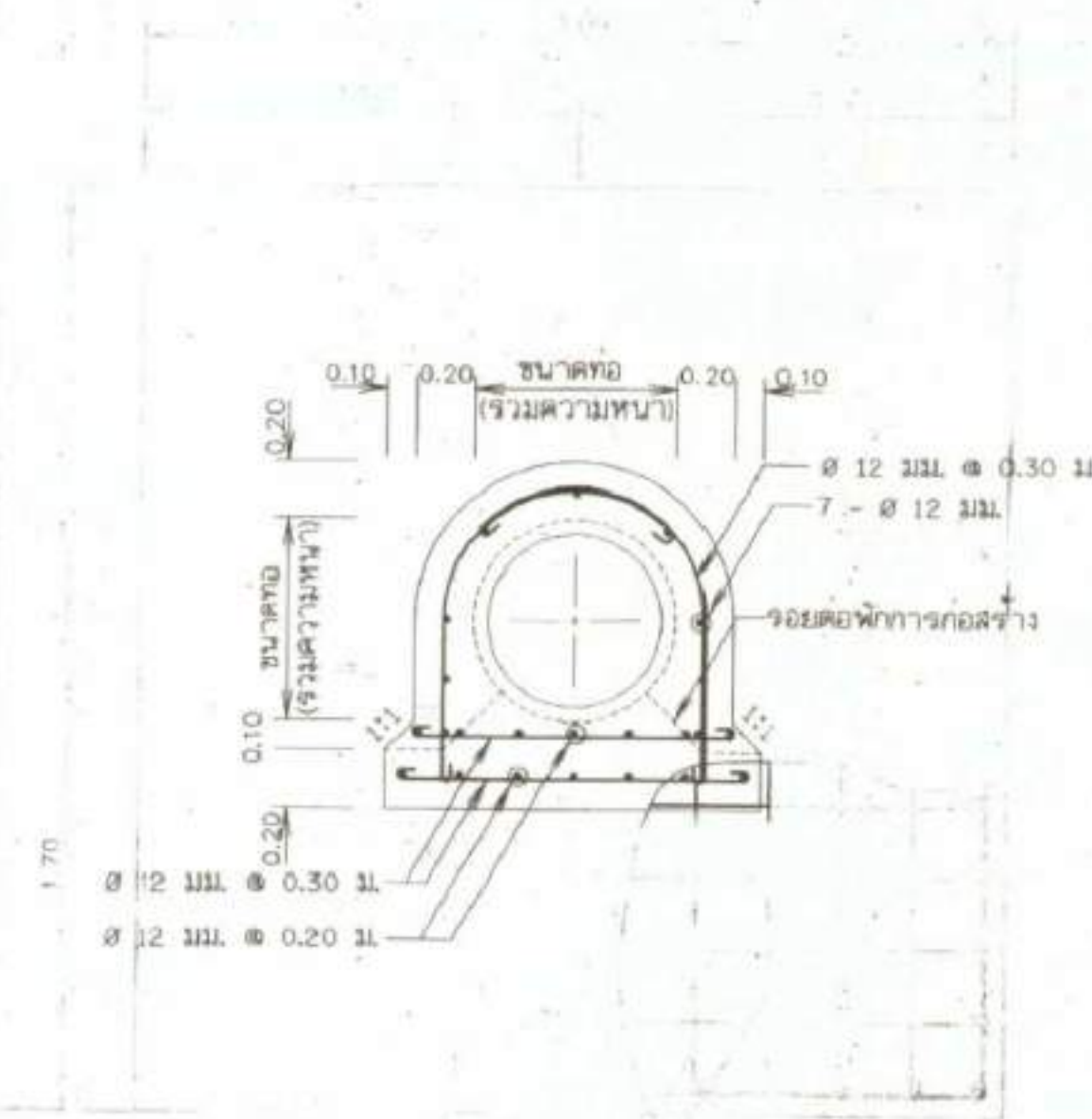
รูปตัด ค - ค
