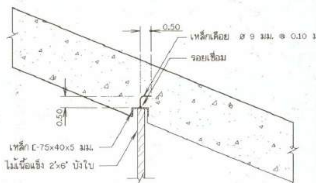
รูปขยาย 4 ร่องใส่ท่อท่อน้ำ มาตราส่วน 1:10
