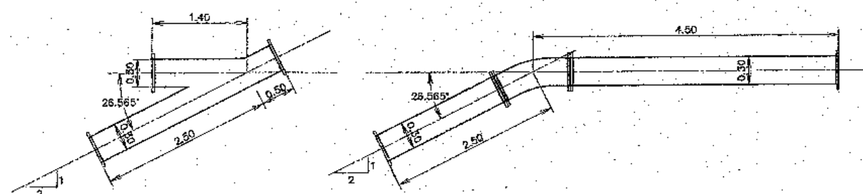
รายละเอียดท่อวัดน้ำ ลาด 1:2 มาตราส่วน 1:40
