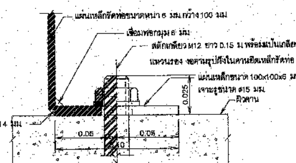
รูปตัด ง-ง
