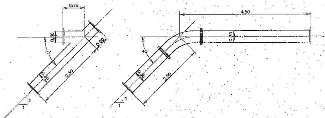
รายละเอียดท่อวัดน้ำ ลาด 1:1 มาตราส่วน 1:40
