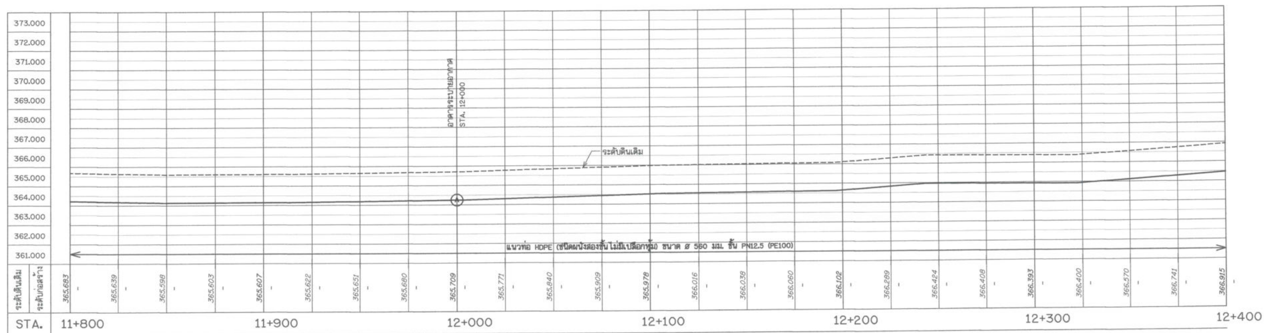
รูปตัดตามแนวยาว สาย LMP STA. 11+800 - 12+400 มาตราส่วน 1:1,000 แนวตั้ง 1:100
