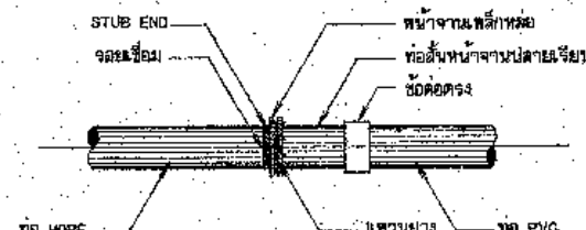
การบรรจบท่อ HDPE กับท่อ PVC.
