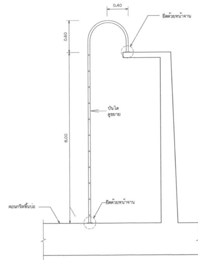
บันไดเหล็ก ไม่แสดงขนาดบางส่วน
