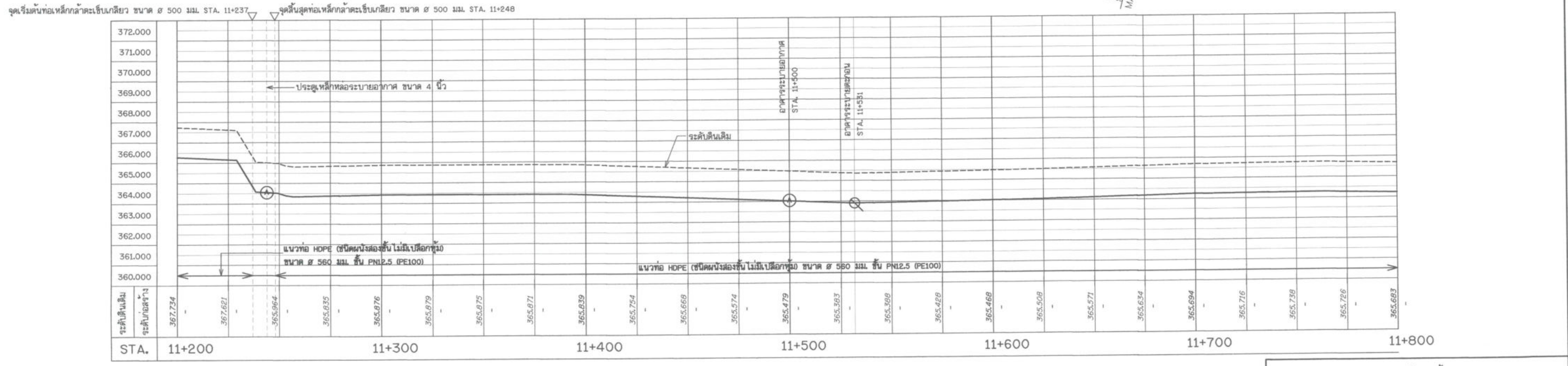
รูปตัดตามแนวยาว สาย LMP STA. 11+200 - 11+800
