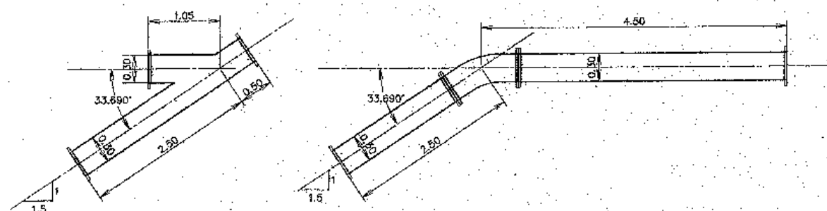
รายละเอียดท่อวัดน้ำ ลาด 1:1.5 มาตราส่วน 1:40
