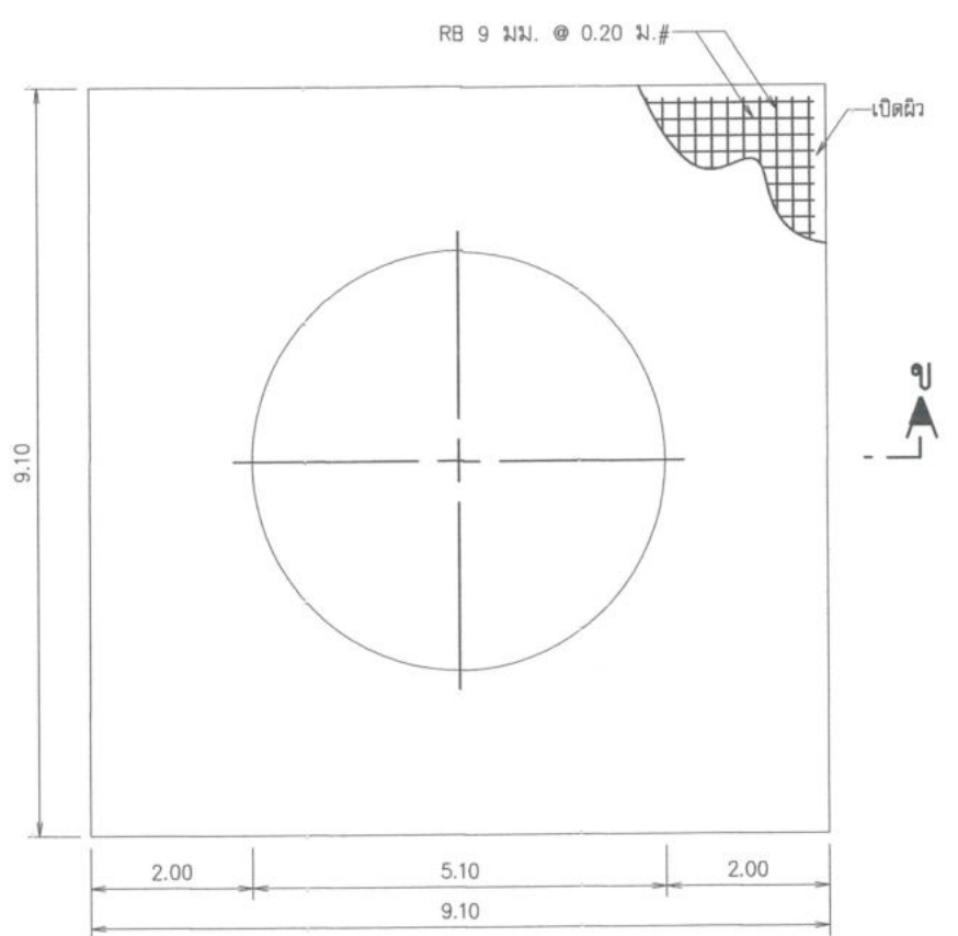
แปลนพื้นคอนกรีตเสริมเหล็ก ไม่แสดงมาตราส่วน
