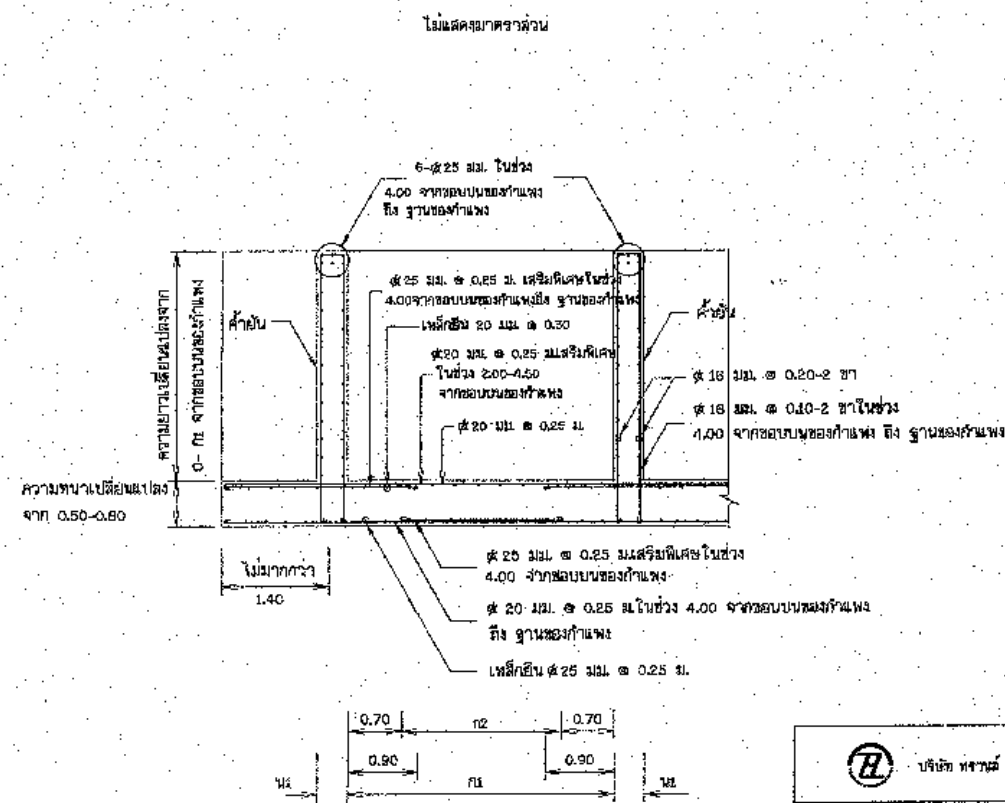
รูปตัด 4-ก
