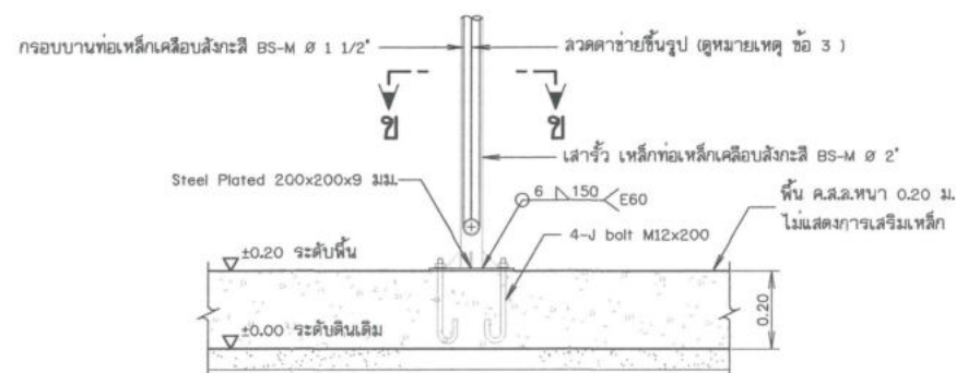
รูปขยายฐานรากโครงสร้างรับแผง F1 (ต่อม่อ คสล. หล่อสำเร็จรูปพร้อมติดตั้ง) ไม่แสดงมาตราส่วน
