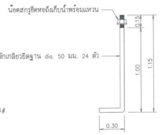
แบบขยายสลักเกลียวยึดฐาน ไม่แสดงมาตราส่วน
