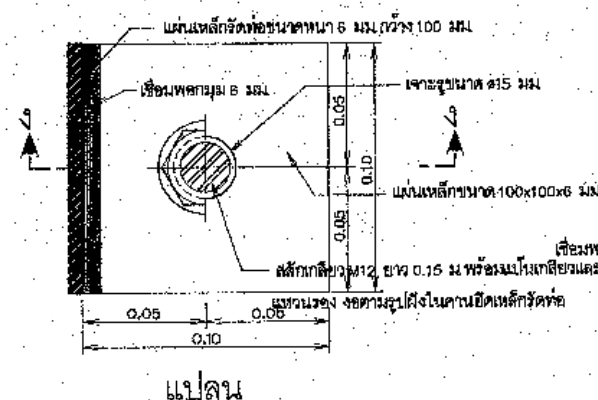
รายละเอียดแผนเหล็กยึดท่อ ในแสดงมาตราส่วน
